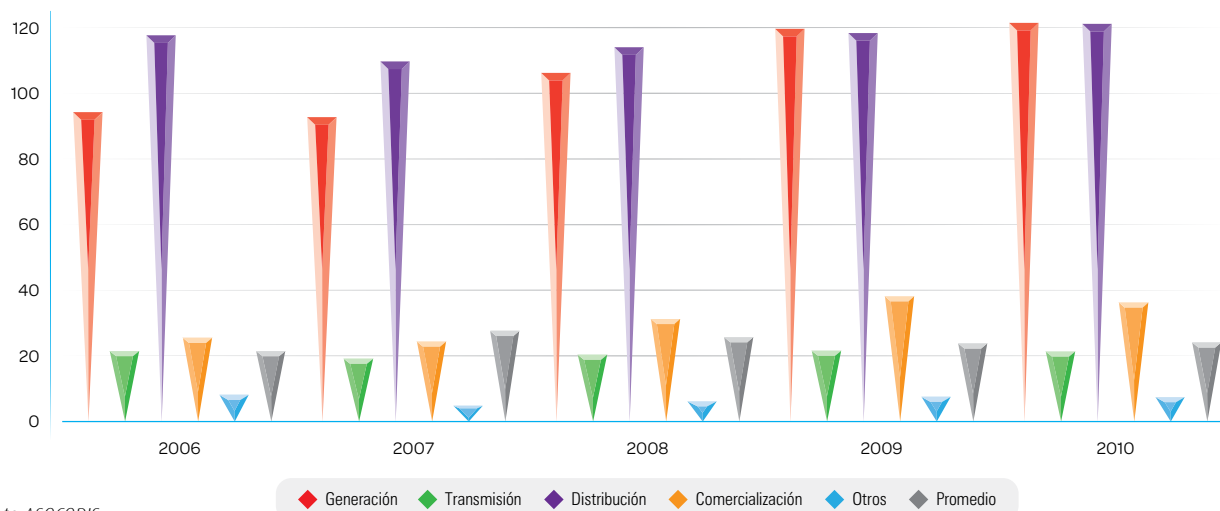
GRÁFICO 19. COSTO UNITARIO PONDERADO NIVEL 1 POR COMPONENTE $ CONSTANTES DIC 2010 $/kWh 2006 - 2010
