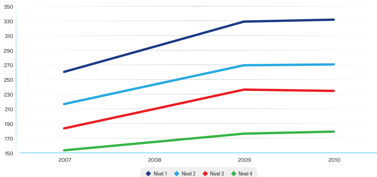
GRÁFICO 20. EVOLUCIÓN DEL COSTO UNITARIO PROMEDIO PONDERADO POR NIVEL DE TENSIÓN 2007 - 2010 $/kWh / Pesos Constantes Diciembre 2010
