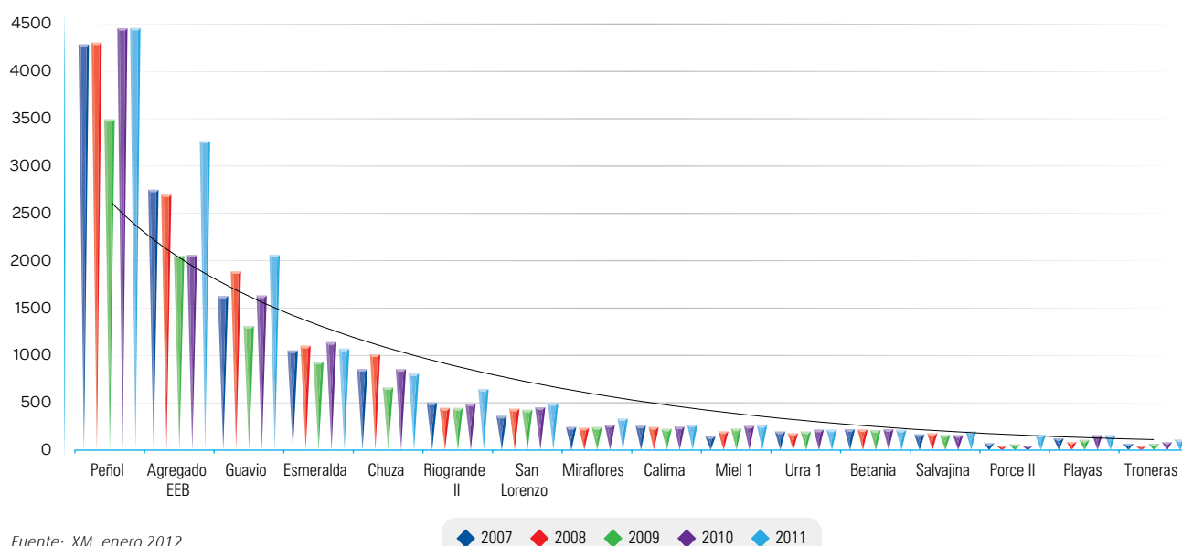
GRÁFICO 4. EVOLUCIÓN DEL VOLUMEN DE LOS EMBALSES GWh 2007 - 2011
