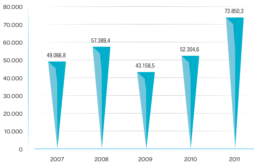
GRÁFICO 1. APORTES RIOS GWh 2007- 2011
