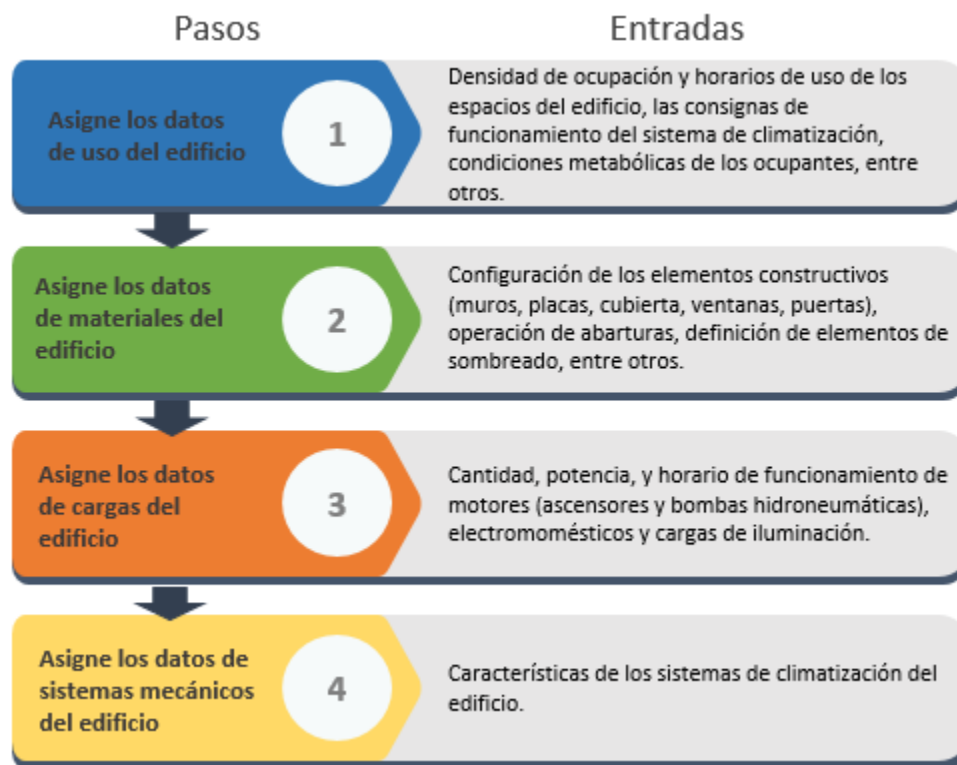
Figura 16. Procedimiento para la asignación de datos al modelo energético.
