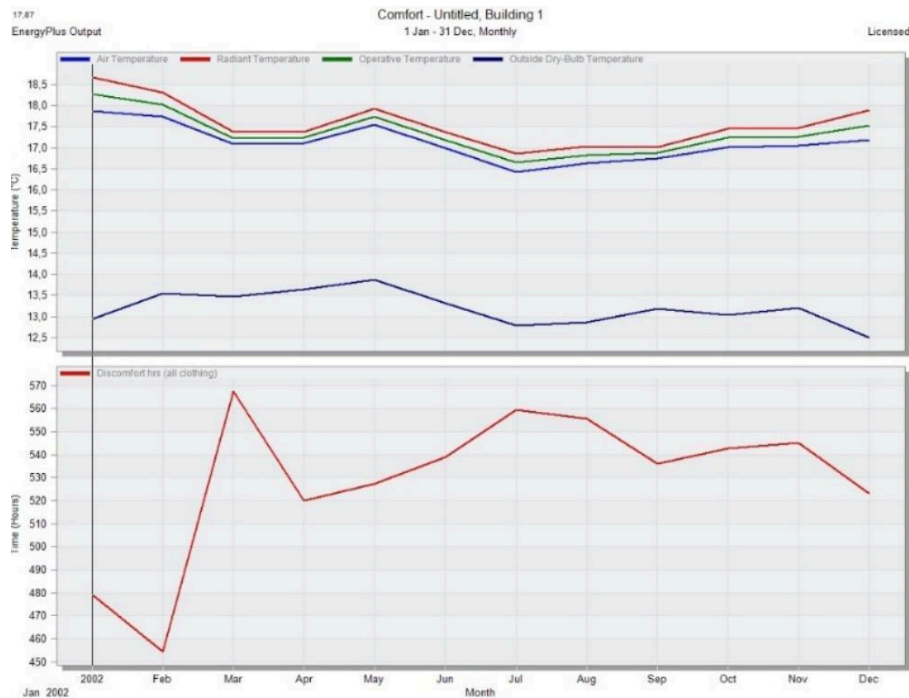
Figura 22. Temperaturas y horas de disconfort unifamiliar NO VIS – Bogotá
