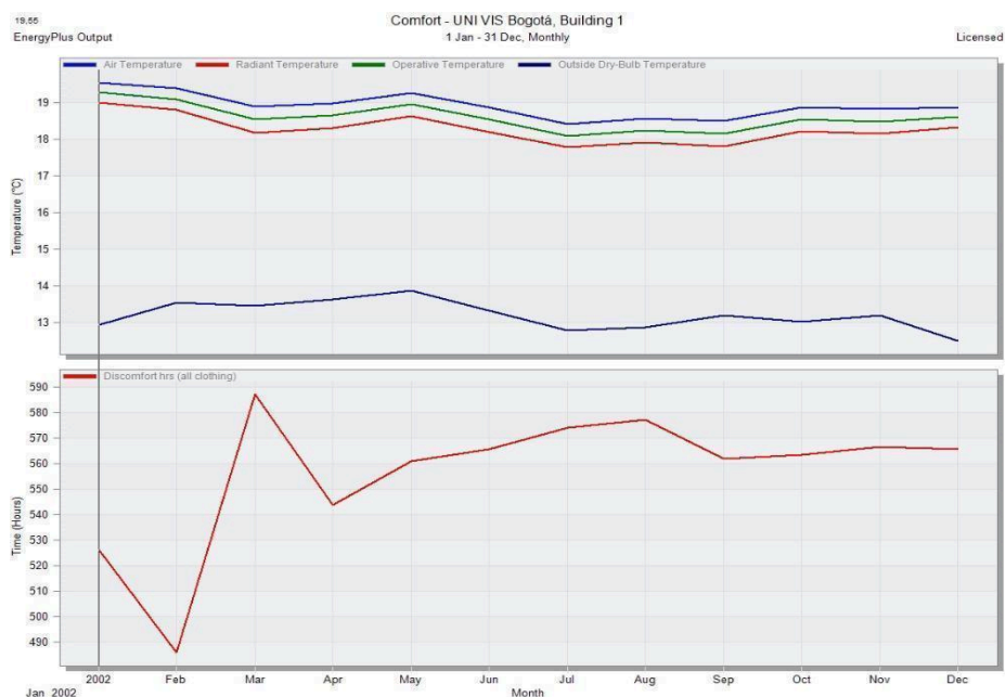
Figura 19. Temperaturas y horas de discomfort unifamiliar VIS – Bogotá
