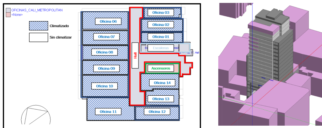
Figura 3. Planta típica y modelo energético de la tipología de oficinas para clima cálido seco.
