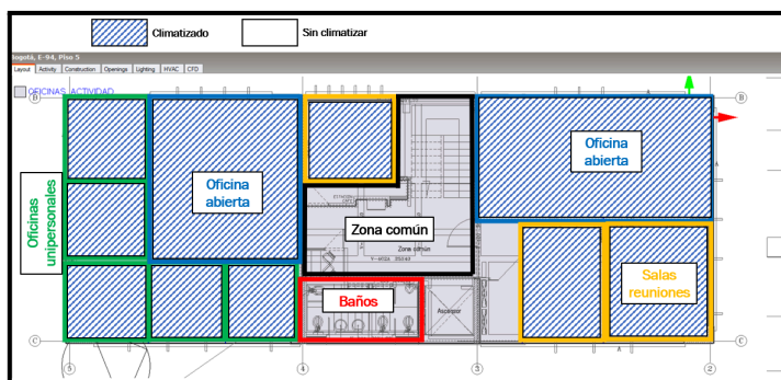
Figura 1. Planta típica y modelo energético de la tipología de oficinas para clima frío.
