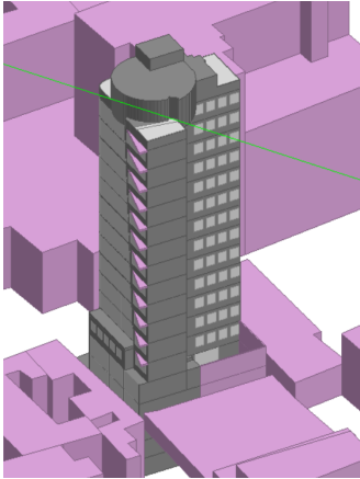
Figura 4. Planta típica y modelo energético de la tipología de oficinas para clima templado,
