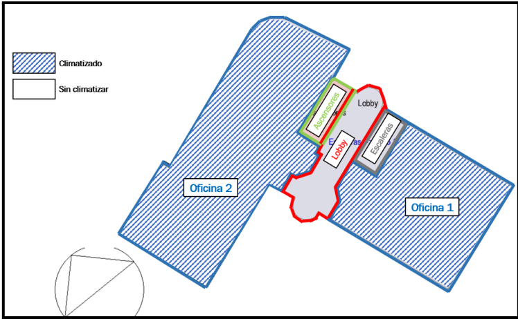
Figura 4. Planta típica y modelo energético de la tipología de oficinas para clima templado,
