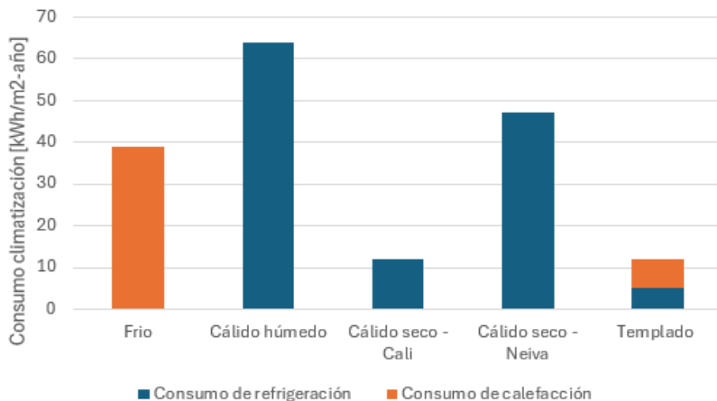
Figura 8. Consumos de climatización para la tipología de Vivienda Multifamiliar NO VIS,
