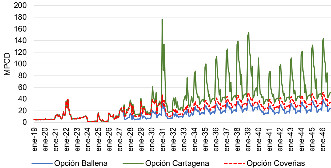
Gráfica 9-4 Comparación del valor esperado de demanda no abastecida de gas natural para las potenciales alternativas de importación
