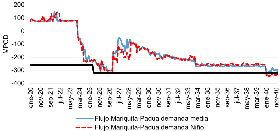
Gráfica 5-9. Proyección de flujo de gas natural entre Padua y Mariquita
