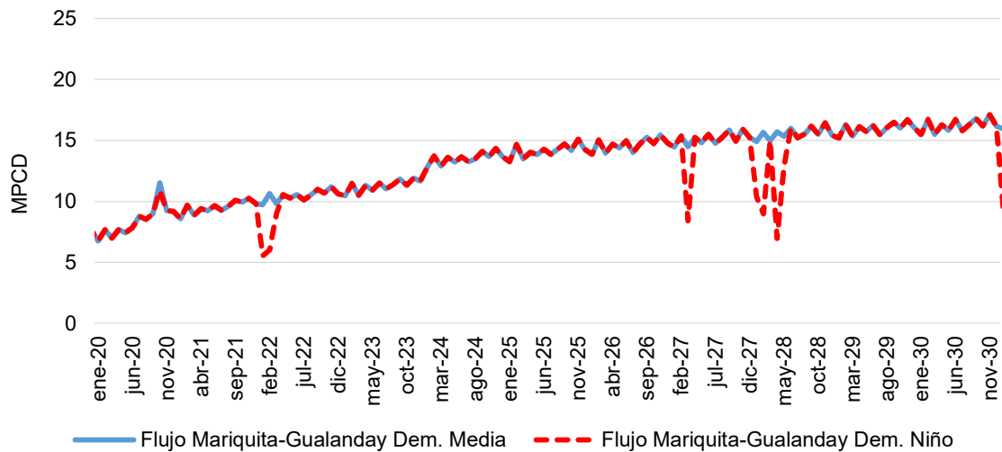
Gráfica 8-6 Proyección de flujo en el Gasoducto Mariquita- Gualanday (a) Flujo (b) Utilización (a)
