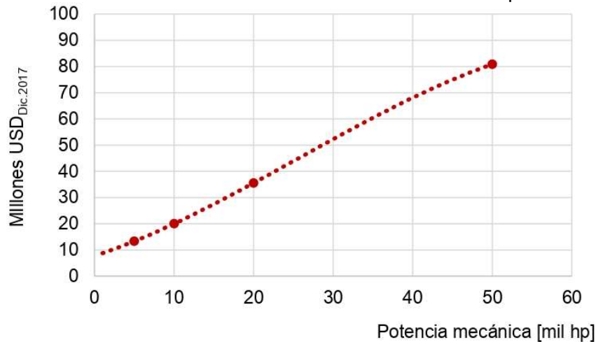
Gráfica 9-2 Estimación de costos de sistemas de compresión
