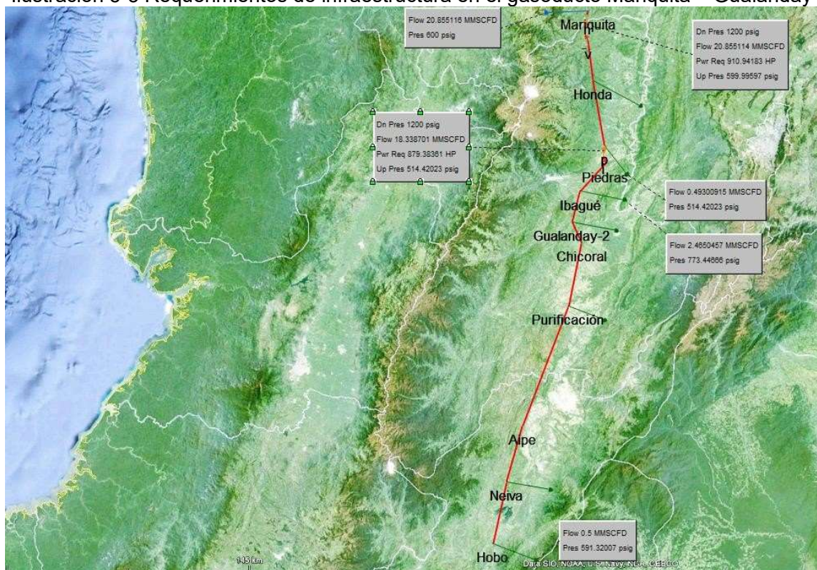
Ilustración 5-3 Requerimientos de infraestructura en el gasoducto Mariquita – Gualanday
