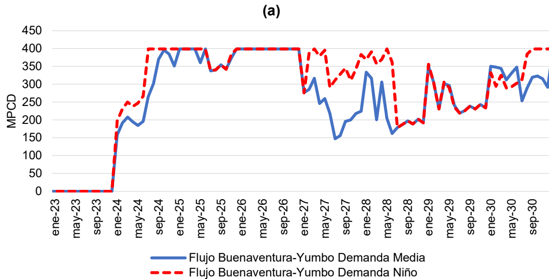
Gráfica 8-4 Proyección de flujo en el Gasoducto Buenaventura – Yumbo (a) Flujo (b) Utilización
