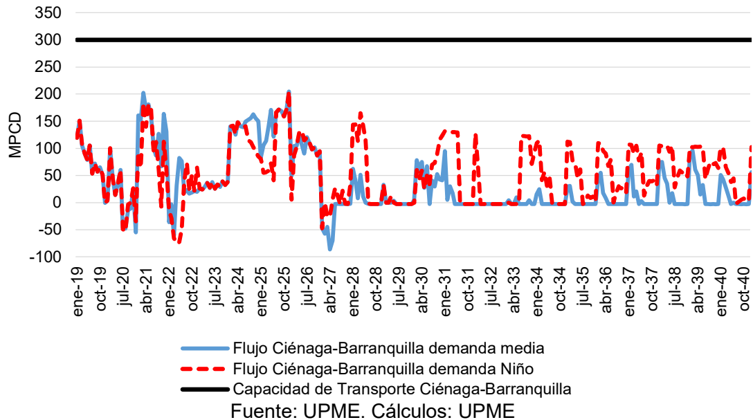
Gráfica 5-4 Proyección de flujo en el tramo Ballena -> Barranquilla
