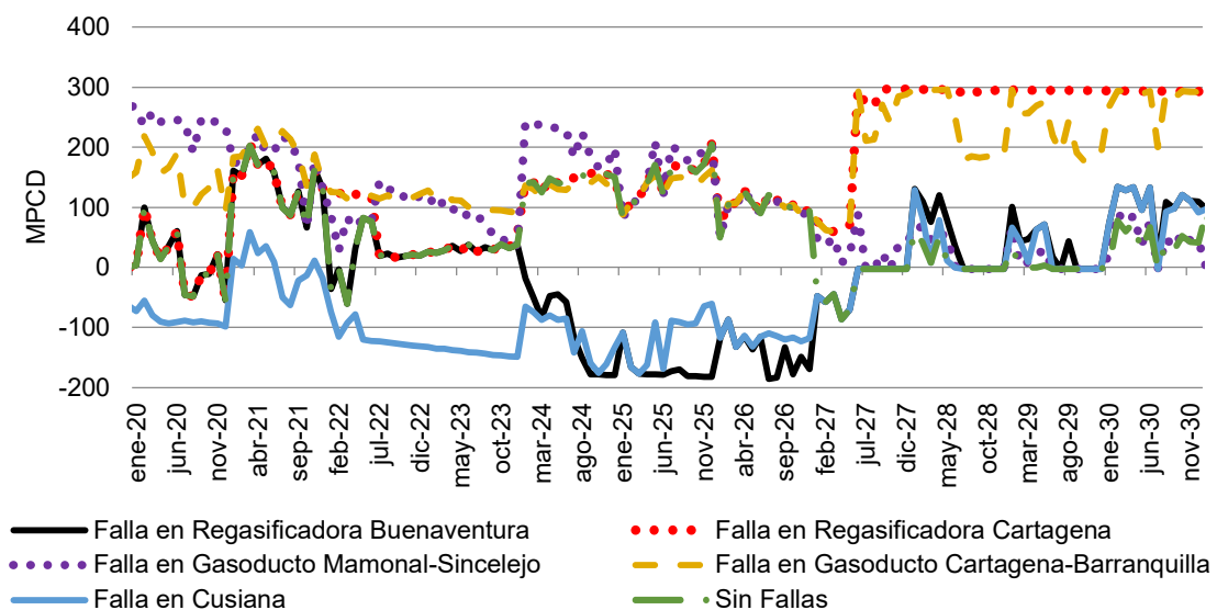
Gráfica 5-5 Proyección de flujo en el tramo Ballena > Barranquilla bajo falla de algunos elementos del sistema
