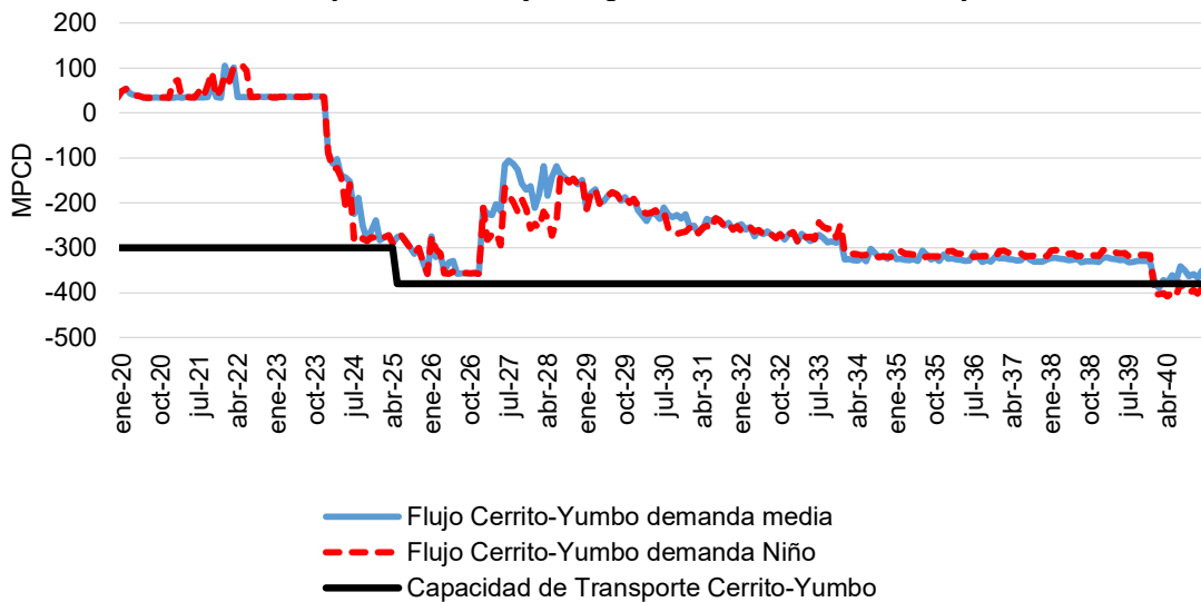
Gráfica 5-8 Proyección de flujo de gas natural entre Yumbo y Cerrito
