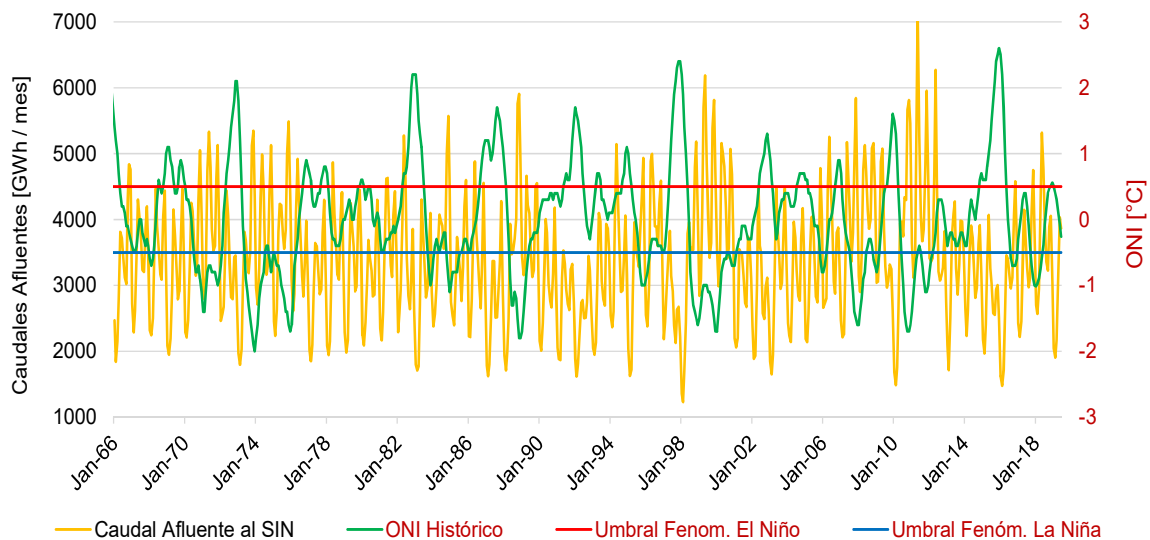
Gráfica 2-5. Caudales Afluentes
