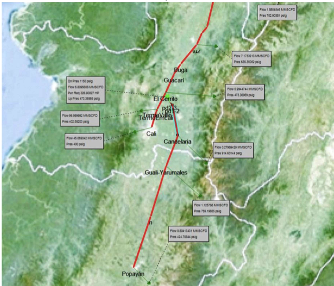
Ilustración 5-5. Requerimiento de Infraestructura ampliación capacidad de transporte ramal Jamundí
