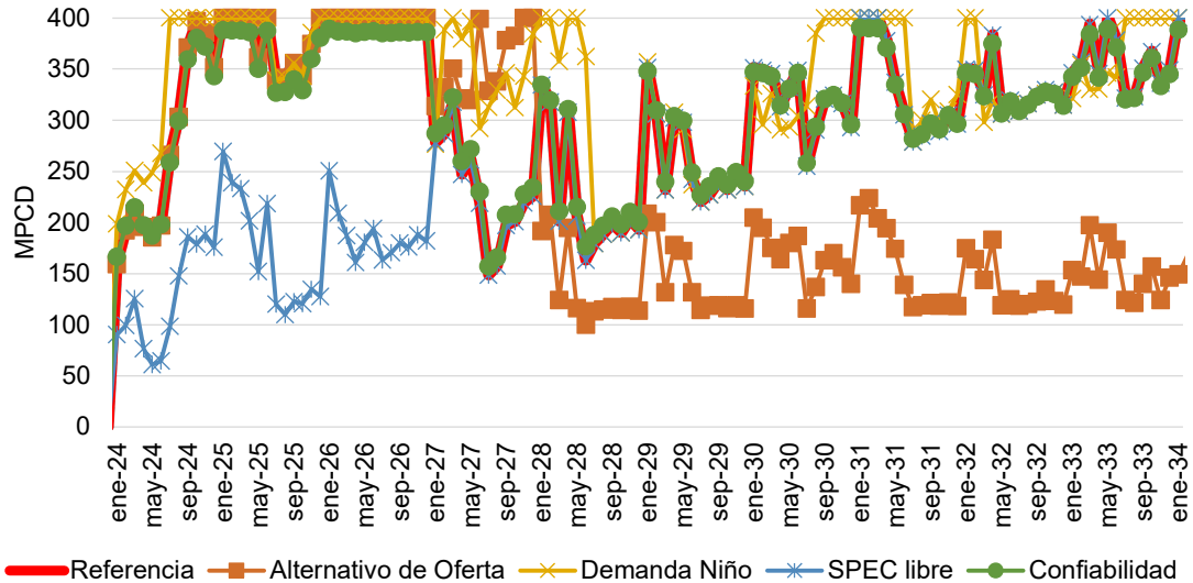
Gráfica 9-8 Perfiles de producción (uso) de la Planta de Buenaventura ante los diferentes escenarios
