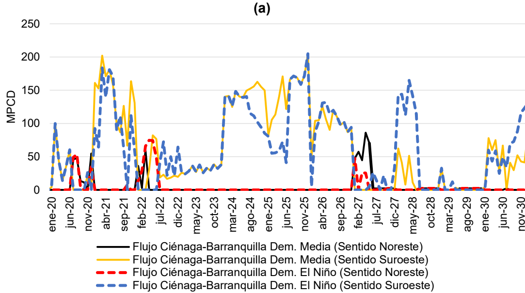
Gráfica 8-2 Proyección de flujo en el Gasoducto Ballena – Barranquilla (a) Flujo (b) Utilización
