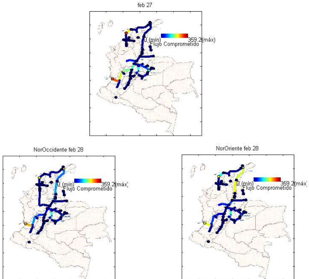
Gráfica 9-7 Comparación de flujos comprometidos por falla de los elementos del sistema de gas natural para las alternativas de interconexión Costa Atlántica – Interior
