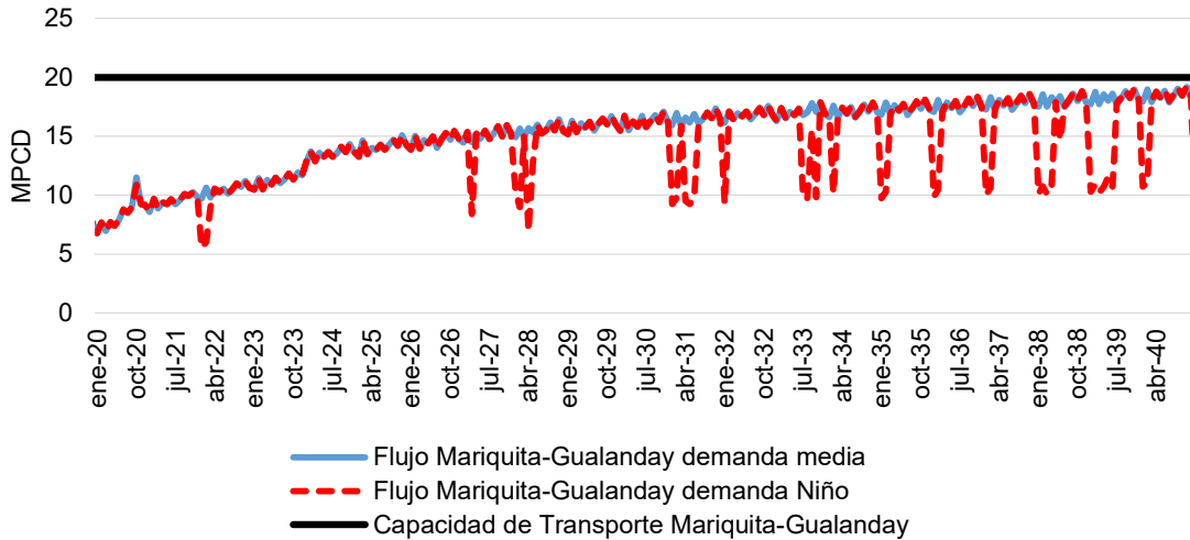
Gráfica 5-6 Proyección de flujo y capacidad de transporte tramo Mariquita - Ibagué
