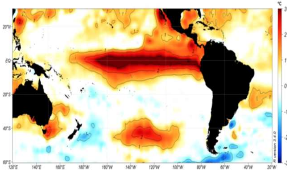
Ilustración 2-1 Calentamiento del Mar área centro-este del Océano Pacífico
