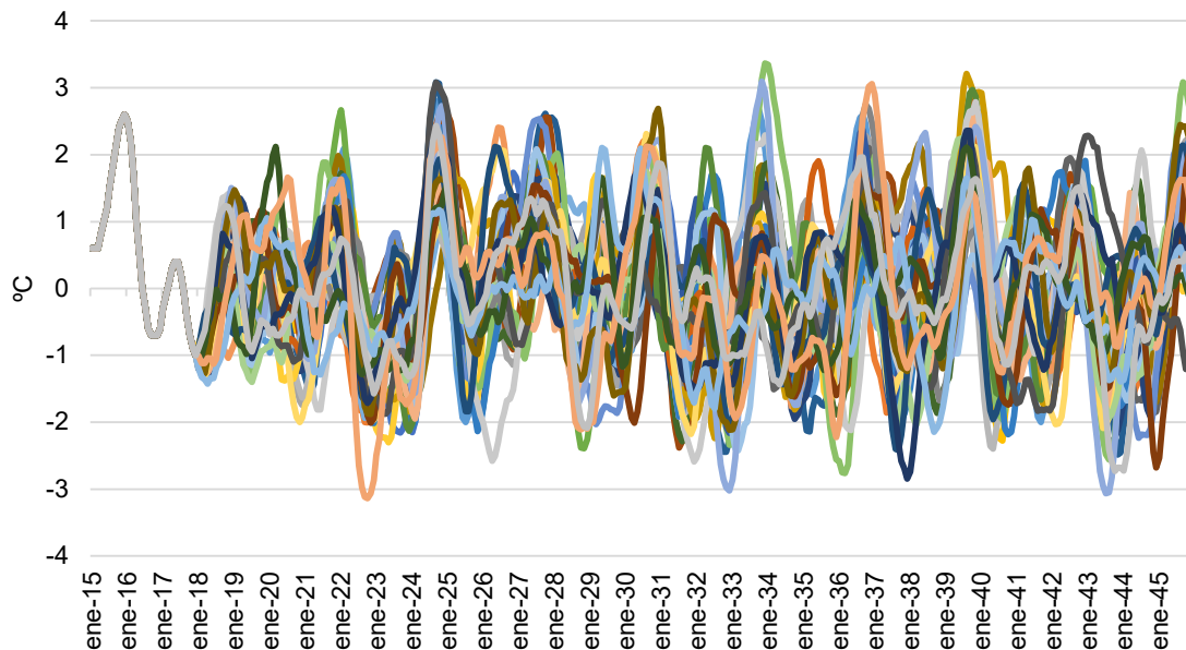
Gráfica 2-8. Series ONI generadas por el modelo de predicción.
