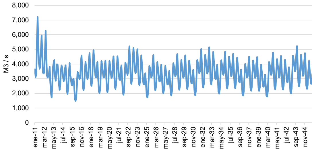
Gráfica 2-9. Hidrología correspondiente al ONI promedio
