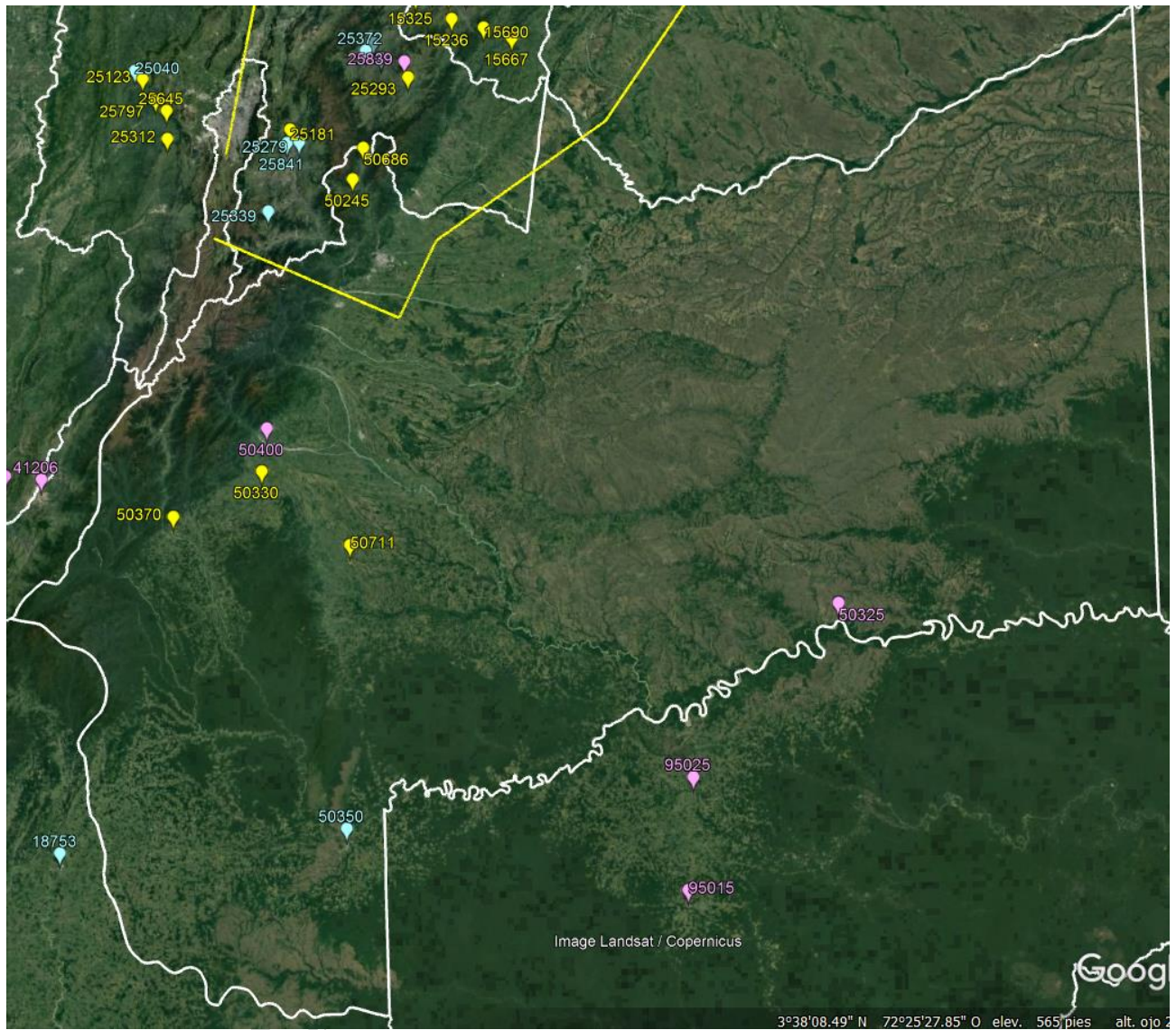
Grafica A5-21. Distribución de gas combustible proyectada -Departamento de Meta
