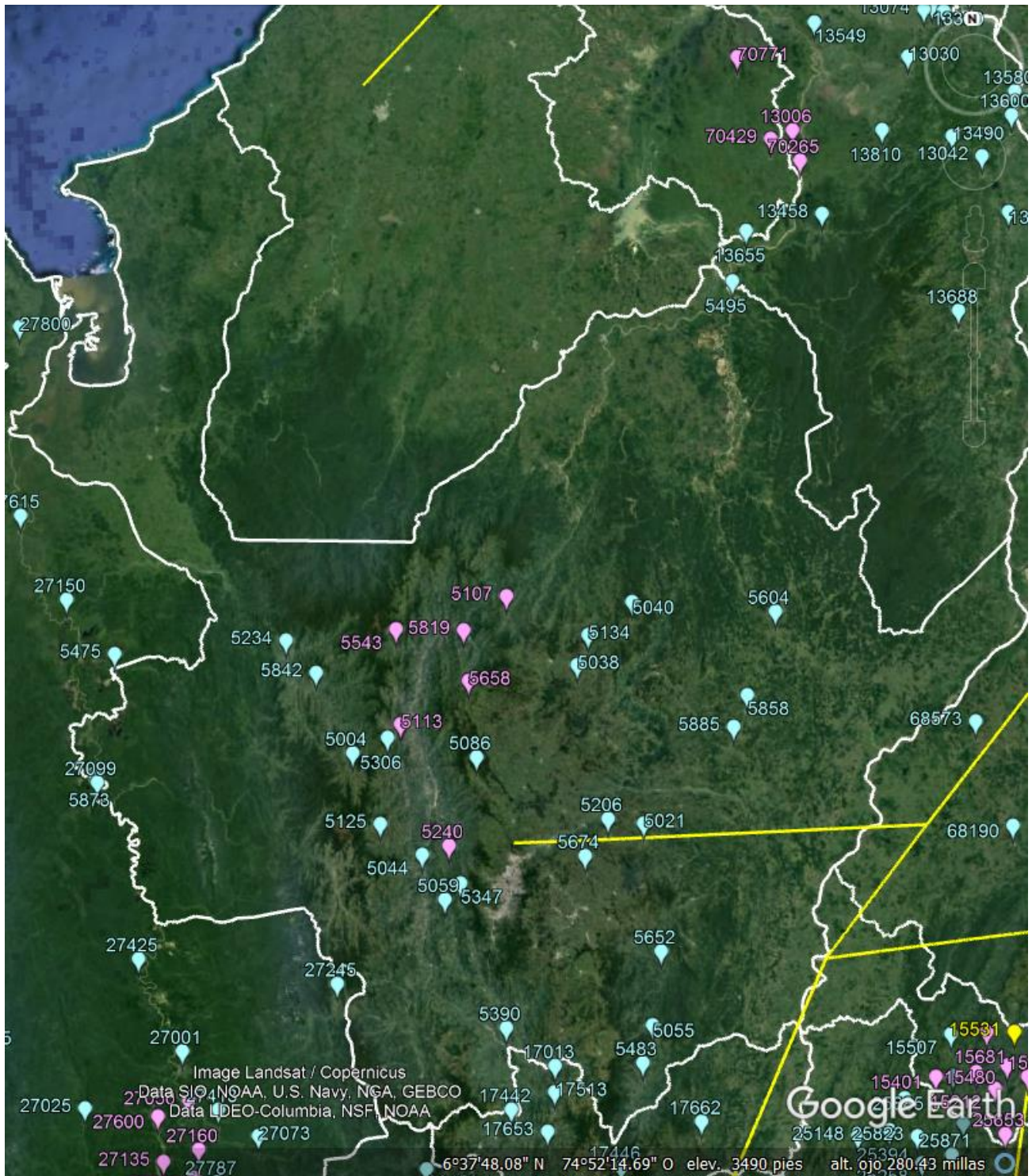
Grafica A5-5. Distribución de gas combustible proyectada -Departamento de Antioquia.
