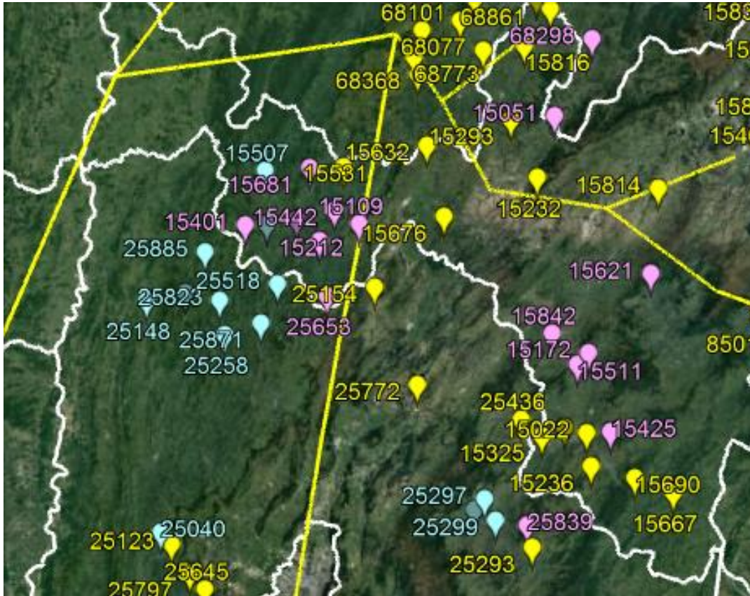
Grafica A5-19. Distribución de gas combustible proyectada - Departamentos de Cundinamarca y Boyacá A
