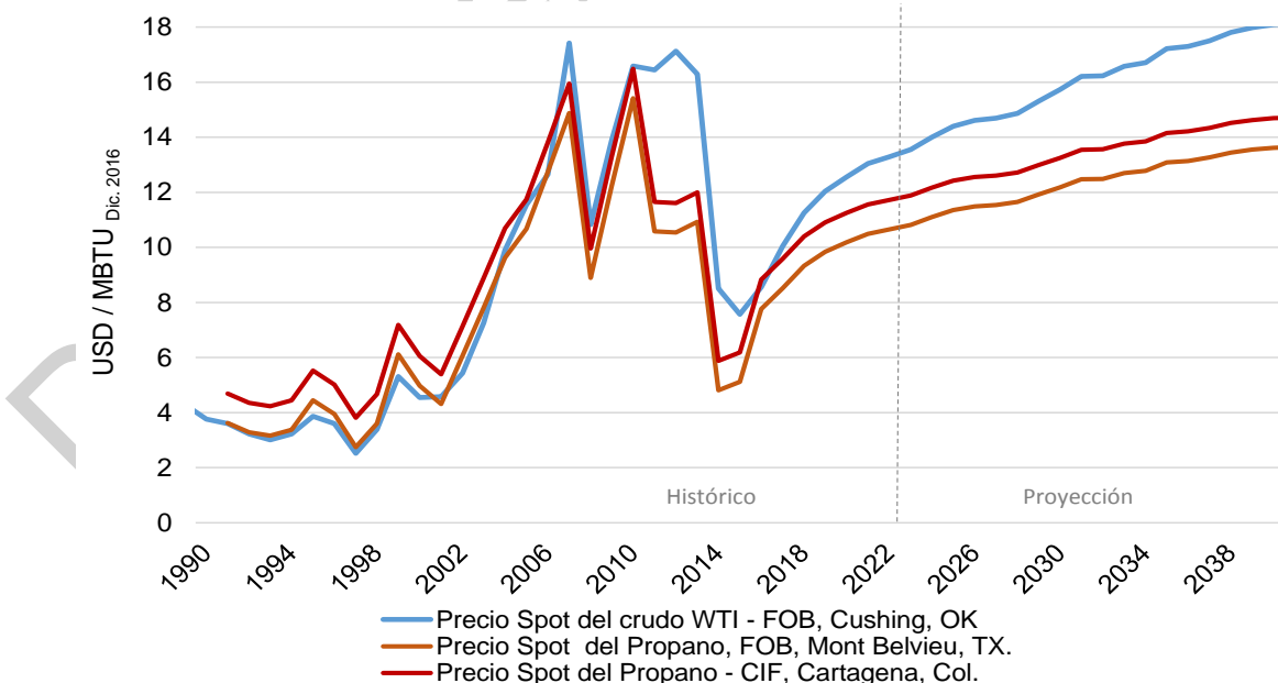
Gráfica 4-18. Proyección de precios del petróleo WTI y del propano Mont Belvieu
