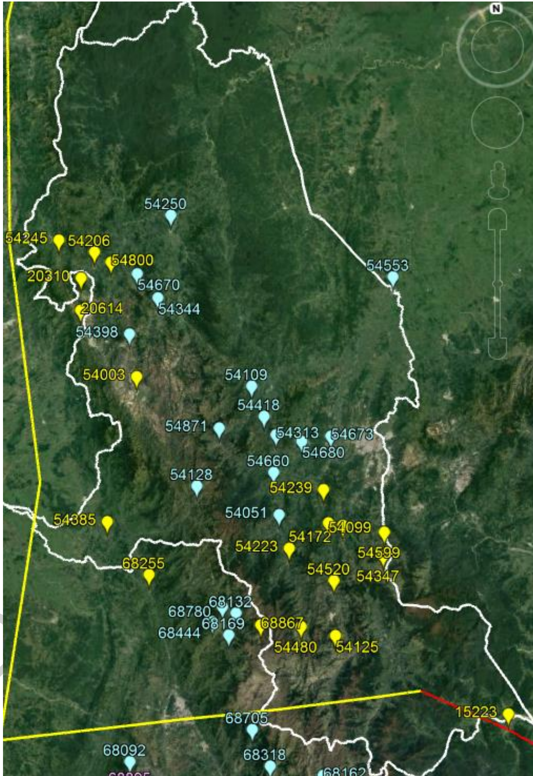
Grafica A5-8. Distribución de gas combustible proyectada -Departamento de Norte de Santander
