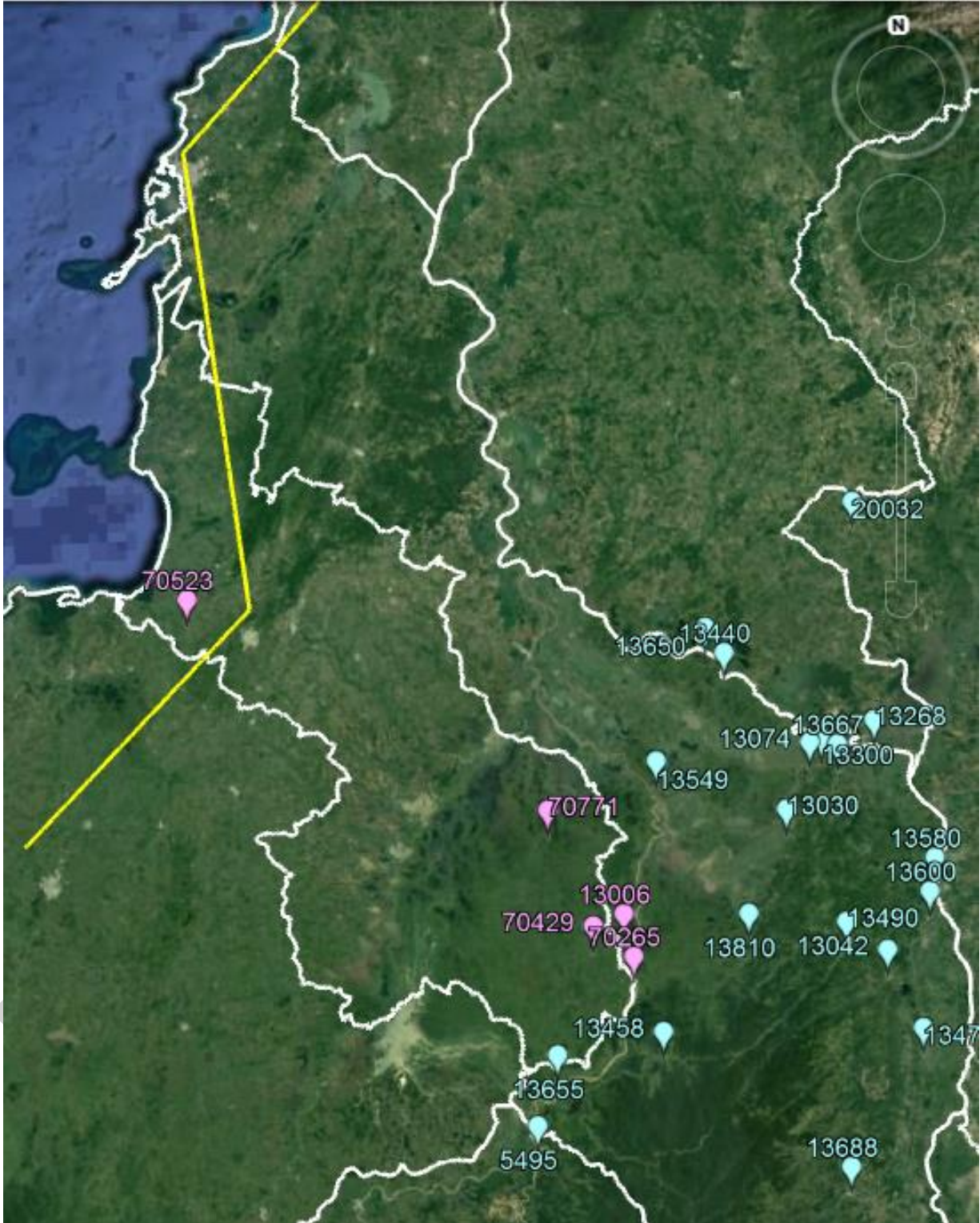
Grafica A5-6. Distribución de gas combustible proyectada -Departamentos de Sucre y Bolívar.
