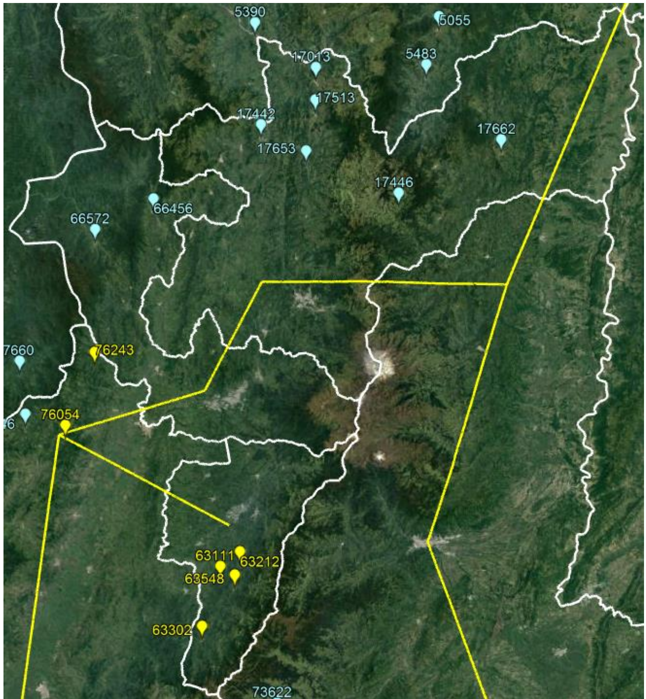
Grafica A5-11. Distribución de gas combustible proyectada –Eje Cafetero
