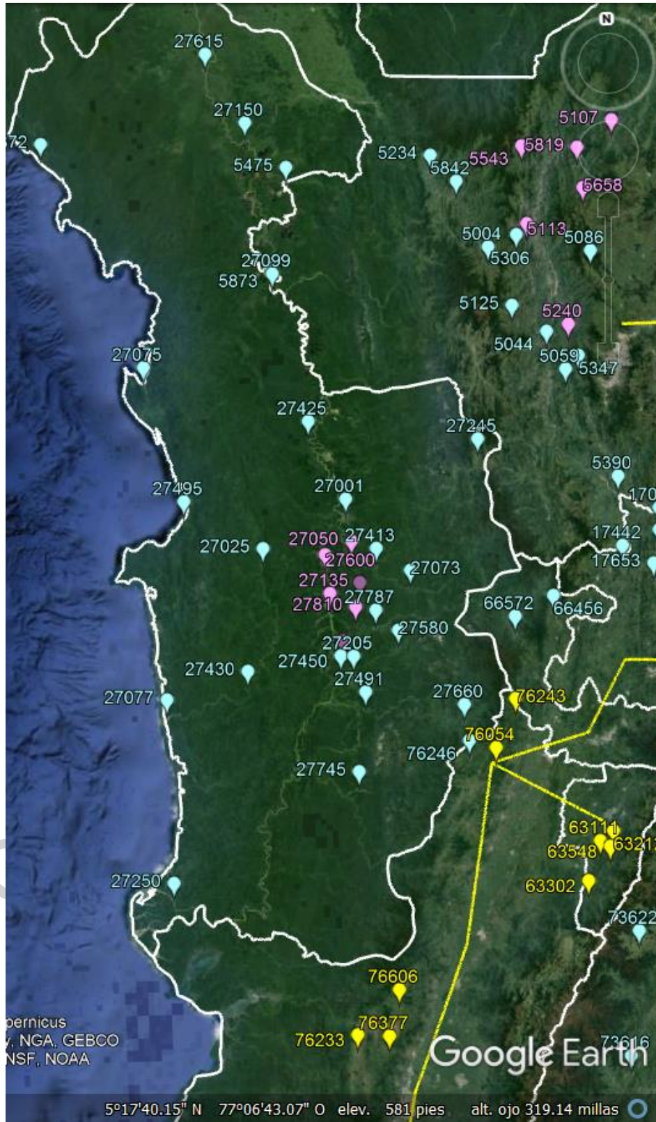
Grafica A5-4. Distribución de gas combustible proyectada -Departamento de Chocó.
