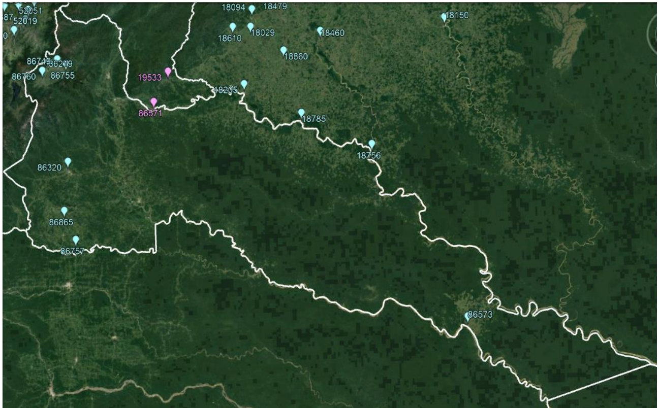
Grafica A5-15. Distribución de gas combustible proyectada -Departamento de Putumayo
