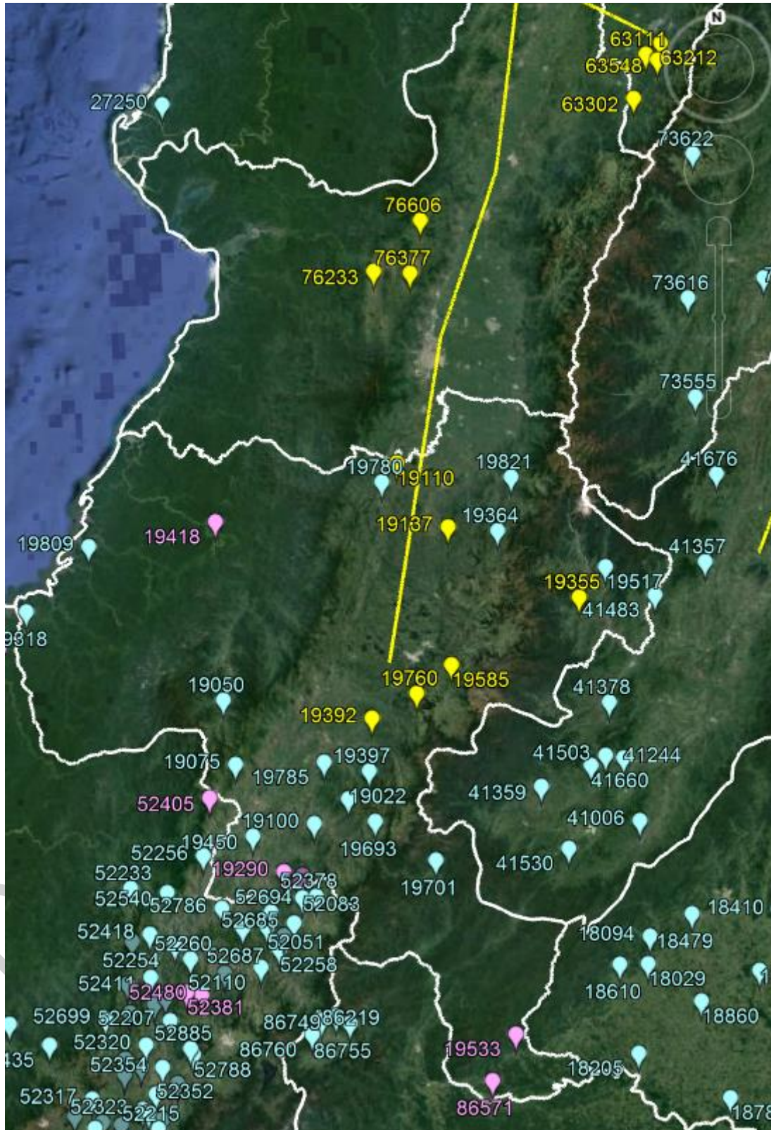
Grafica A5-3. Distribución de gas combustible proyectada -Departamentos de Cauca y Valle.
