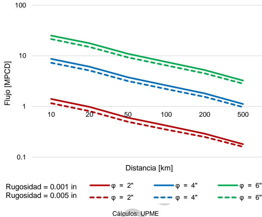
Gráfica 4-4. Relación entre la capacidad de transporte y la distancia, según el diámetro del gasoducto.
