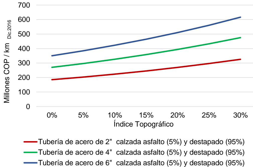
Gráfica 4-5. Relación entre la capacidad de transporte y la distancia, según el diámetro del gasoducto.
