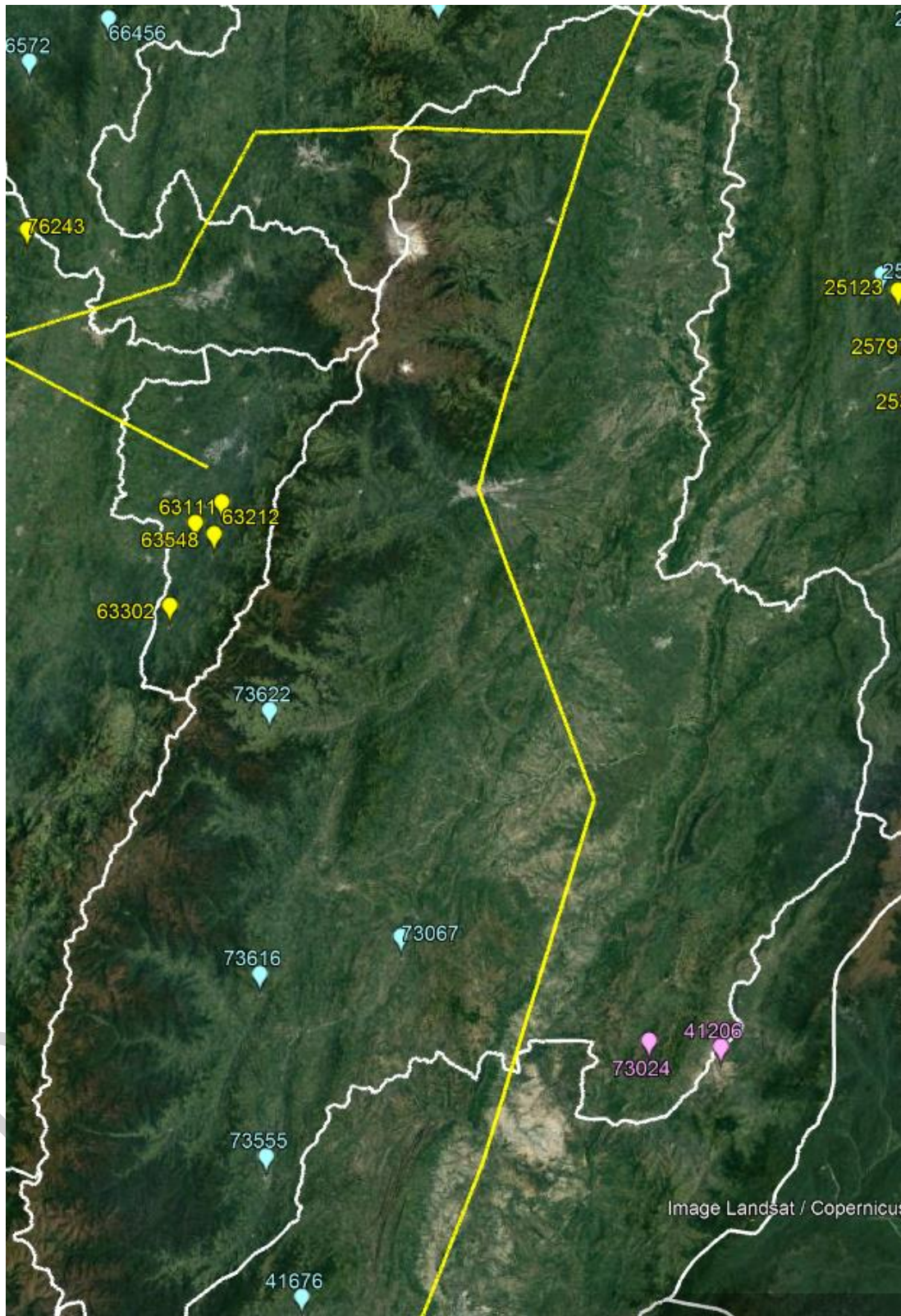
Grafica A5-12. Distribución de gas combustible proyectada -Departamento del Tolima
