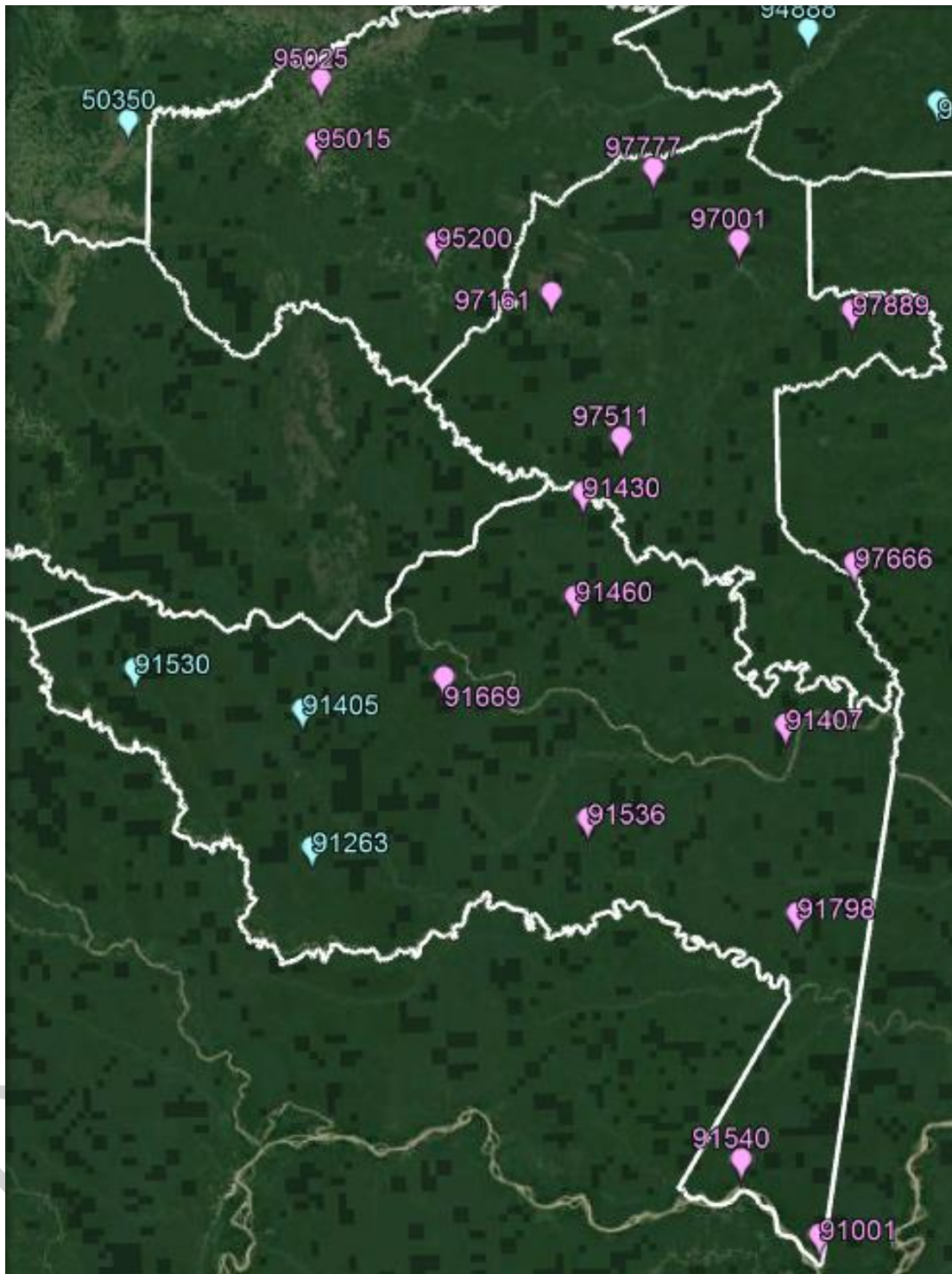
Grafica A5-16. Distribución de gas combustible proyectada – Región Amazónica
