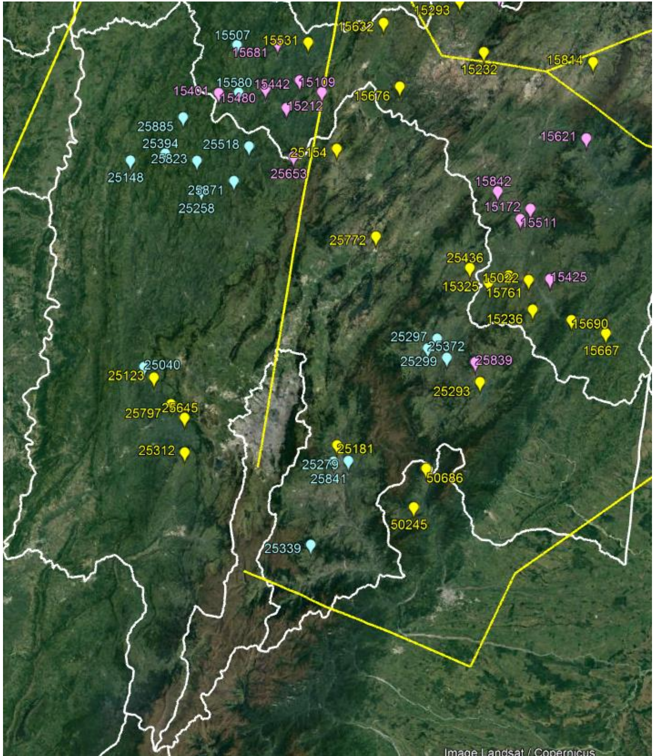
Grafica A5-18. Distribución de gas combustible proyectada – Departamentos de Cundinamarca
