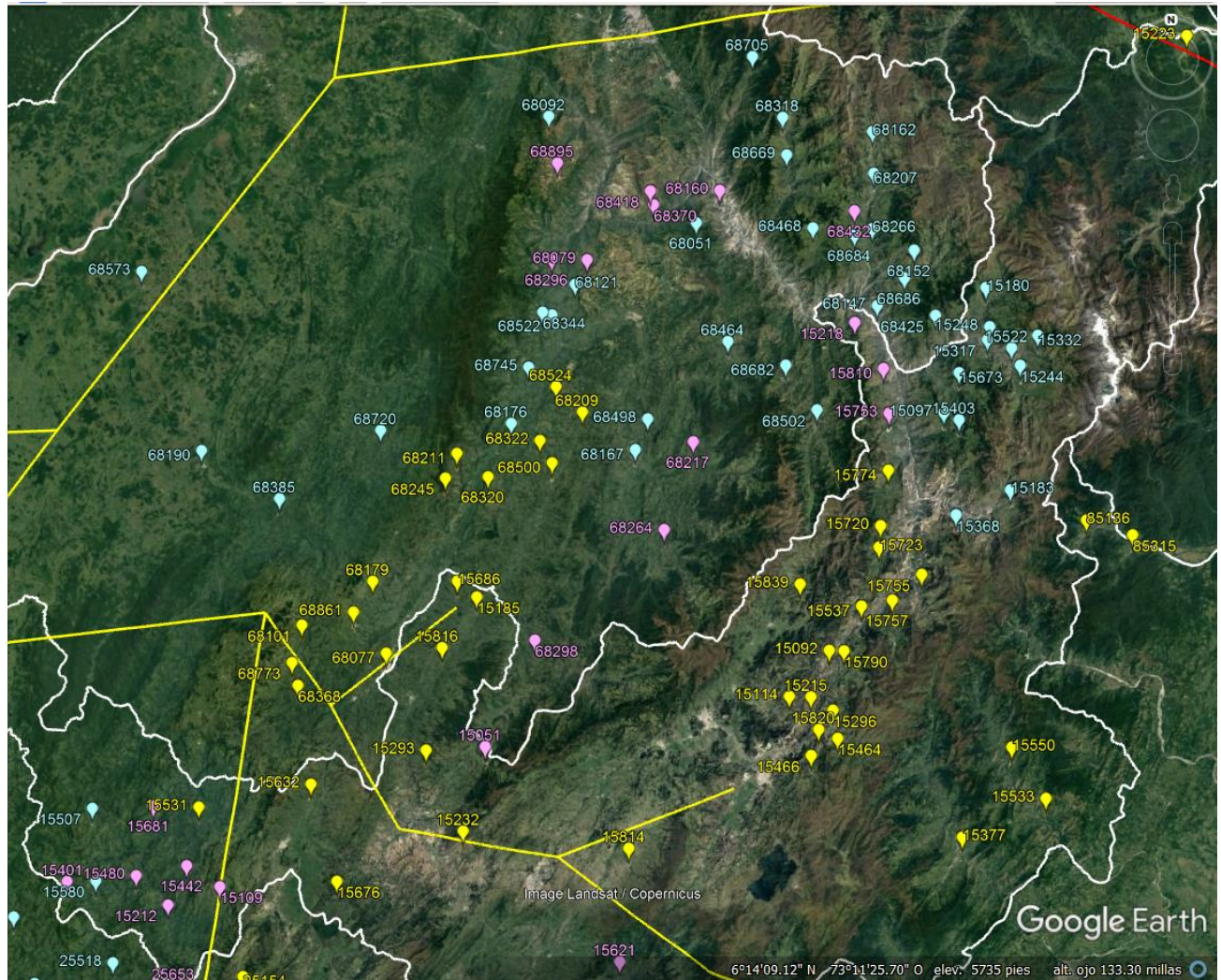
Grafica A5-9. Distribución de gas combustible proyectada -Departamento de Boyacá
