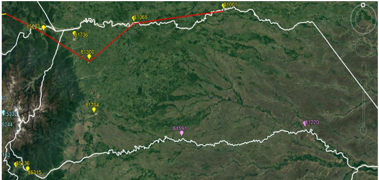
Grafica A5-10. Distribución de gas combustible proyectada -Departamento de Arauca
