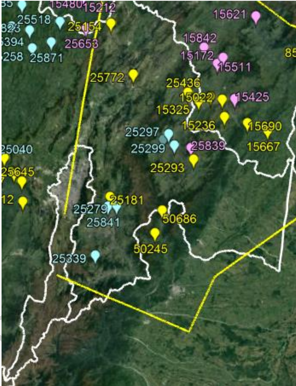
Grafica A5-20. Distribución de gas combustible proyectada - Departamentos de Cundinamarca y Boyacá B
