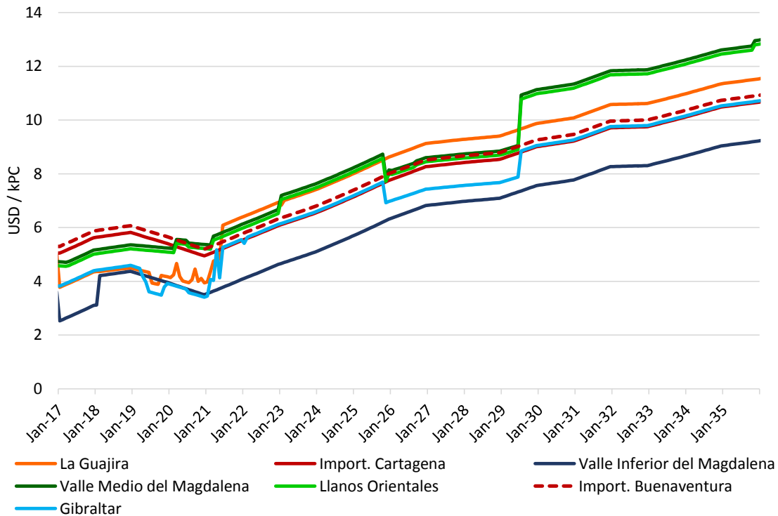
Gráfica 4-3. Proyección de los precios de importación y boca de pozo de gas natural
