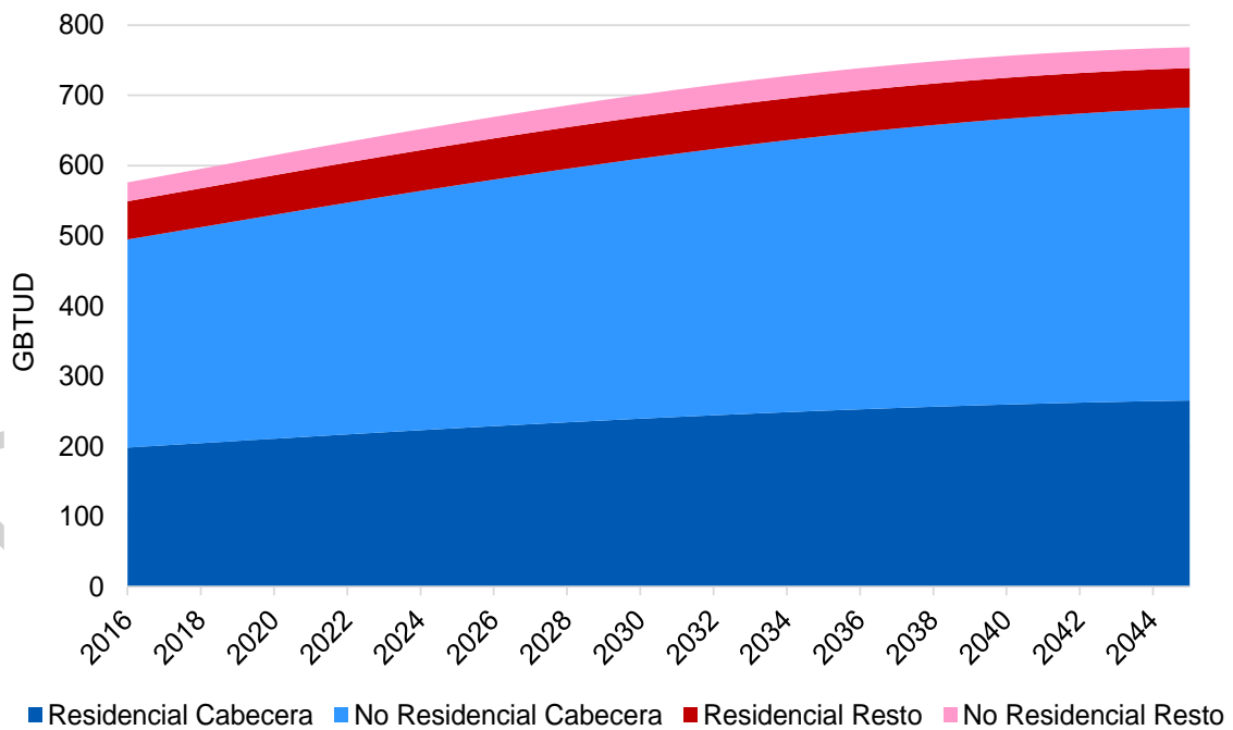
Gráfica 4-13. Proyección de demanda nacional residencial y no residencial de gas combustible
