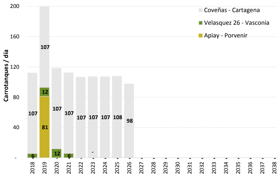
Gráfica 7-2 Demanda de Vehículos para Transporte de Crudo – Escenario Bajo Oferta Crudo 12
