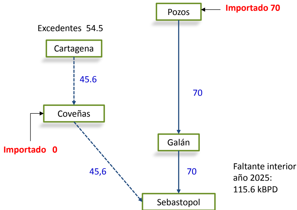
Gráfica 7-20 Opción de Abastecimiento Cartagena-Coveñas-Sebastopol (kBPD)
