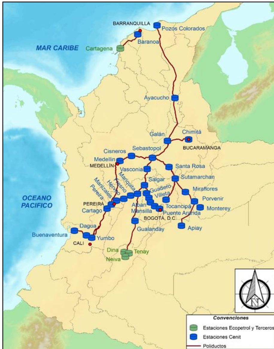
Gráfica 2-26 Mapa de transporte de refinados
