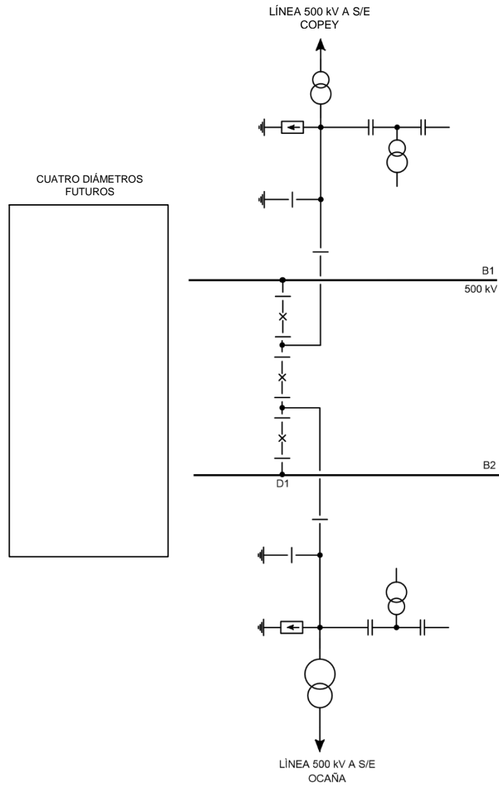
FIGURA 3 ESQUEMA UNIFILAR SUBESTACIÓN LA LOMA 500 kV
