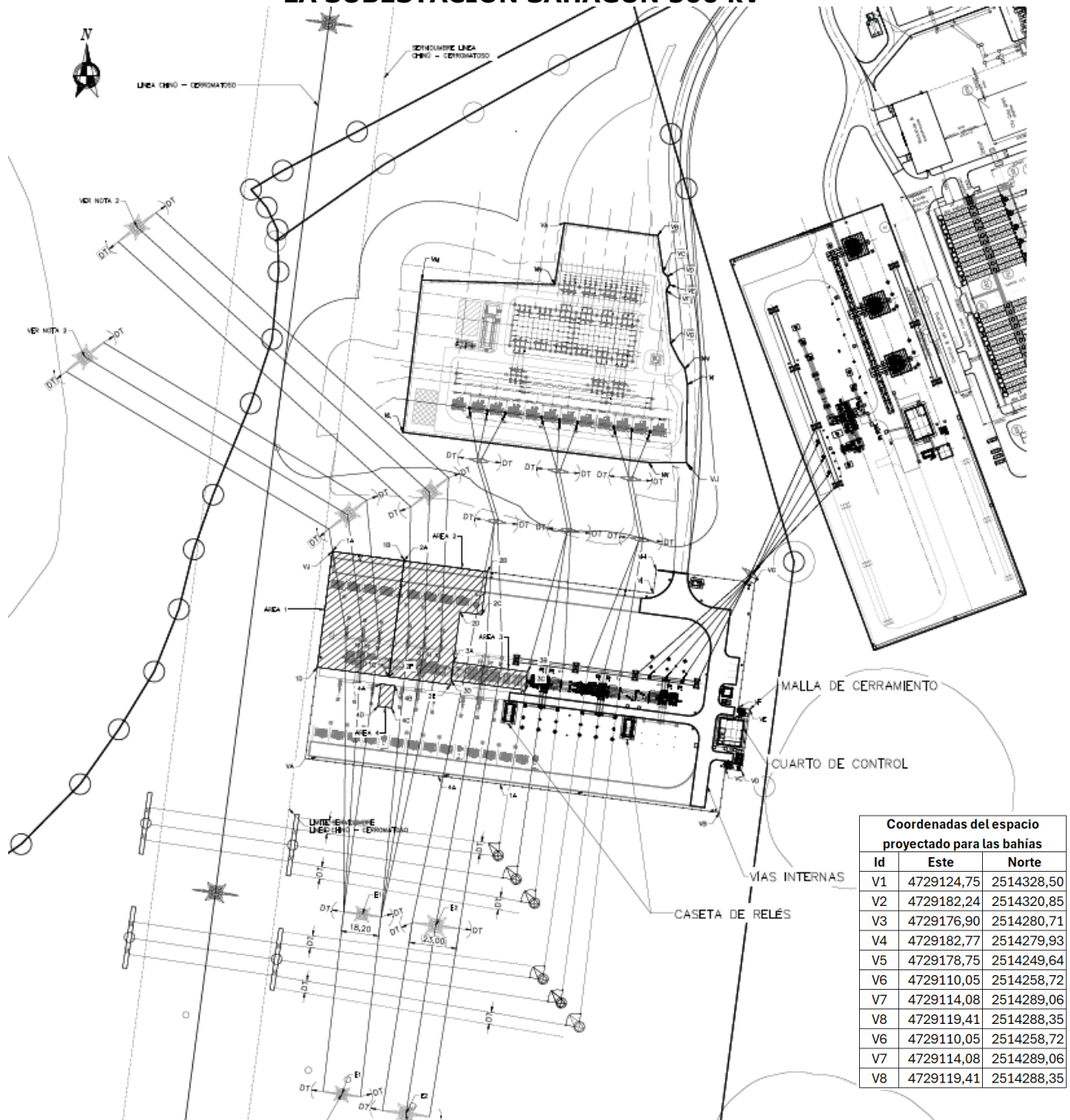
Anexo 1.2. - Figura 2 - Plano de Planta Subestación Sahagún 500 kV.
