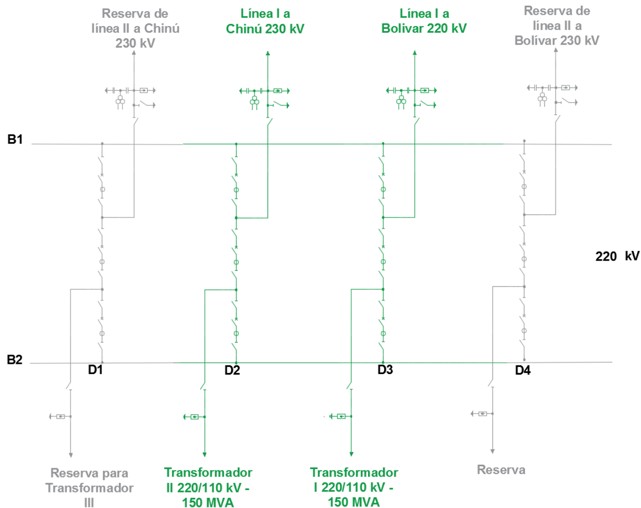
Figura 2 - Diagrama Unifilar Subestación Tolu Viejo 220 kV
