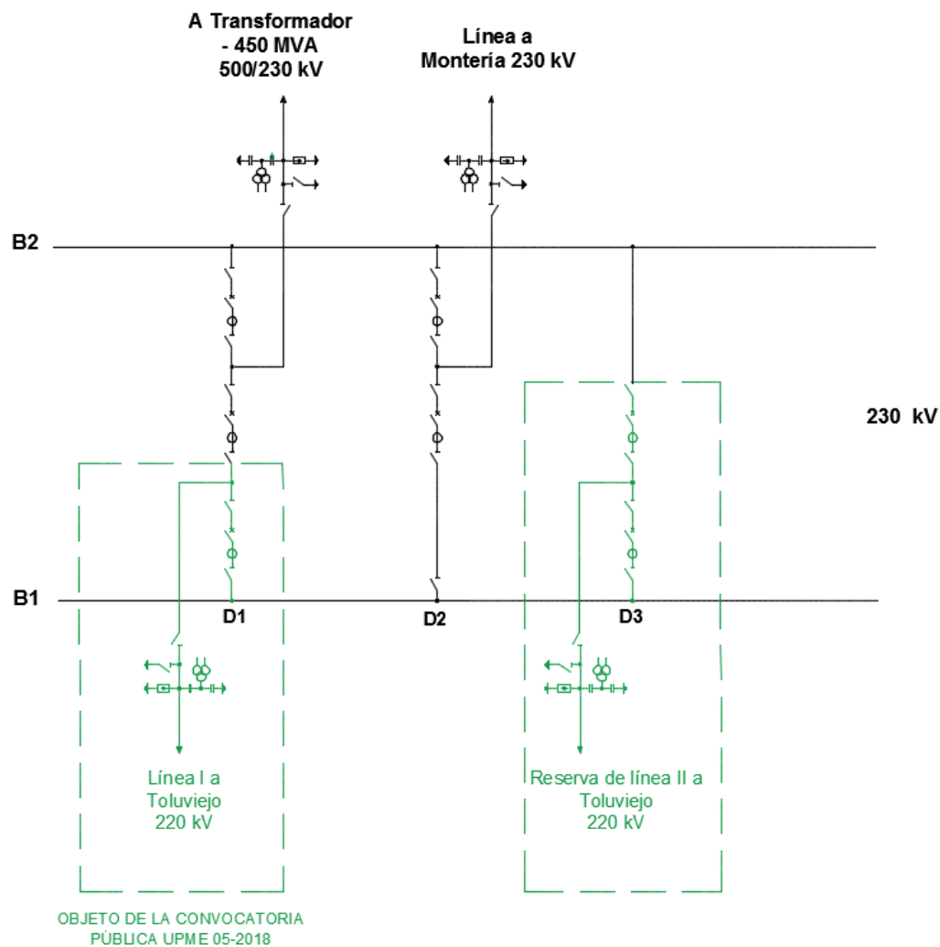
Figura 3 - Diagrama Unifilar Subestación Chinú 230 kV
