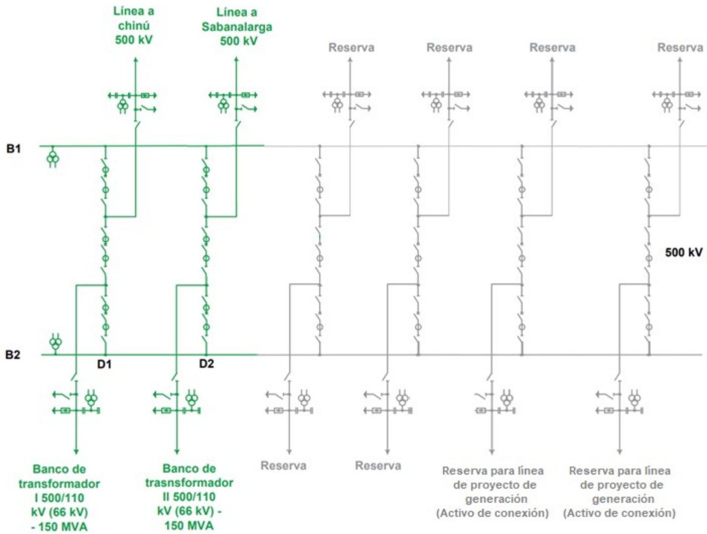
FIGURA 2 DIAGRAMA UNIFILAR SUBESTACIÓN CARRETO 500 kV
