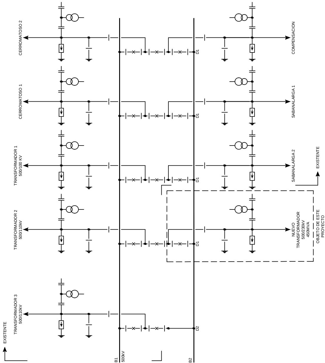
FIGURA 3 ESQUEMA UNIFILAR SUBESTACIÓN CHINU 500kV
