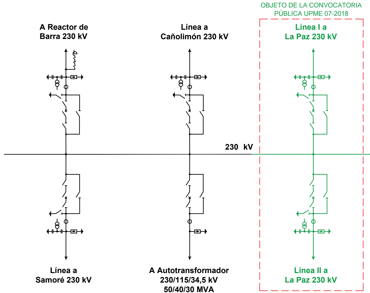
Figura 4. Diagrama Unifilar Subestación Banadía 230 kV (Prepublicación)
