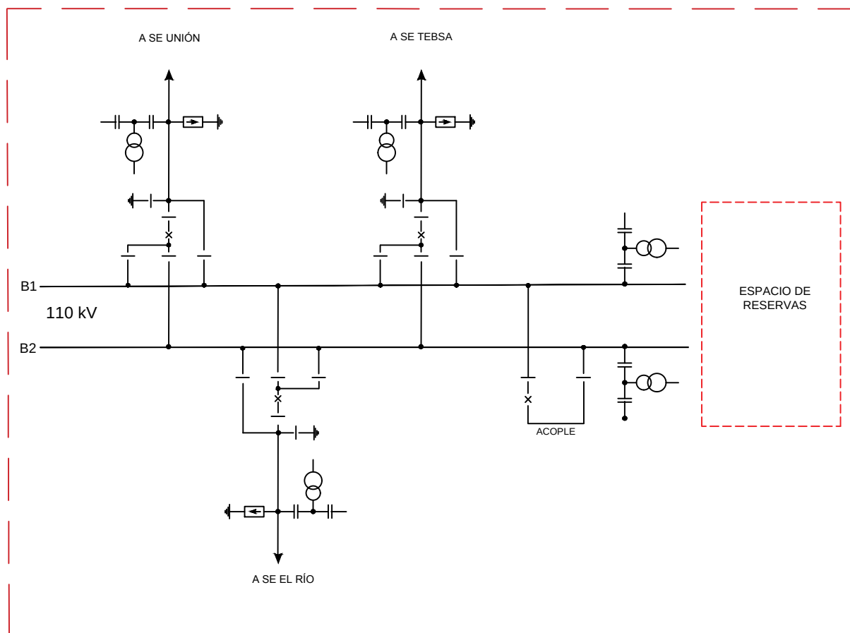
FIGURA 7 ESQUEMA UNIFILAR SUBESTACIÓN MAGDALENA 110 kV
