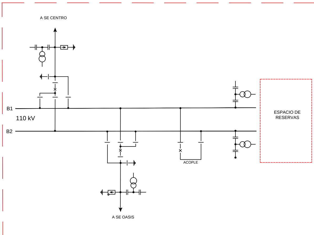
FIGURA 3 ESQUEMA UNIFILAR SUBESTACIÓN ESTADIO 110 kV
