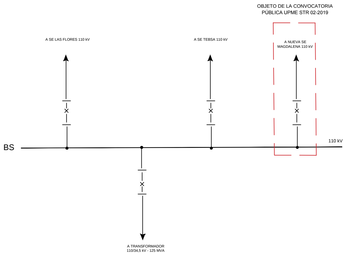
FIGURA 6 ESQUEMA UNIFILAR SUBESTACIÓN EL RIO 110 kV
