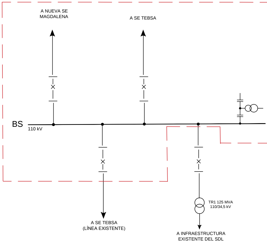
FIGURA 8B FUTURO ESQUEMA UNIFILAR SUBESTACIÓN UNIÓN 110 kV (PREPUBLICACIÓN)
