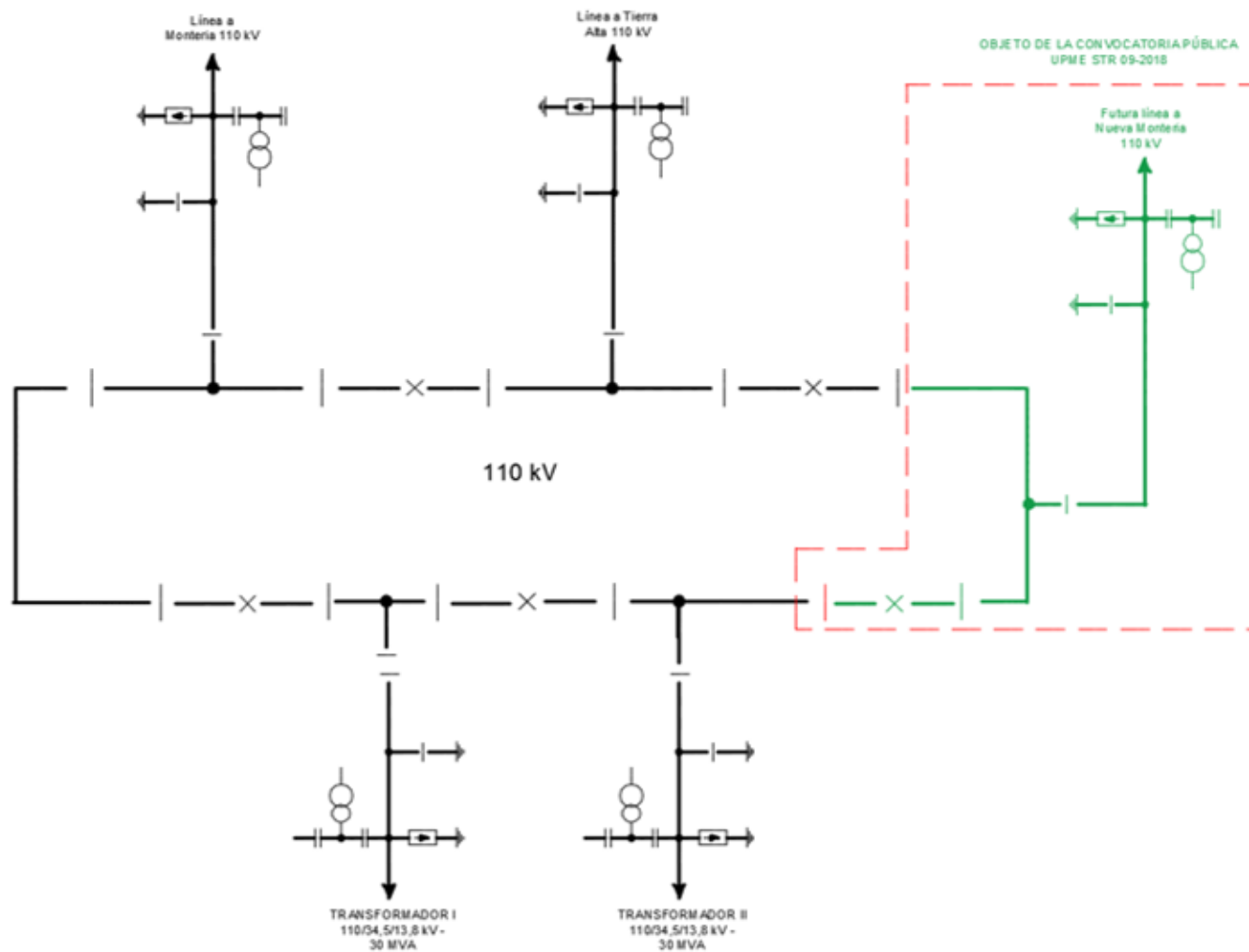
Figura 2. Diagrama Unifilar Subestación Rio Sinú 110 kV.
