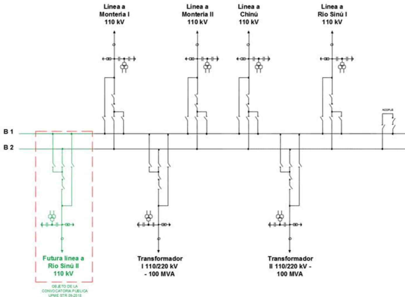
Figura 3. Diagrama Unifilar Subestación Nueva Montería 110 kV.
