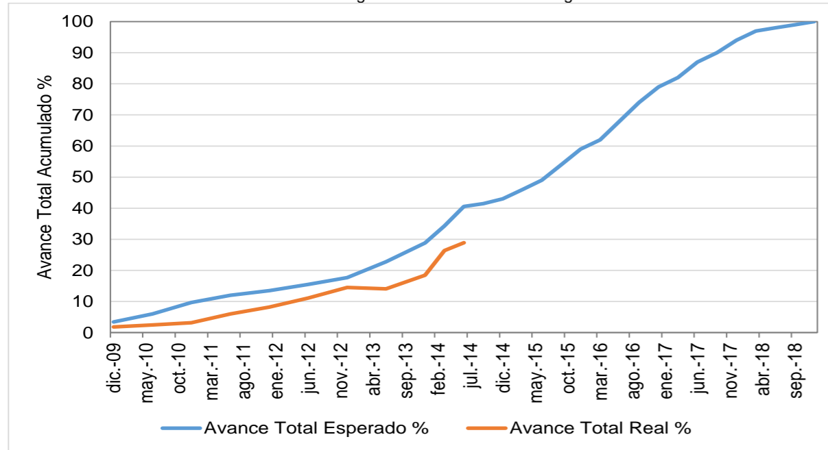
Gráfica 6 Seguimiento a la Curva S Ituango
