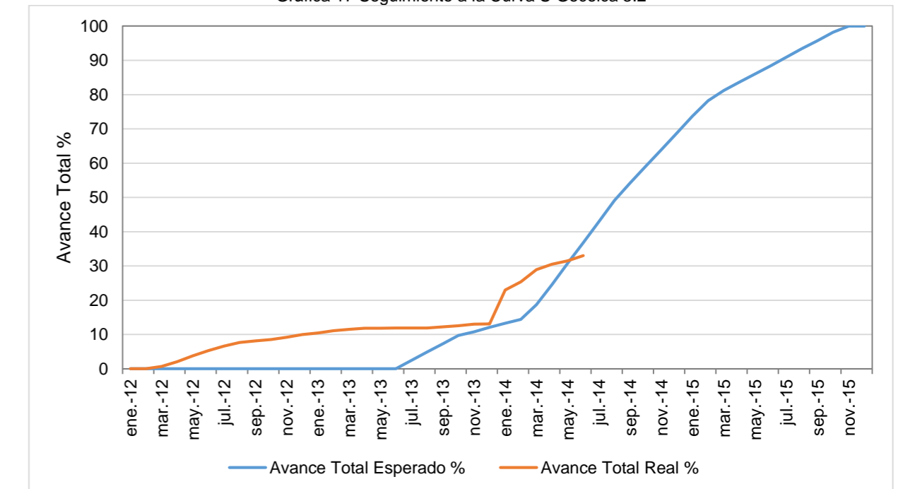
Gráfica 17 Seguimiento a la Curva S Gecelca 3.2
