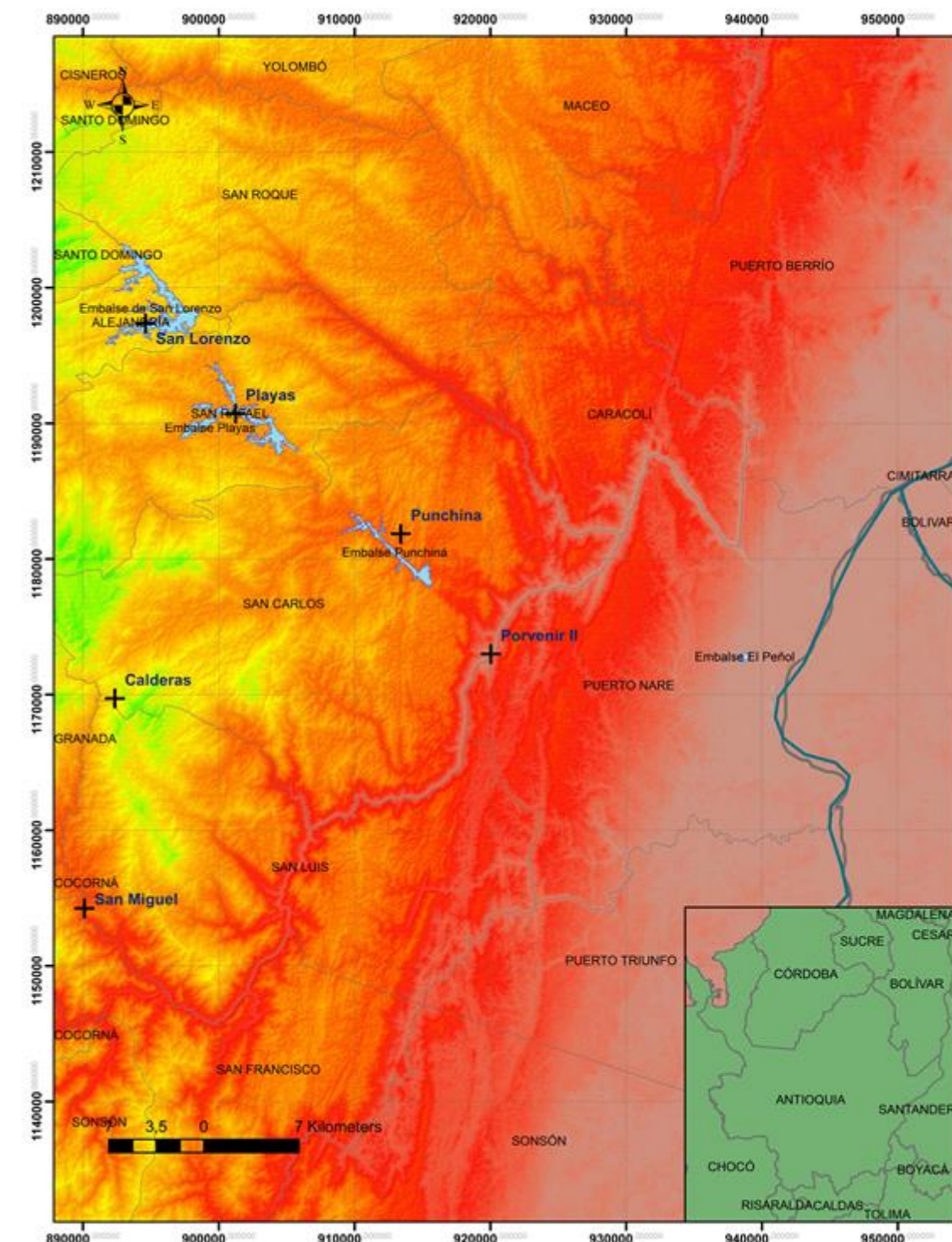
Gráfica 9 Ubicación Porvenir 2
