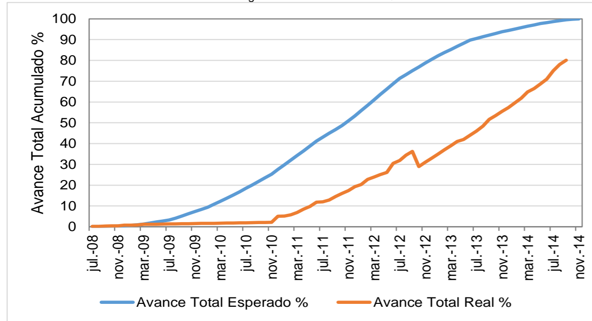
Gráfica 2 Seguimiento a la Curva S El Quimbo
