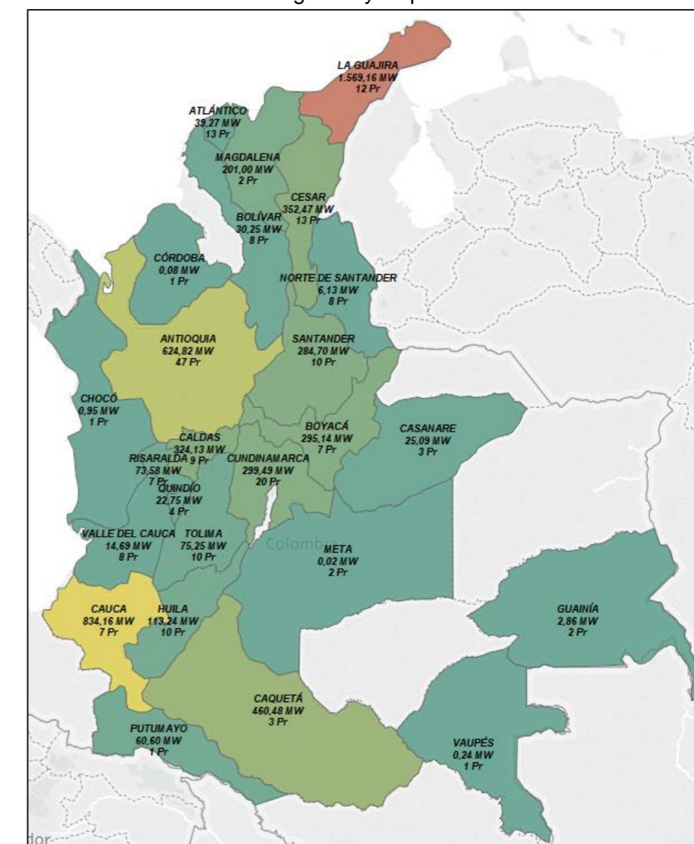
Gráfica 14: Ubicación de proyectos registrados en Fase 1 Número de registros y Capacidad Instalada
