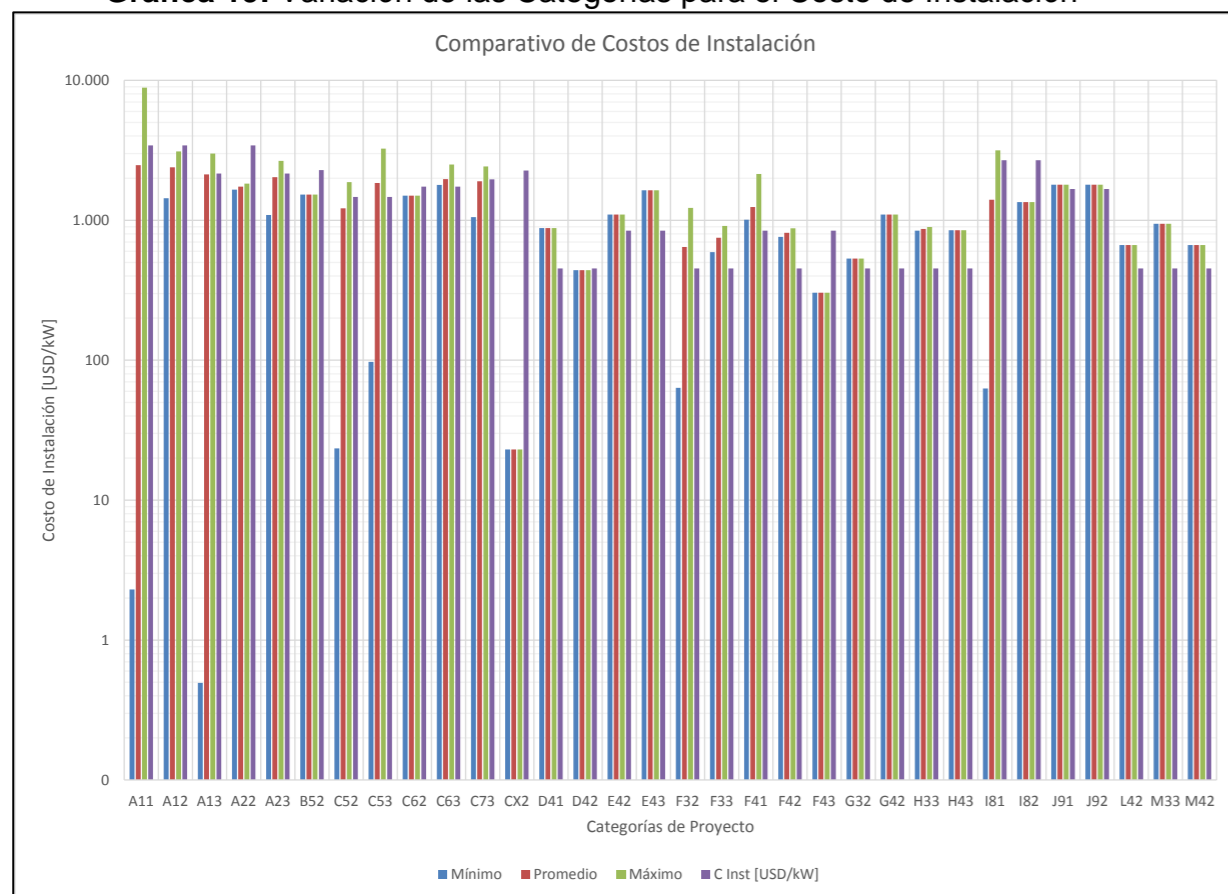
Gráfica 19: Variación de las Categorías para el Costo de Instalación
