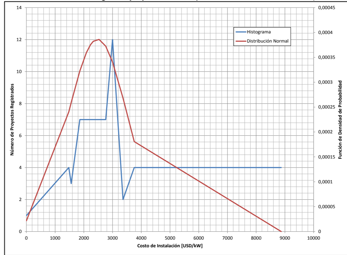
Gráfica 17: Histograma y Ajuste Normal para el Costo de Instalación (Cat. A11)
