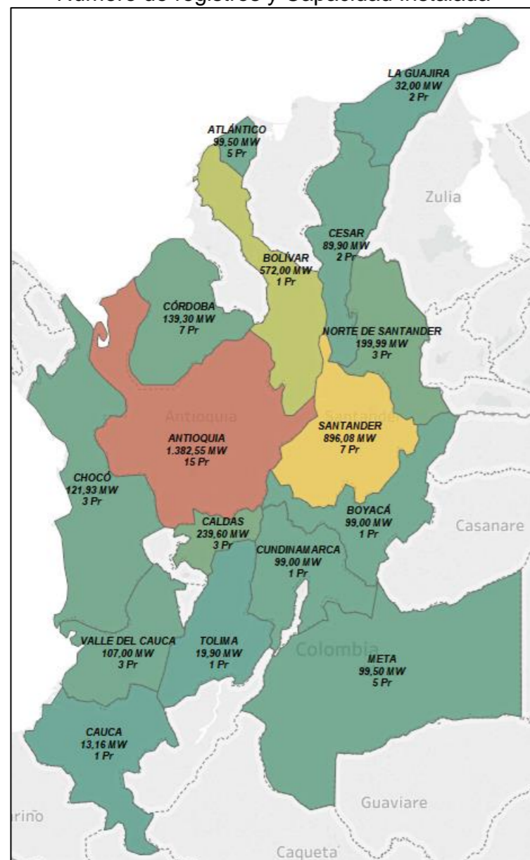
Gráfica 15: Ubicación de proyectos registrados en Fase 2 Número de registros y Capacidad Instalada
