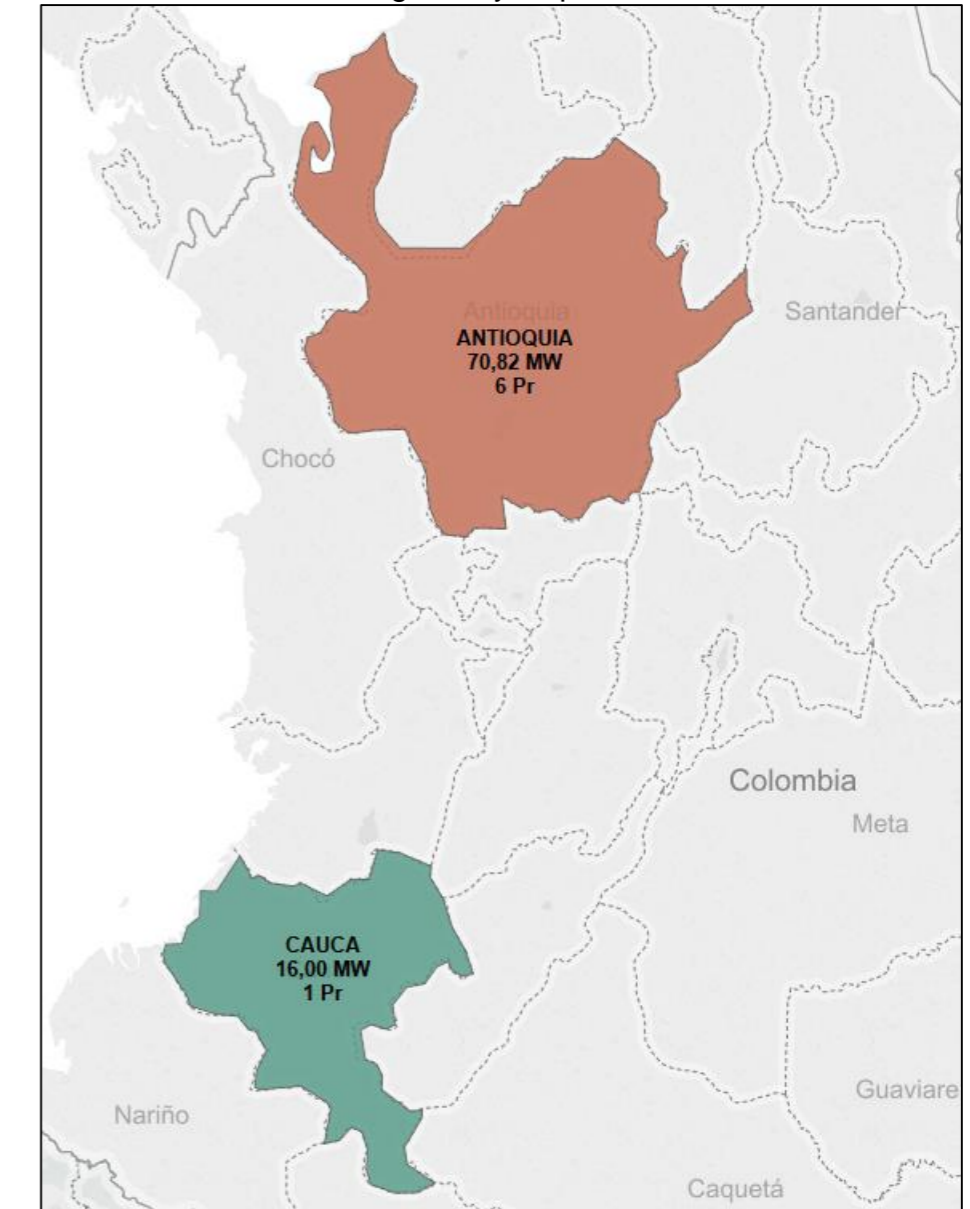
Gráfica 15: Ubicación de proyectos registrados en Fase 3 Número de registros y Capacidad Instalada
