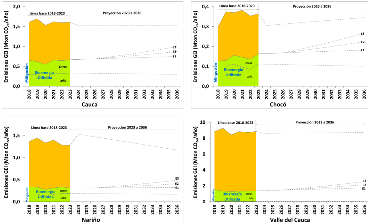
Figura 19. Generación y mitigación (por bioenergía utilizada) de emisiones de CO 2e el periodo 2018 a 2023 y proyecciones 2023 a 2036. Fuente: elaboración UPME con información de (SUI-Superservicios, 2024), (UPRA, 2025), (MinAgricultura, 2025), (UPME, 2023), (MinEnergía, 2025b), (DANE, 2025a).
