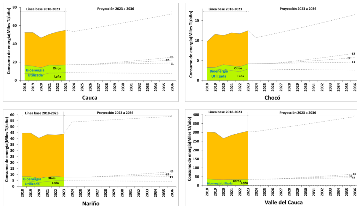
Figura 18. Consumo de energía en el periodo 2018 a 2023 y proyecciones 2023 a 2036. Fuente: elaboración UPME con información de (SUI-Superservicios, 2024), (UPRA, 2025), (MinAgricultura, 2025), (UPME, 2023), (MinEnergía, 2025b), (DANE, 2025a).
