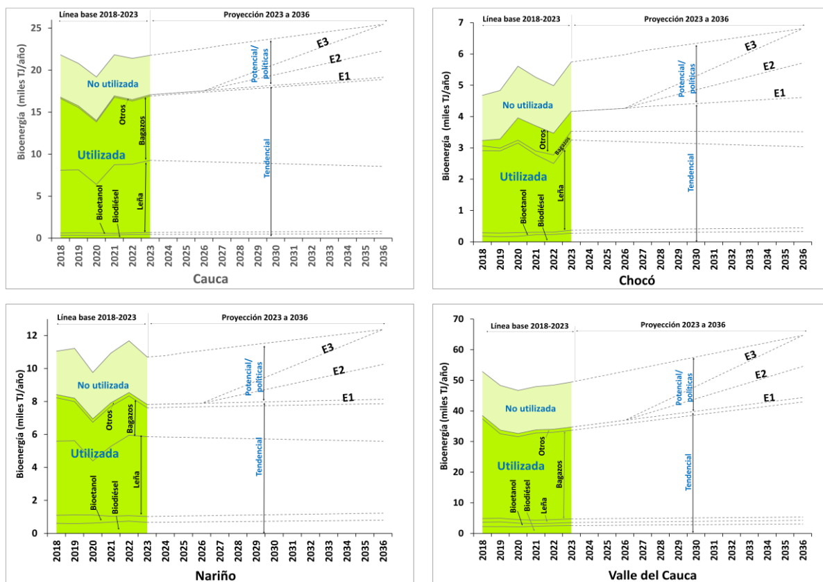
Figura 17. Potencial de bioenergía utilizada y no utilizada entre 2018 a 2023 y proyecciones 2023 a 2036 para la región del Pacífico. Fuente: elaboración UPME con información de (SUI-Superservicios, 2024), (UPRA, 2025), (MinAgricultura, 2025), (UPME, 2023), (MinEnergía, 2025b).
