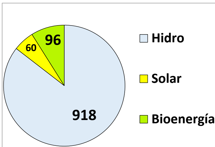
Figura 4. Capacidad efectiva neta instalada por tecnología Fuente: elaboración UPME con información de (UPME, 2025a).
