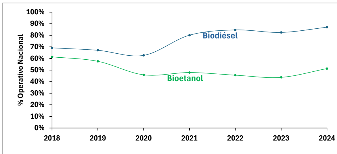
Figura 22. Porcentaje operativo (despachos) 2018-2024 de las plantas de biodiésel y bioetanol. Fuente: elaboración UPME con información de (MinEnergía, 2025b), (Fedebiocombustibles, 2024a).
