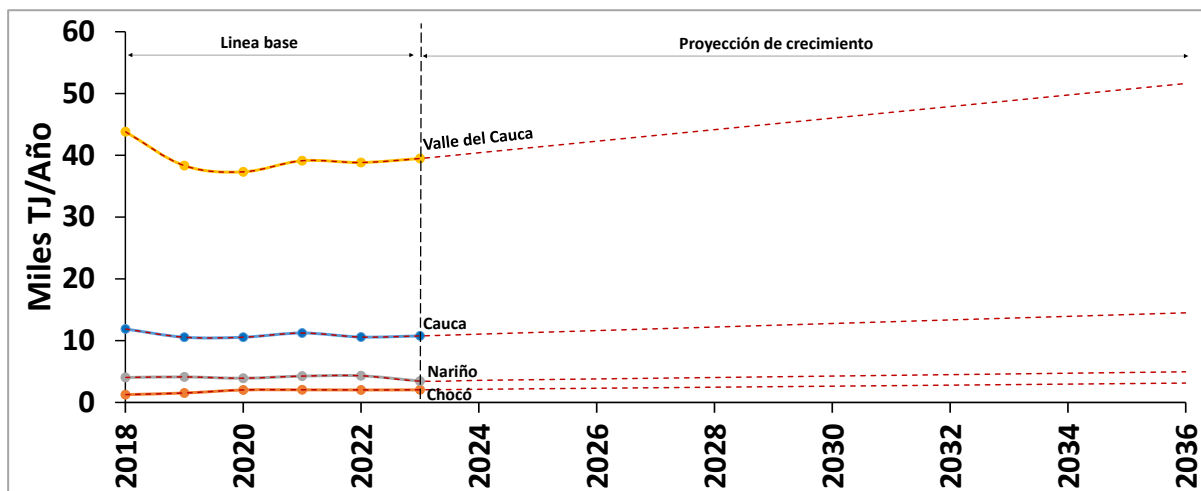
Figura 11. Línea base y proyección de crecimiento del potencial bioenergético técnico de residuos/subproductos agrícolas y forestales que incluyen biogás y aplicaciones termoquímicas.
