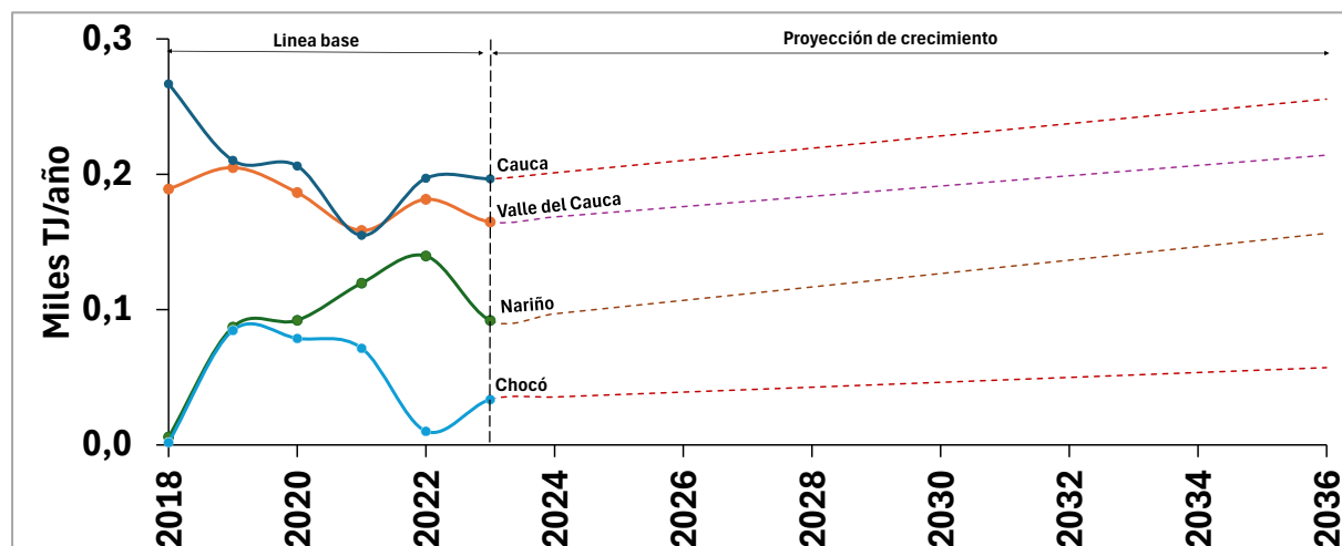
Figura 12. Línea base y proyección del potencial bioenergético técnico de solo residuos/subproductos forestales. Fuente: elaboración UPME con información de (MinAgricultura, 2025).
