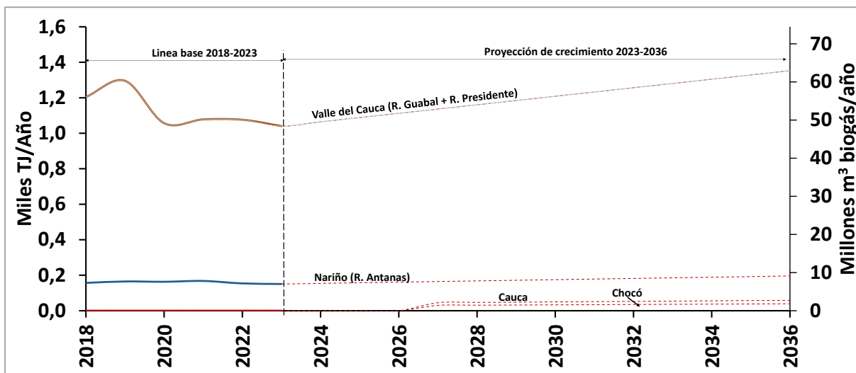
Figura 15. Línea base del potencial bioenergético técnico de rellenos sanitarios. Fuente: elaboración UPME con información de (SUI-Superservicios, 2024).
