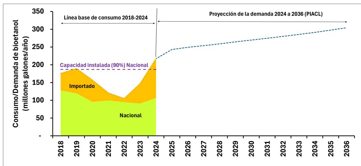
Figura 20. Consumo y Proyección de demanda nacional de bioetanol. Fuente: elaboración UPME con información de (MinEnergía, 2025b), (Fedebiocombustibles, 2024a).
