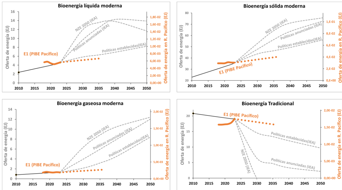
Figura 28. Escenarios prospectivos de bioenergía moderna y tradicional de la IEA y el escenario E1 del PIBE Pacífico. Fuente: elaboración UPME con información de (IEA, 2024).
