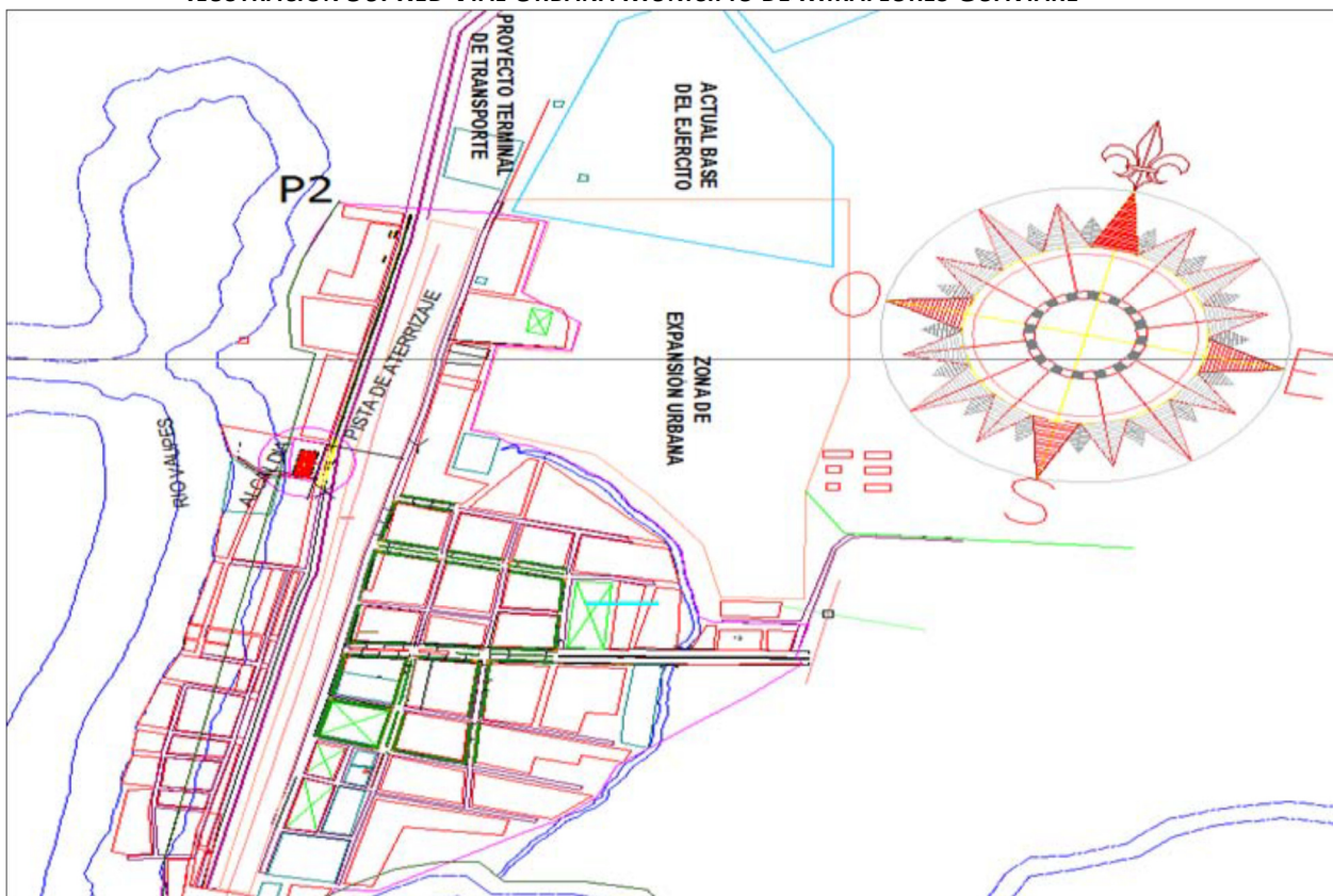
ILUSTRACIÓN 56. RED VIAL URBANA MUNICIPIO DE MIRAFLORES GUAVIARE
