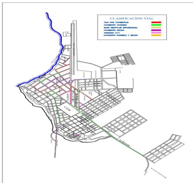
ILUSTRACIÓN 45. RED VIAL URBANA MUNICIPIO SAN JOSÉ DEL GUAVIARE
