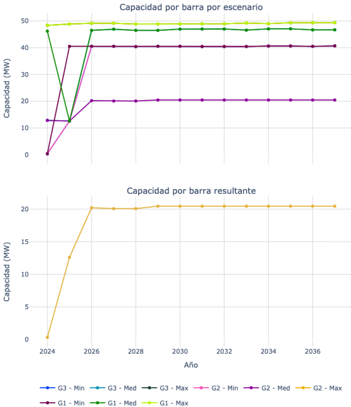
Figura 43. Capacidad de transporte de la subestación Jamundi 34.5 kV.
