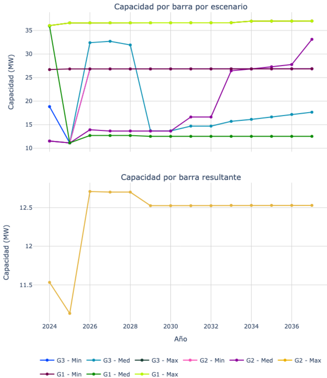
Figura 75. Capacidad de transporte de la subestación Santa Maria 34.5.
