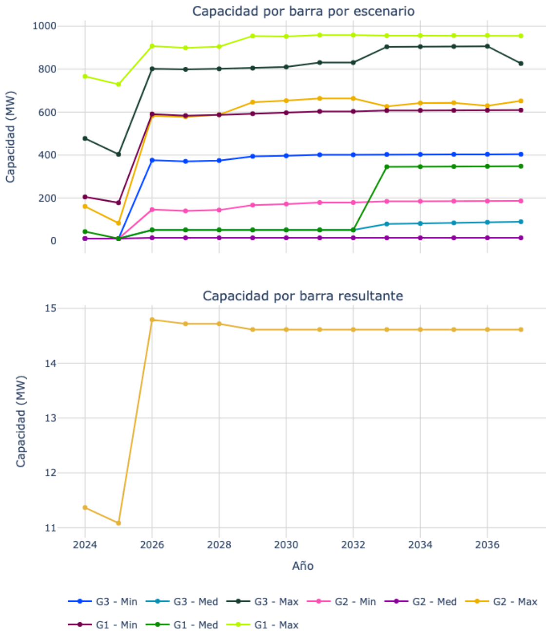
Figura 71. Capacidad de transporte de la subestación San Marcos 220.
