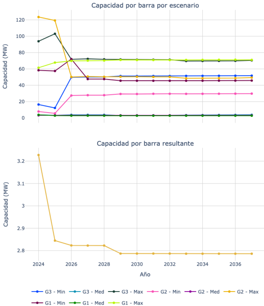
Figura 82. Capacidad de transporte de la subestación Tulua 115.
