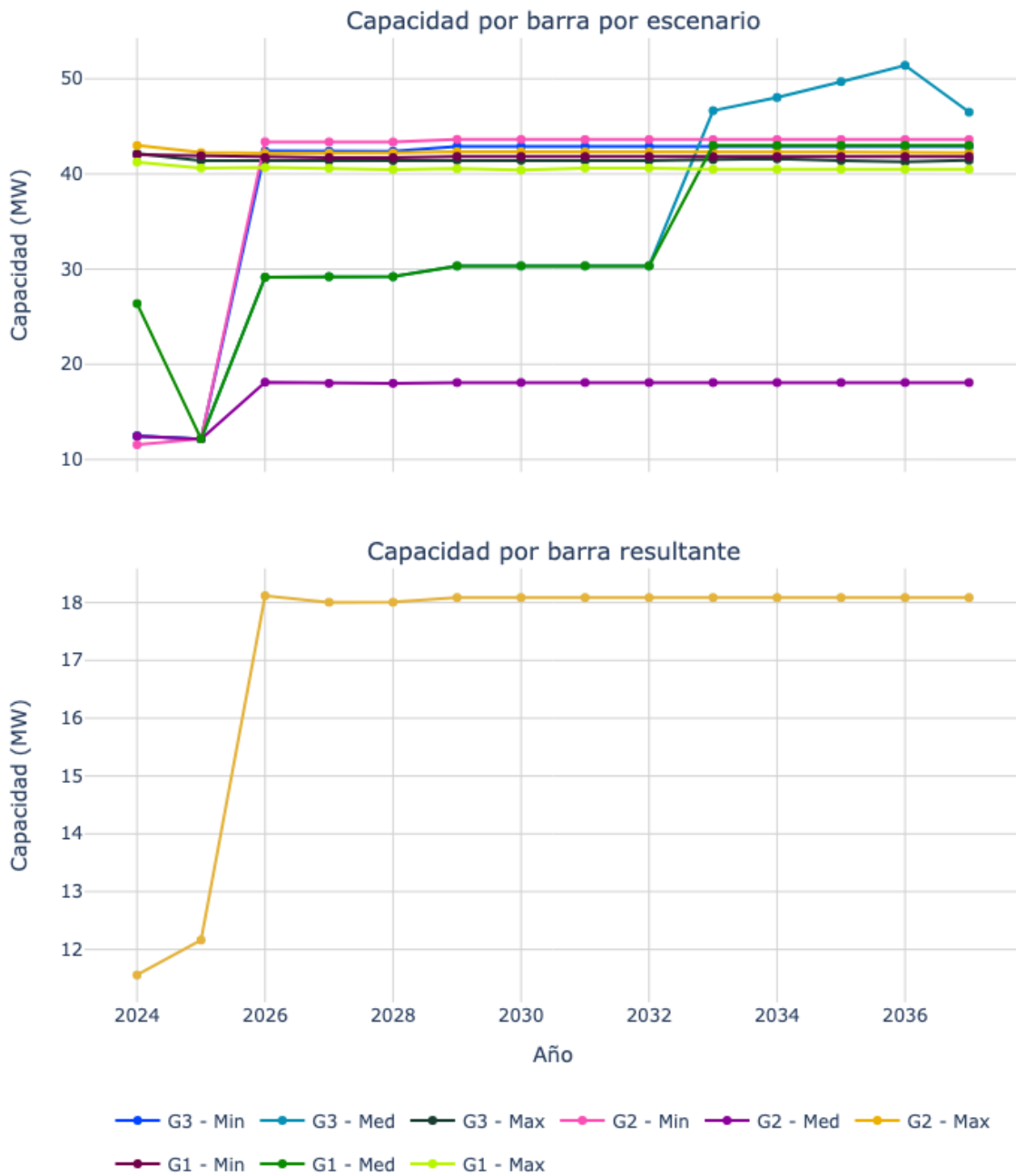
Figura 60. Capacidad de transporte de la subestación Palmaseca 34.5.
