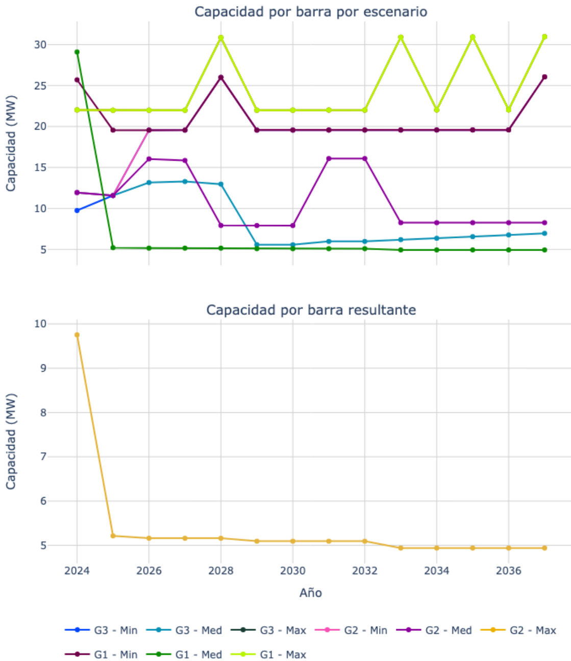
Figura 66. Capacidad de transporte de la subestación Roldanillo 34.5.
