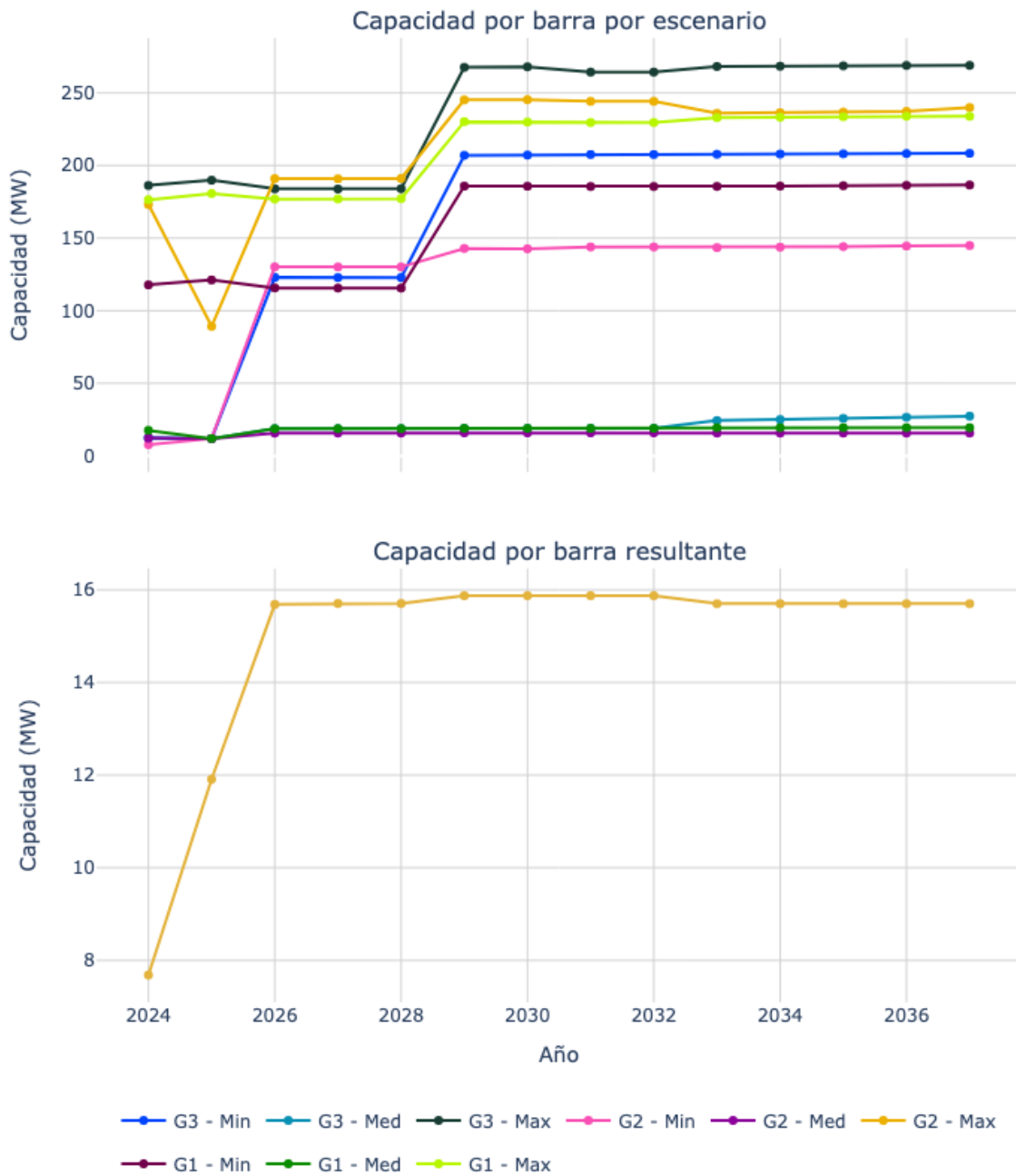
Figura 41. Capacidad de transporte de la subestación Guachal 115.
