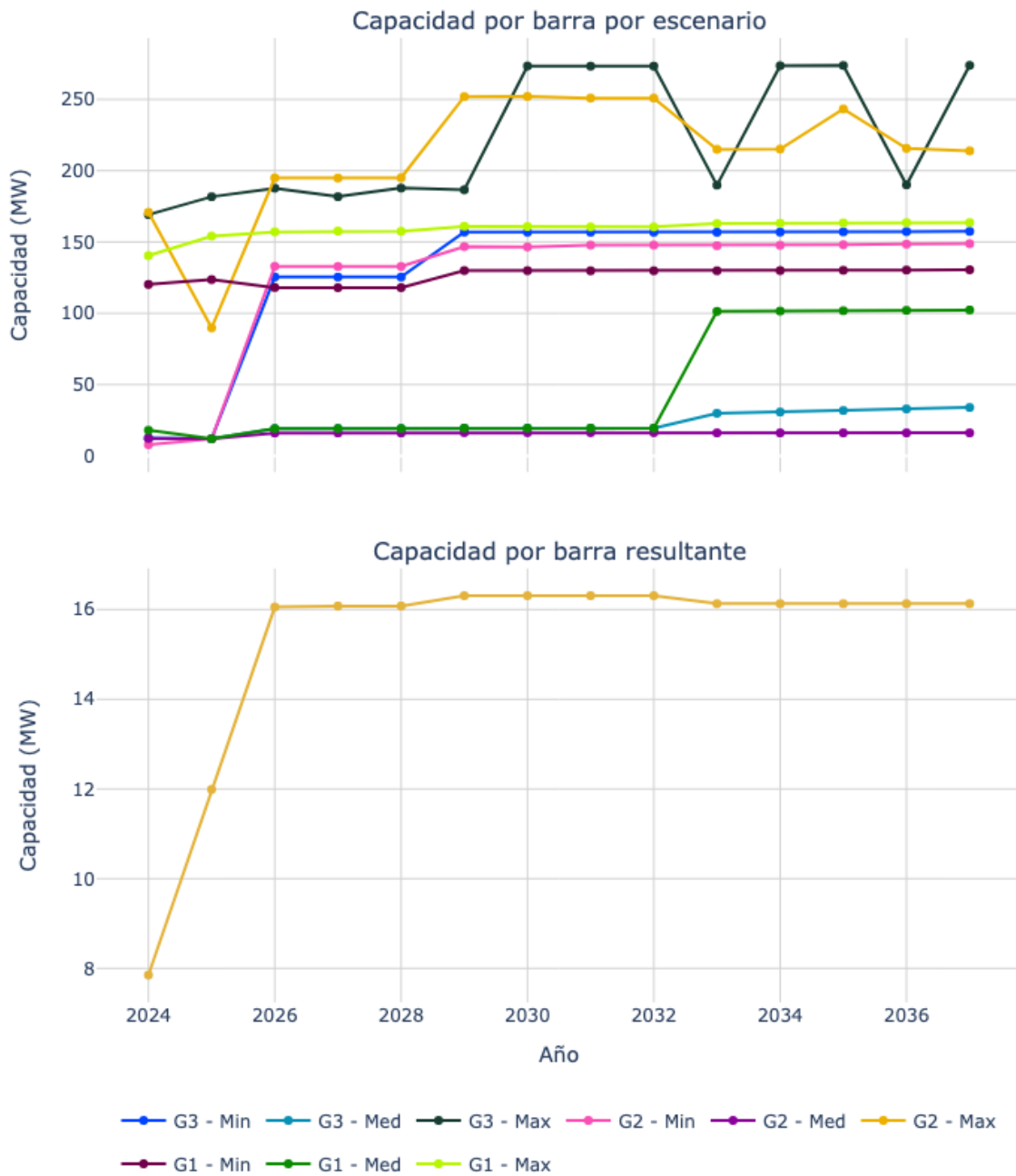
Figura 51. Capacidad de transporte de la subestación Las Palmas 115.
