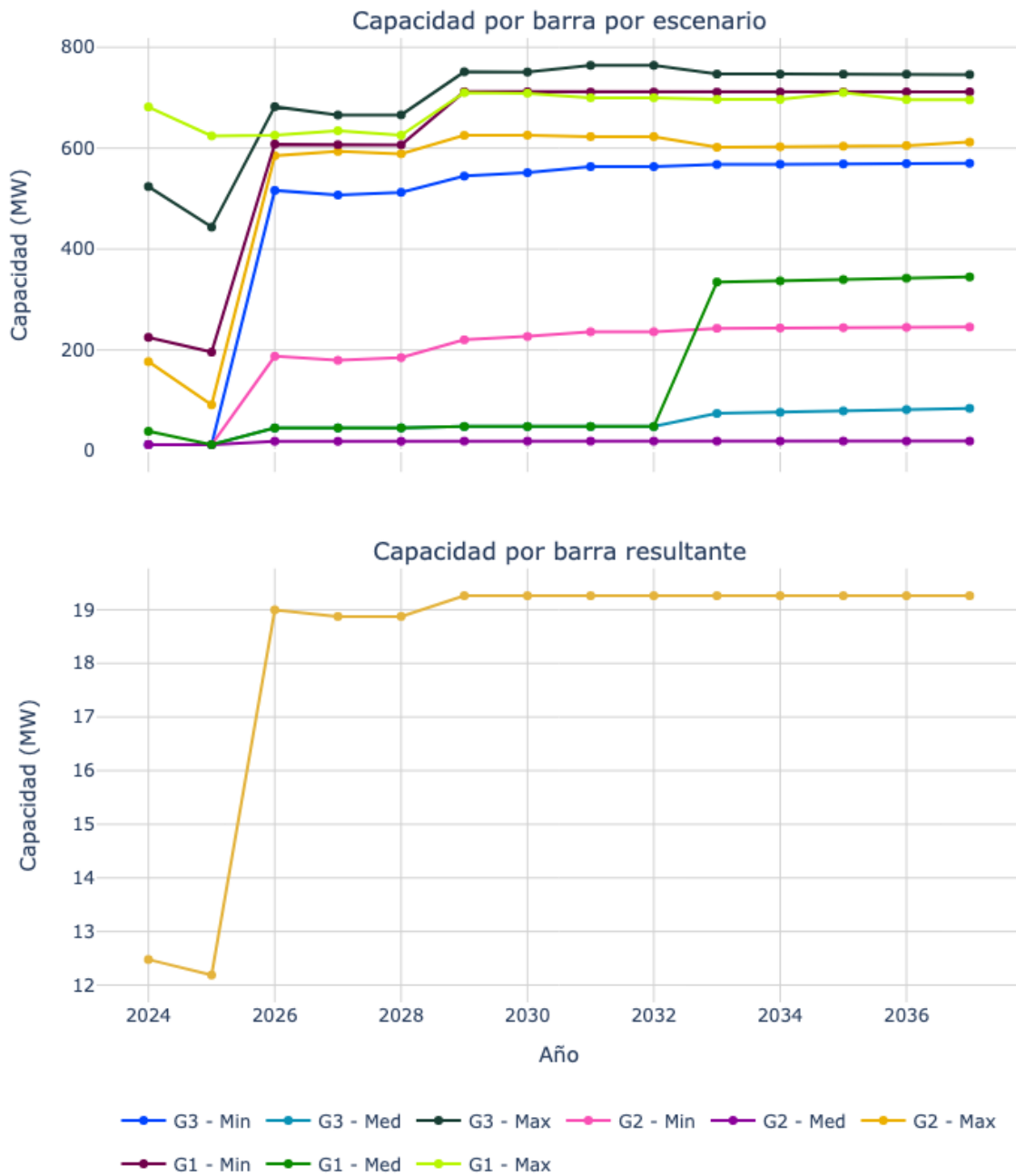
Figura 46. Capacidad de transporte de la subestación Juanchito 220 (115).
