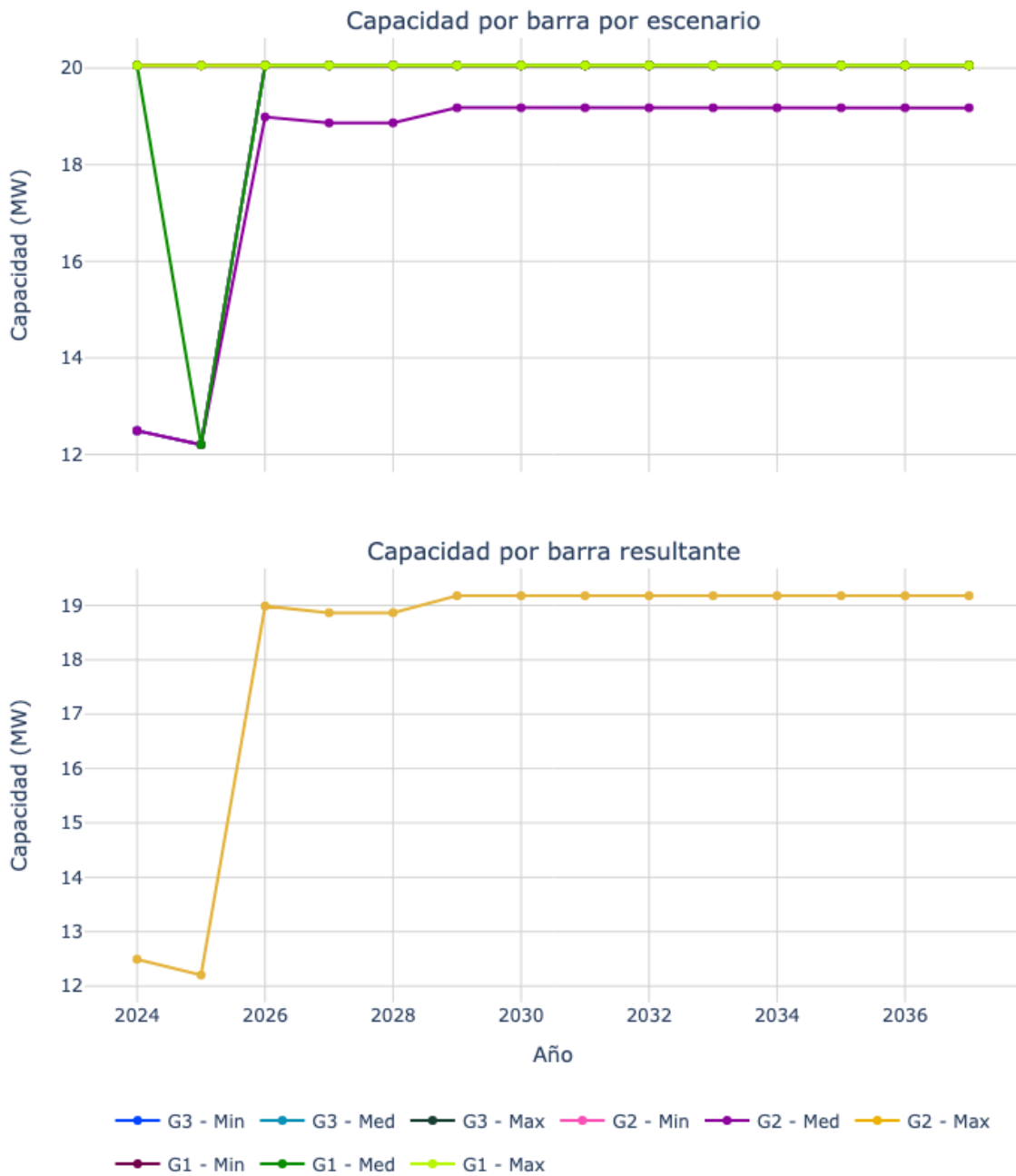
Figura 54. Capacidad de transporte de la subestación Mayaguez 115.
