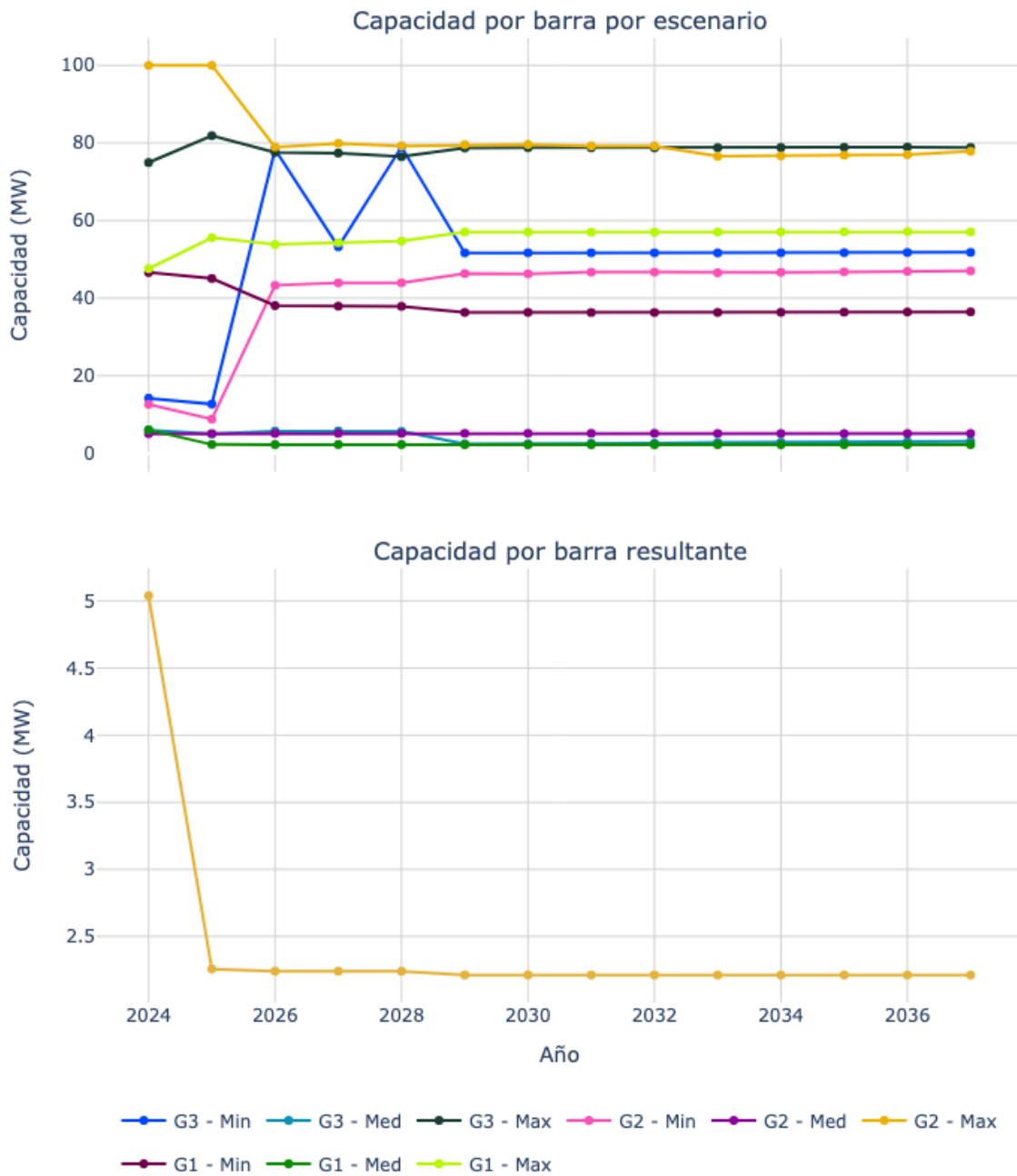
Figura 53. Capacidad de transporte de la subestación Loboguerrero 34.5.
