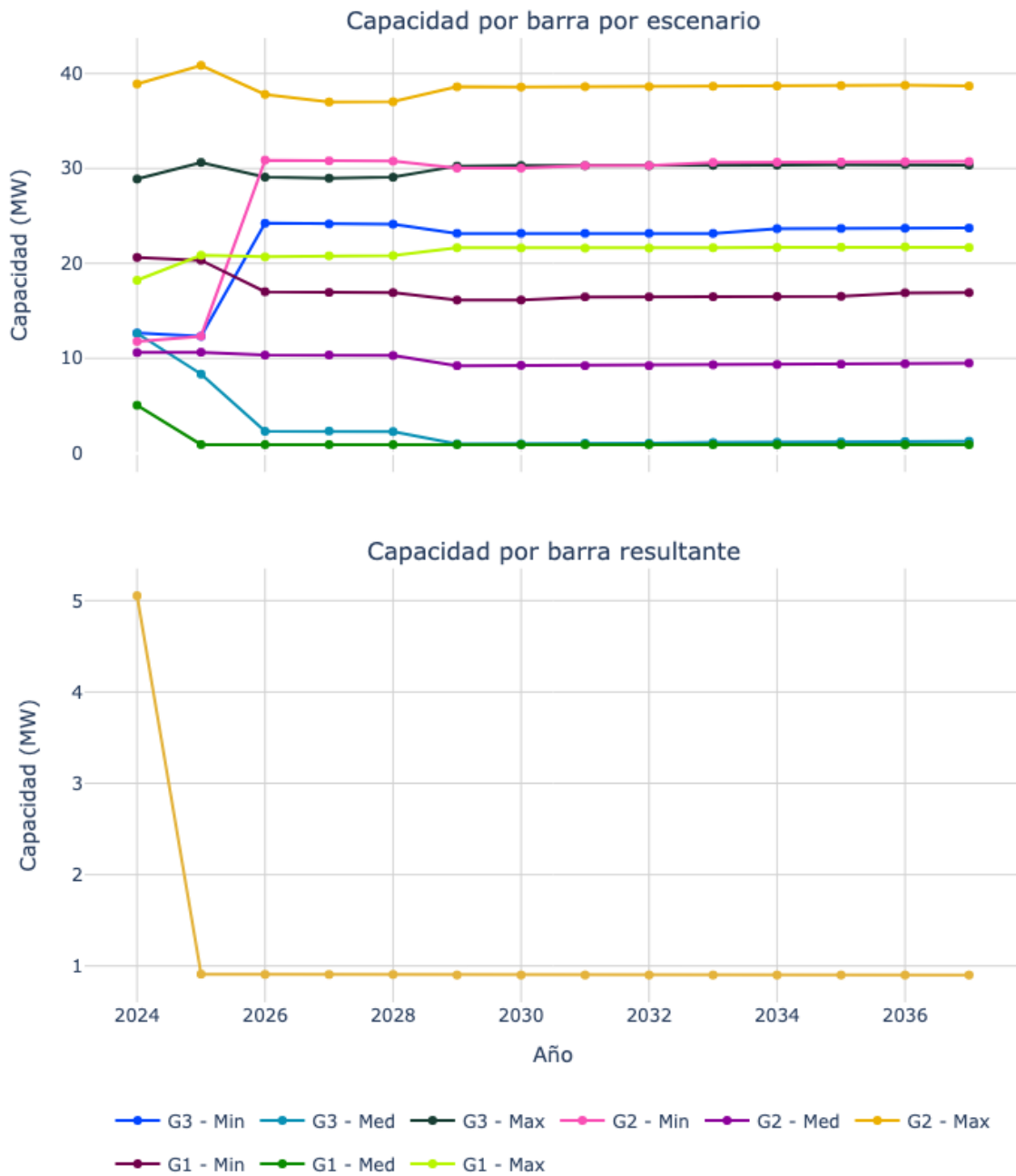
Figura 65. Capacidad de transporte de la subestación Providencia 115.
