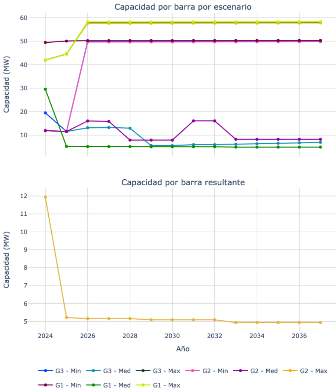
Figura 49. Capacidad de transporte de la subestación La Union 34.5.
