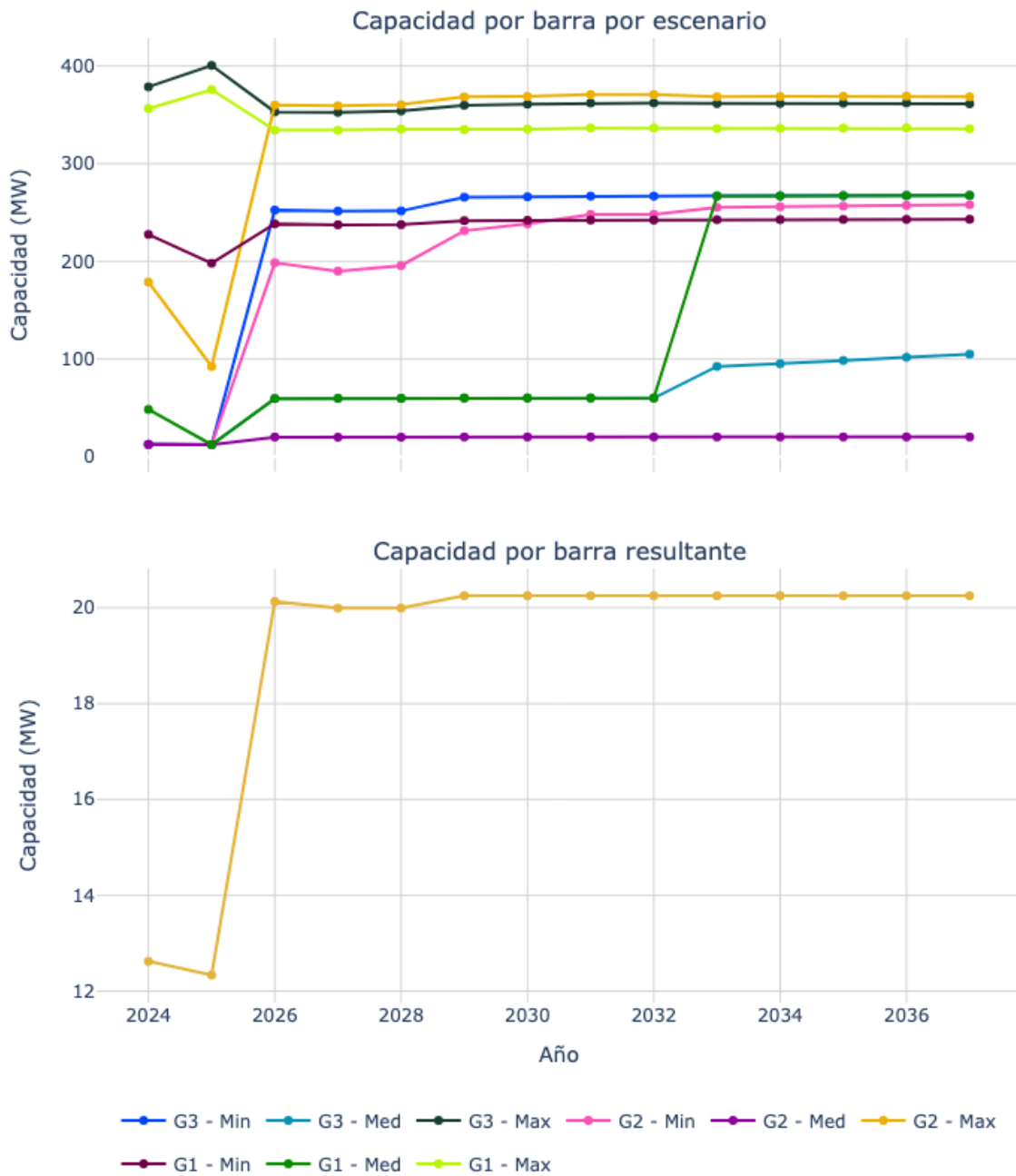
Figura 62. Capacidad de transporte de la subestación Pance 220.
