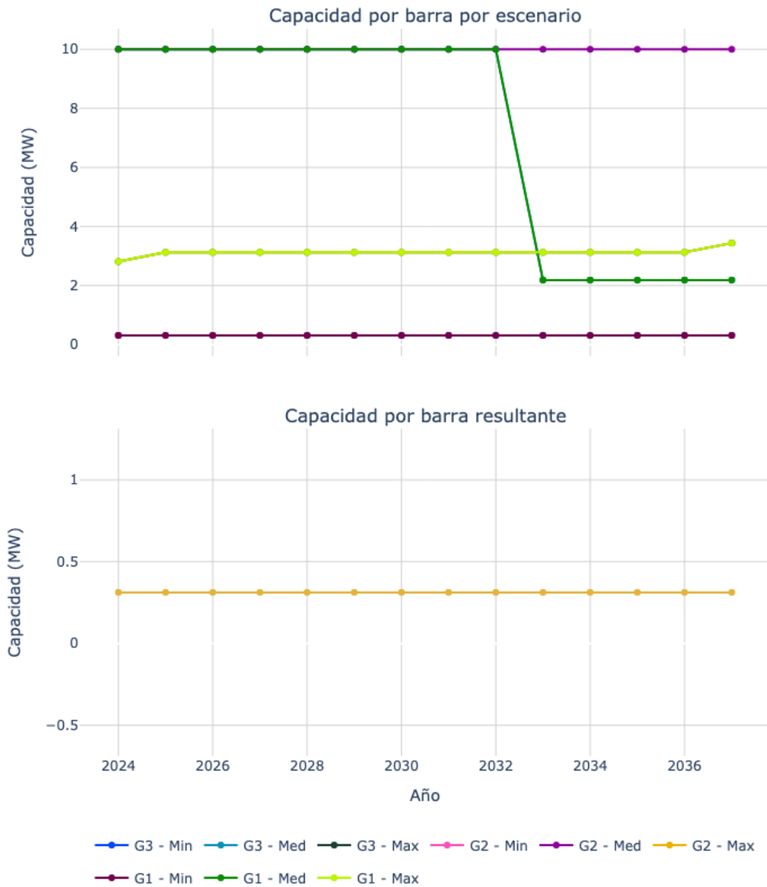
Figura 52. Capacidad de transporte de la subestación Las Palmas 34.5.
