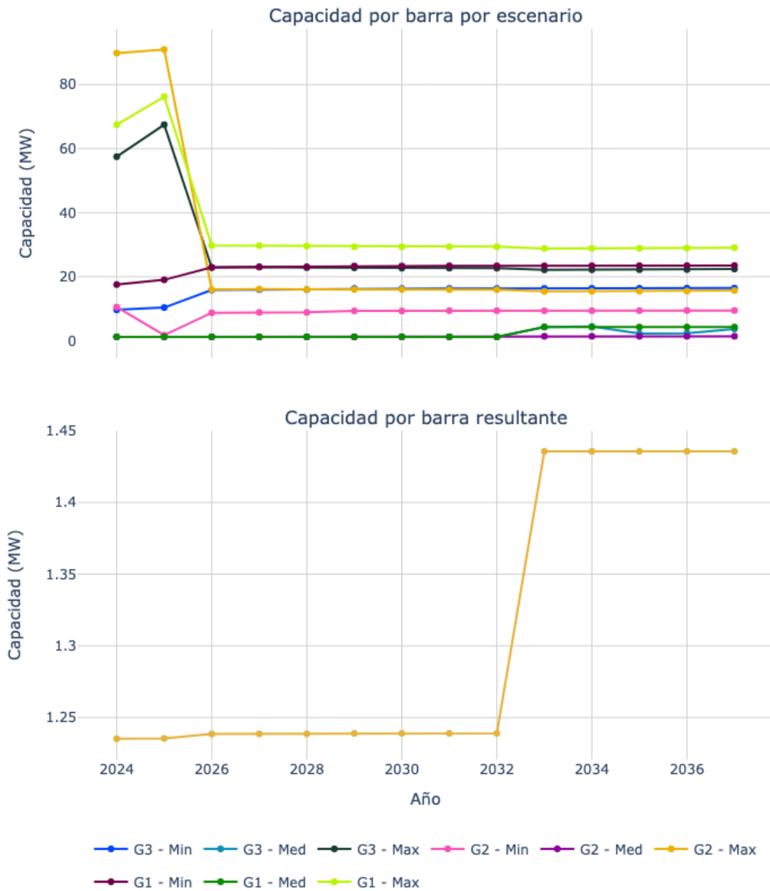
Figura 89. Capacidad de transporte de la subestación Zarzal 34.5.
