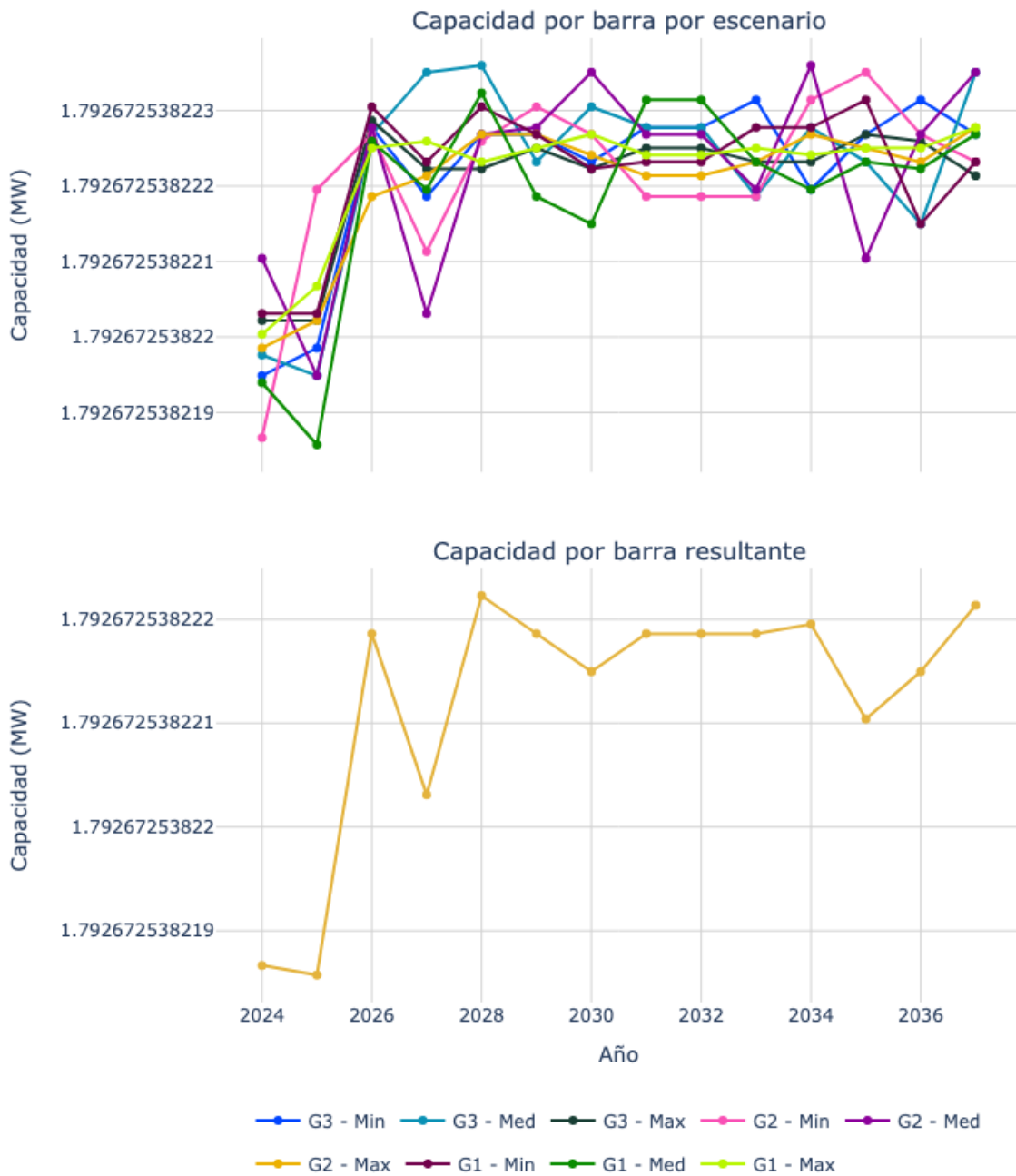
Figura 80. Capacidad de transporte de la subestación Termovalle 115.
