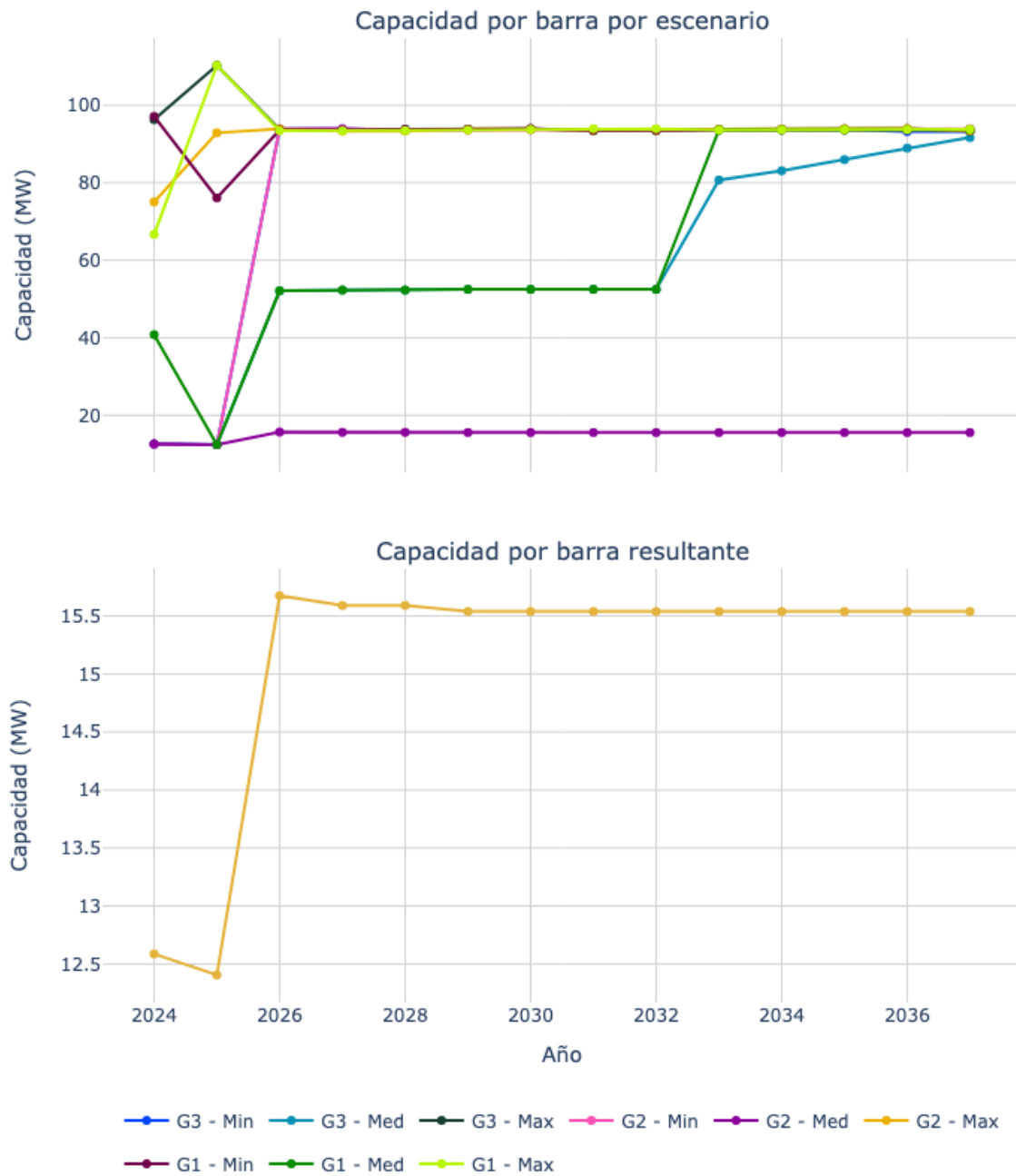
Figura 79. Capacidad de transporte de la subestación Tabor (Bventura) 115.
