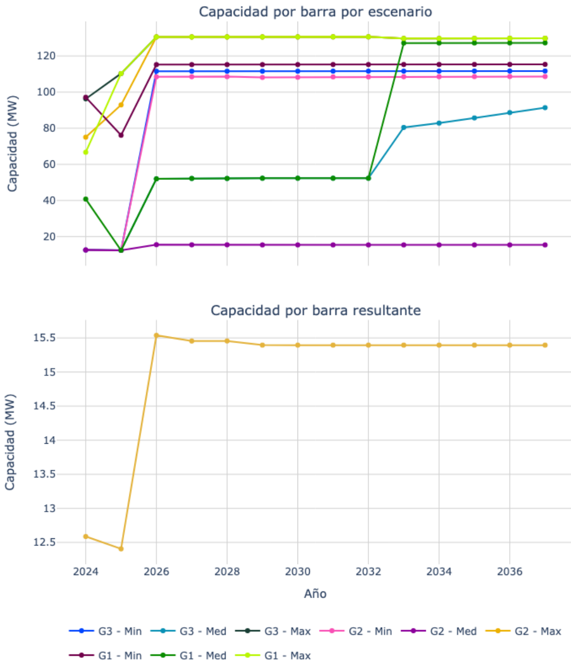
Figura 58. Capacidad de transporte de la subestación Pailon 115.
