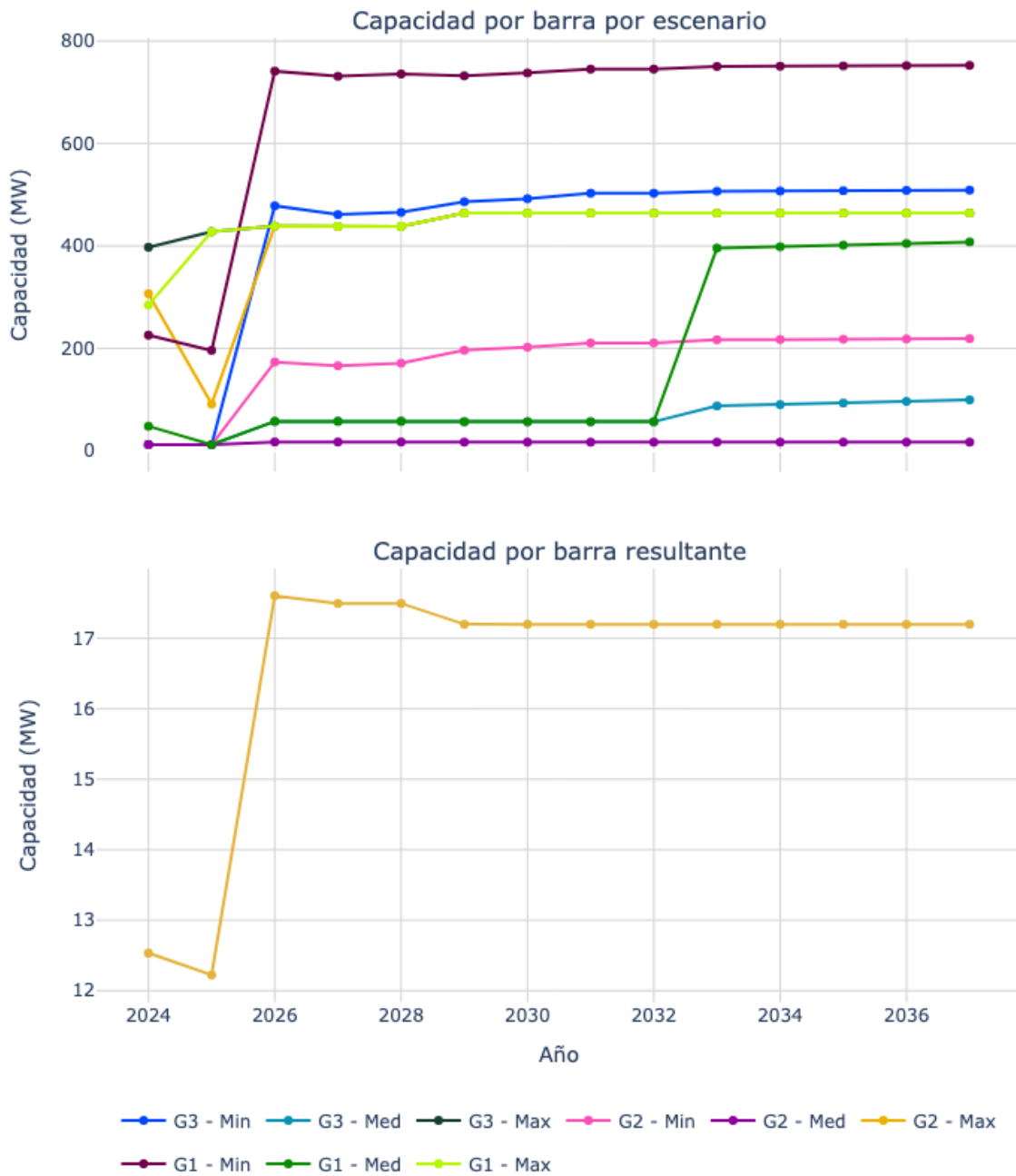
Figura 87. Capacidad de transporte de la subestación Yumbo 220.
