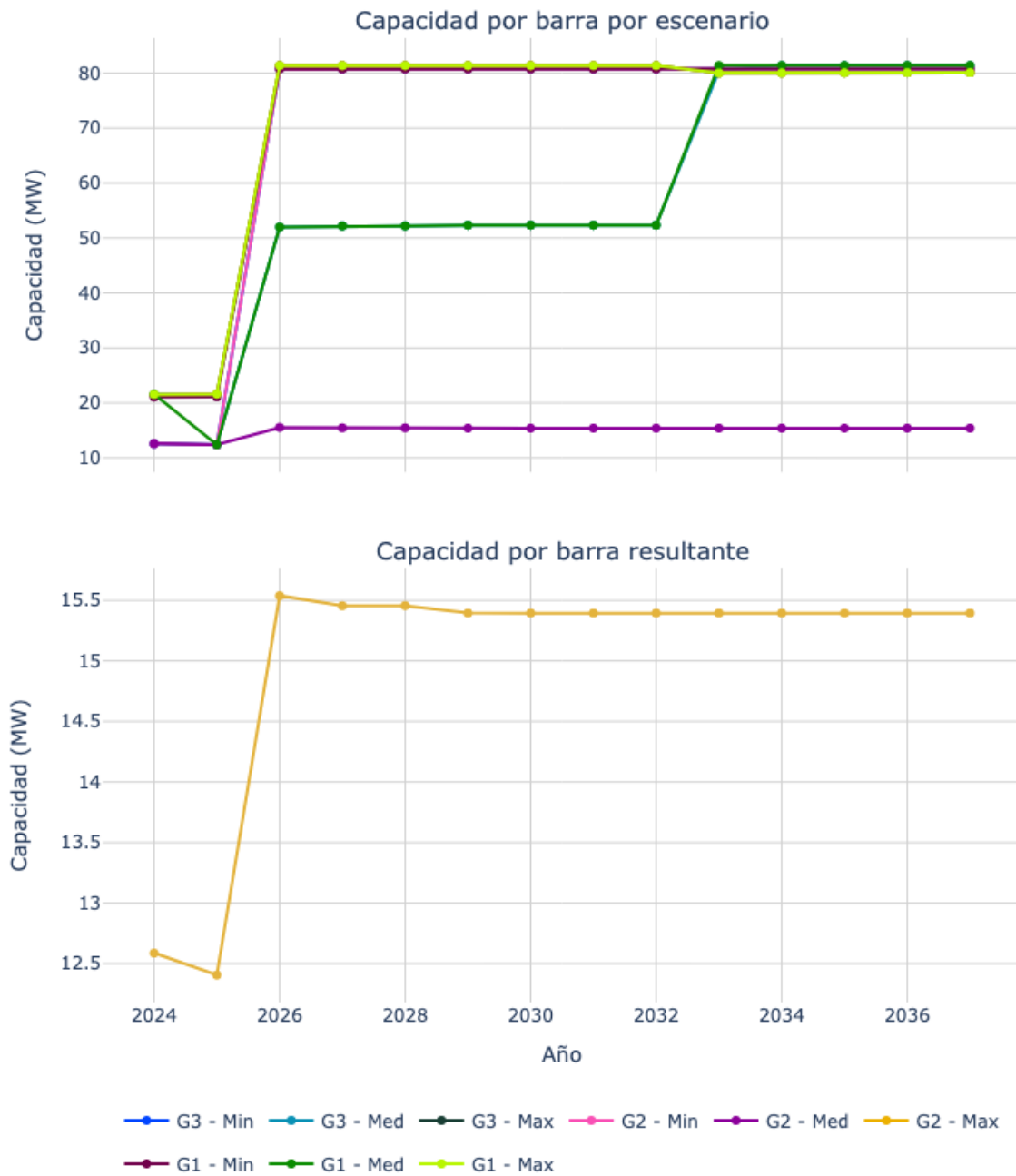
Figura 17. Capacidad de transporte de la subestación BMalaga 115.
