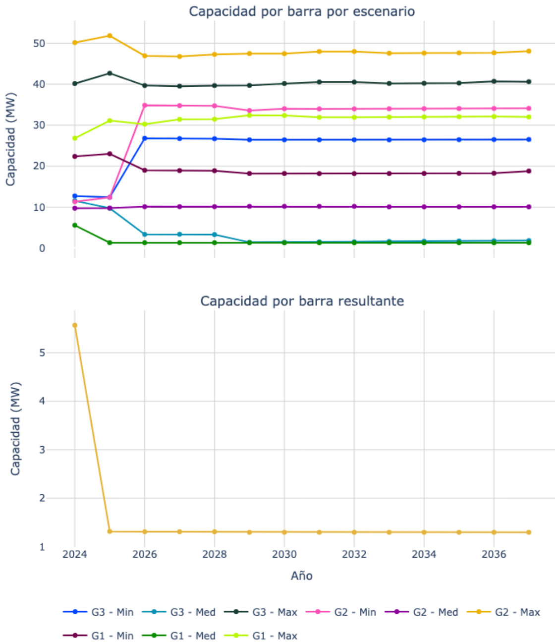
Figura 84. Capacidad de transporte de la subestación Vijes 115.
