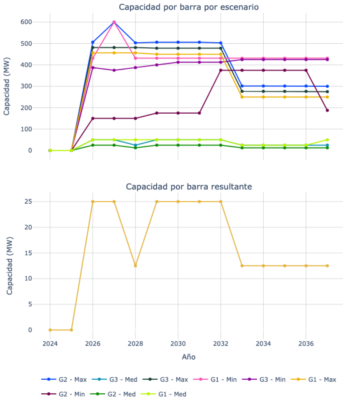
Figura 57. Capacidad de transporte de la subestación Pacifico 220.
