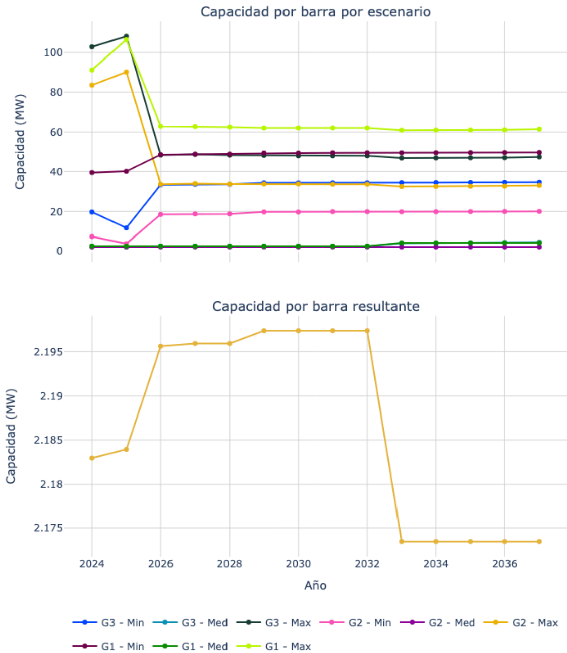
Figura 88. Capacidad de transporte de la subestación Zarzal 115.
