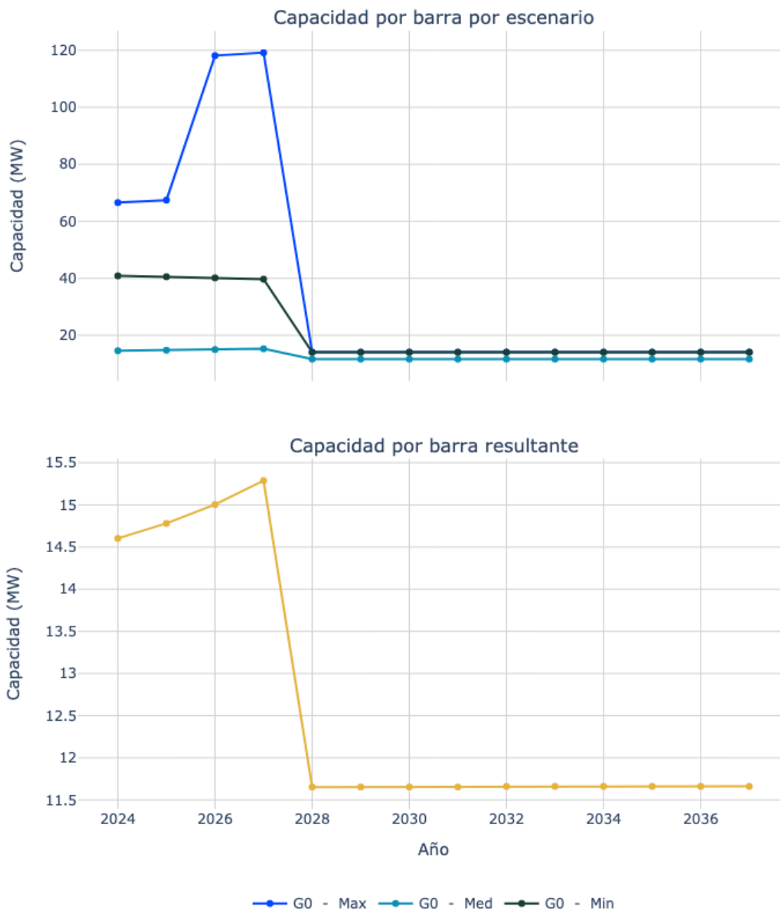
Figura 124. Capacidad de transporte de la subestación SAN JUAN 1 13.8 kV.
