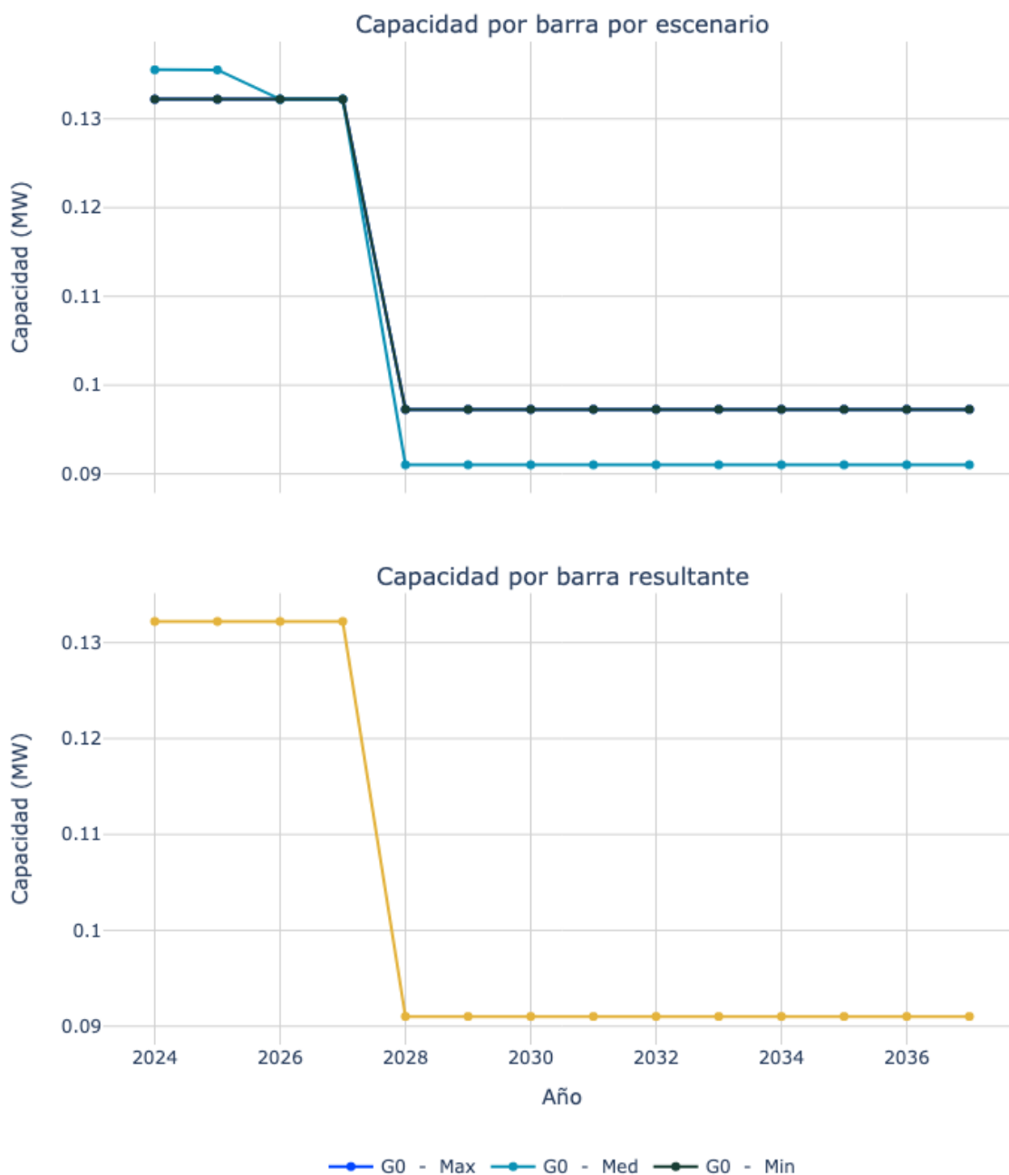
Figura 130. Capacidad de transporte de la subestación Santa Elena 34.5.
