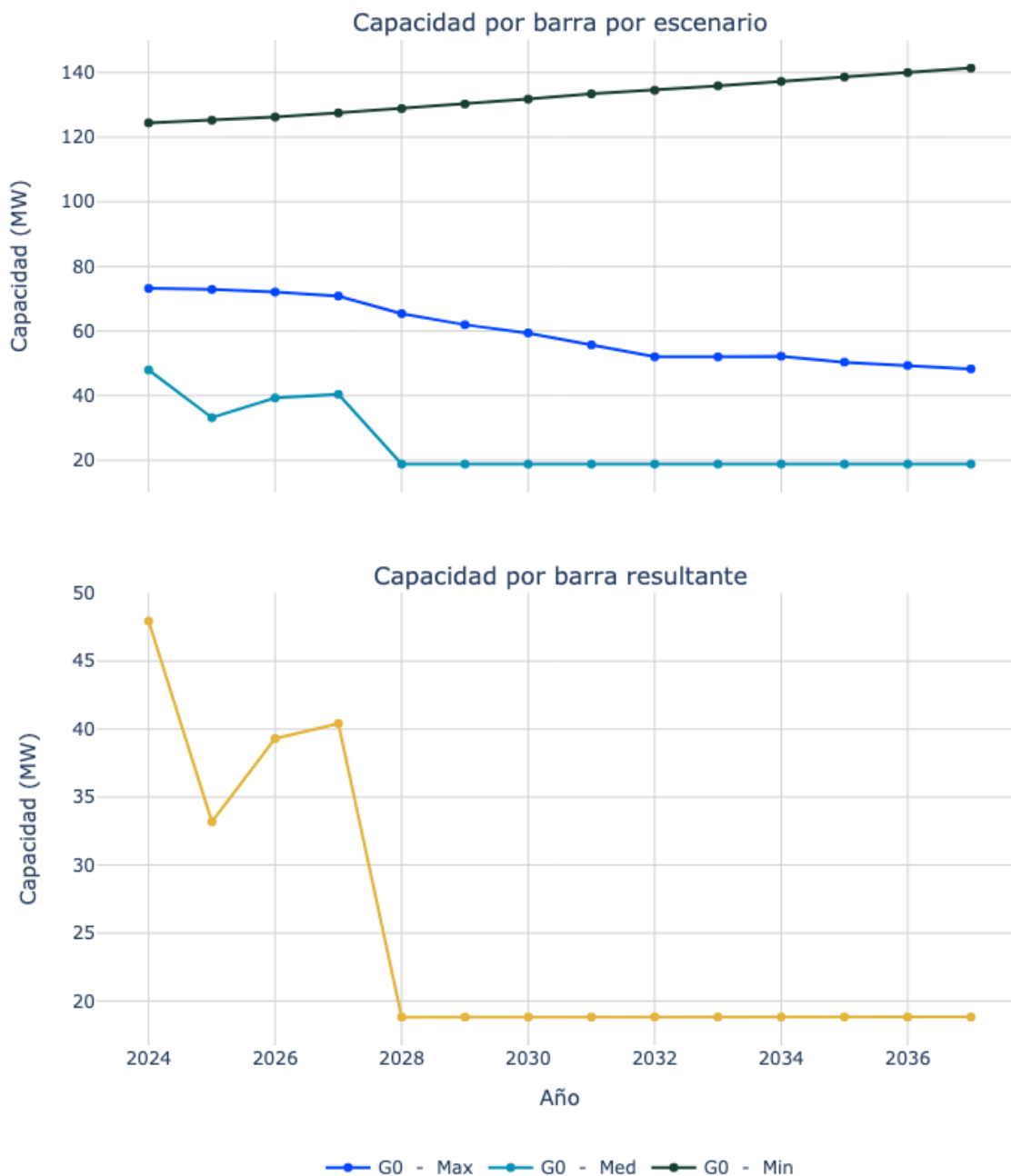
Figura 85. Capacidad de transporte de la subestación La Jagua 110.
