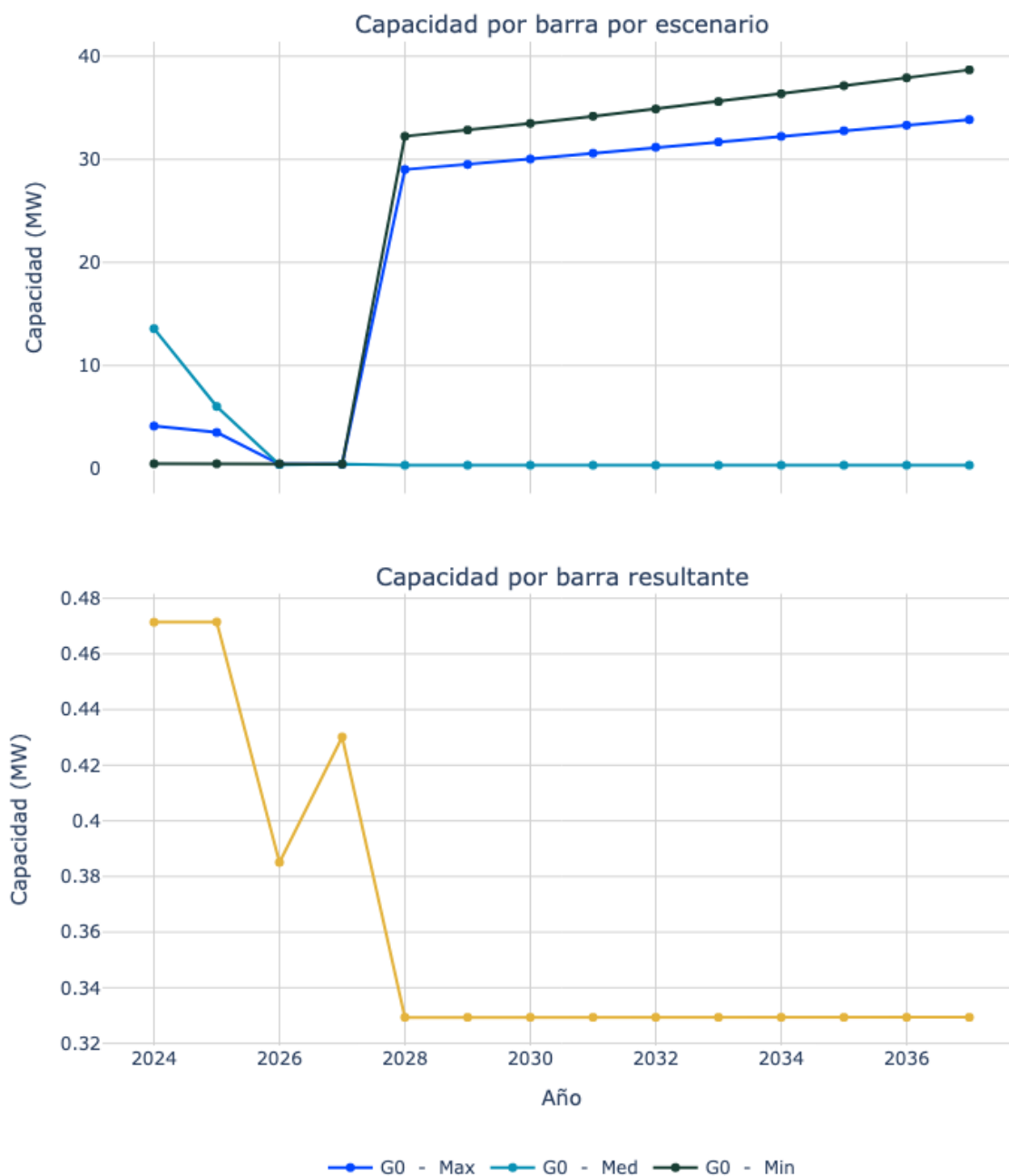
Figura 51. Capacidad de transporte de la subestación Curumani 34.5.
