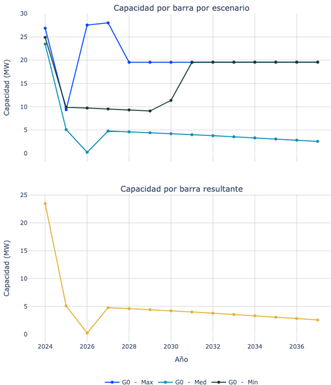
Figura 117. Capacidad de transporte de la subestación RIOHACHA 2 34.5 kV.
