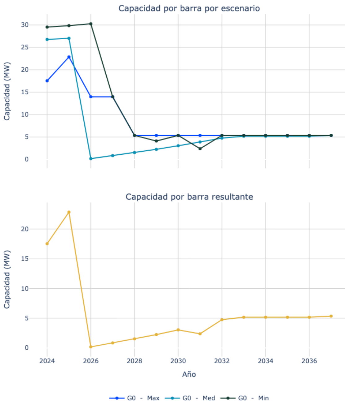
Figura 31. Capacidad de transporte de la subestación CODAZZI (CESAR) 1 13.8 kV.
