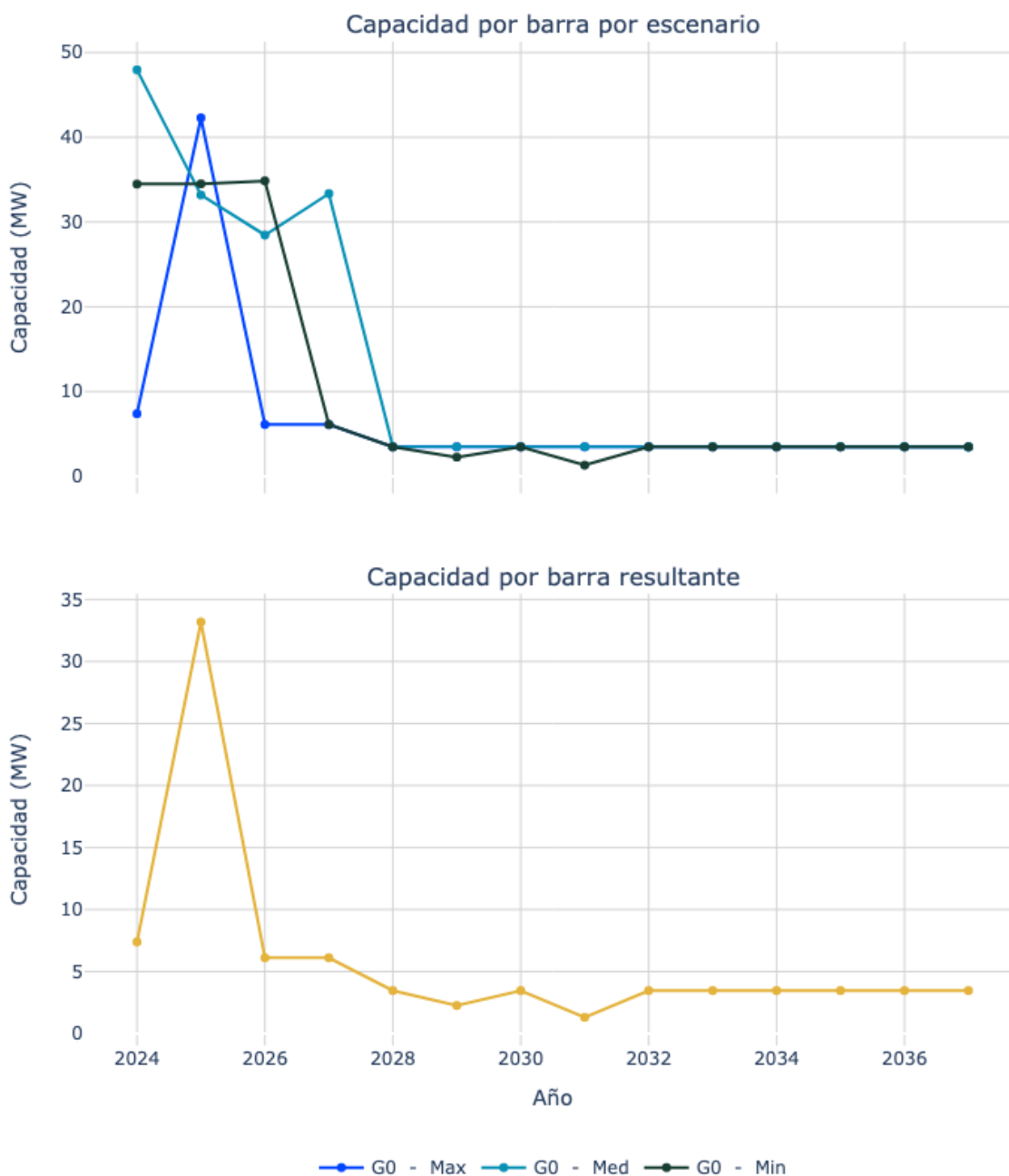
Figura 80. Capacidad de transporte de la subestación LA JAGUA 1 34.5 kV.
