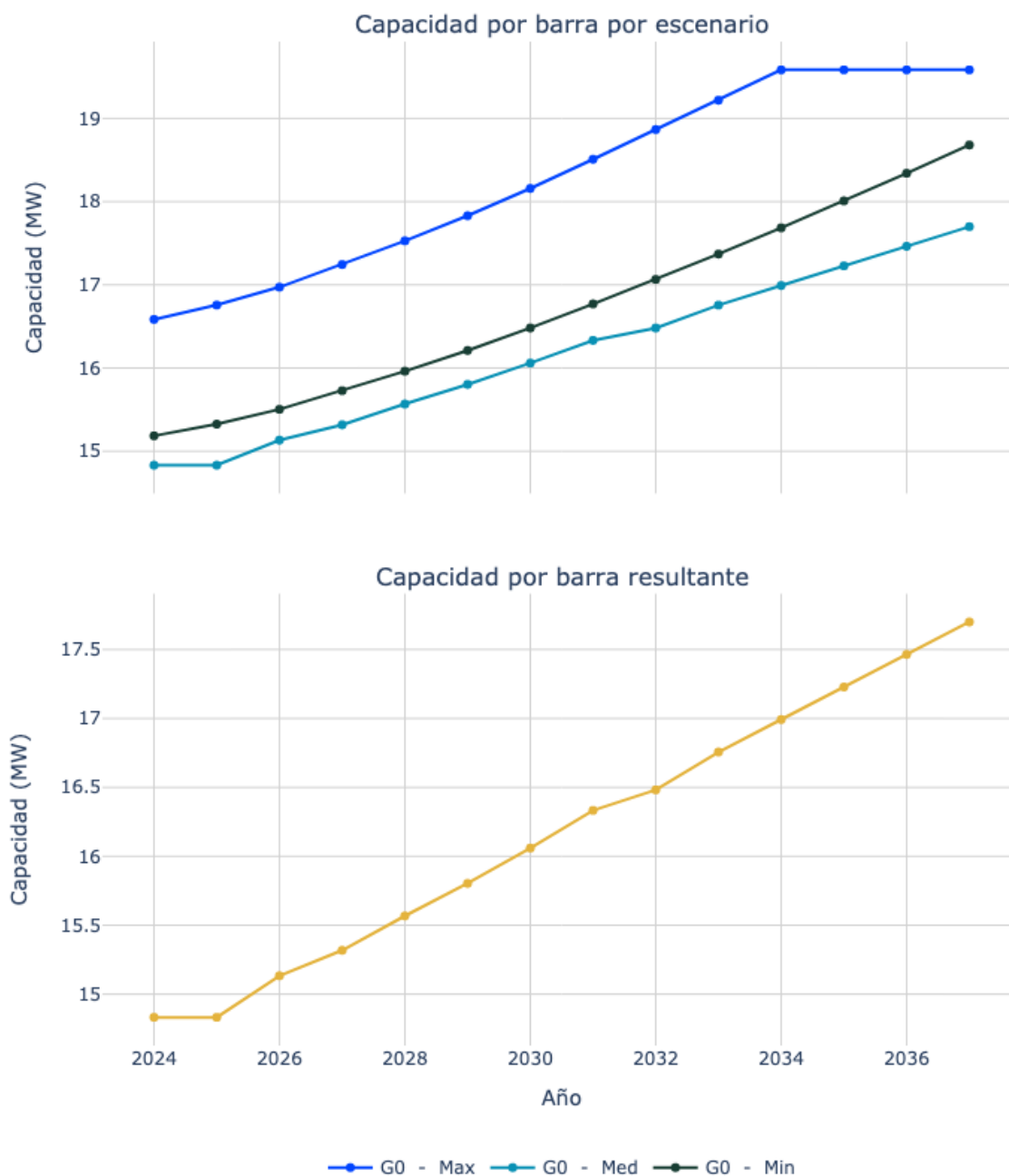
Figura 141. Capacidad de transporte de la subestación Uribea 34.5.
