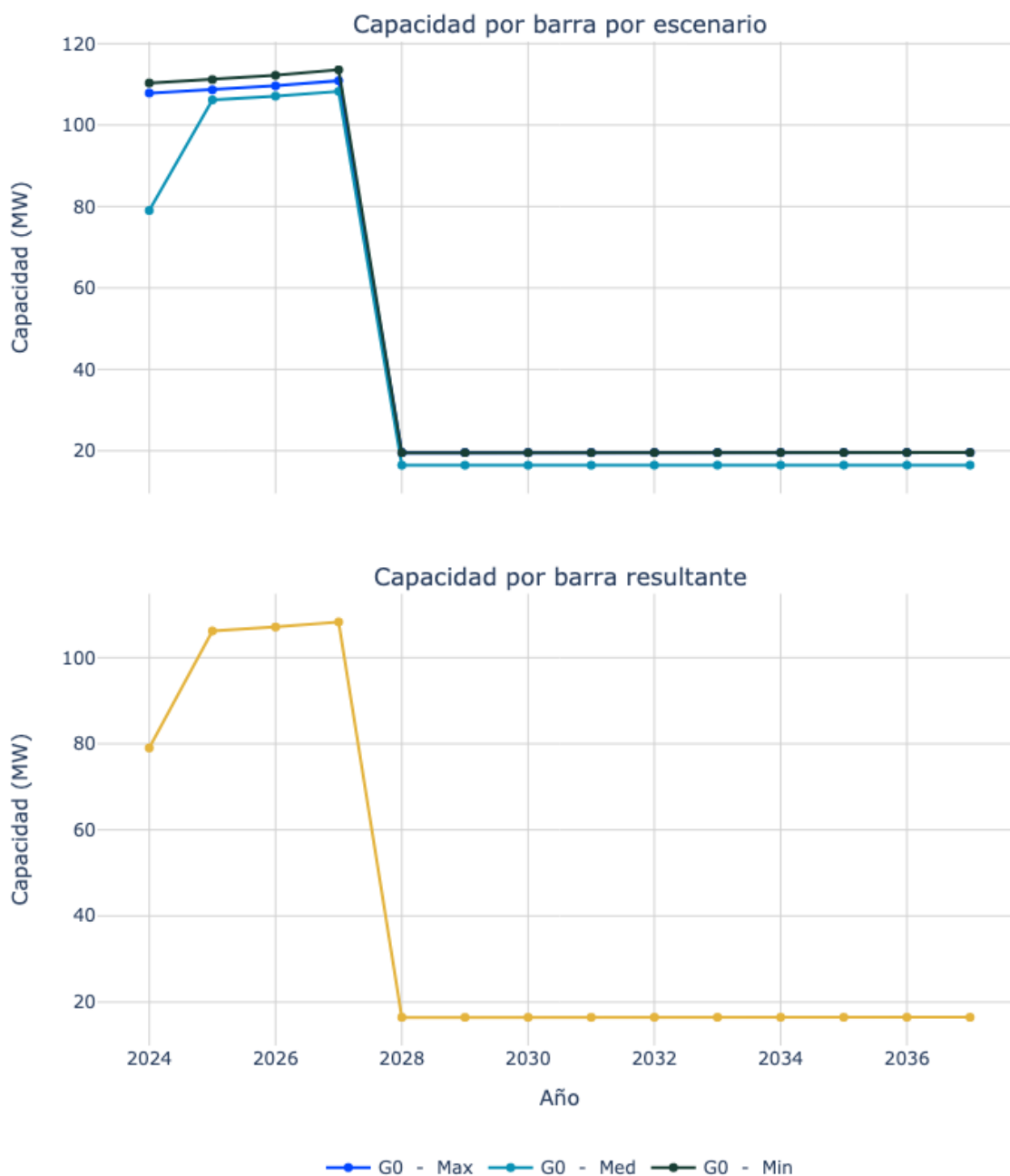
Figura 95. Capacidad de transporte de la subestación MAICAO 1 13.8 kV.
