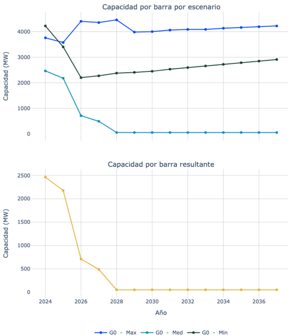
Figura 87. Capacidad de transporte de la subestación La Loma 500.
