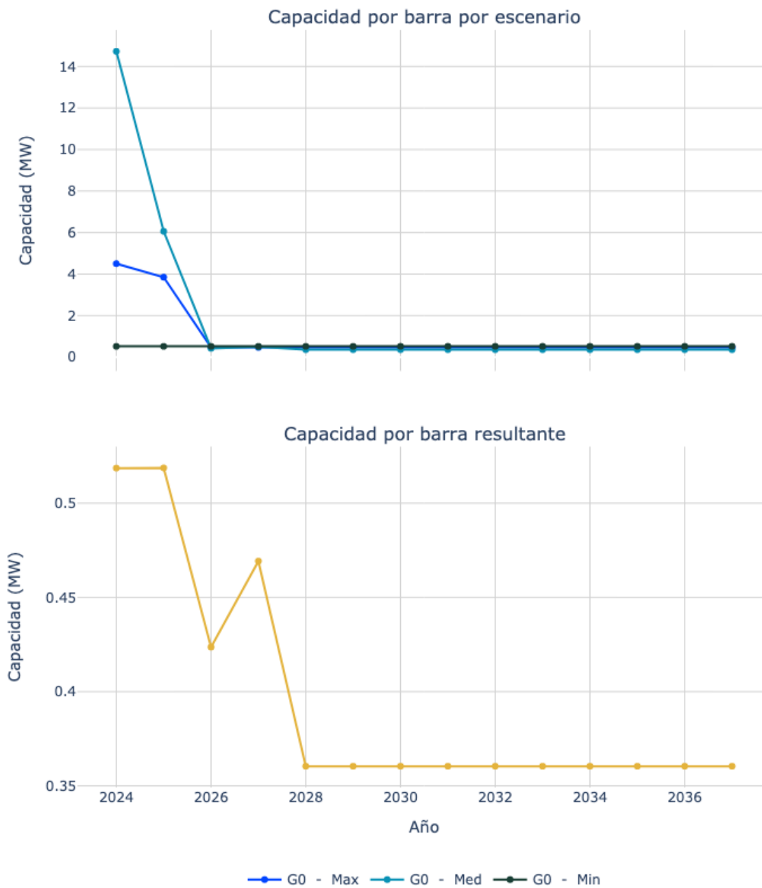
Figura 129. Capacidad de transporte de la subestación San Roque 34.5.
