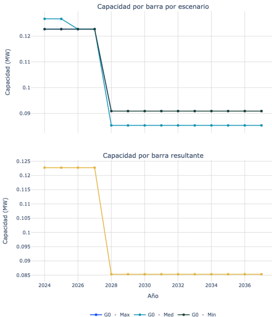
Figura 54. Capacidad de transporte de la subestación EL PASO 1 13.8 kV.
