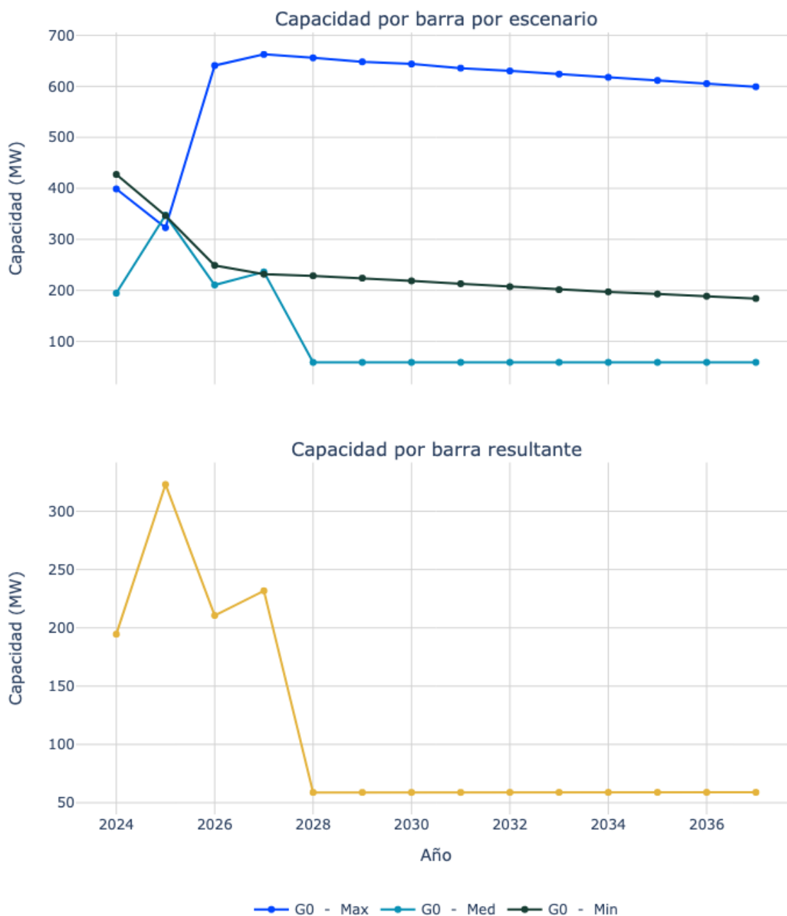
Figura 74. Capacidad de transporte de la subestación Guajira 220.
