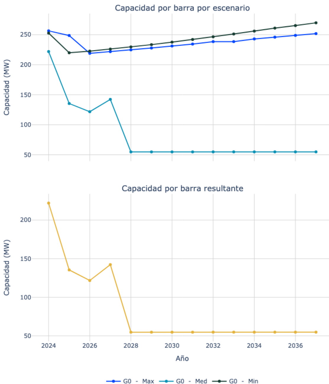
Figura 123. Capacidad de transporte de la subestación Riohacha 110.
