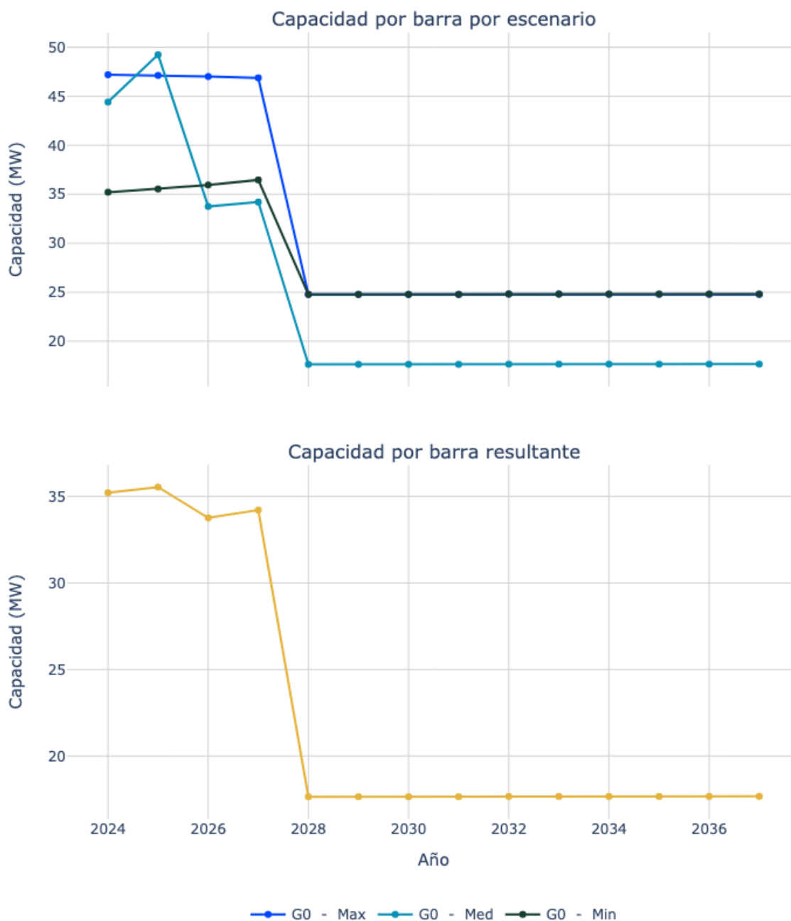
Figura 63. Capacidad de transporte de la subestación FUNDACION 2 13.8 kV.
