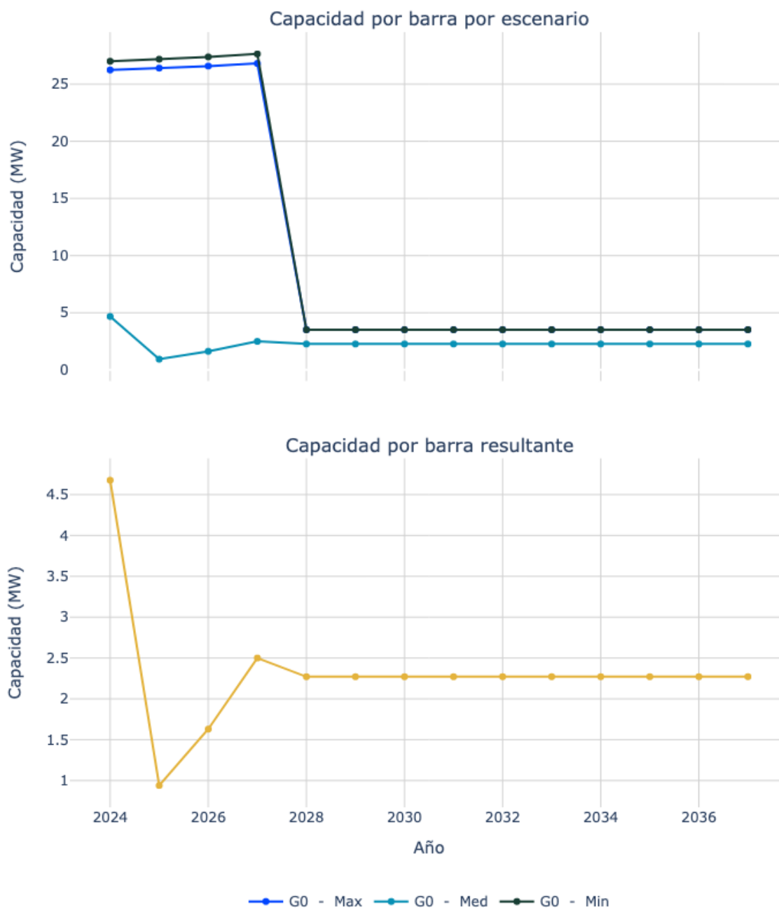
Figura 140. Capacidad de transporte de la subestación Tres esquinas 34.5.
