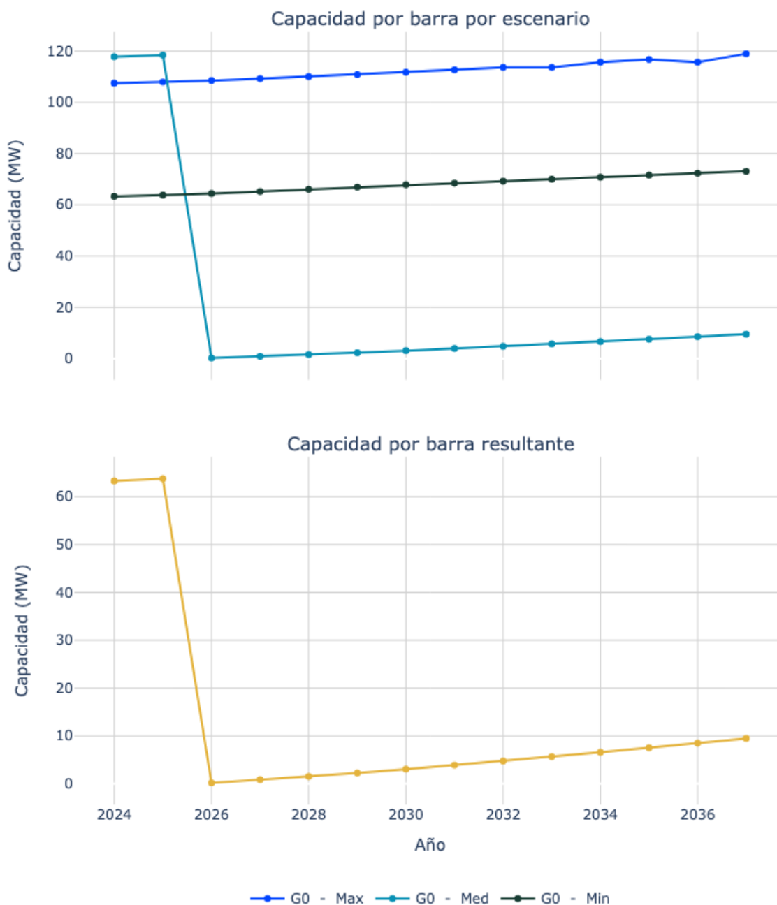
Figura 40. Capacidad de transporte de la subestación Codazzi GCM 110.
