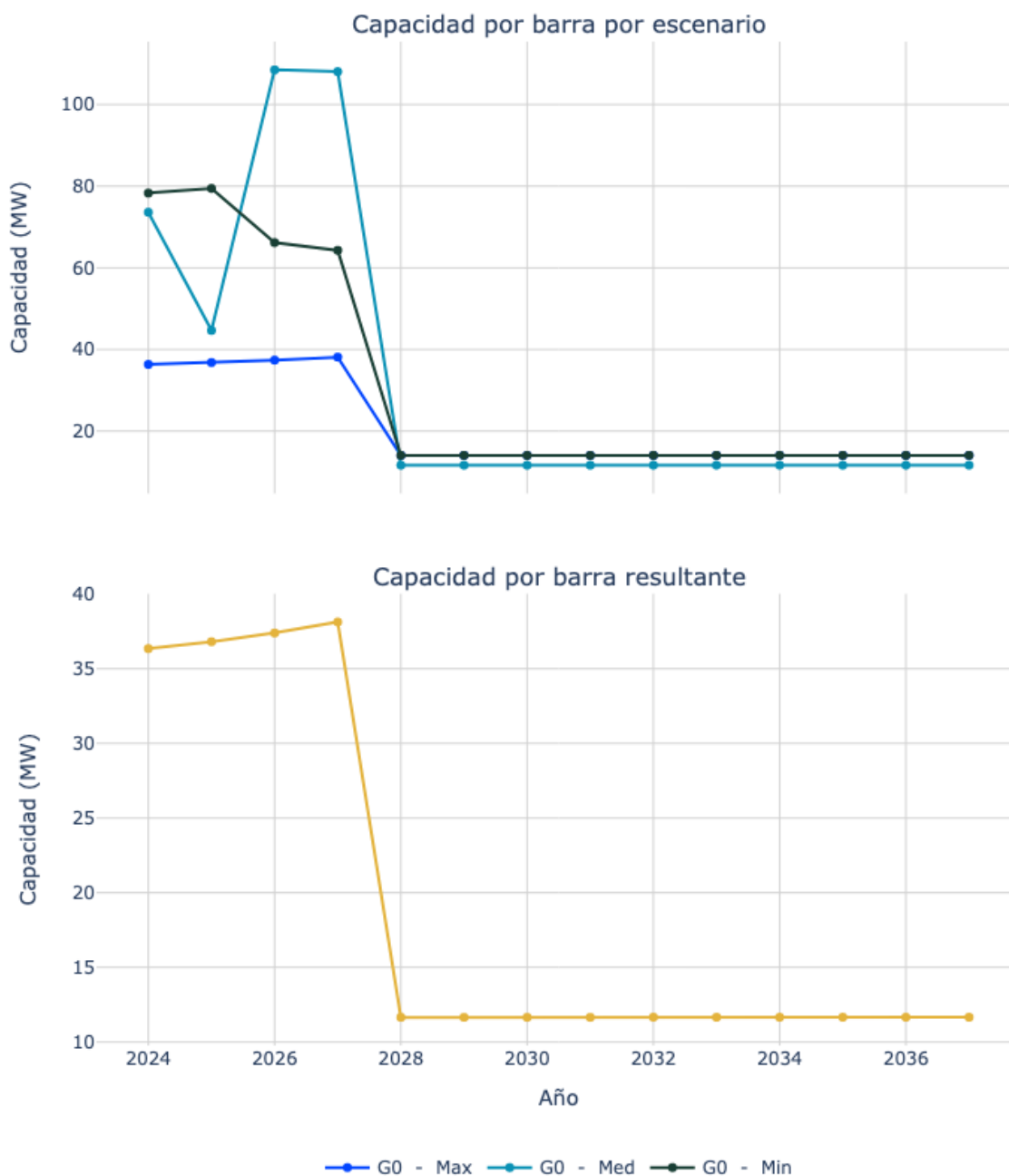
Figura 125. Capacidad de transporte de la subestación SAN JUAN 1 34.5 kV.
