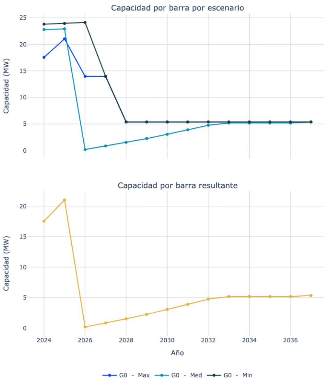
Figura 84. Capacidad de transporte de la subestación La Europa 34.5.
