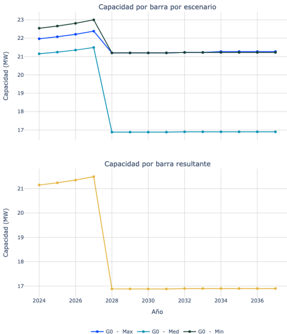
Figura 139. Capacidad de transporte de la subestación Termoguajira 34.5.
