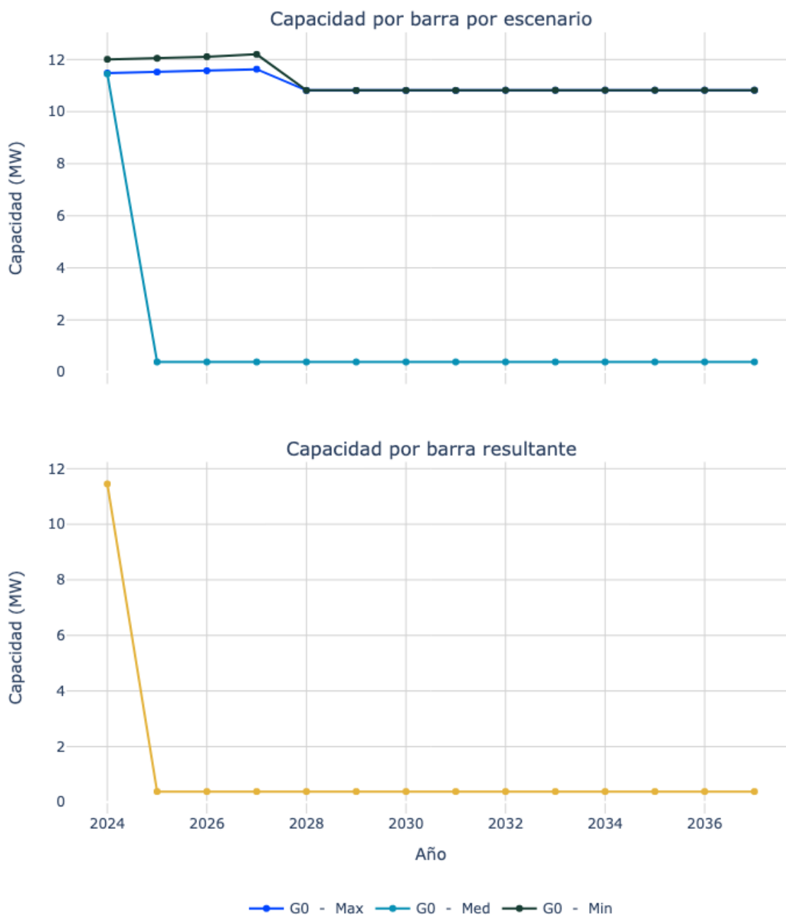
Figura 13. Capacidad de transporte de la subestación Aguas Blancas 34.5.
