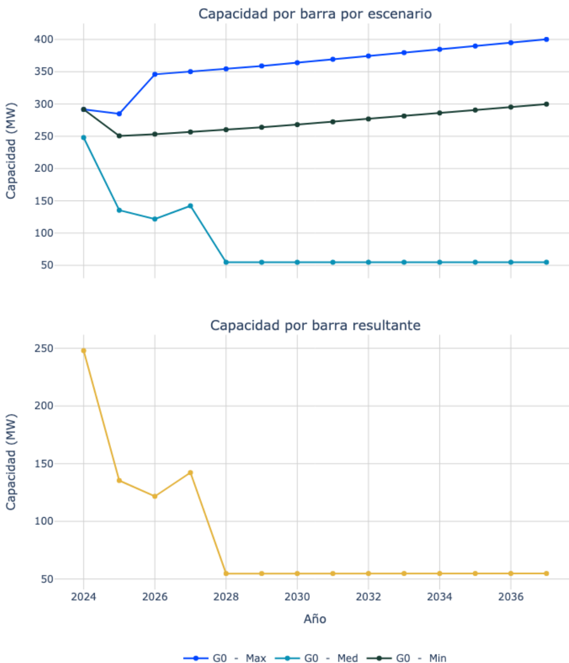
Figura 48. Capacidad de transporte de la subestación Cuestecitas 110.
