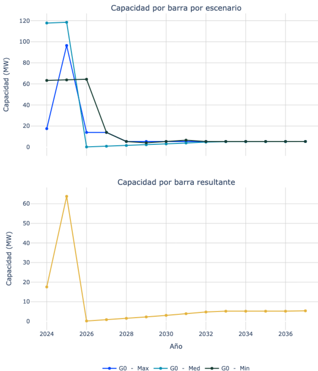
Figura 32. Capacidad de transporte de la subestación CODAZZI (CESAR) 1 34.5 kV.
