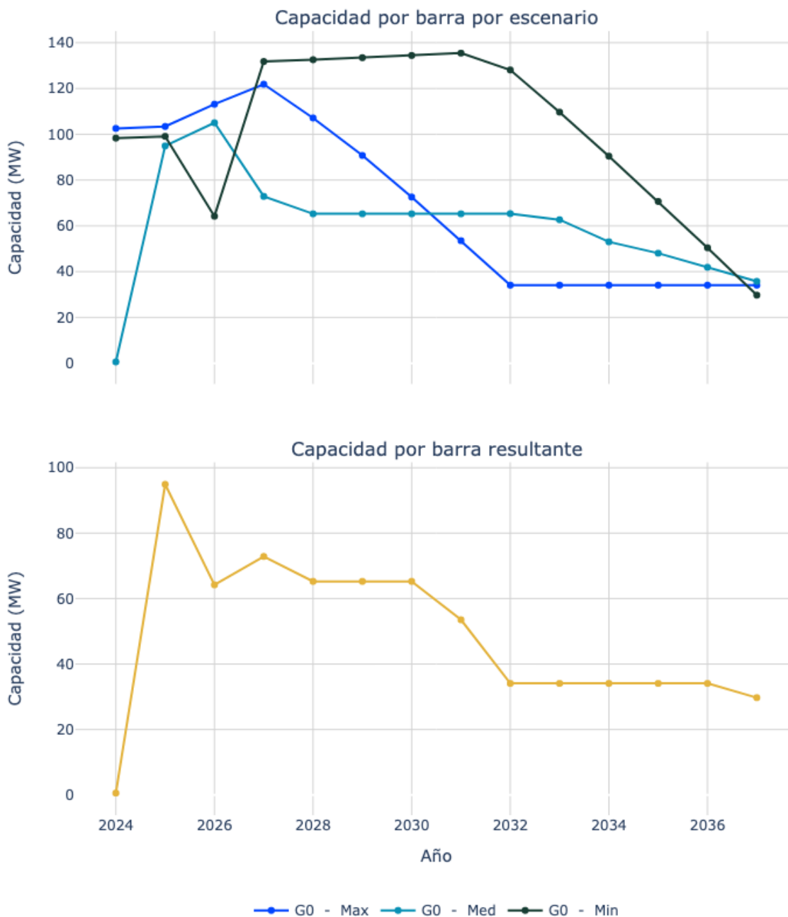
Figura 39. Capacidad de transporte de la subestación Cienaga 110.
