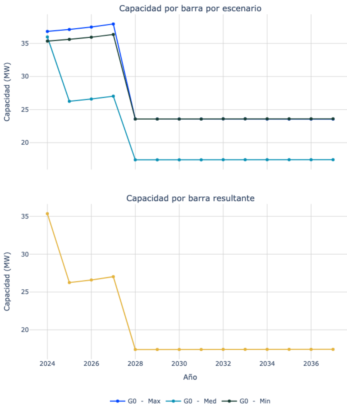
Figura 26. Capacidad de transporte de la subestación Bonda 34.5.
