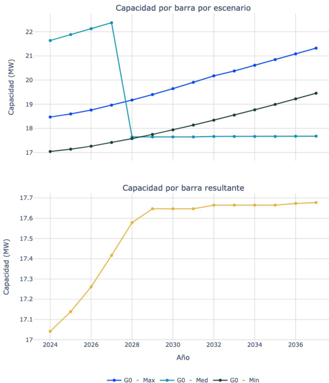
Figura 72. Capacidad de transporte de la subestación Guacamayal 13.8.
