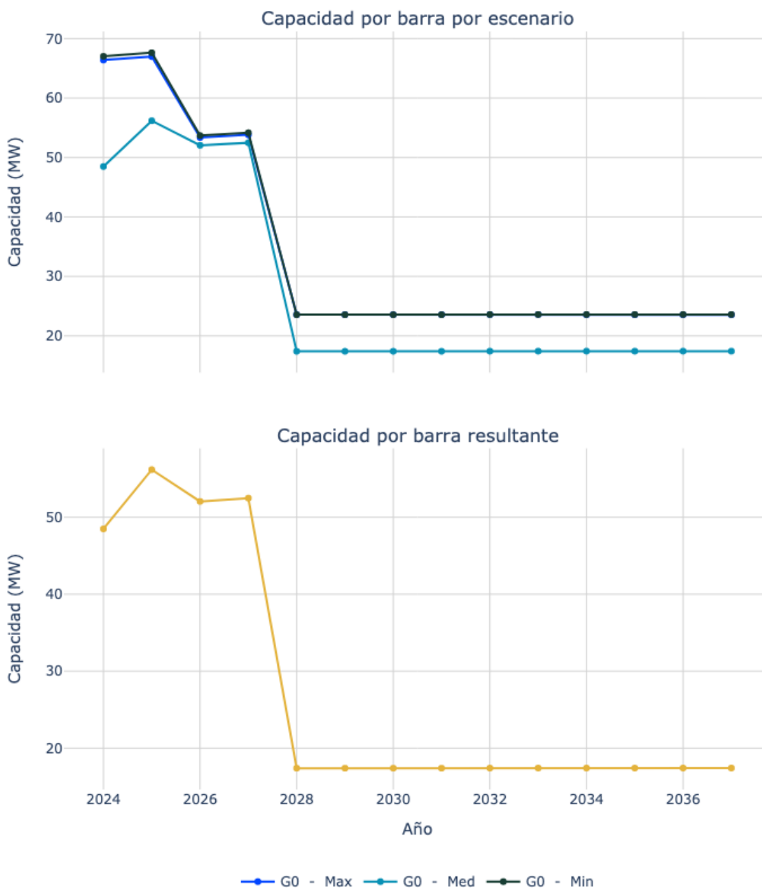
Figura 83. Capacidad de transporte de la subestación LIBERTADOR 1 13.8 kV.
