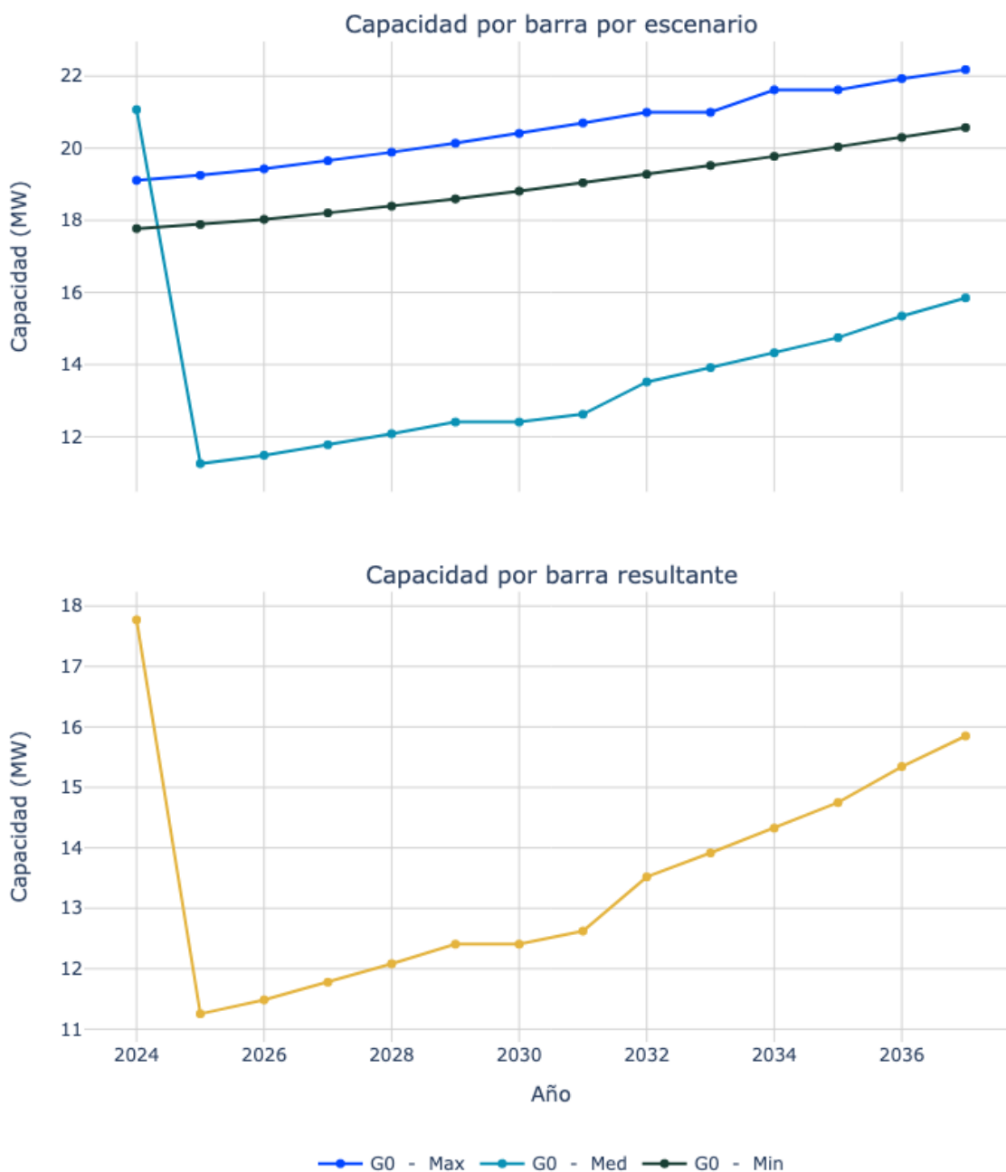
Figura 153. Capacidad de transporte de la subestación Zawady 13.8 T2.
