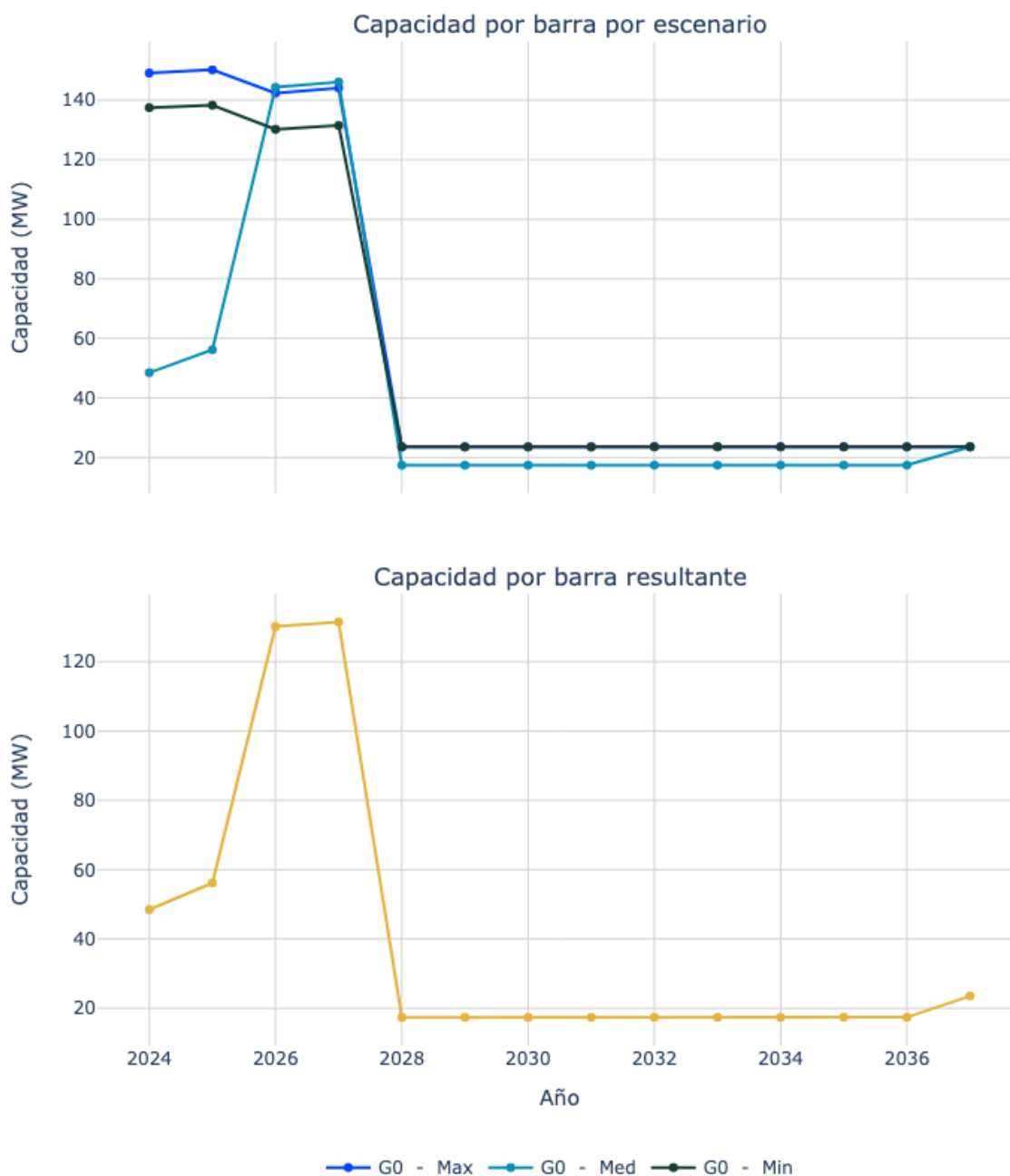
Figura 98. Capacidad de transporte de la subestación MANZANARES (MAGDALENA) 2 13.8 kV.
