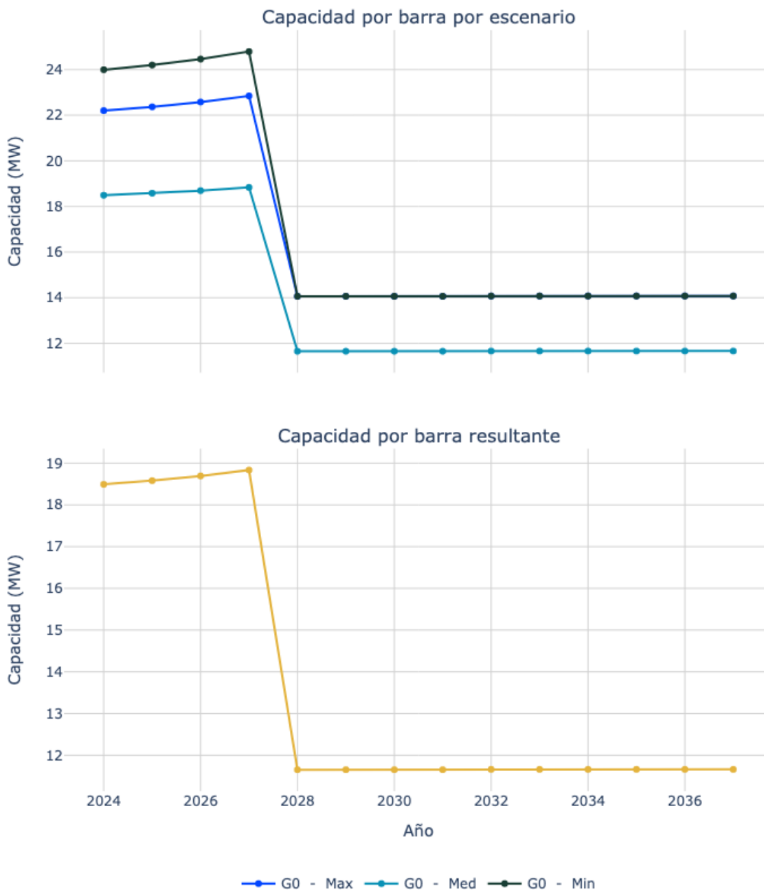
Figura 151. Capacidad de transporte de la subestación Villanueva 34.5.
