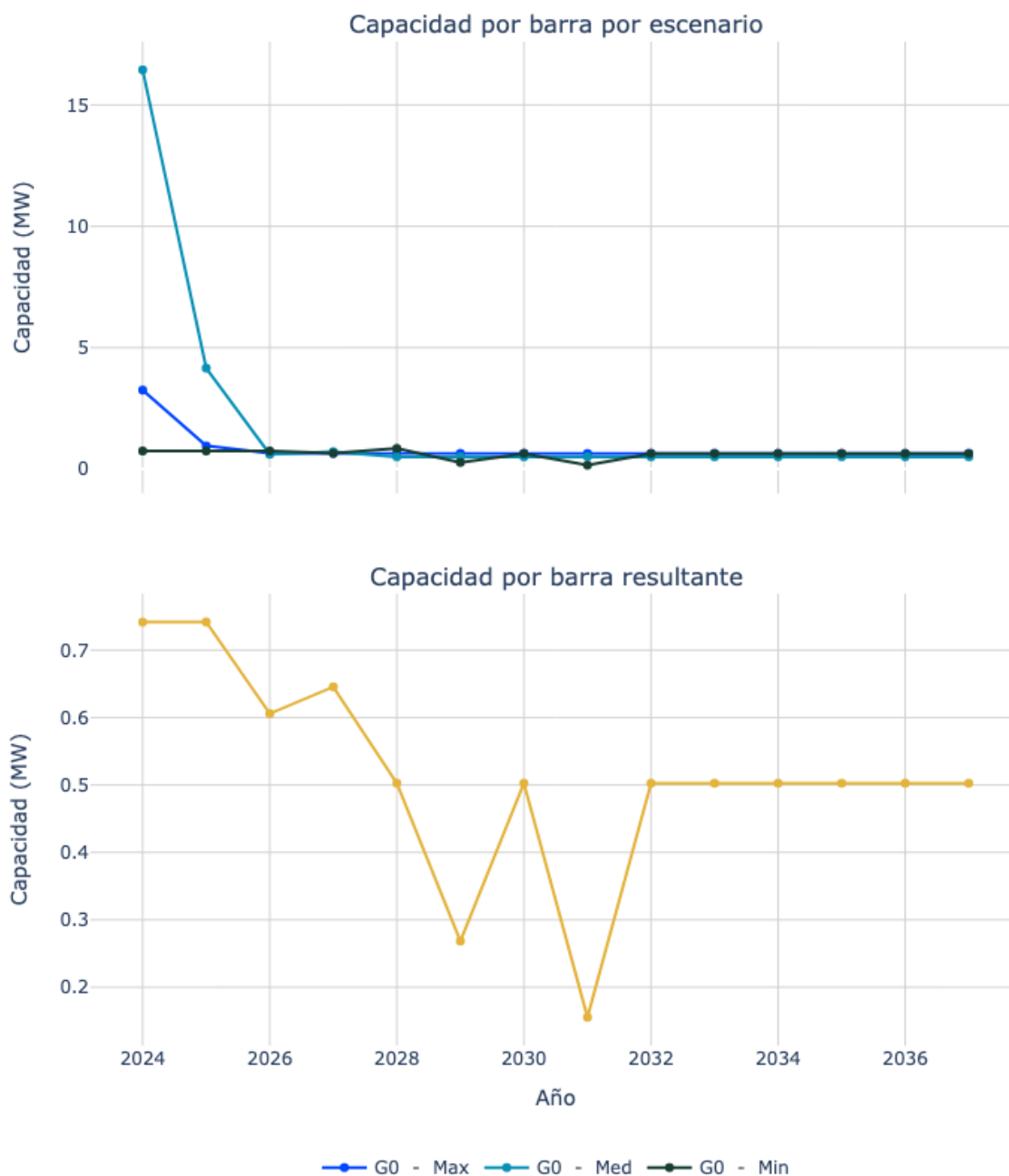
Figura 88. Capacidad de transporte de la subestación La aurora 34.5.
