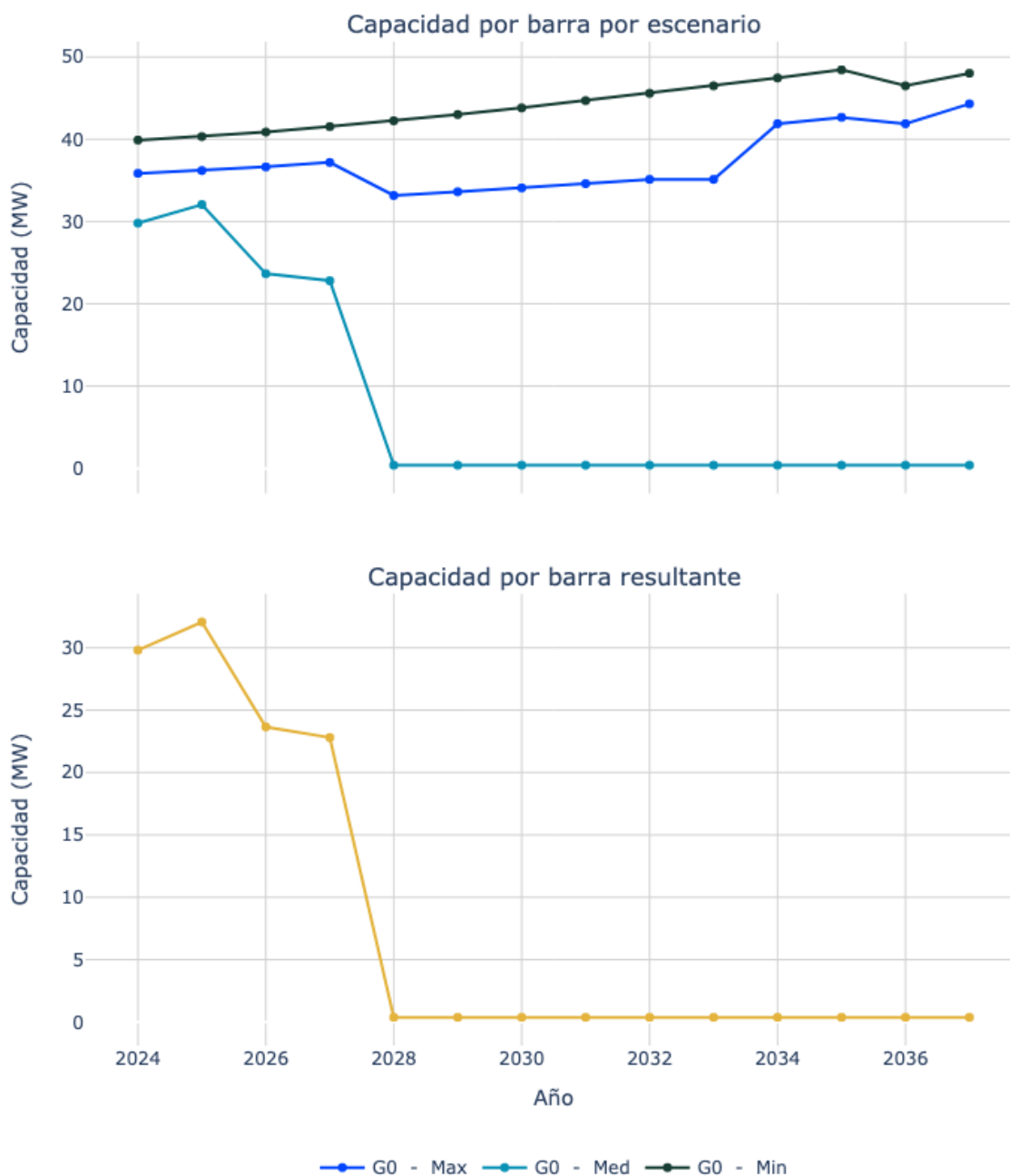
Figura 59. Capacidad de transporte de la subestación El burro 34.5.
