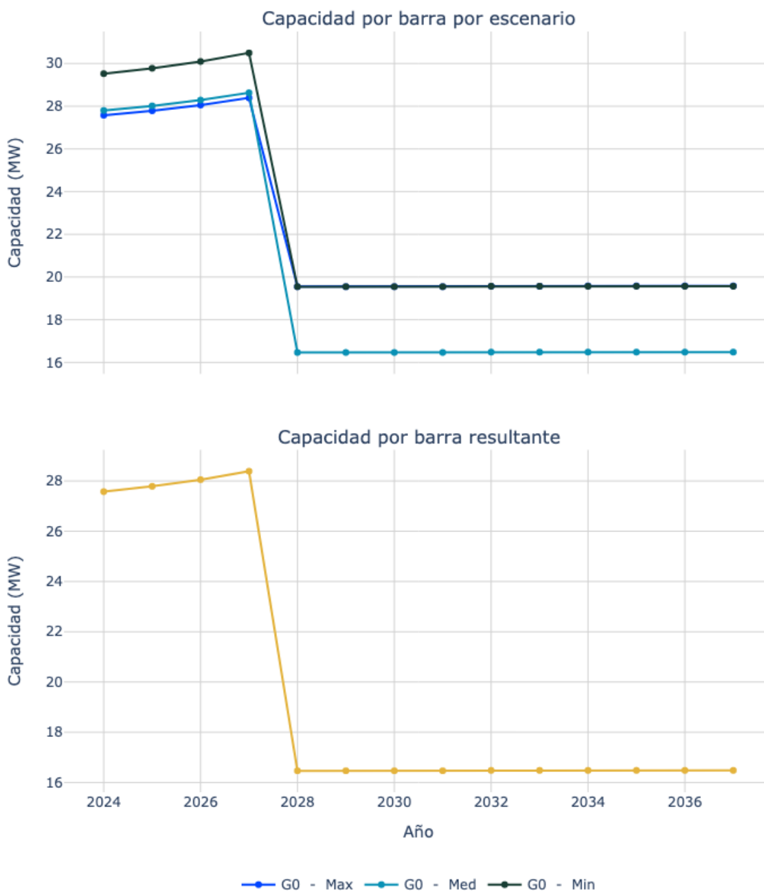
Figura 78. Capacidad de transporte de la subestación Hato Nuevo 34.5.
