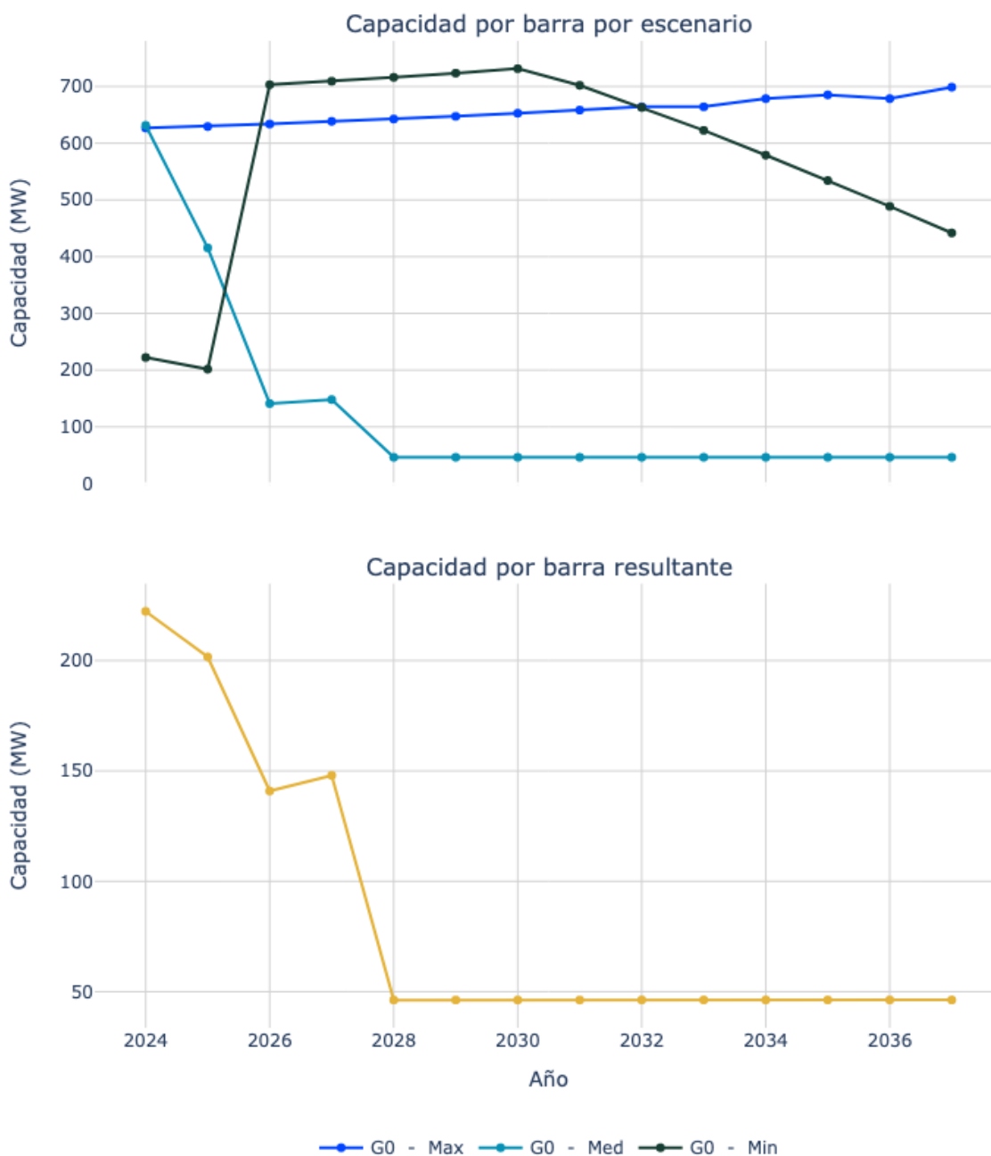
Figura 147. Capacidad de transporte de la subestación Valledupar 220.
