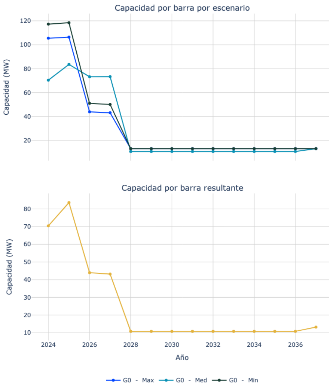
Figura 76. Capacidad de transporte de la subestación Guatapuri 34.5.
