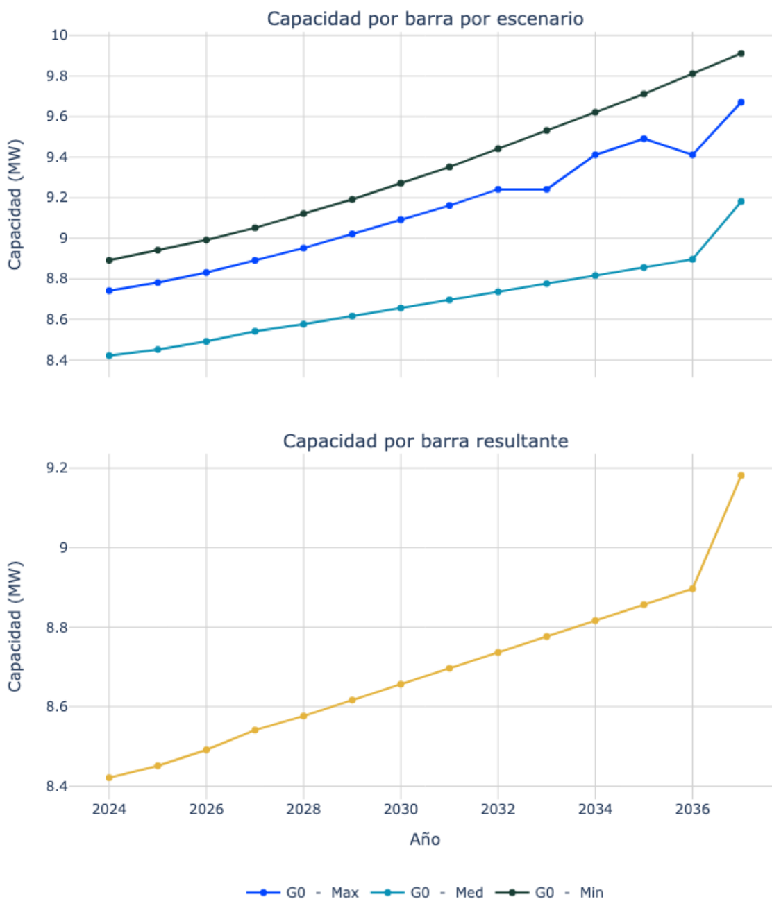
Figura 122. Capacidad de transporte de la subestación Rio viejo 34.5.
