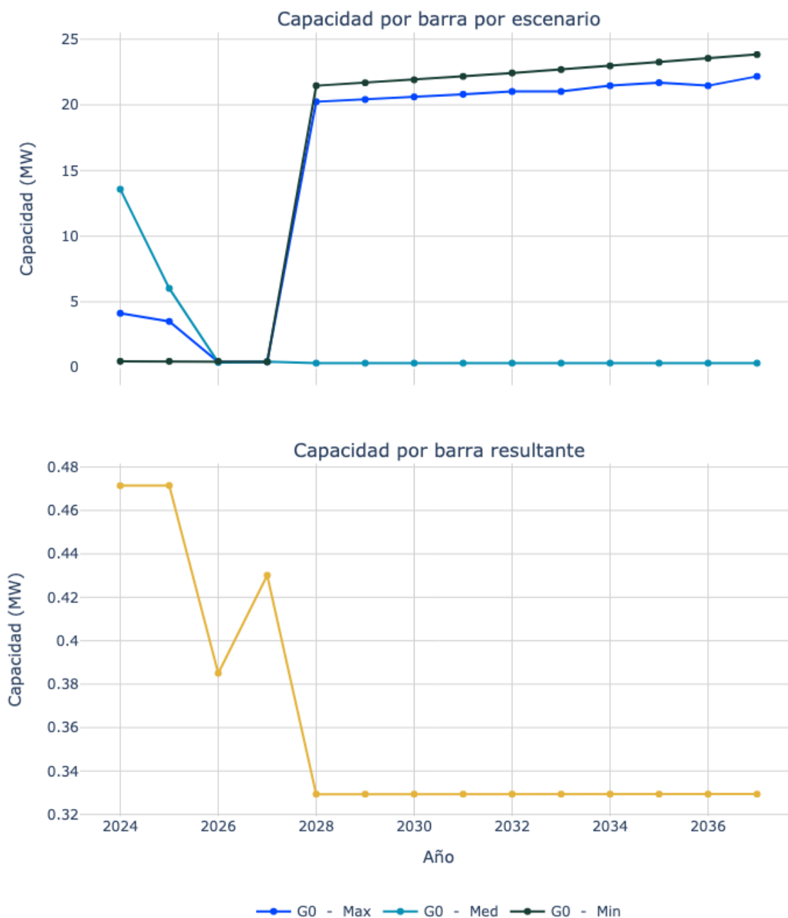
Figura 50. Capacidad de transporte de la subestación Curumani 13.8.
