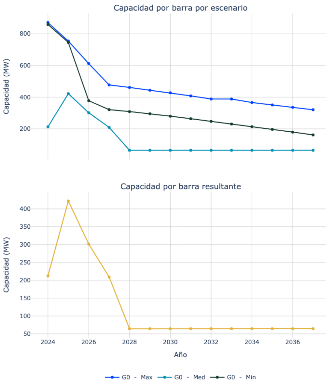
Figura 132. Capacidad de transporte de la subestación Santa Marta 220.
