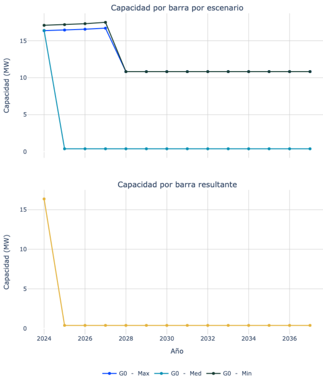
Figura 143. Capacidad de transporte de la subestación Valencia 34.5.
