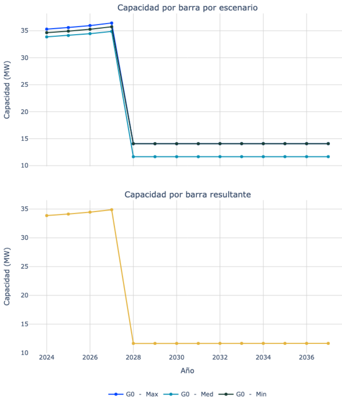
Figura 65. Capacidad de transporte de la subestación Fonseca 34.5.
