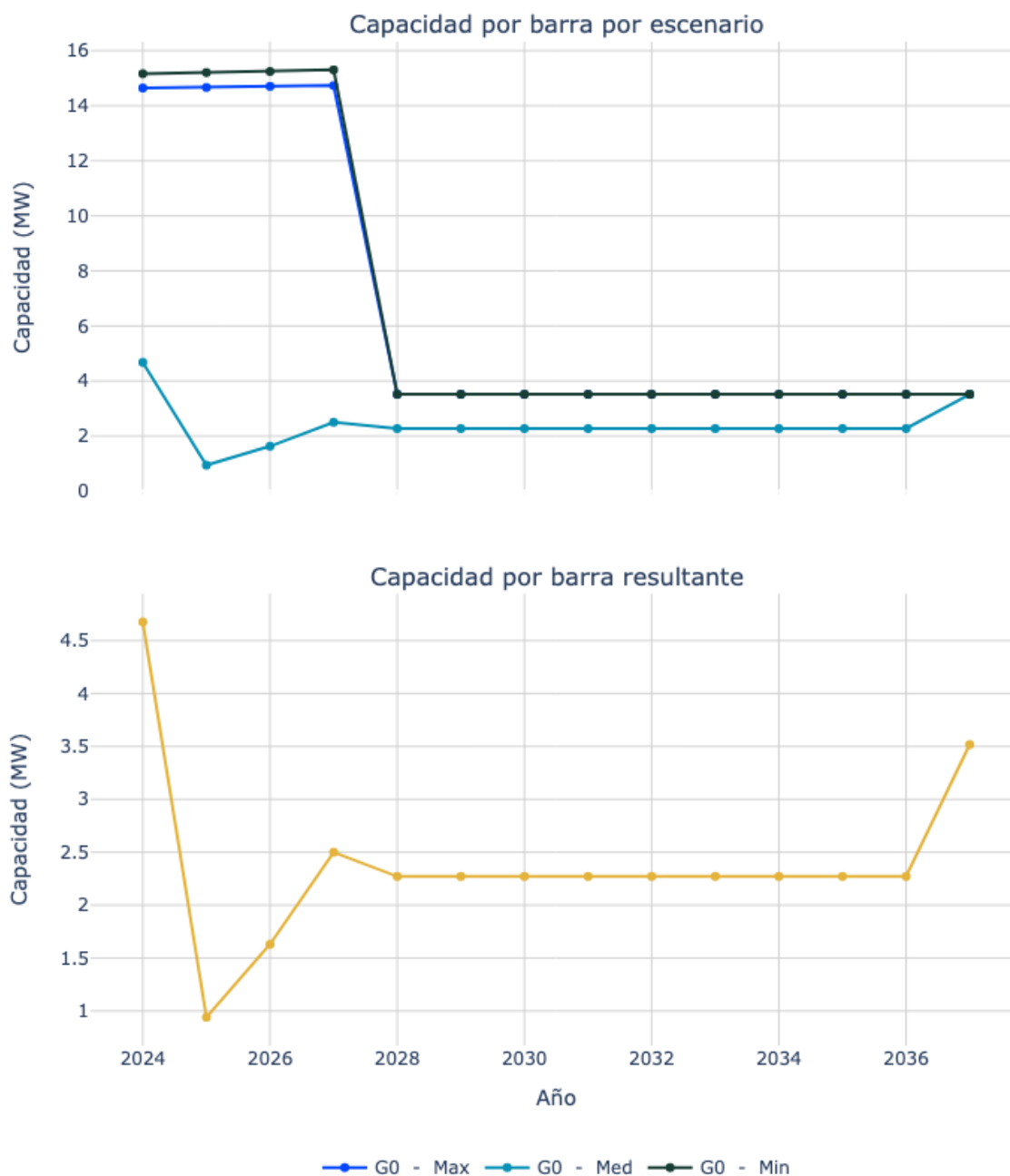
Figura 14. Capacidad de transporte de la subestación Algarrobo 34.5.
