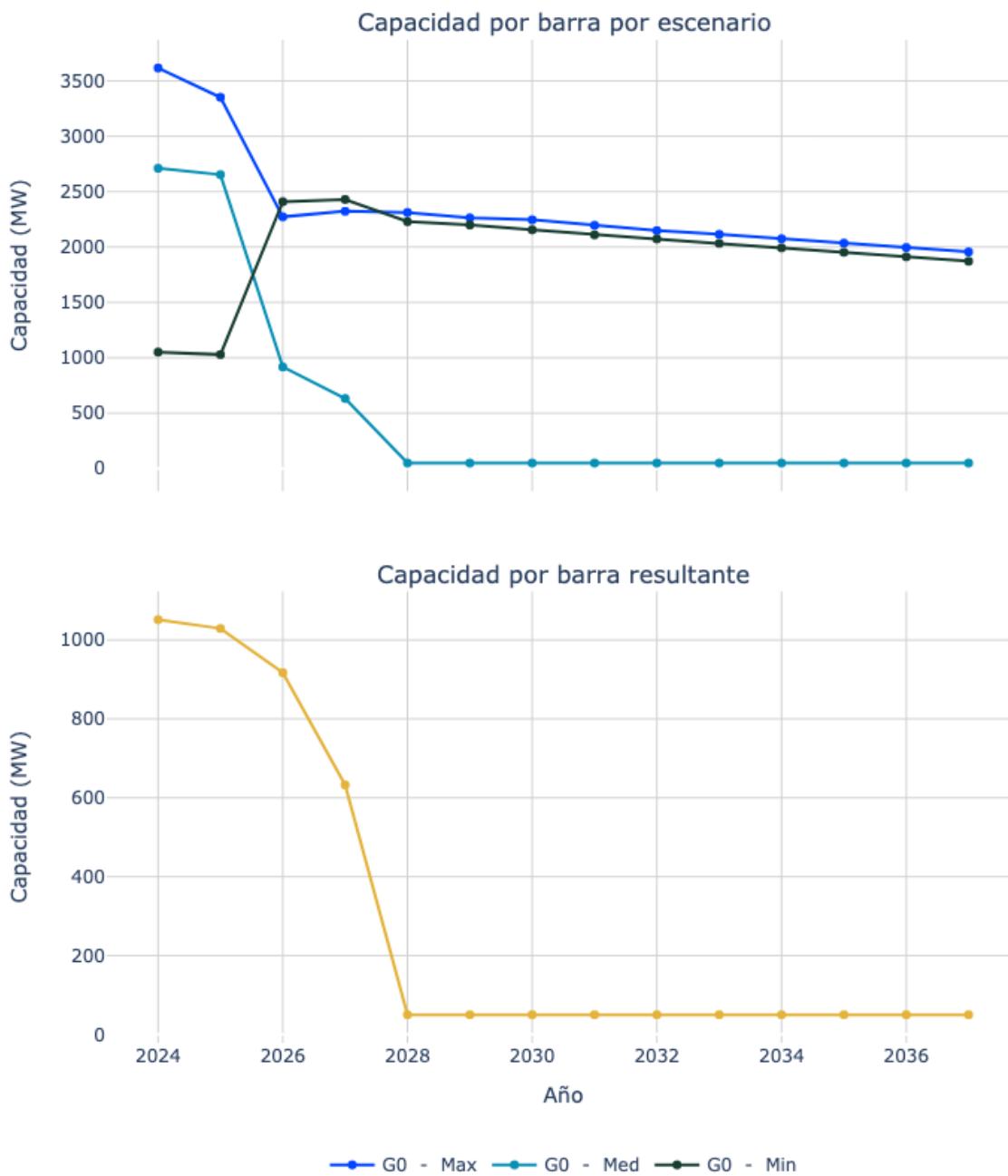
Figura 43. Capacidad de transporte de la subestación Copey 220.
