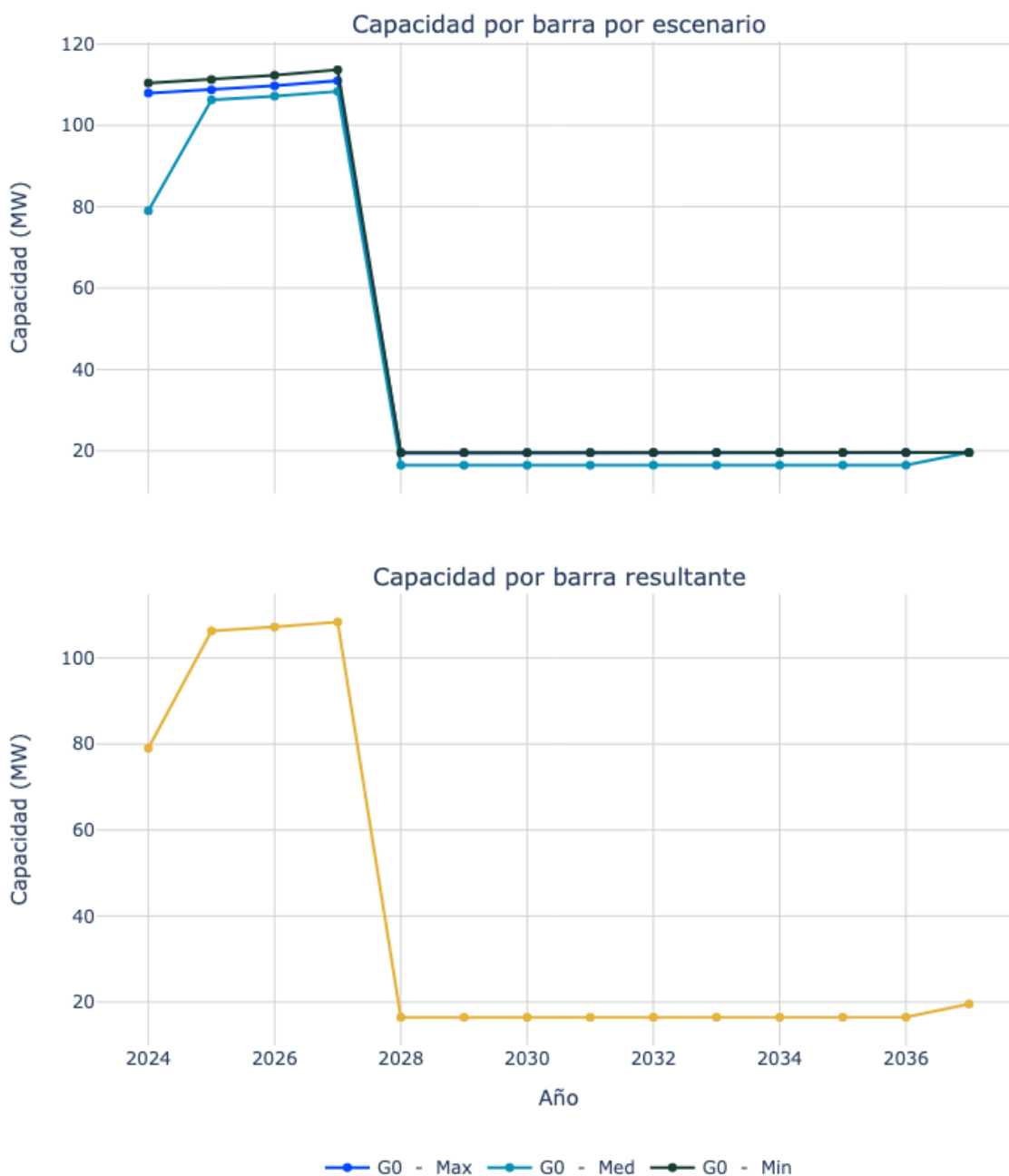
Figura 96. Capacidad de transporte de la subestación MAICAO 2 13.8 kV.
