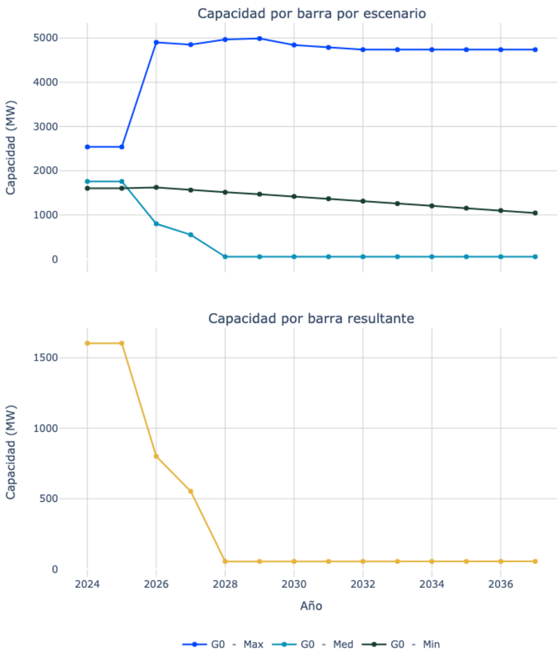
Figura 49. Capacidad de transporte de la subestación Cuestecitas 500.
