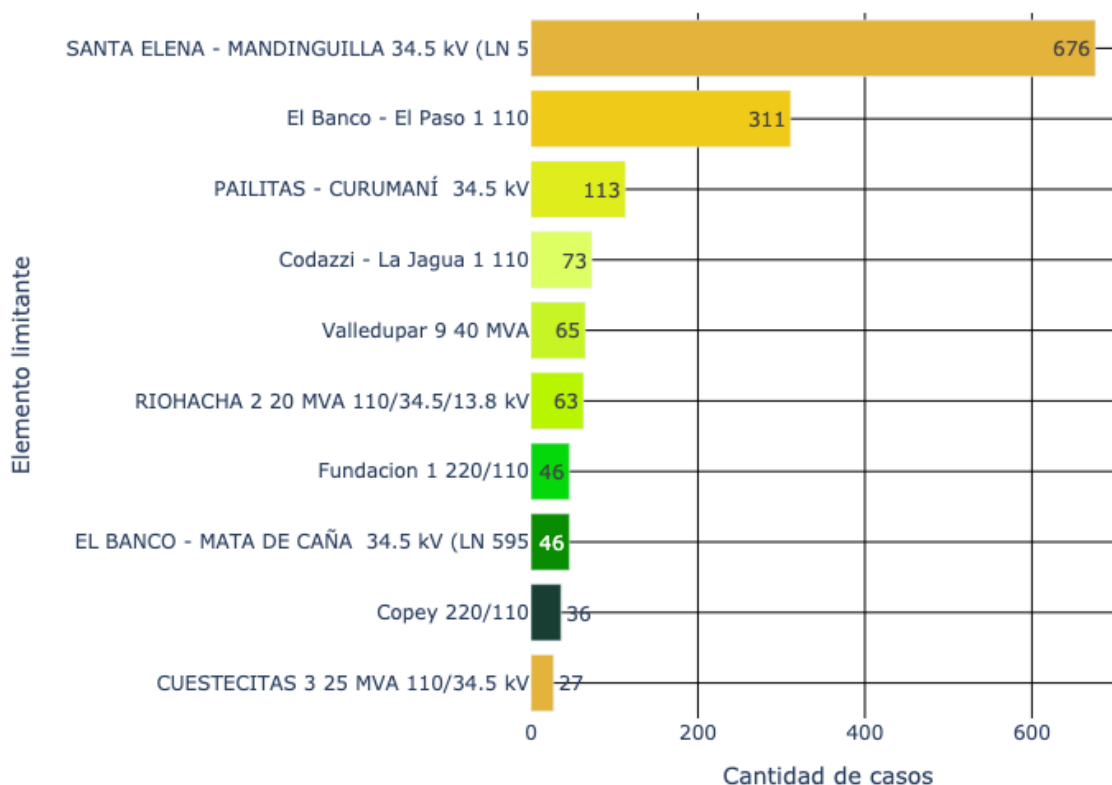
Figura 11. Elementos críticos identificados en la subárea GCM
