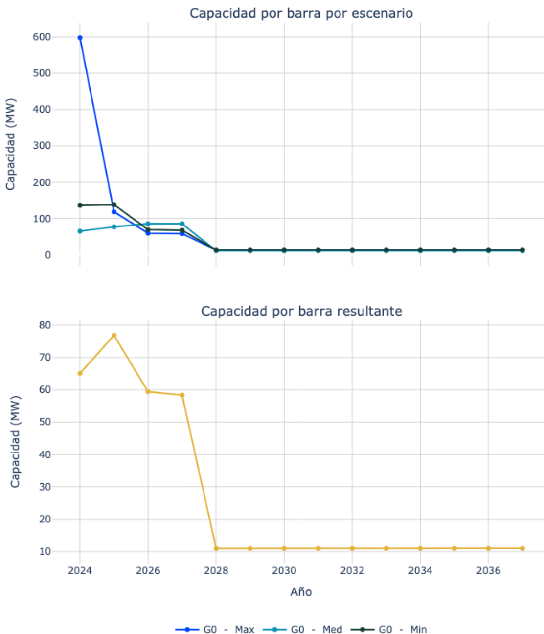
Figura 148. Capacidad de transporte de la subestación Valledupar34.5_B1.
