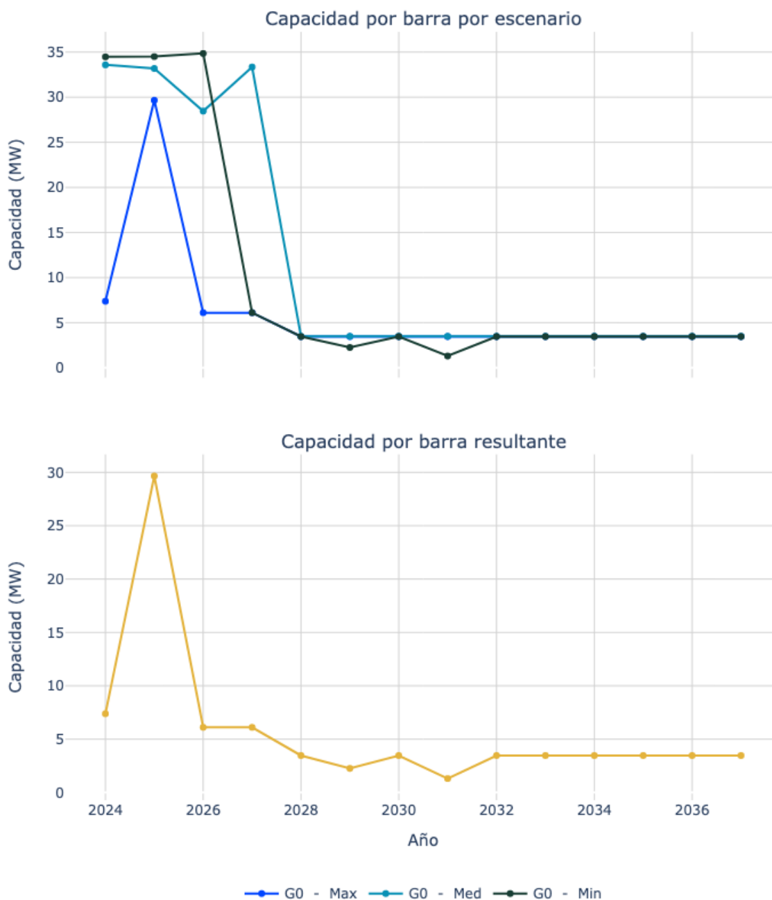
Figura 79. Capacidad de transporte de la subestación LA JAGUA 1 13.8 kV.
