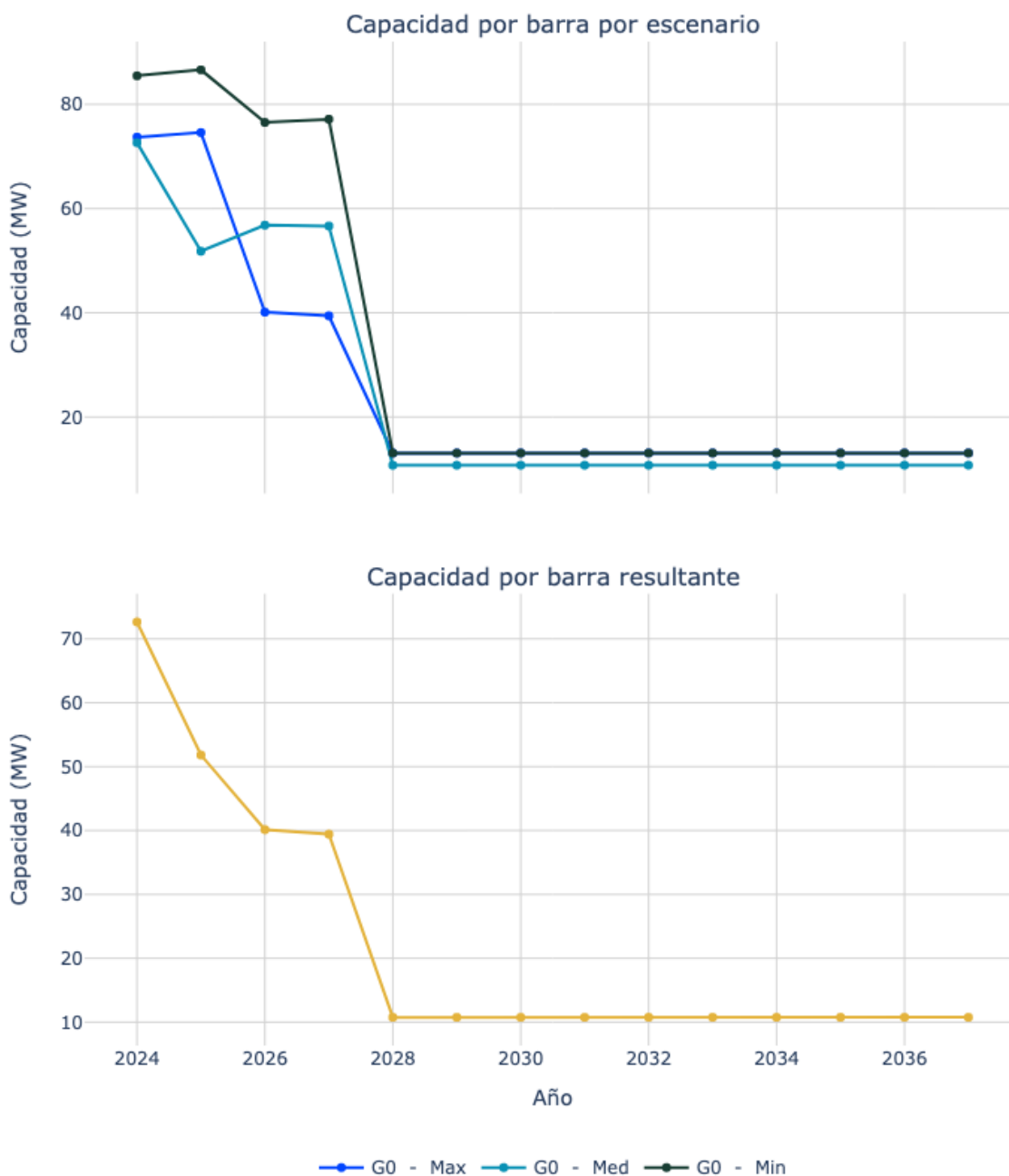
Figura 107. Capacidad de transporte de la subestación Nueva Guatapuri 34.5.
