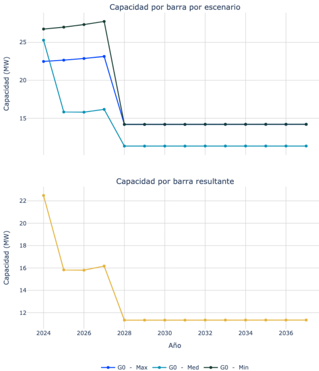
Figura 89. Capacidad de transporte de la subestación La paz 34.5.
