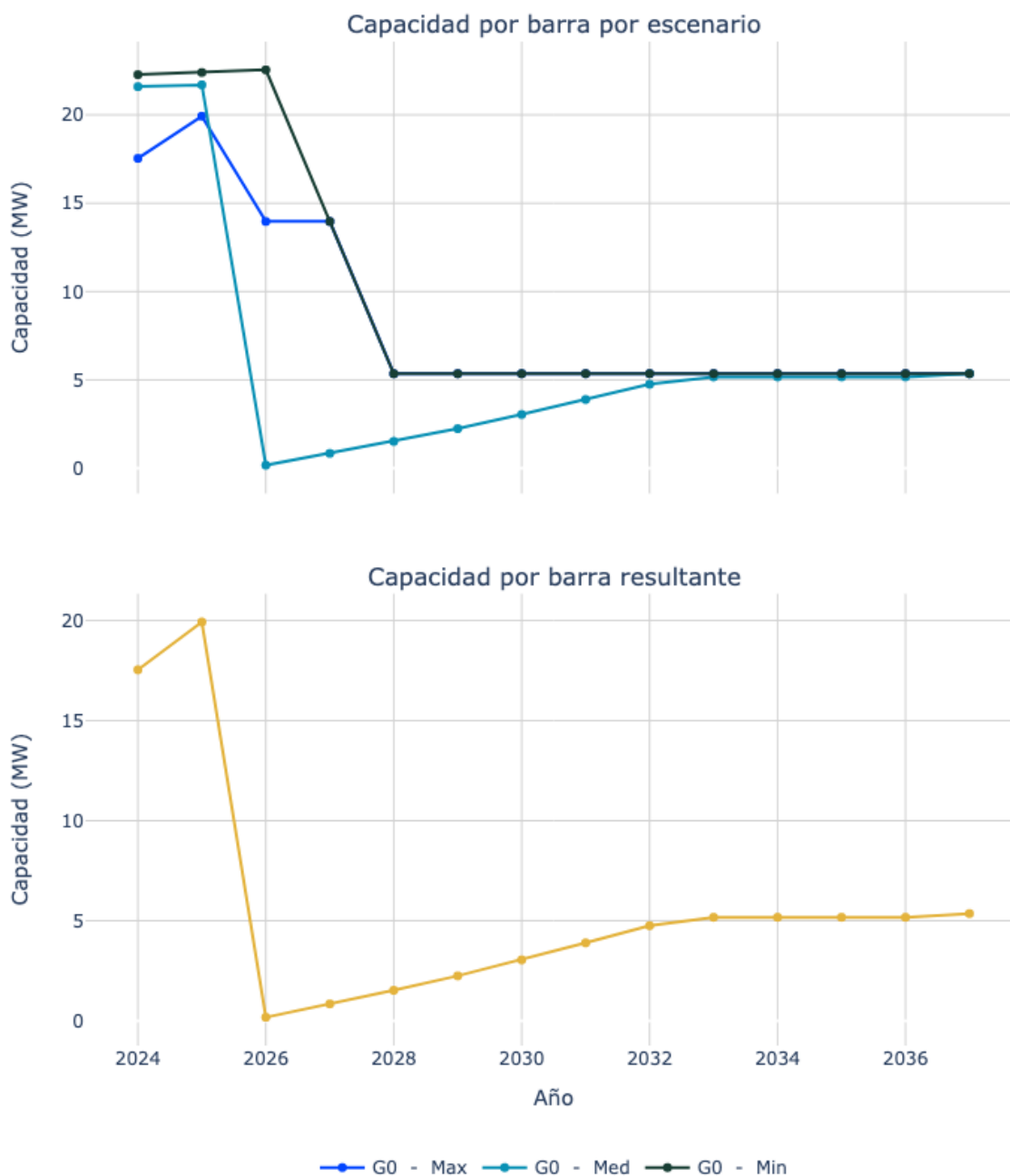
Figura 24. Capacidad de transporte de la subestación Becerril 34.5.
