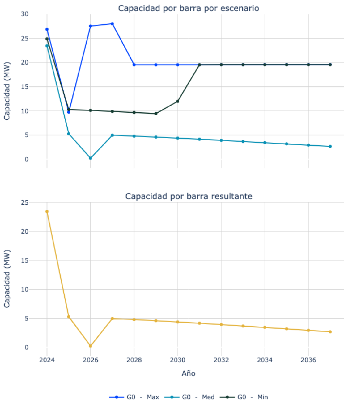
Figura 119. Capacidad de transporte de la subestación RIOHACHA 3 34.5 kV.
