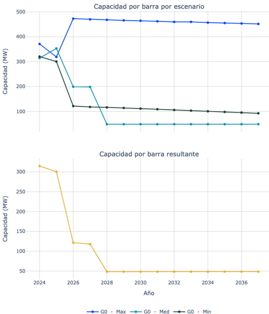
Figura 128. Capacidad de transporte de la subestación San Juan 220.
