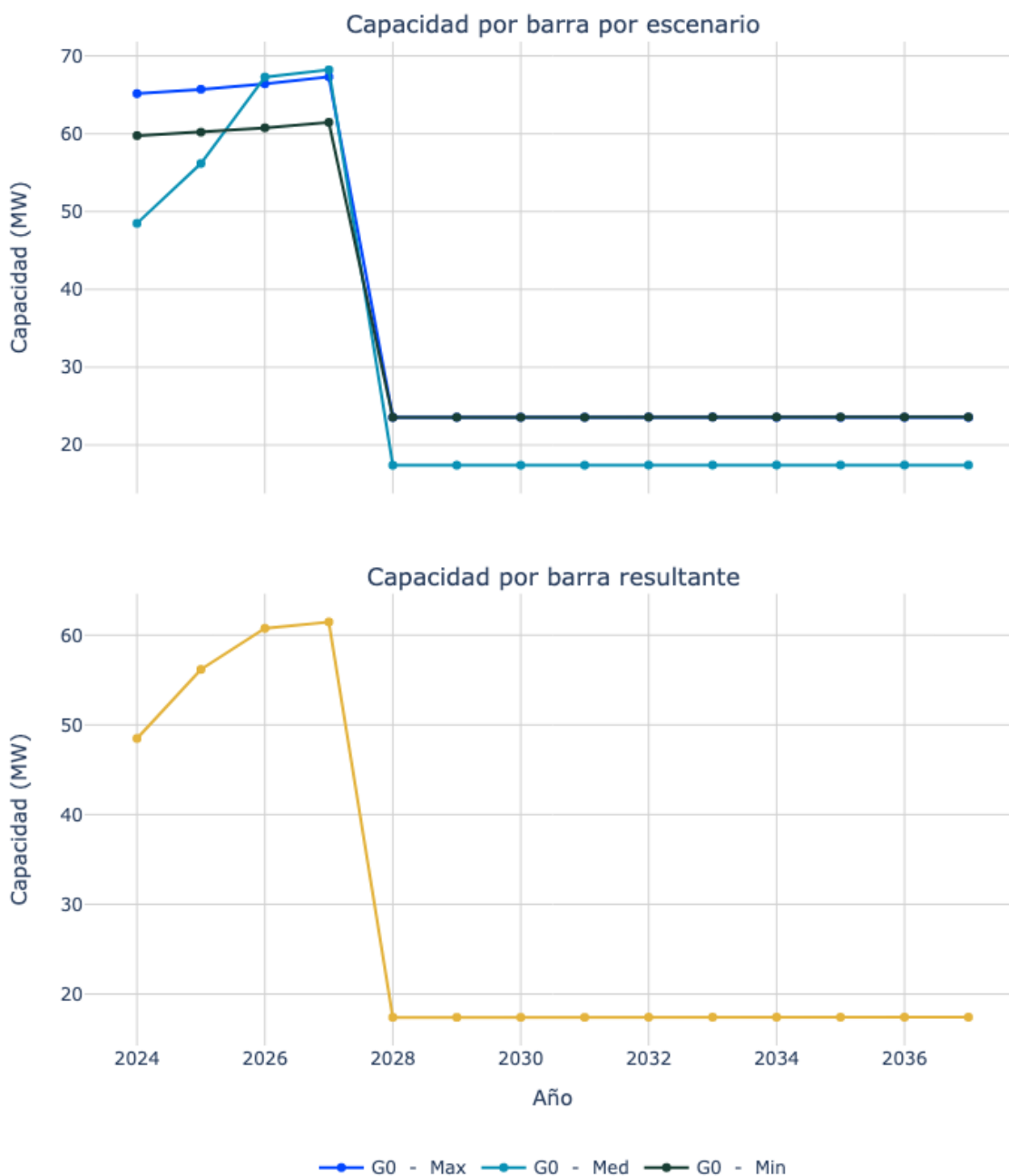
Figura 97. Capacidad de transporte de la subestación MANZANARES (MAGDALENA) 1 13.8 kV.
