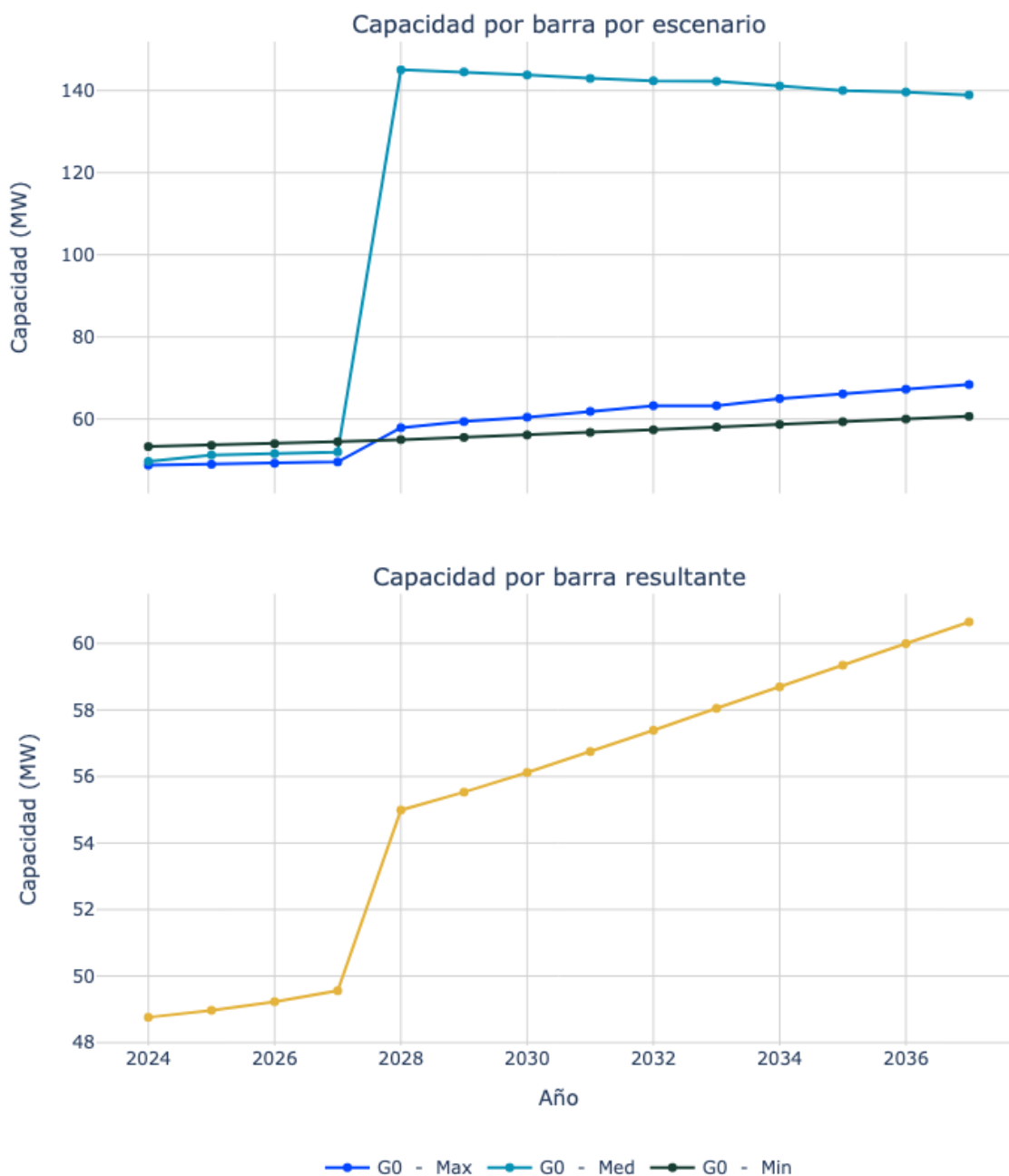
Figura 52. Capacidad de transporte de la subestación EL BANCO 1 13.8 kV.
