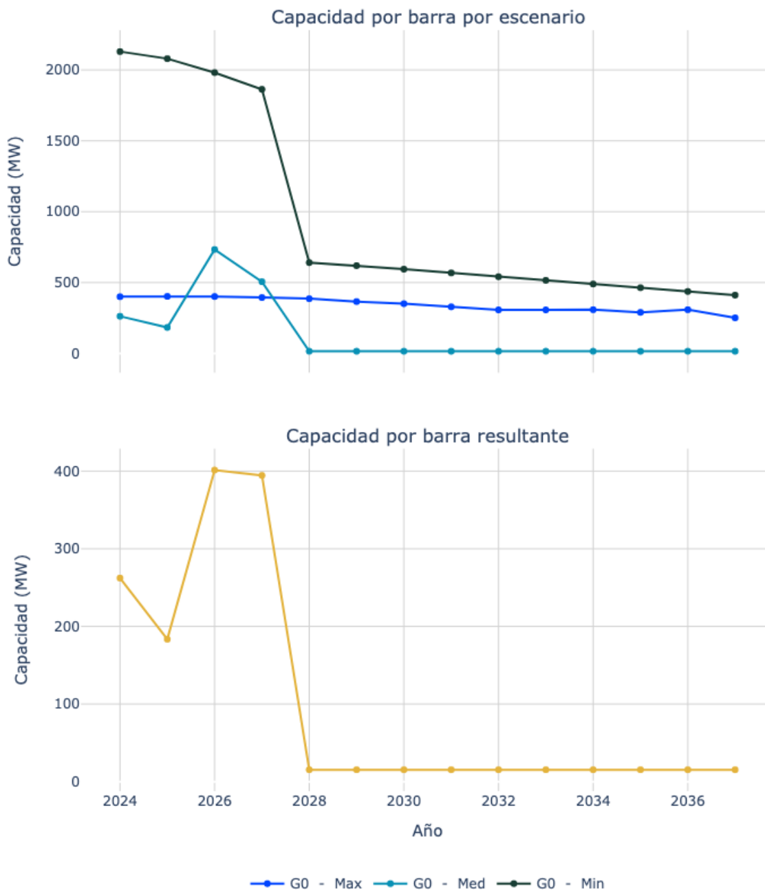
Figura 86. Capacidad de transporte de la subestación La Loma 110.
