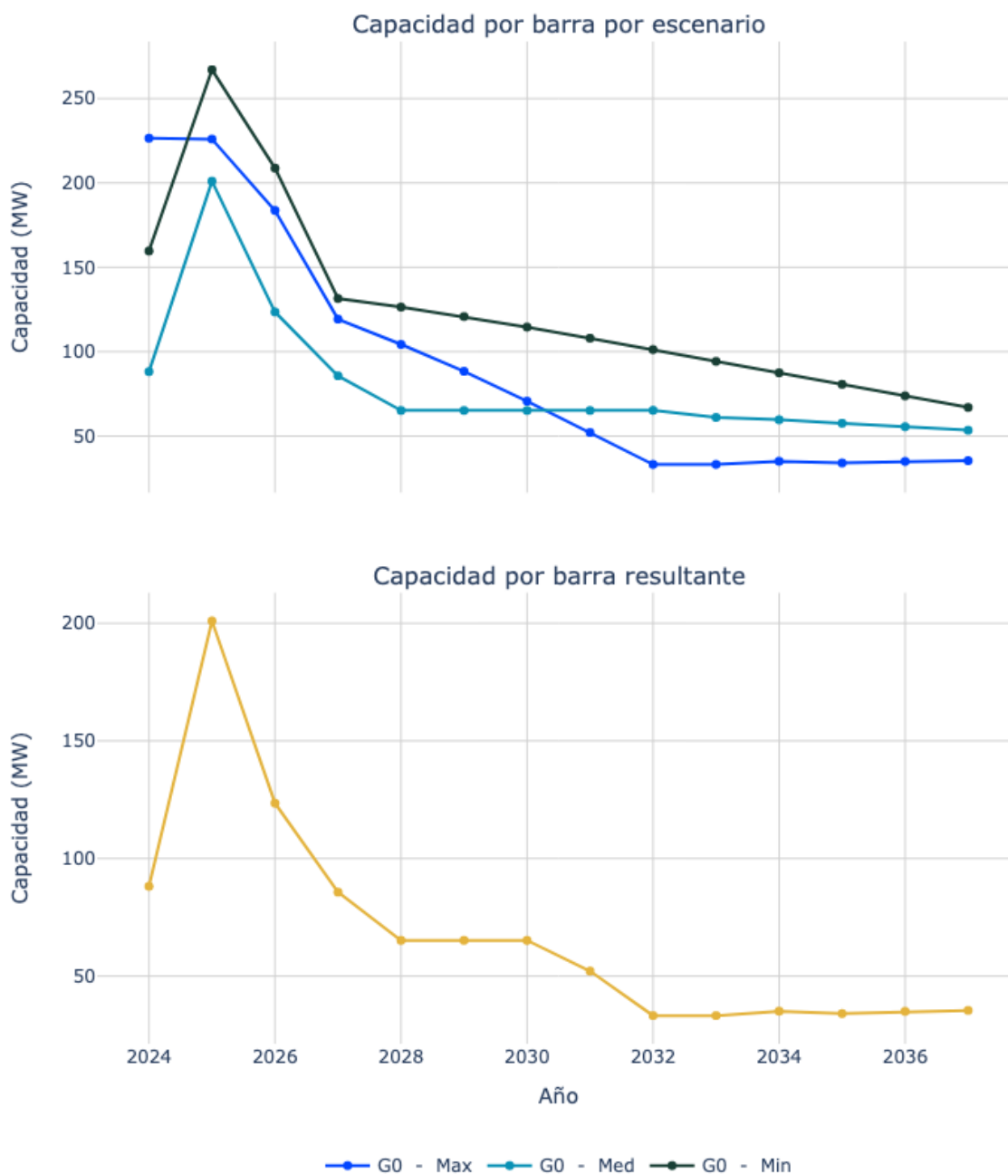
Figura 121. Capacidad de transporte de la subestación Rio Cordoba 110.
