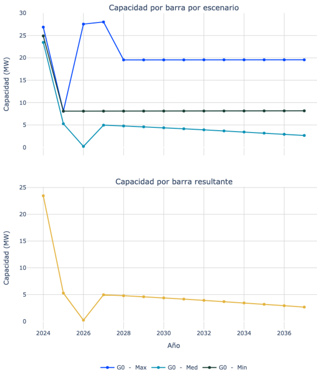
Figura 20. Capacidad de transporte de la subestación Ballenas 34.5.
