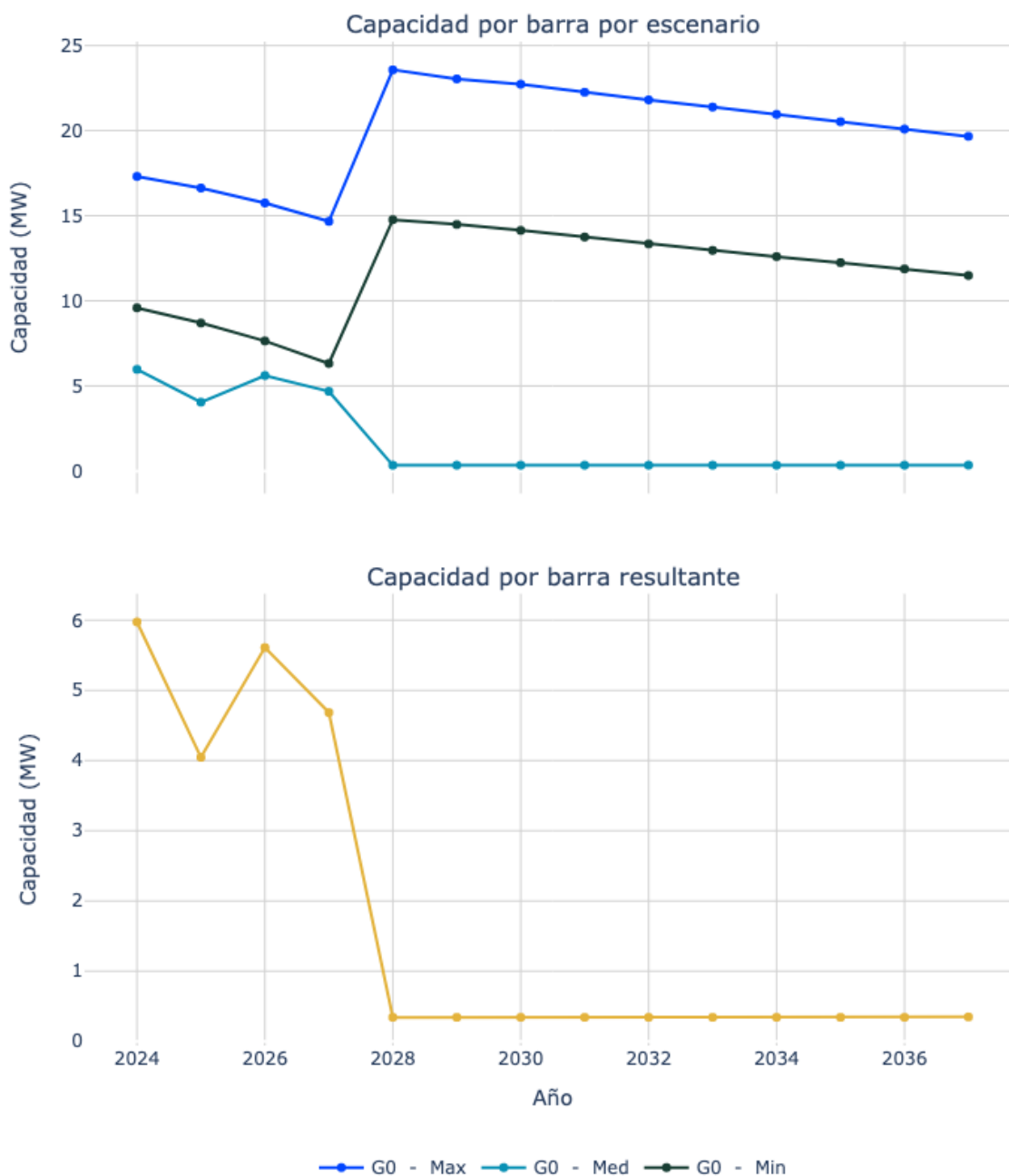
Figura 101. Capacidad de transporte de la subestación Mandinguilla 34.5.
