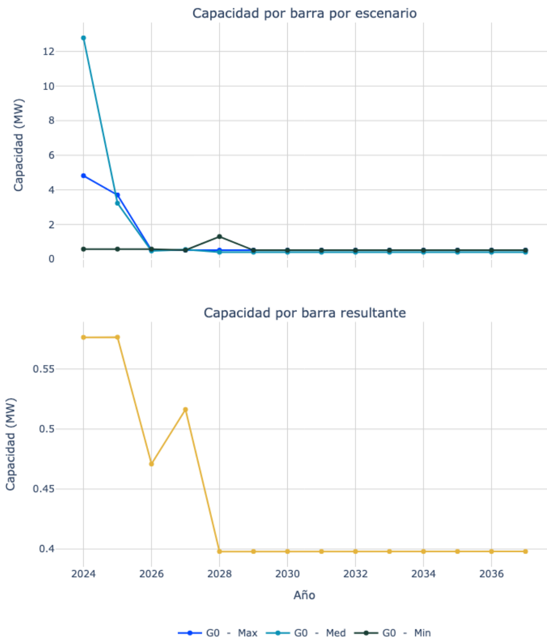
Figura 38. Capacidad de transporte de la subestación Chiriguana 34.5.
