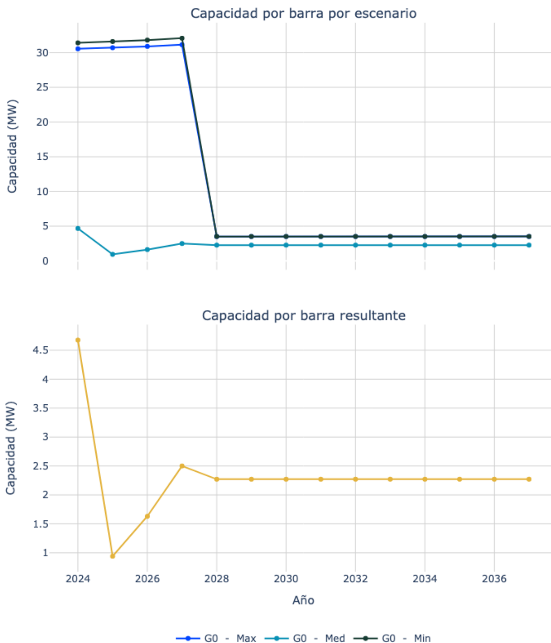
Figura 17. Capacidad de transporte de la subestación Ariguani 34.5.
