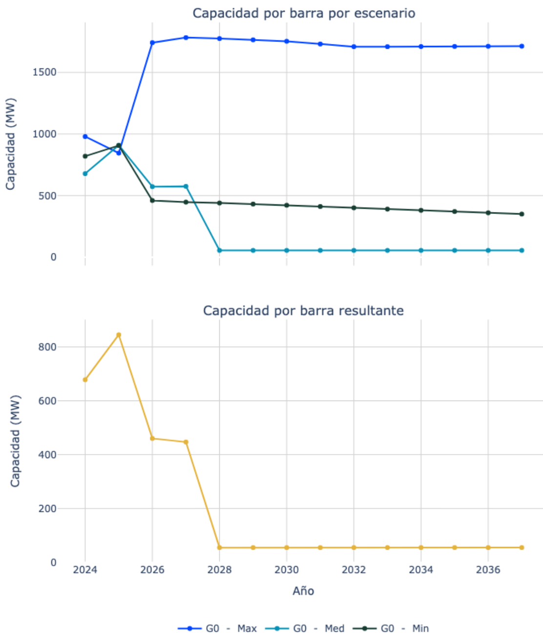
Figura 46. Capacidad de transporte de la subestación Cuestecita 220.
