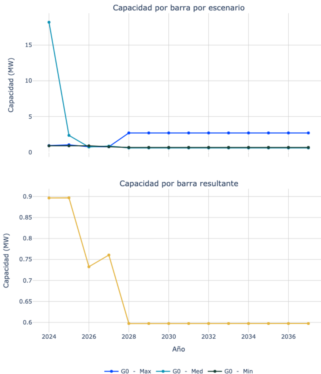
Figura 82. Capacidad de transporte de la subestación LA LOMA 3 34.5 kV.
