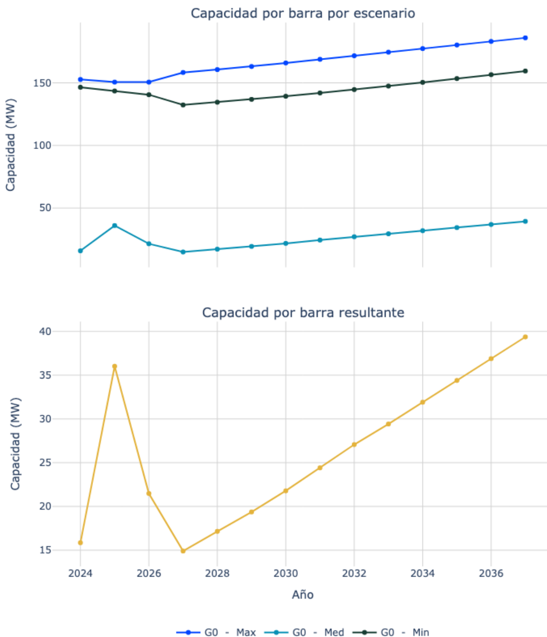
Figura 66. Capacidad de transporte de la subestación Fundación 110.
