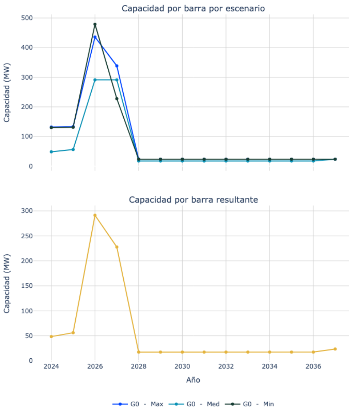
Figura 135. Capacidad de transporte de la subestación Sta Marta 1 Sec 2 34.5.
