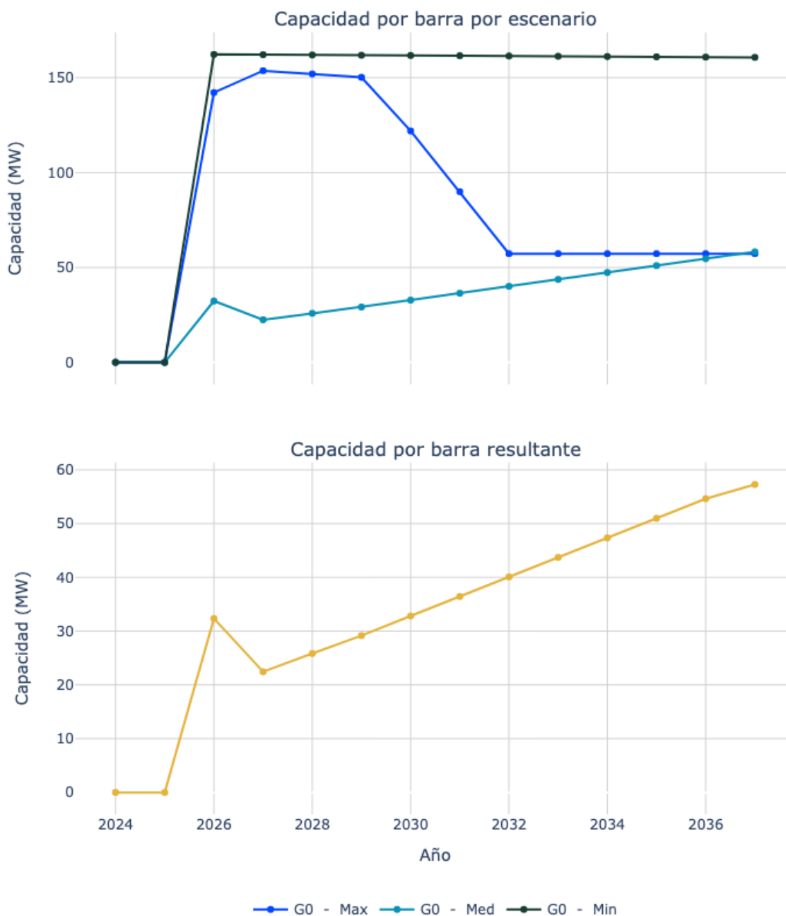
Figura 71. Capacidad de transporte de la subestación Guacamayal 110.
