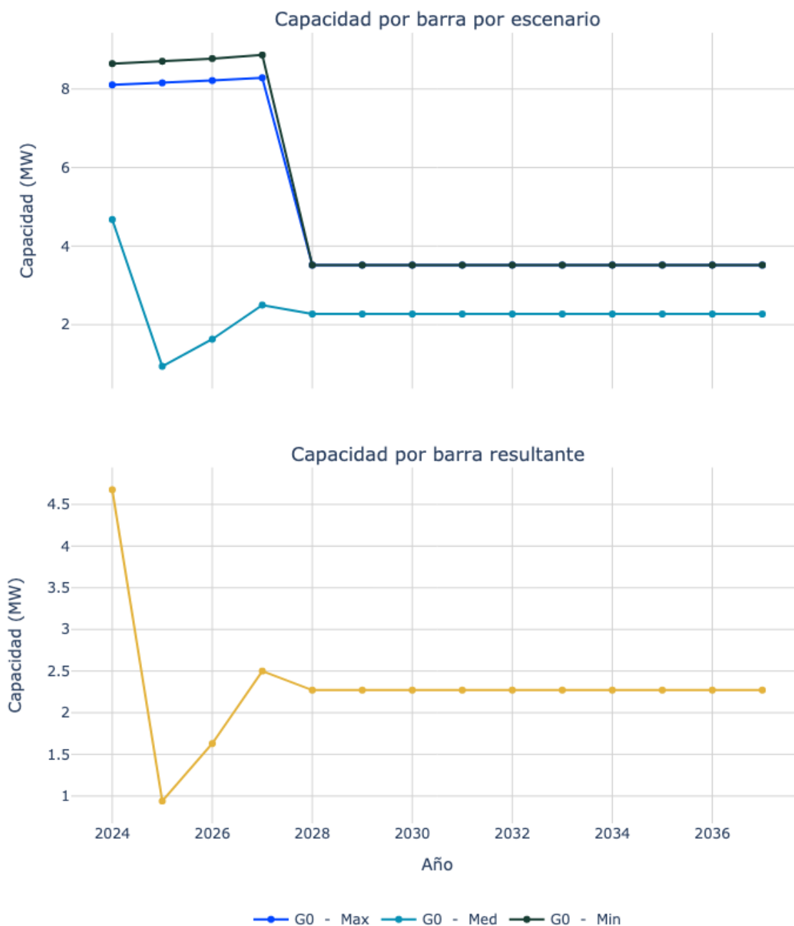
Figura 105. Capacidad de transporte de la subestación Nueva Granada 34.5.
