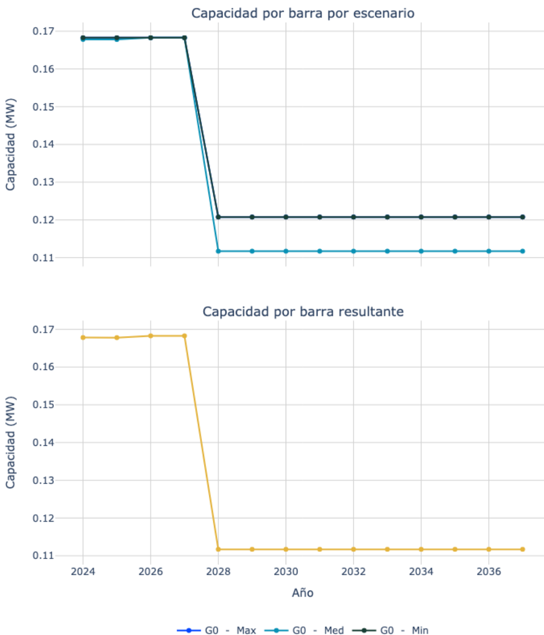
Figura 55. Capacidad de transporte de la subestación EL PASO 1 34.5 kV.
