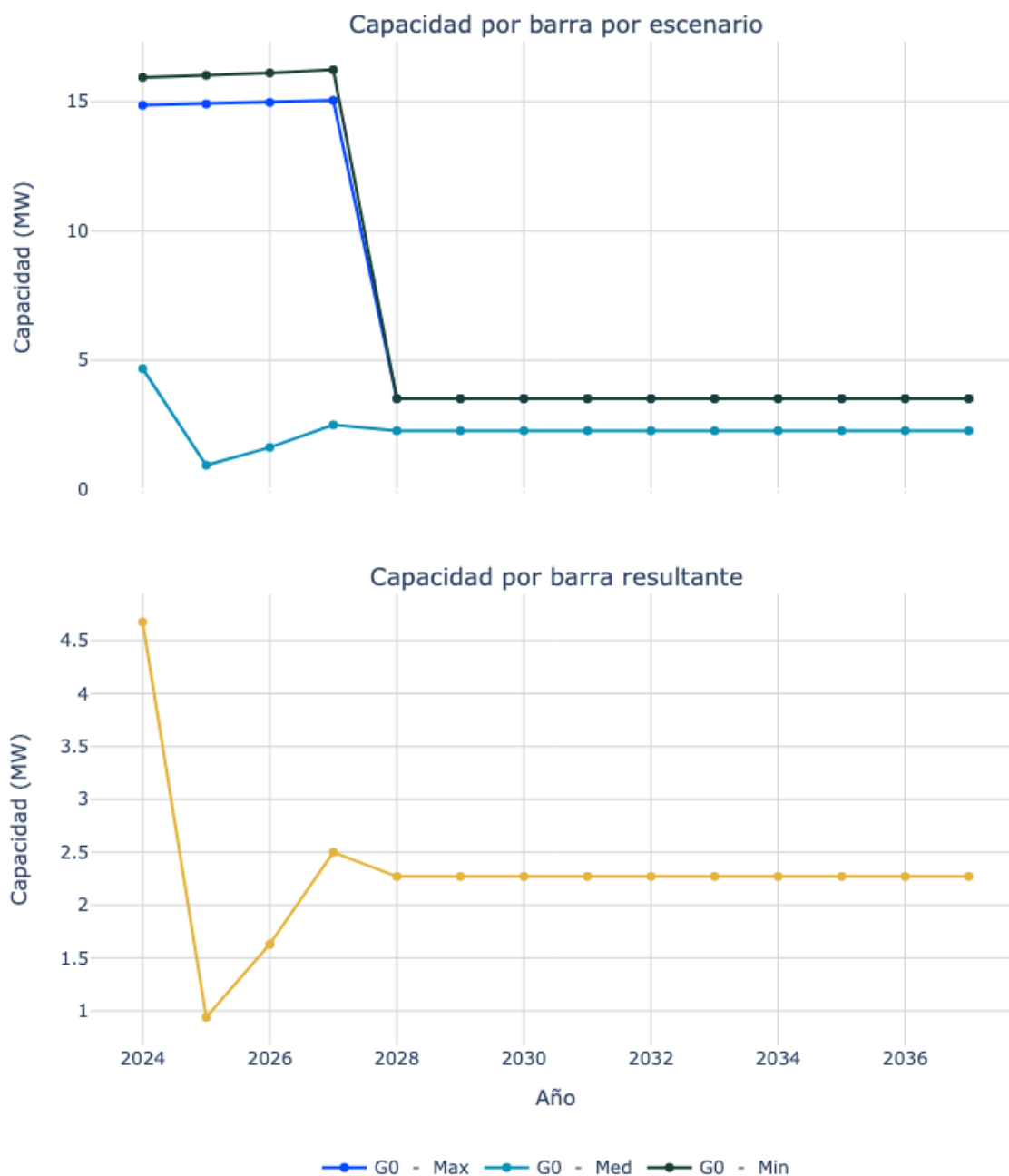
Figura 90. Capacidad de transporte de la subestación La salvacion 13.8.
