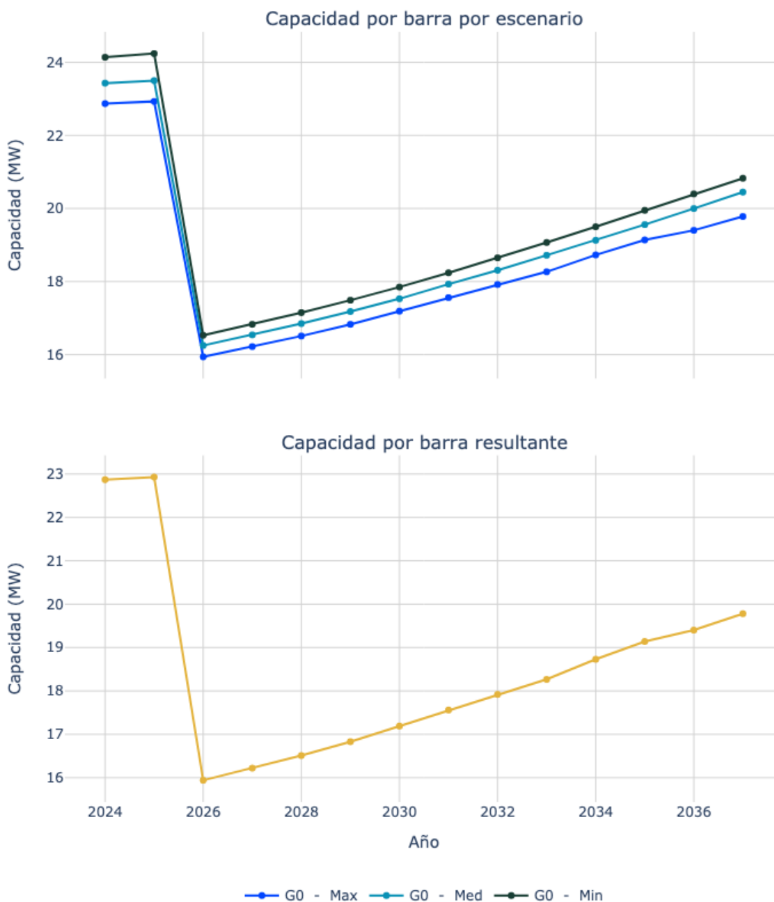
Figura 126. Capacidad de transporte de la subestación San Felipe 34.5.
