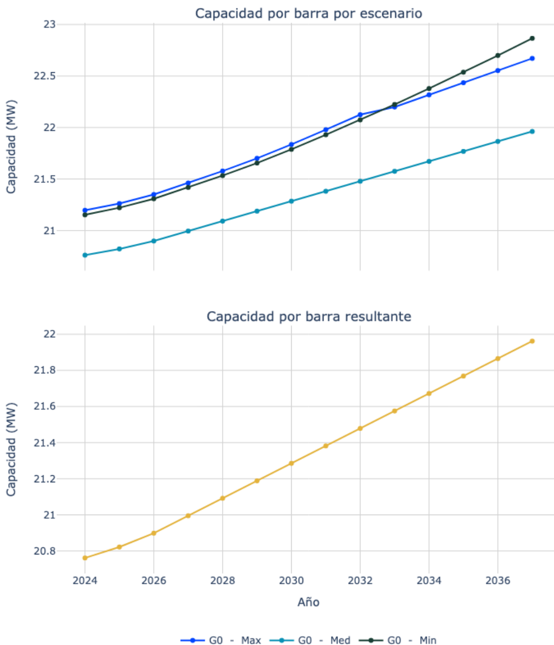
Figura 62. Capacidad de transporte de la subestación El reten 34.5.
