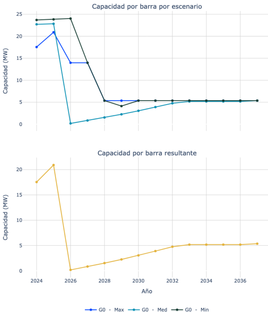
Figura 93. Capacidad de transporte de la subestación Llerasca 34.5.
