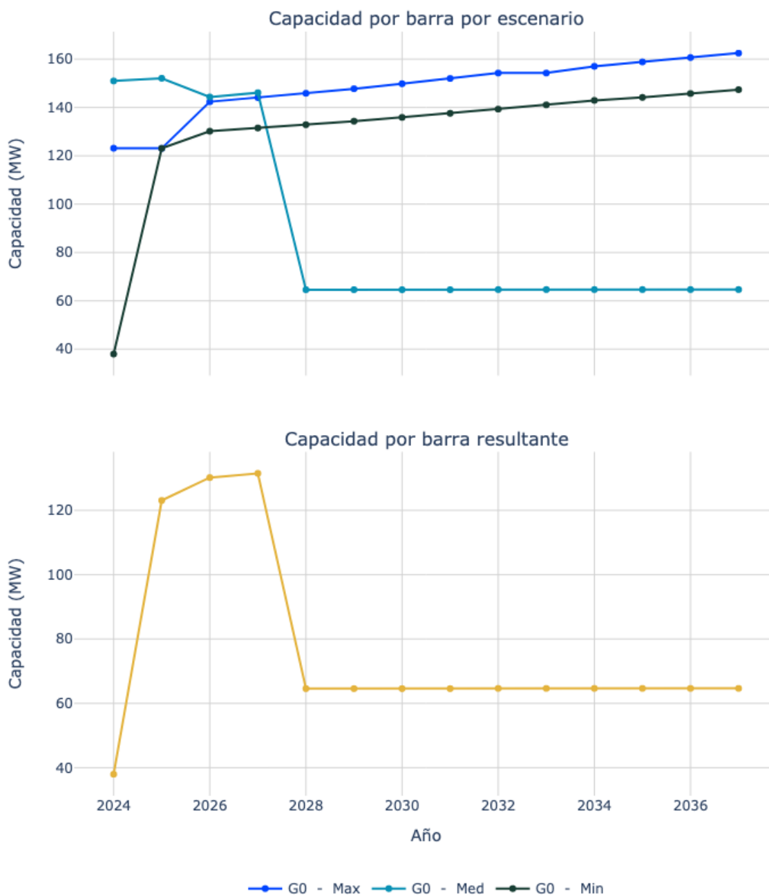
Figura 102. Capacidad de transporte de la subestación Manzanares 110.
