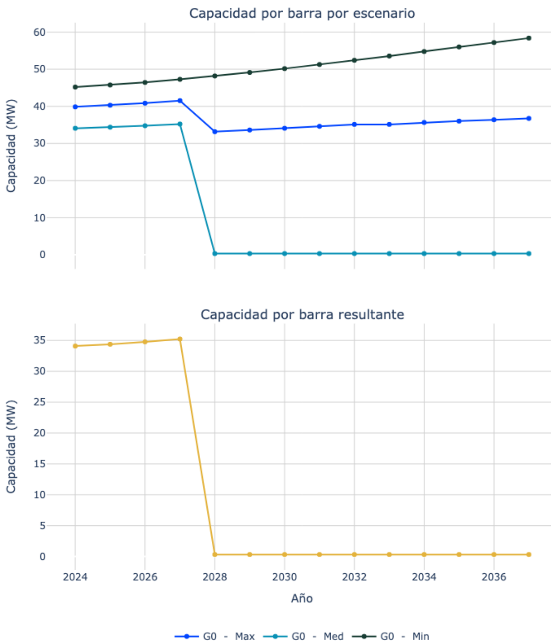
Figura 133. Capacidad de transporte de la subestación Santa Teresa 34.5.
