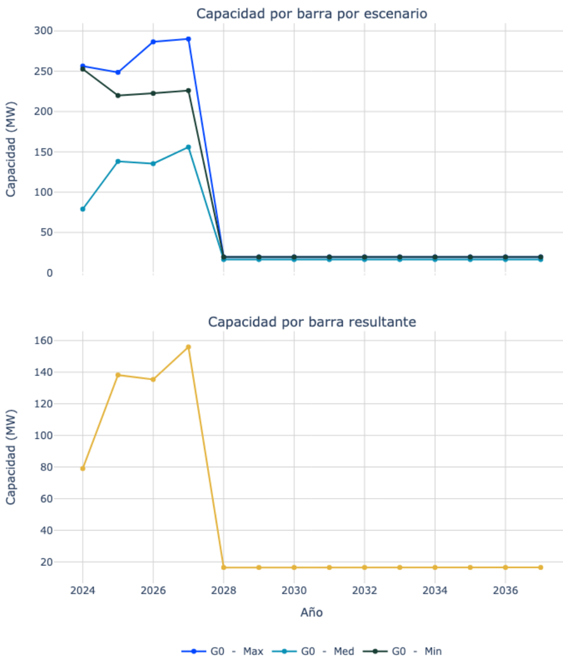
Figura 115. Capacidad de transporte de la subestación RIOHACHA 1 34.5 kV.
