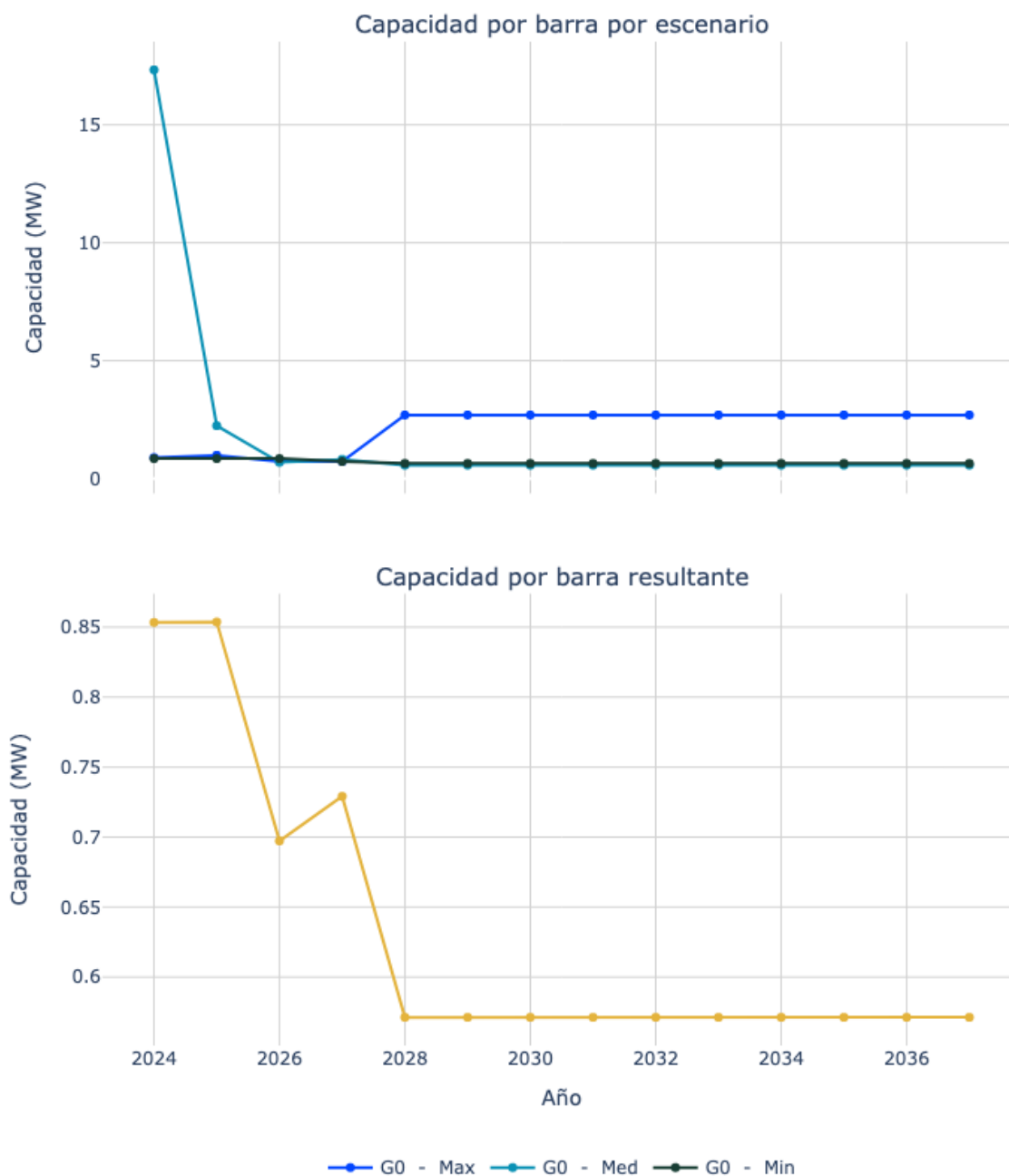
Figura 81. Capacidad de transporte de la subestación LA LOMA 3 13.8 kV.
