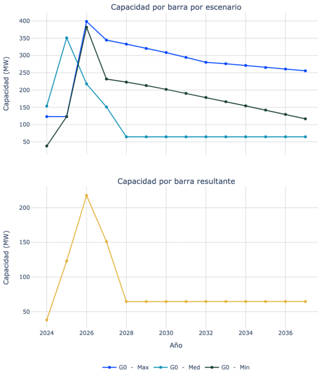
Figura 131. Capacidad de transporte de la subestación Santa Marta 110.
