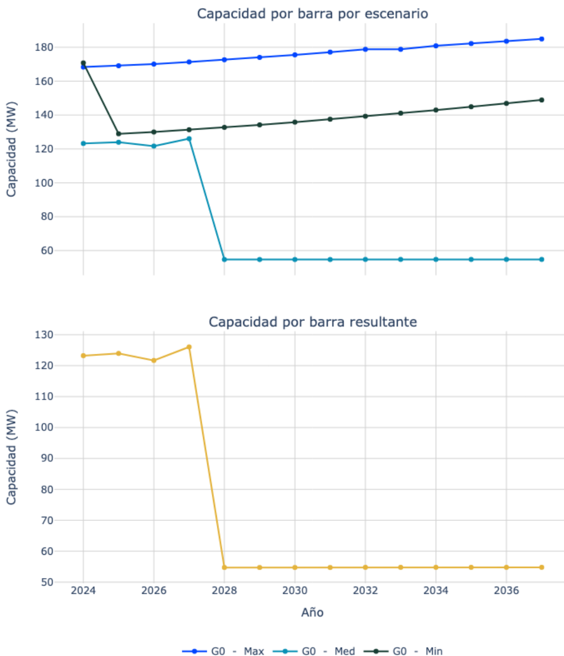
Figura 99. Capacidad de transporte de la subestación Maicao 110.
