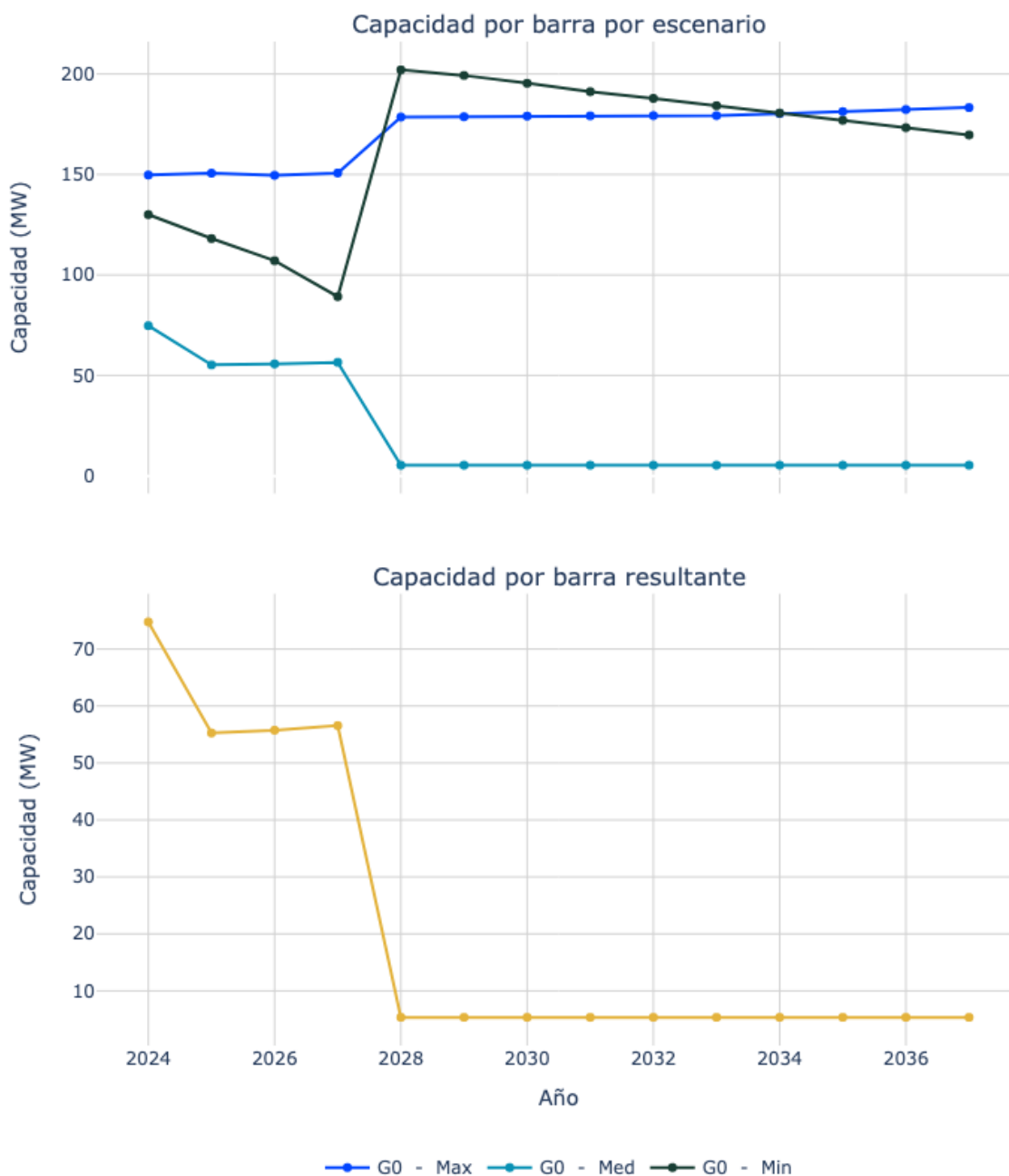
Figura 58. Capacidad de transporte de la subestación El Paso 110.
