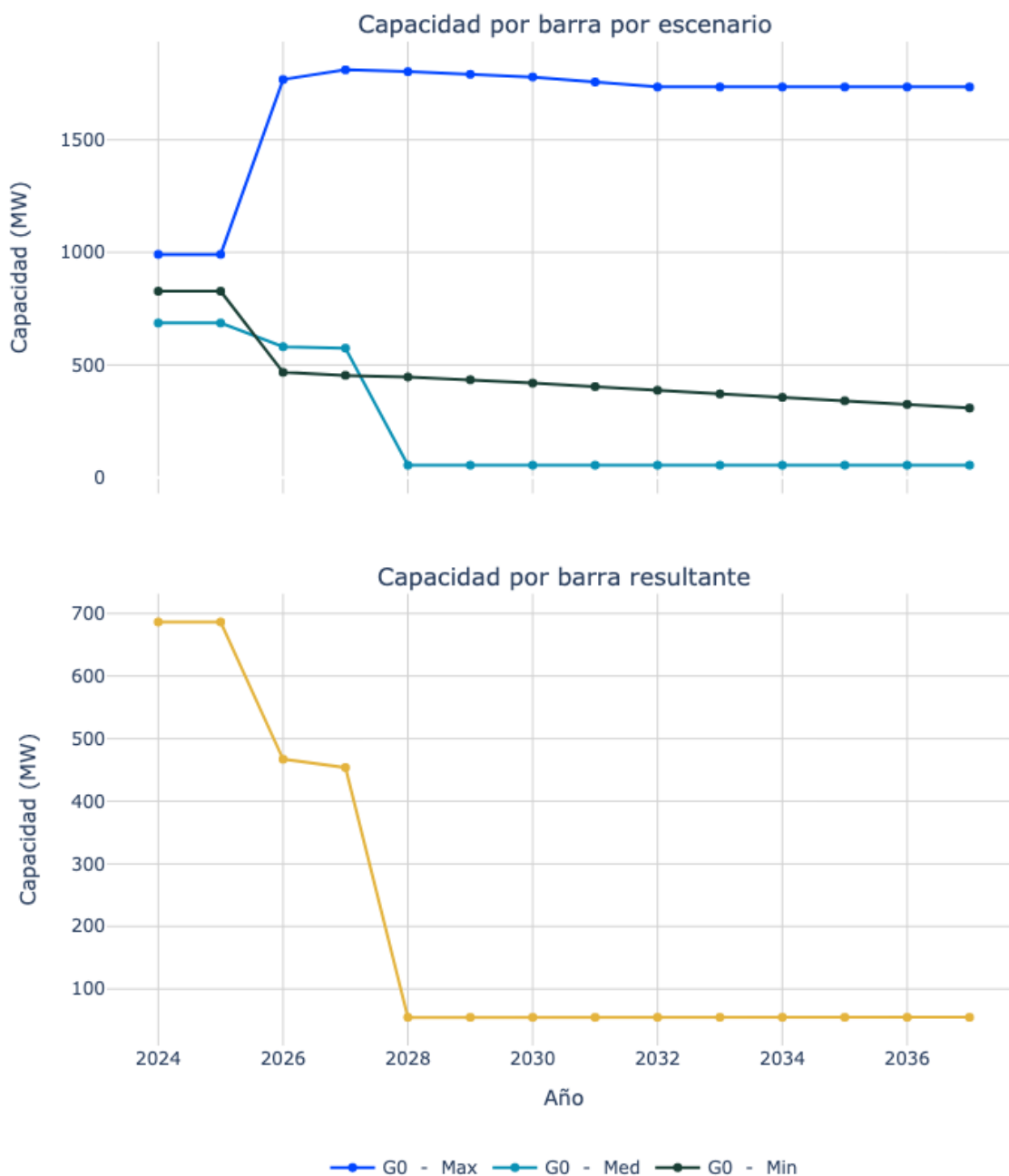
Figura 47. Capacidad de transporte de la subestación Cuestecita II 220.
