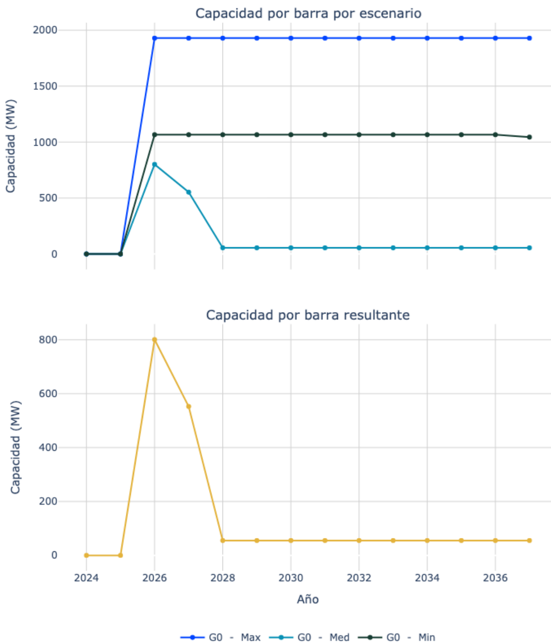
Figura 41. Capacidad de transporte de la subestación Colectora 1 Eolica 500.
