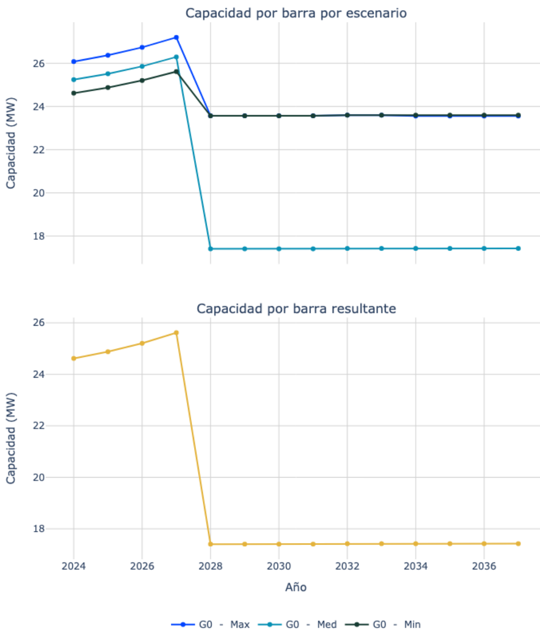
Figura 25. Capacidad de transporte de la subestación Bonda 13.8.
