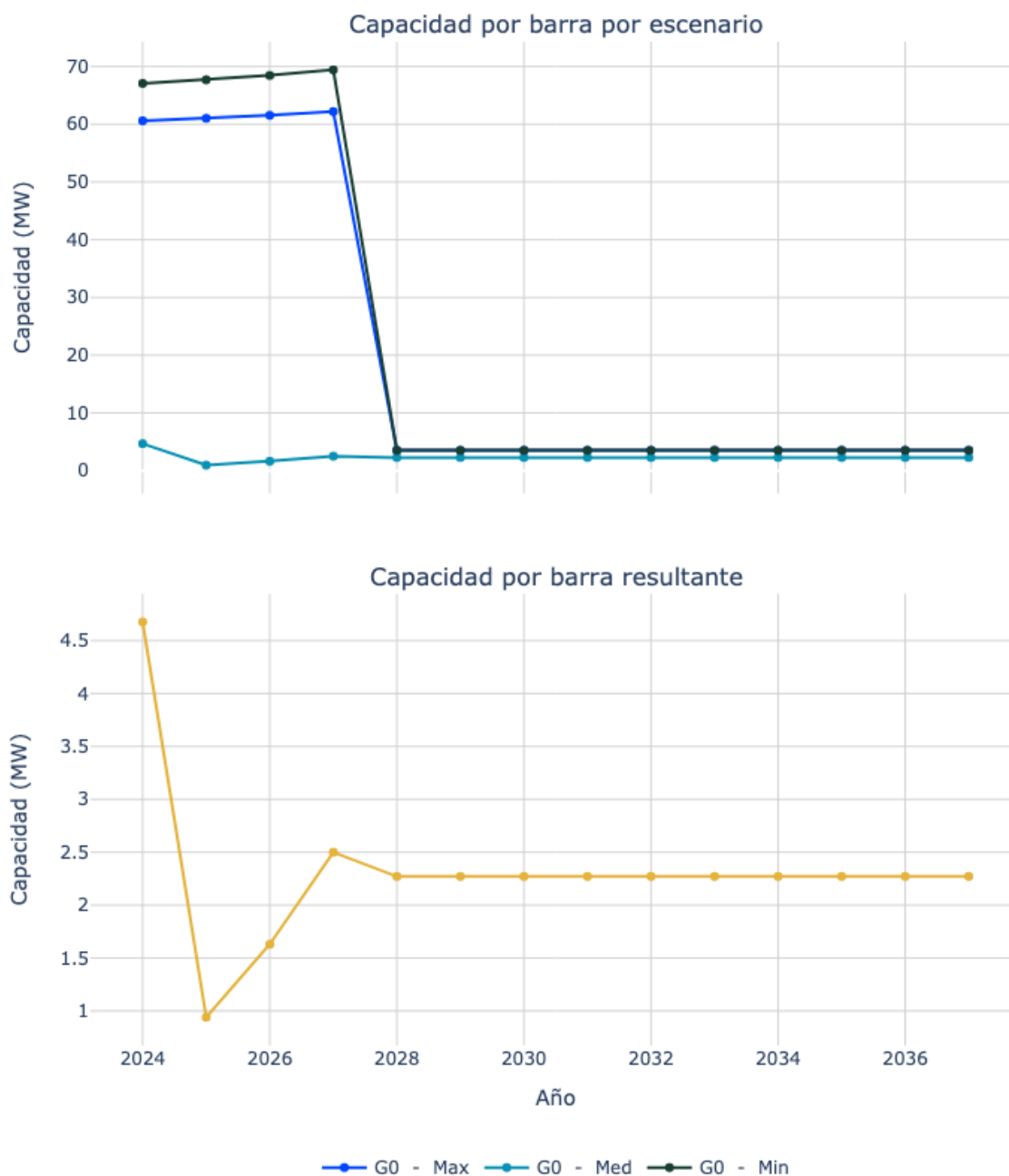
Figura 44. Capacidad de transporte de la subestación Copey 34.5 1.
