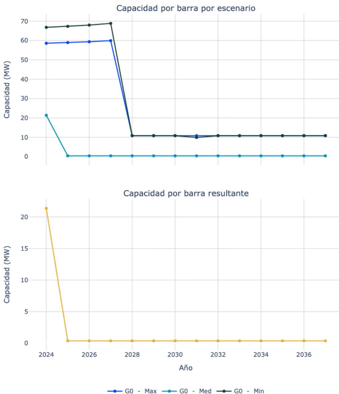
Figura 150. Capacidad de transporte de la subestación Valledupar34.5_B3.
