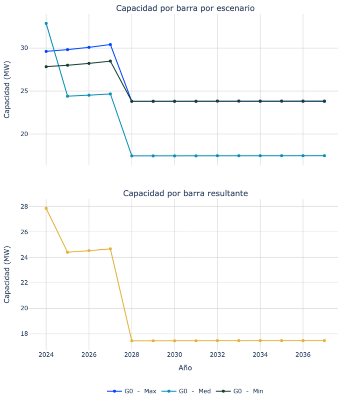
Figura 154. Capacidad de transporte de la subestación Zawady 34.5.
