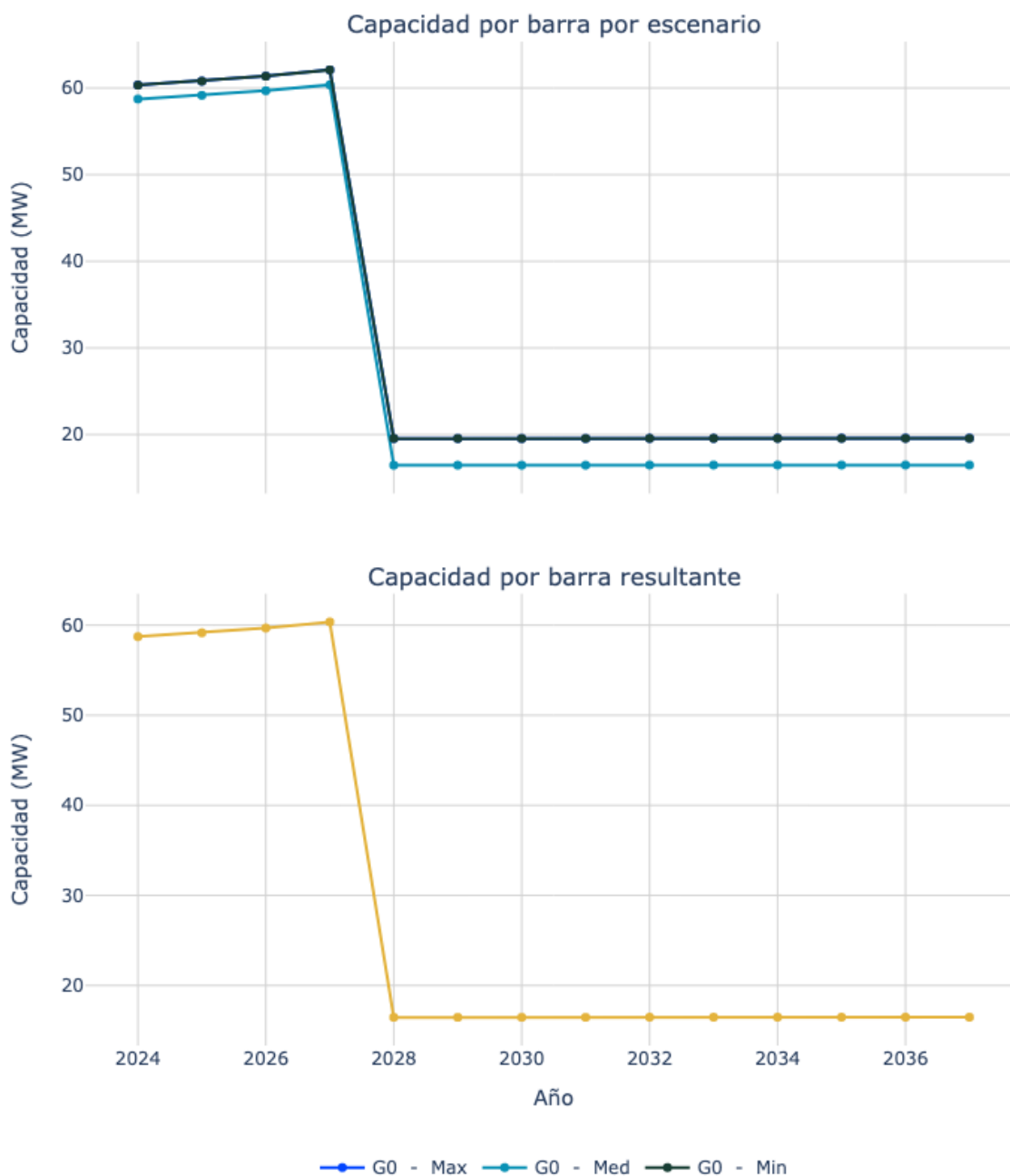
Figura 120. Capacidad de transporte de la subestación RIOHACHA 4 13.8 kV.
