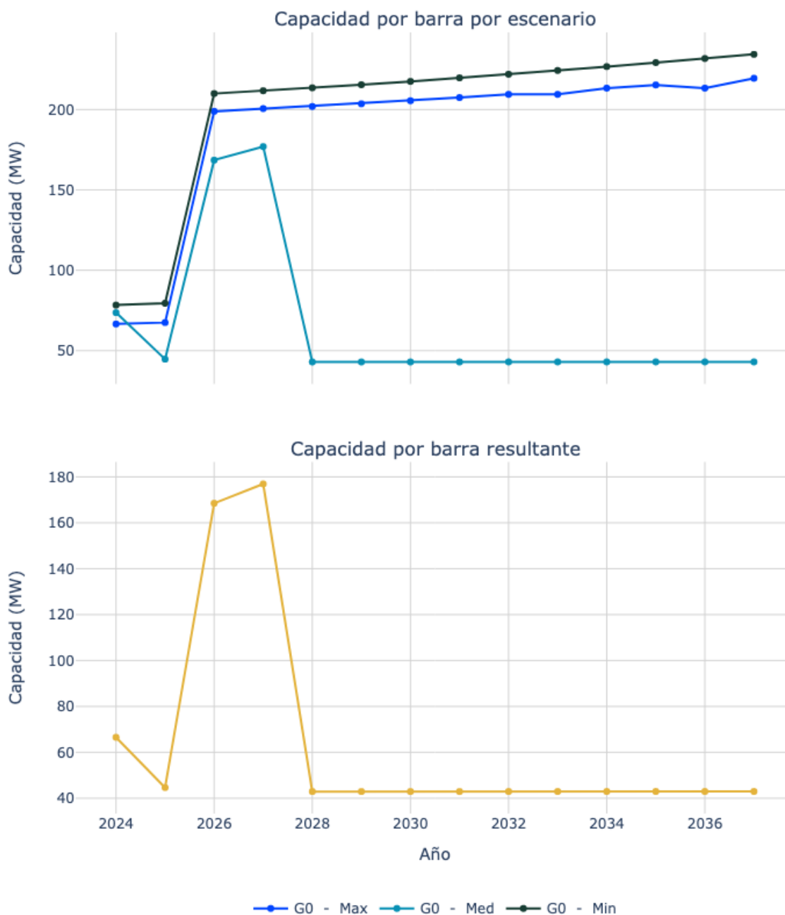
Figura 77. Capacidad de transporte de la subestación Guatapurí 110.
