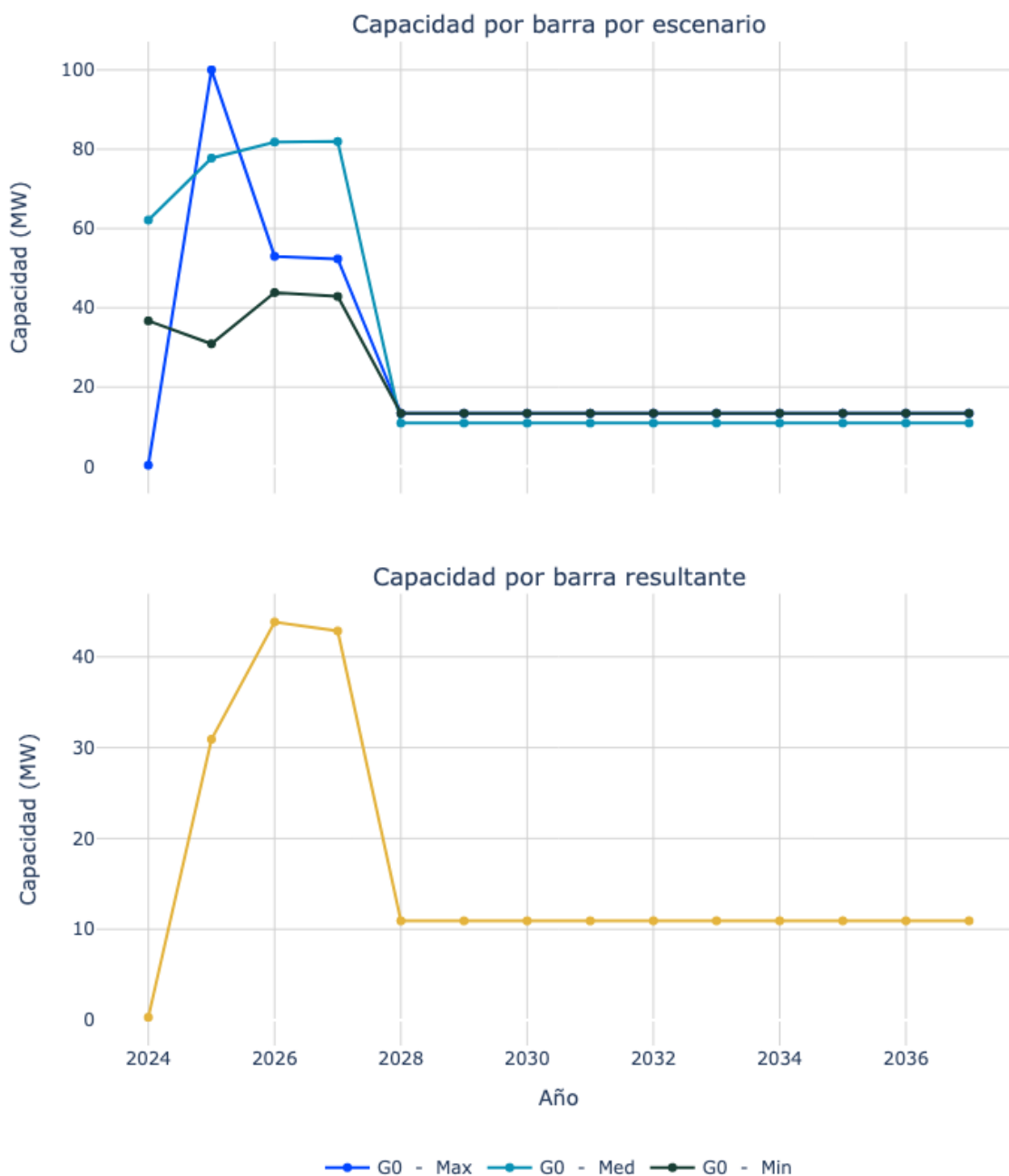
Figura 145. Capacidad de transporte de la subestación Valledupar 13.8 T1.
