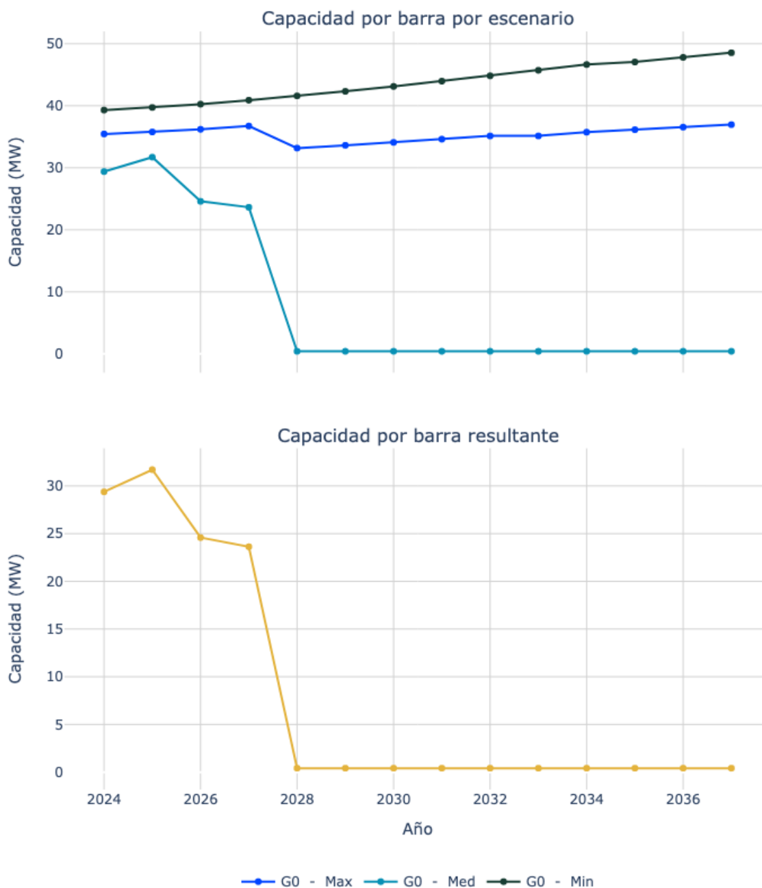
Figura 109. Capacidad de transporte de la subestación Pailitas 34.5.
