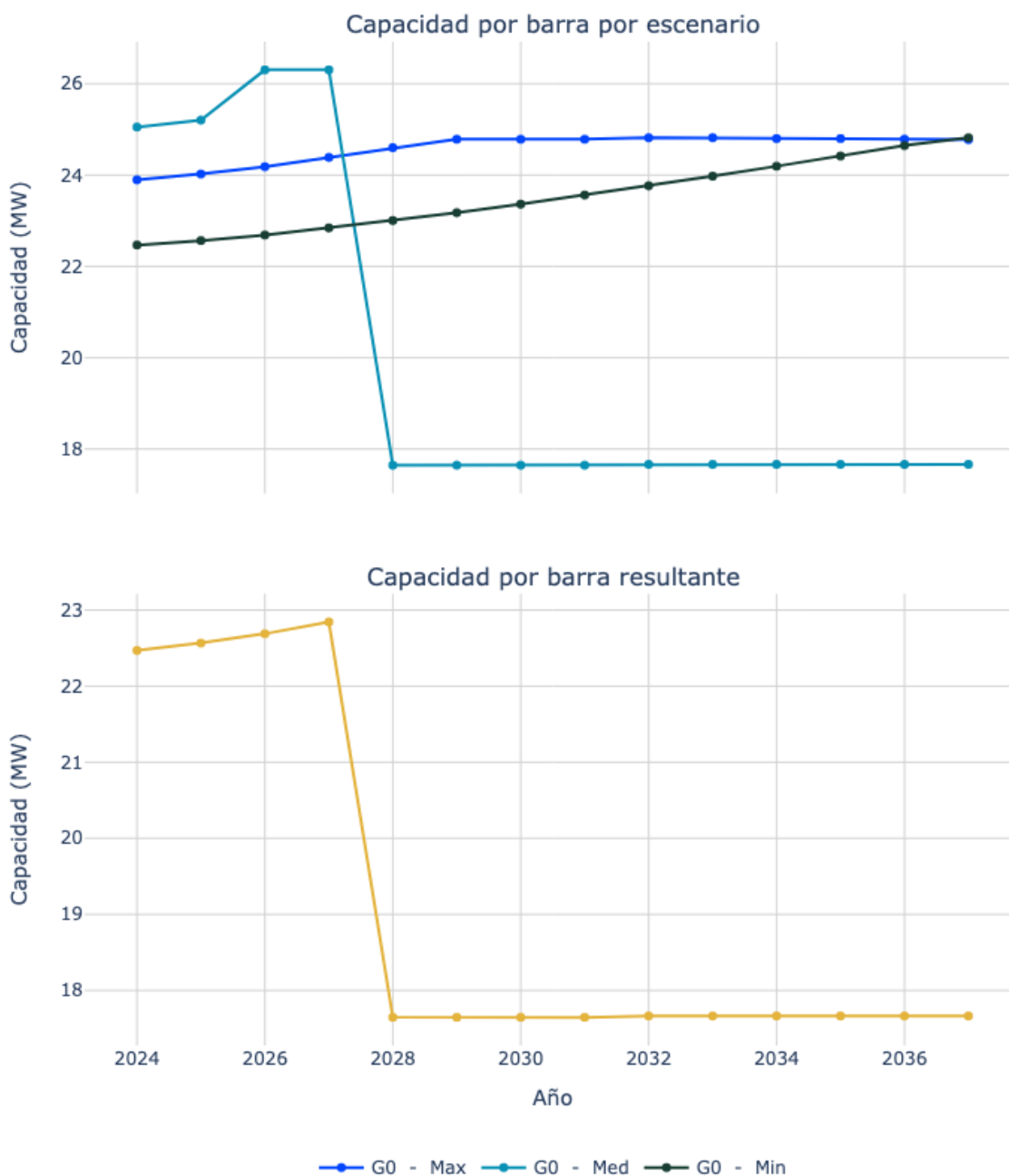
Figura 73. Capacidad de transporte de la subestación Guacamayal 34.5.
