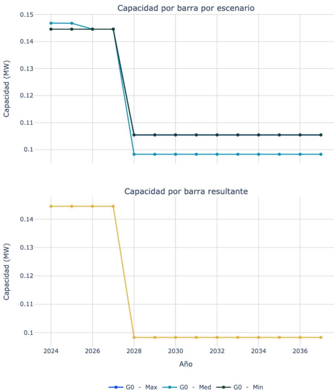
Figura 61. Capacidad de transporte de la subestación El paraíso 34.5.
