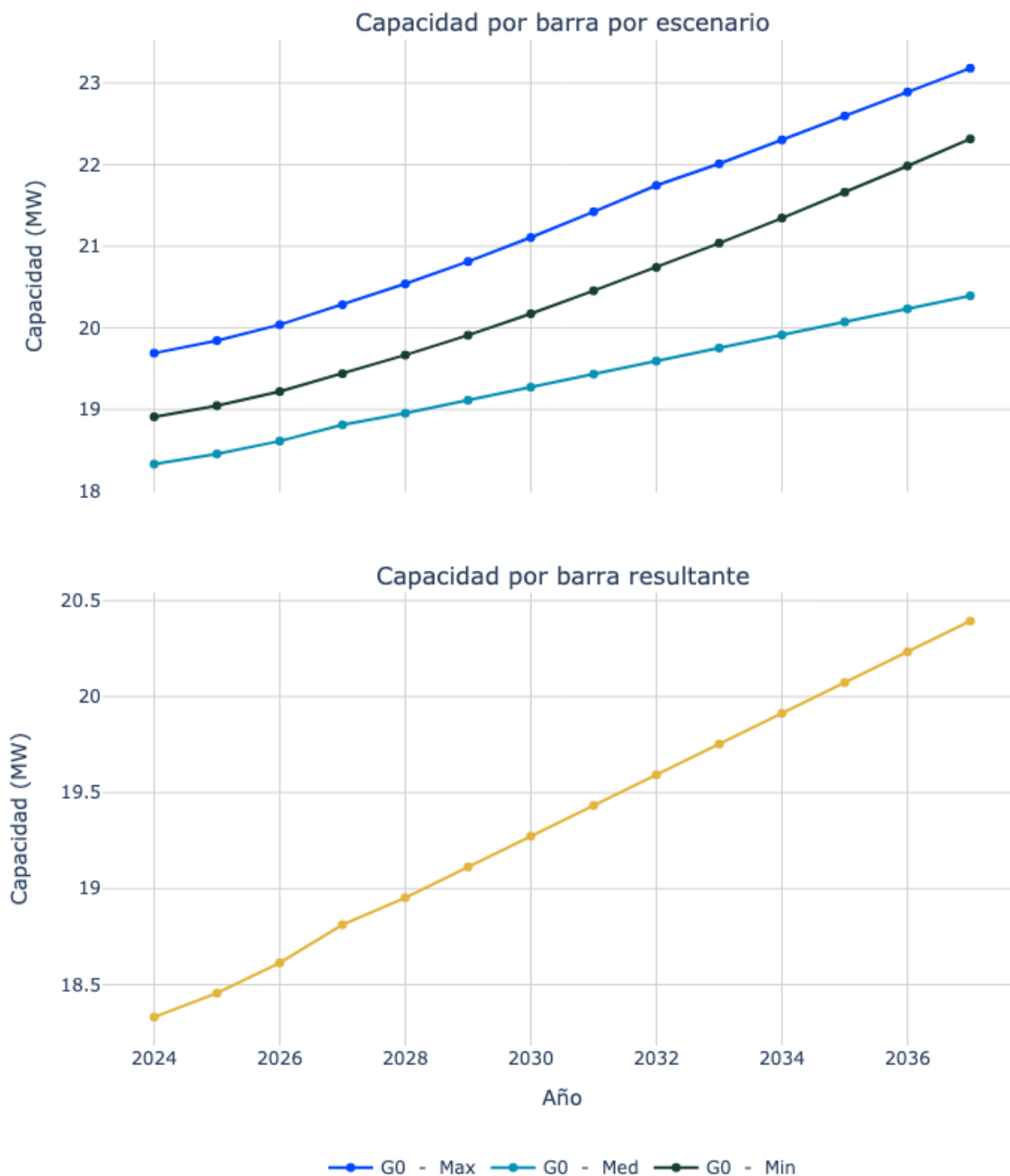
Figura 15. Capacidad de transporte de la subestación Aracataca 13.8.
