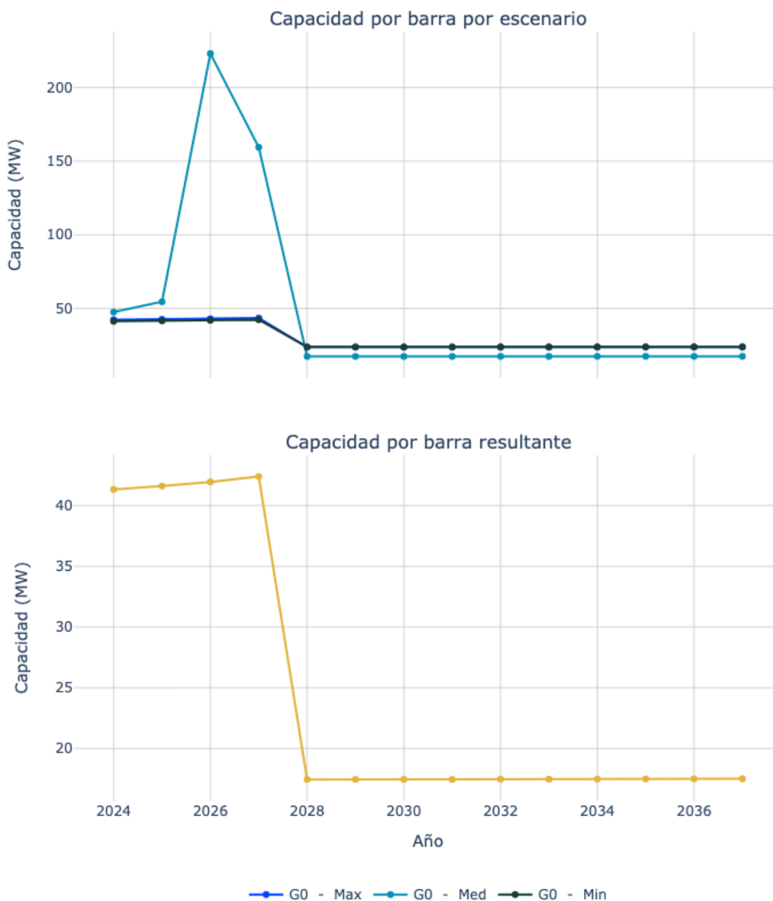
Figura 113. Capacidad de transporte de la subestación RIO CORDOBA 1 34.5 kV.
