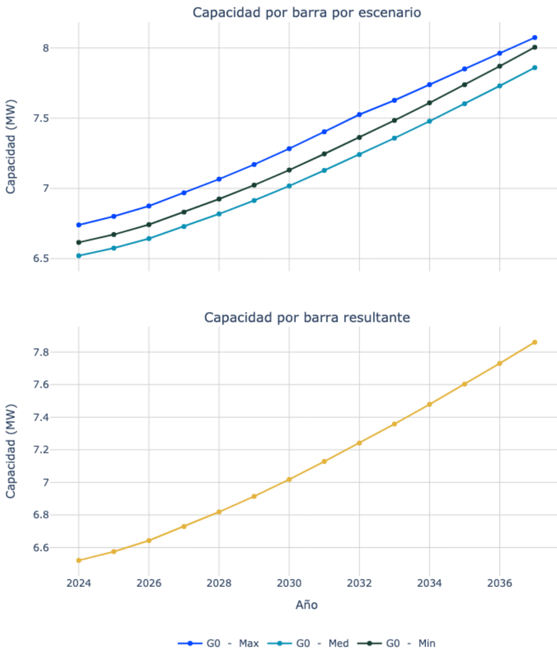
Figura 22. Capacidad de transporte de la subestación Barrancas 13.8 2.
