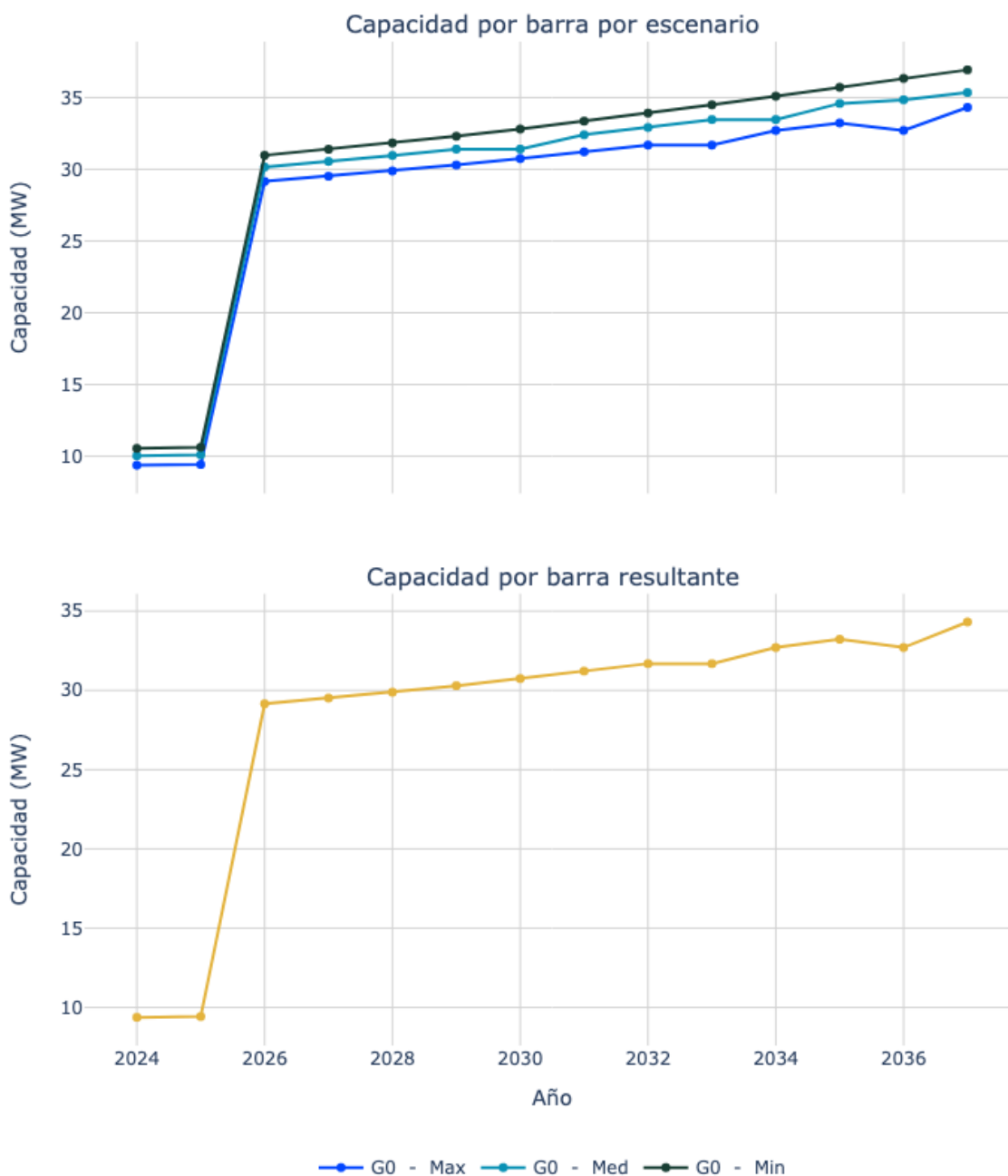
Figura 75. Capacidad de transporte de la subestación Guamal 34.5.
