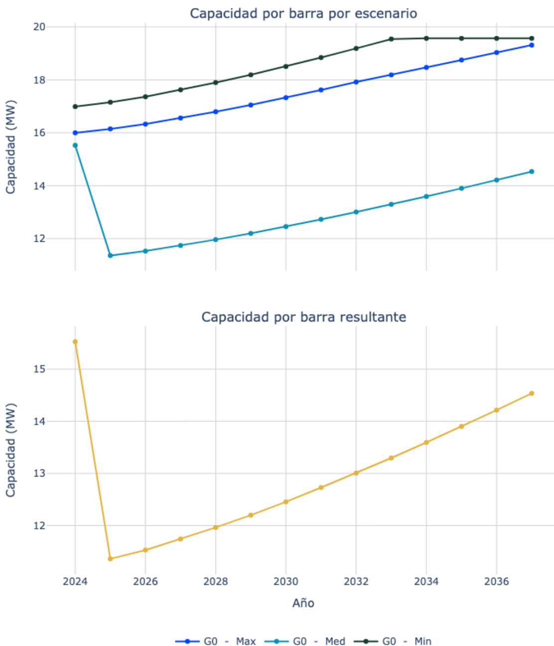
Figura 45. Capacidad de transporte de la subestación Cuestecita 13.8.
