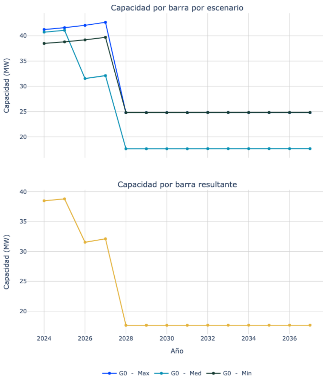
Figura 16. Capacidad de transporte de la subestación Aracataca 34.5.
