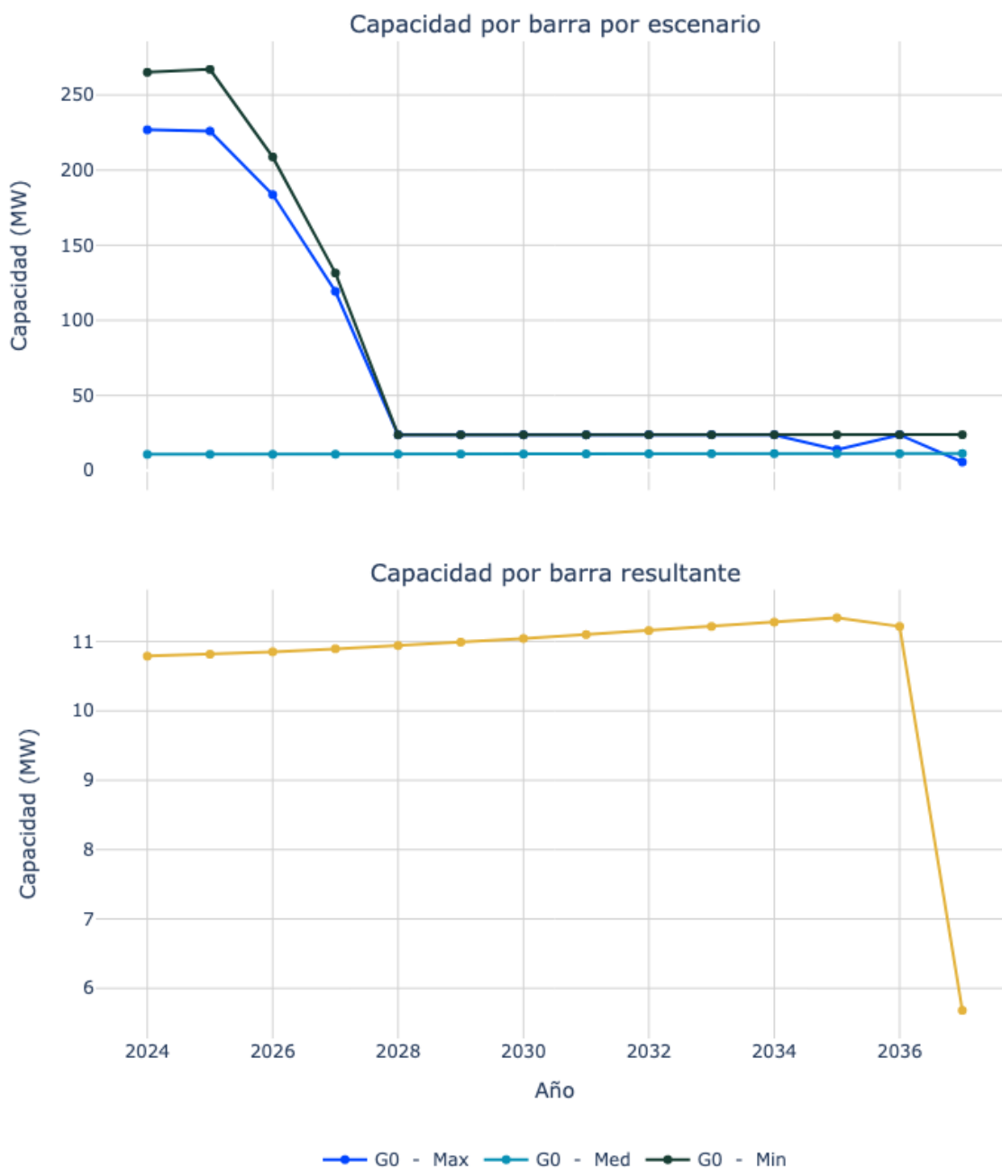
Figura 112. Capacidad de transporte de la subestación RIO CORDOBA 1 13.8 kV.
