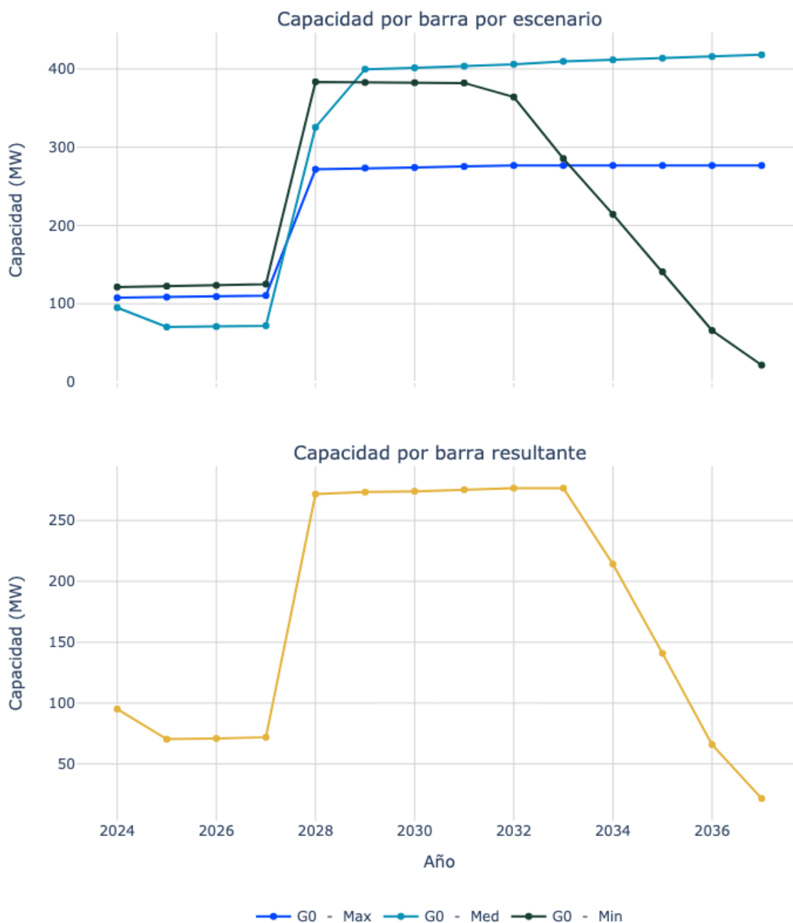
Figura 56. Capacidad de transporte de la subestación El Banco 110.
