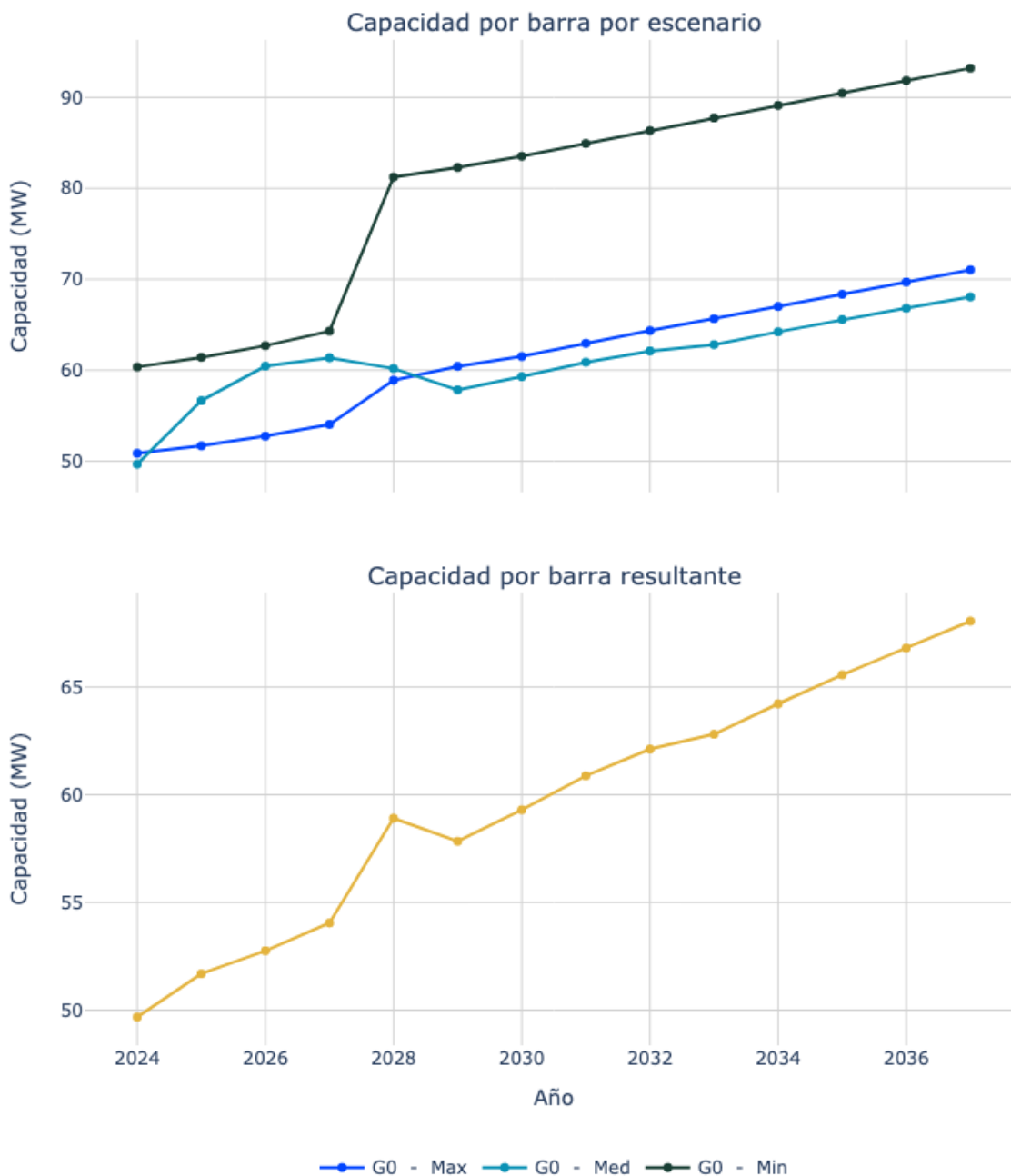
Figura 53. Capacidad de transporte de la subestación EL BANCO 1 34.5 kV.
