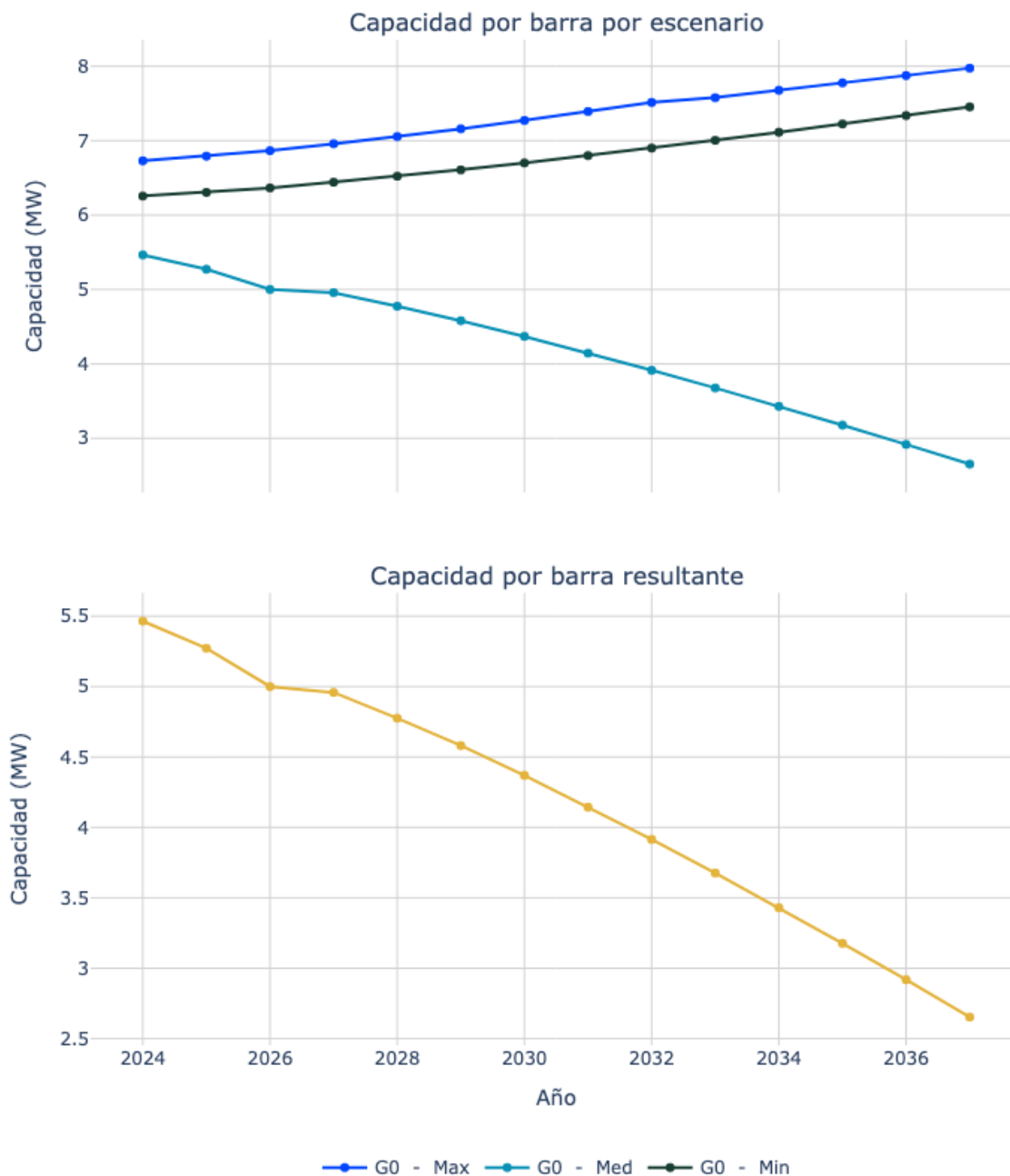
Figura 34. Capacidad de transporte de la subestación Camarones 13.8.
