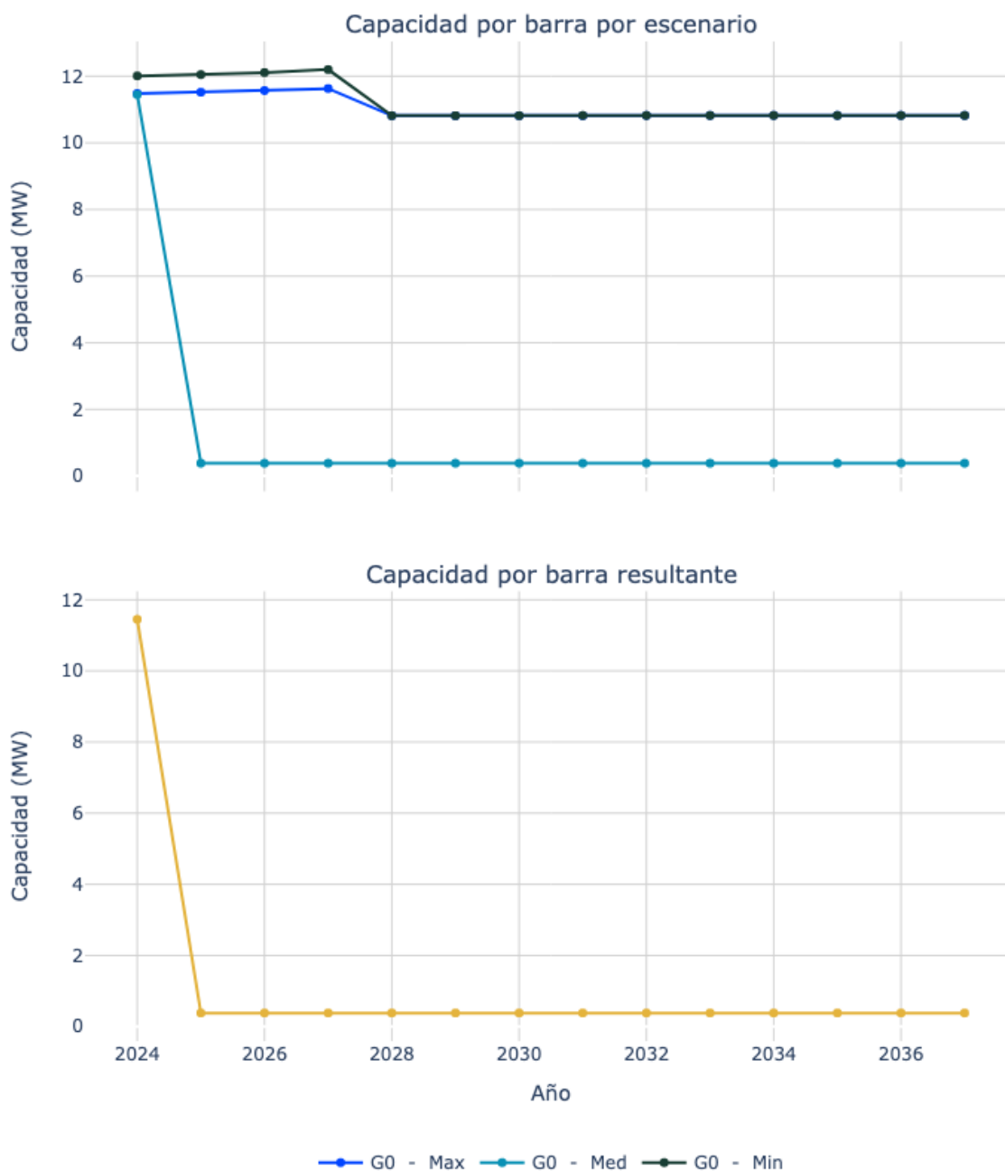
Figura 103. Capacidad de transporte de la subestación Maria Angola 34.5.
