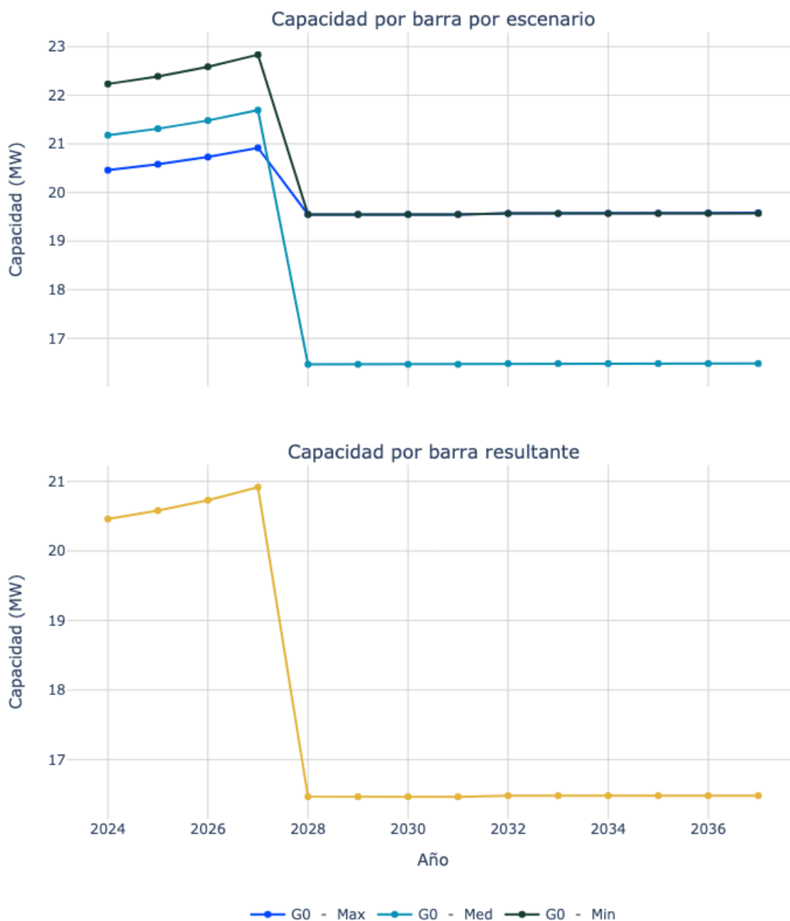
Figura 23. Capacidad de transporte de la subestación Barrancas 34.5.
