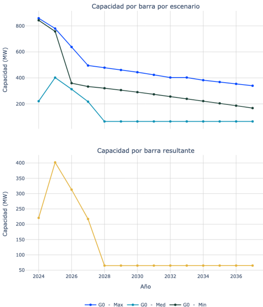
Figura 111. Capacidad de transporte de la subestación R Cordoba 220.
