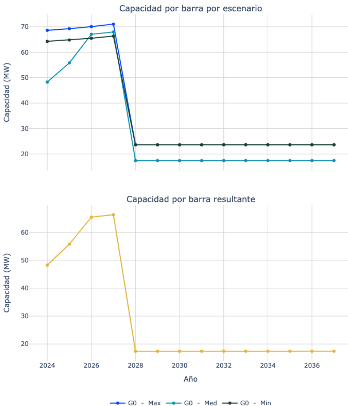
Figura 68. Capacidad de transporte de la subestación GAIRA 1 13.8 kV.
