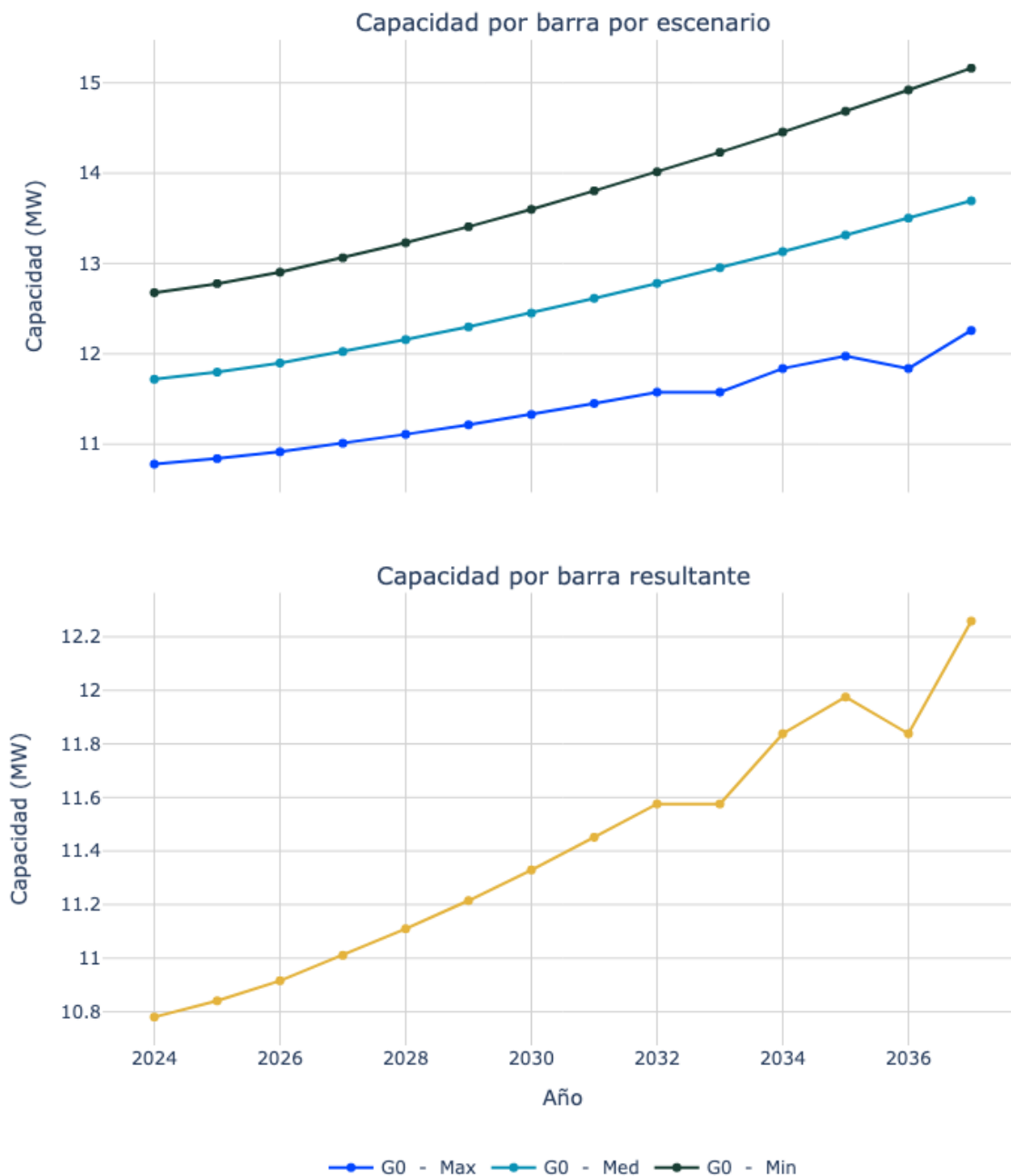
Figura 21. Capacidad de transporte de la subestación Barrancas 13.8 1.
