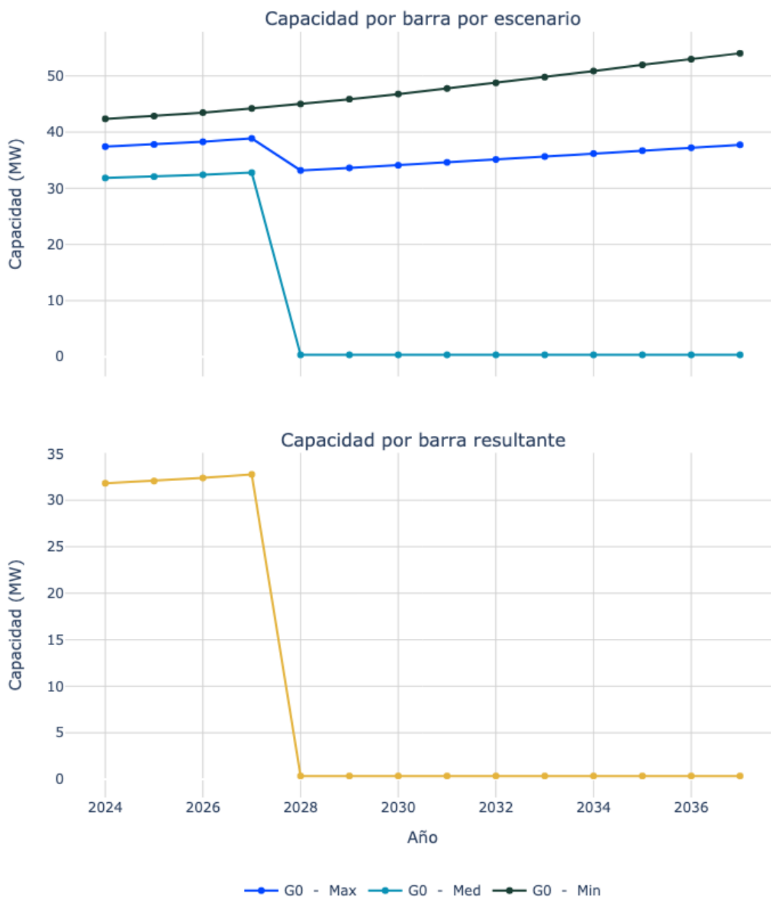
Figura 136. Capacidad de transporte de la subestación Tamalameque 34.5.
