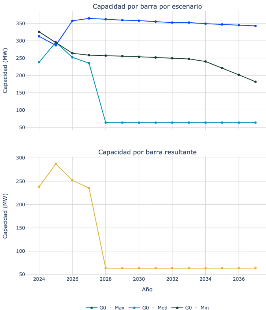
Figura 137. Capacidad de transporte de la subestación Termocol 220.
