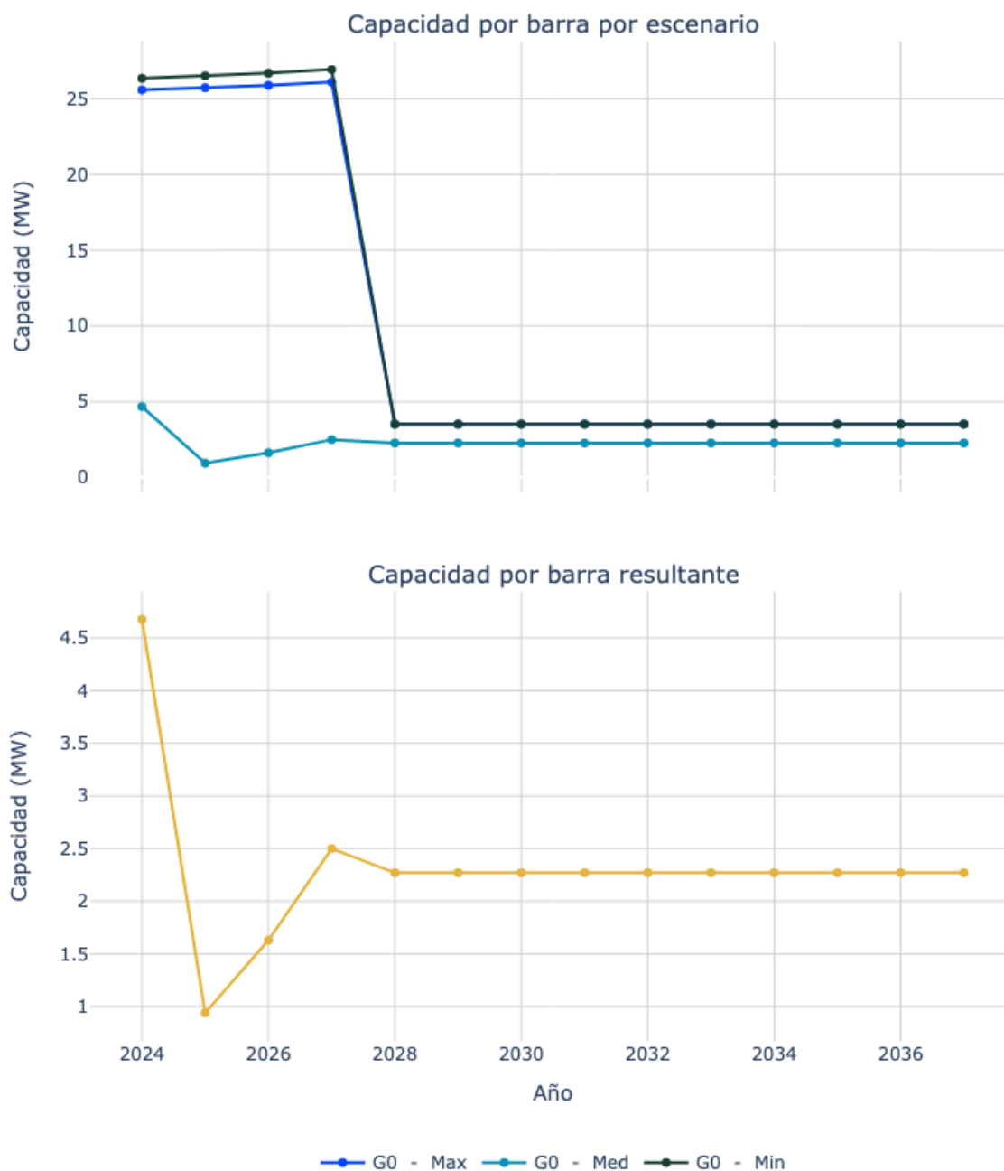
Figura 110. Capacidad de transporte de la subestación Pueblo nuevo 34.5.
