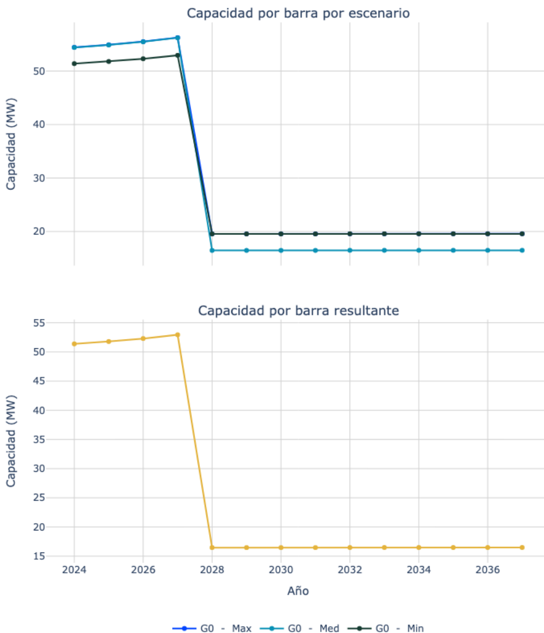
Figura 114. Capacidad de transporte de la subestación RIOHACHA 1 13.2 kV.
