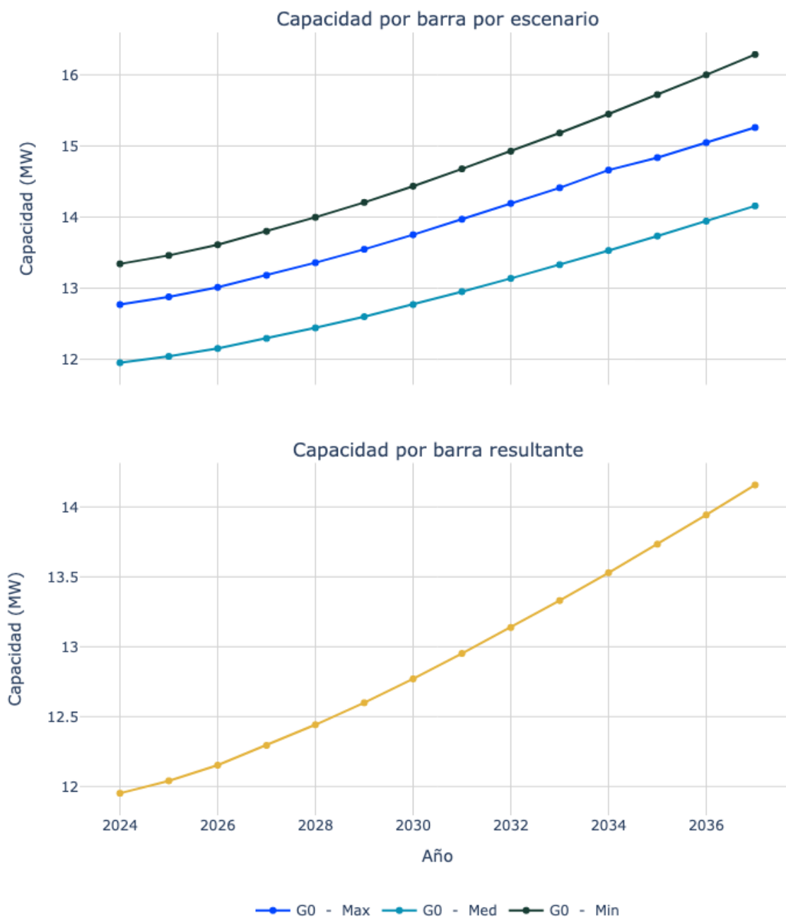
Figura 138. Capacidad de transporte de la subestación Termoguajira 13.8.
