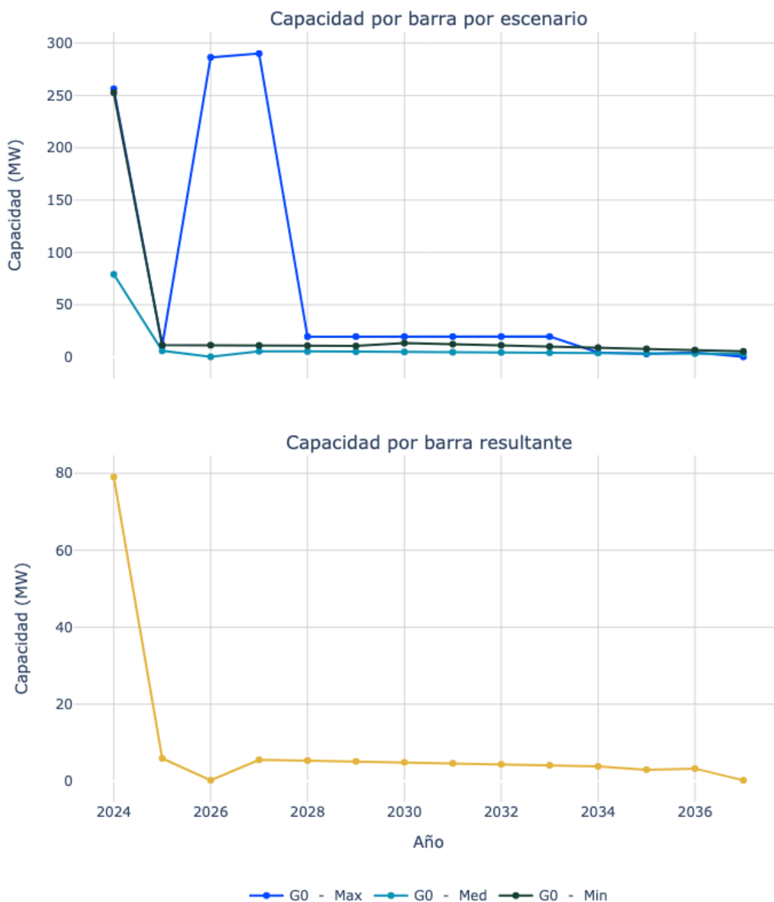
Figura 118. Capacidad de transporte de la subestación RIOHACHA 3 (13.8) kV.
