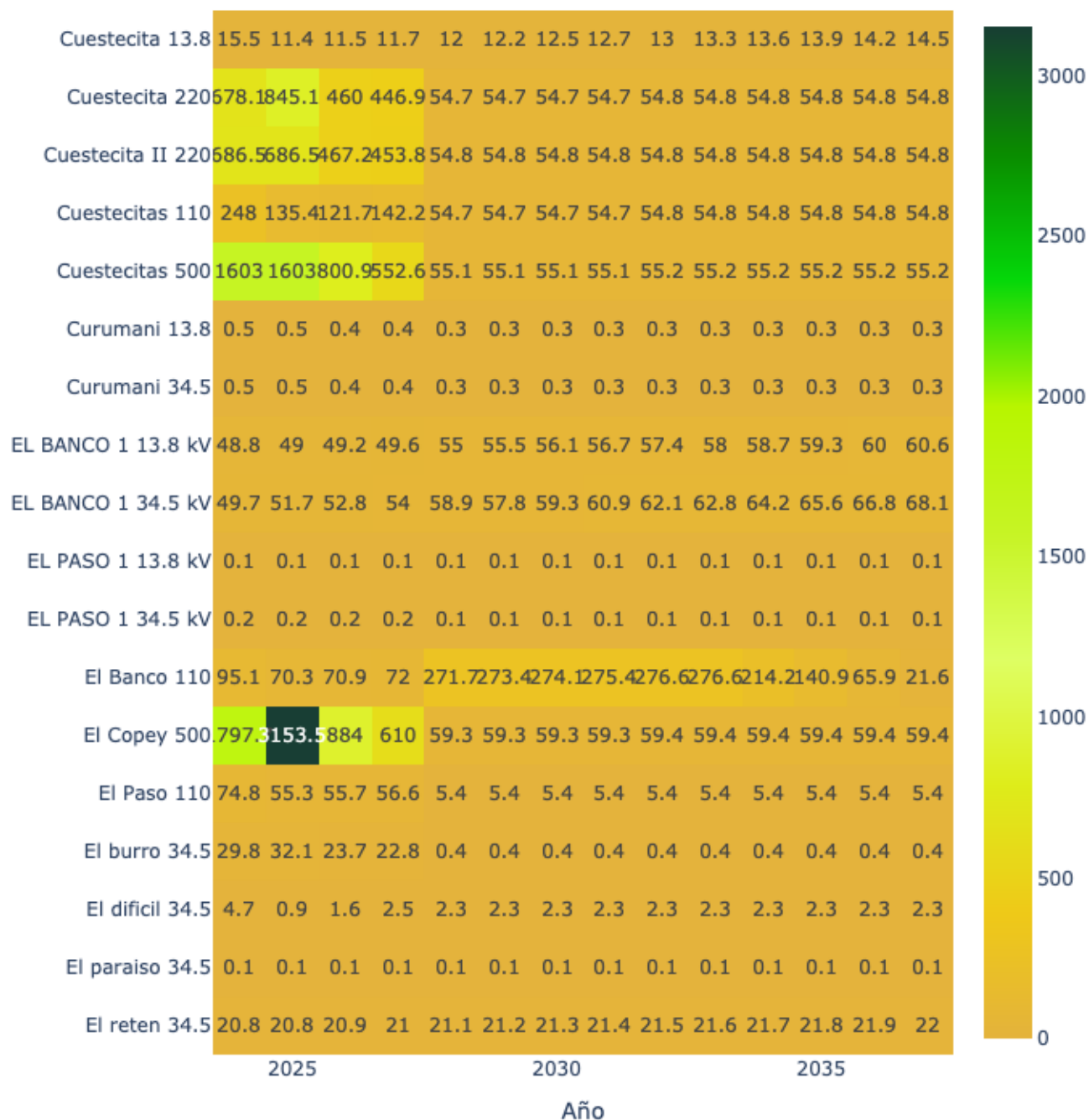
Figura 3. Mapa de calor con las capacidades de barra en la subárea GCM - Parte 3
