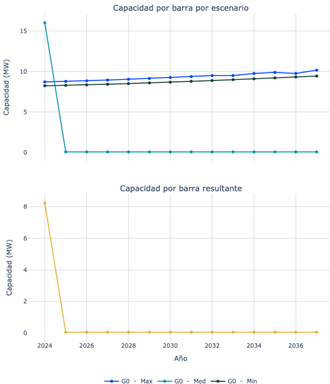
Figura 35. Capacidad de transporte de la subestación Camarones 34.5.
