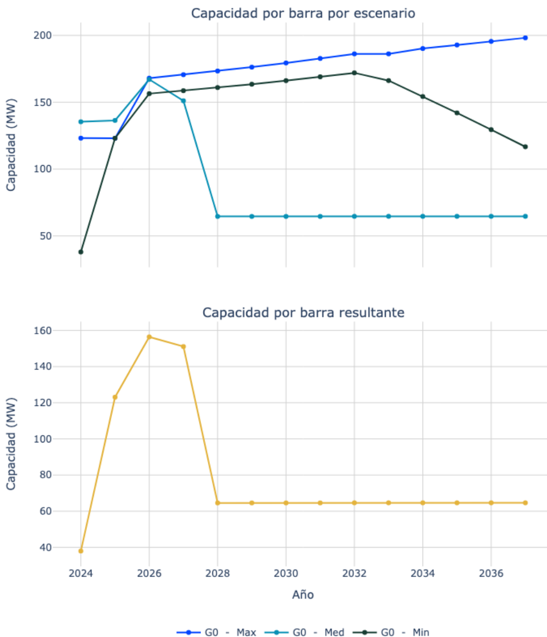
Figura 92. Capacidad de transporte de la subestación Libertad 110.
