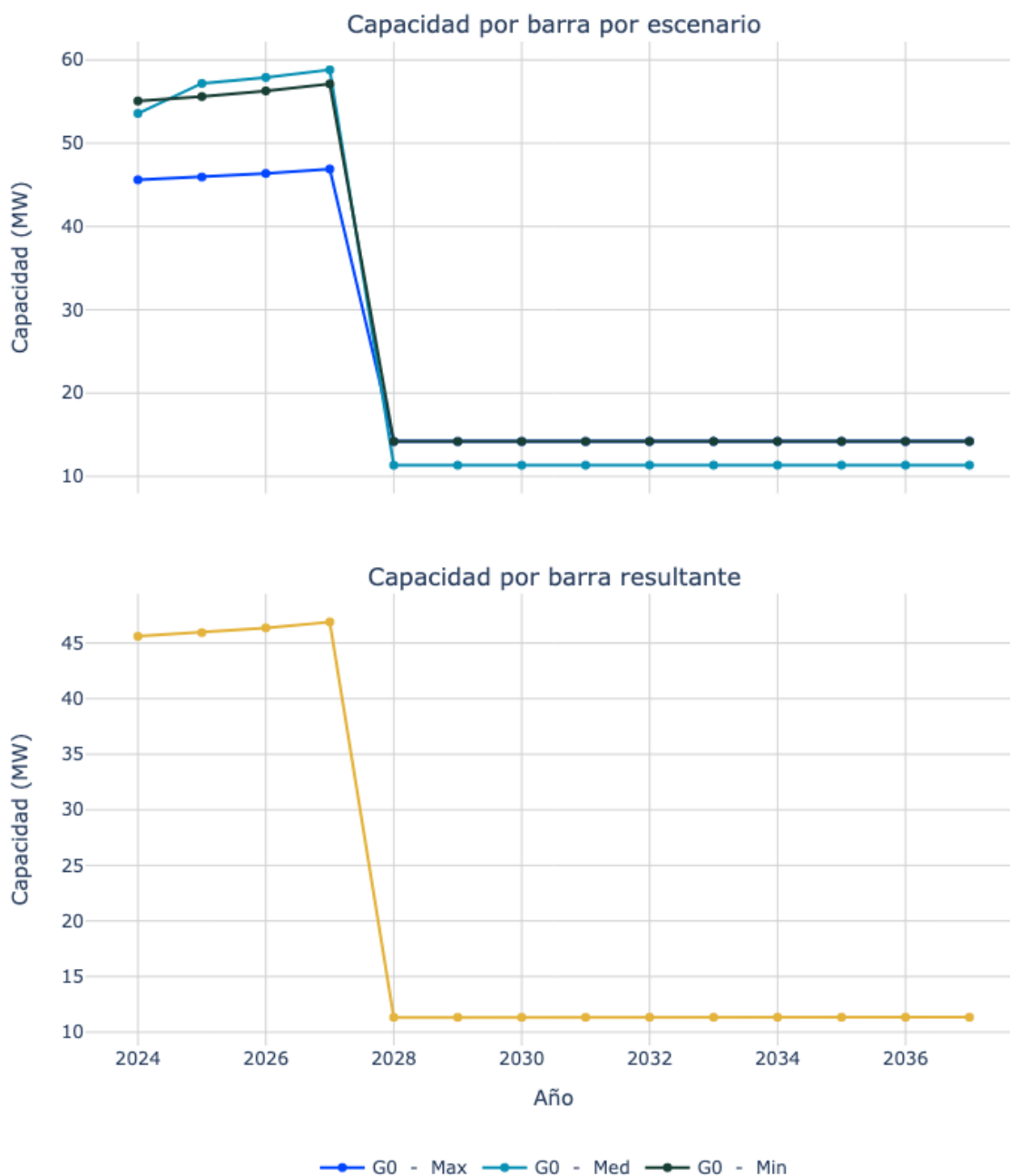
Figura 146. Capacidad de transporte de la subestación Valledupar 13.8 T3.
