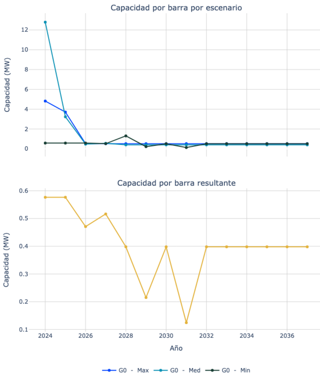
Figura 37. Capacidad de transporte de la subestación Chiriguana 13.8.
