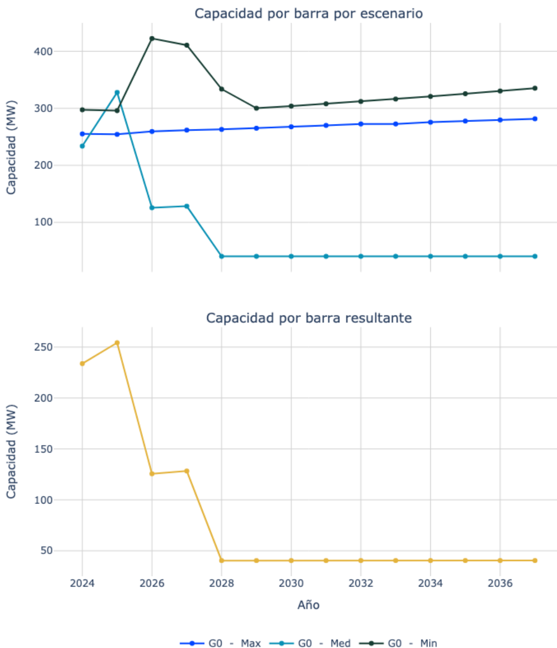
Figura 144. Capacidad de transporte de la subestación Valledupar 110.
