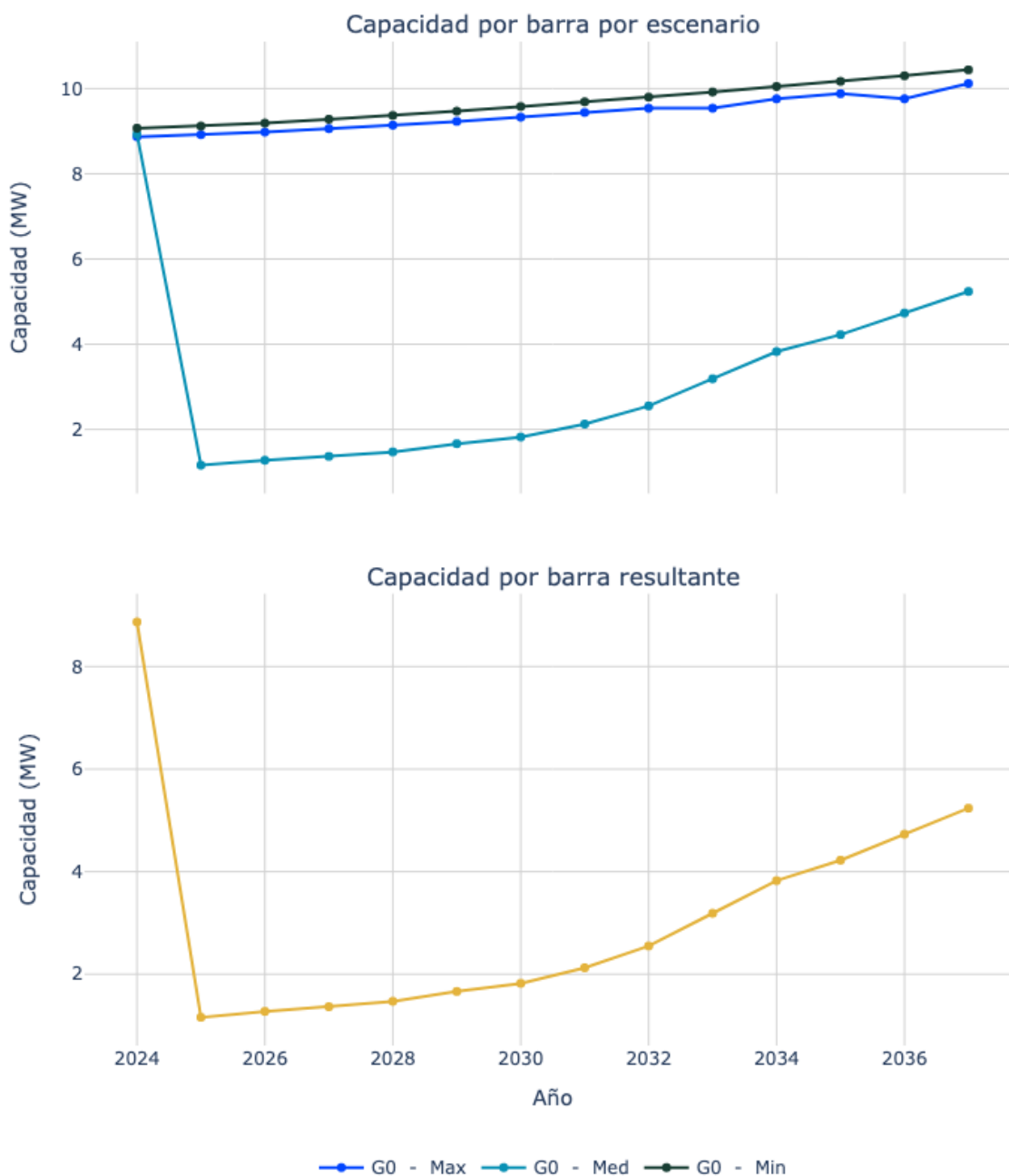
Figura 142. Capacidad de transporte de la subestación Valencia 13.8.
