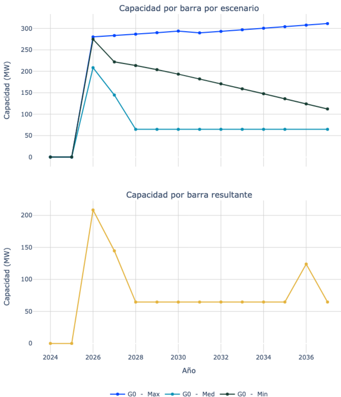
Figura 29. Capacidad de transporte de la subestación Bureche 110.
