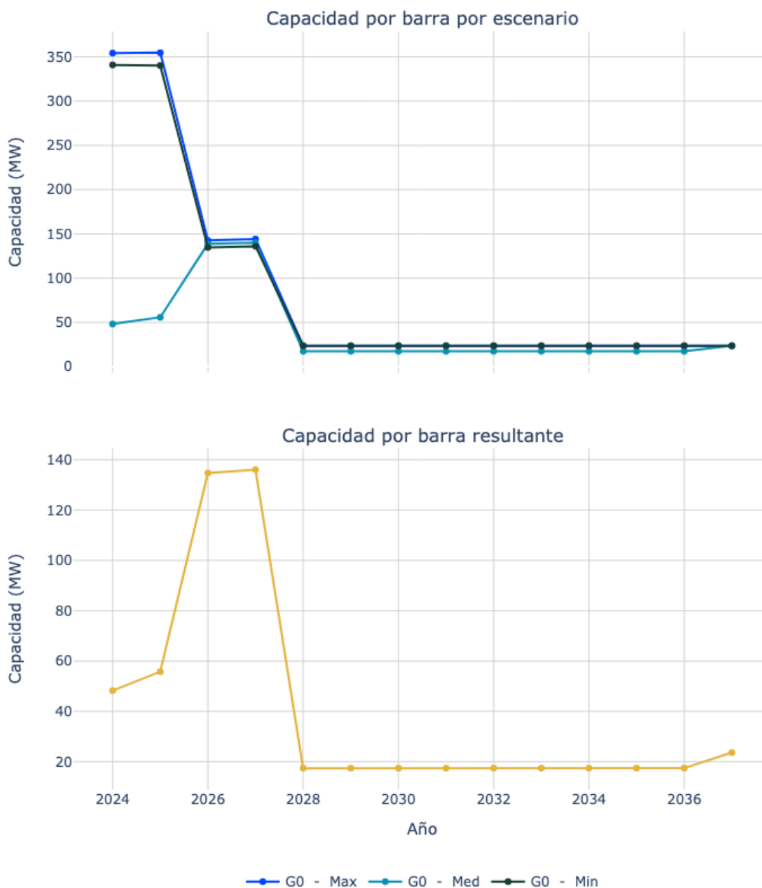
Figura 69. Capacidad de transporte de la subestación GAIRA 1 34.5 kV.
