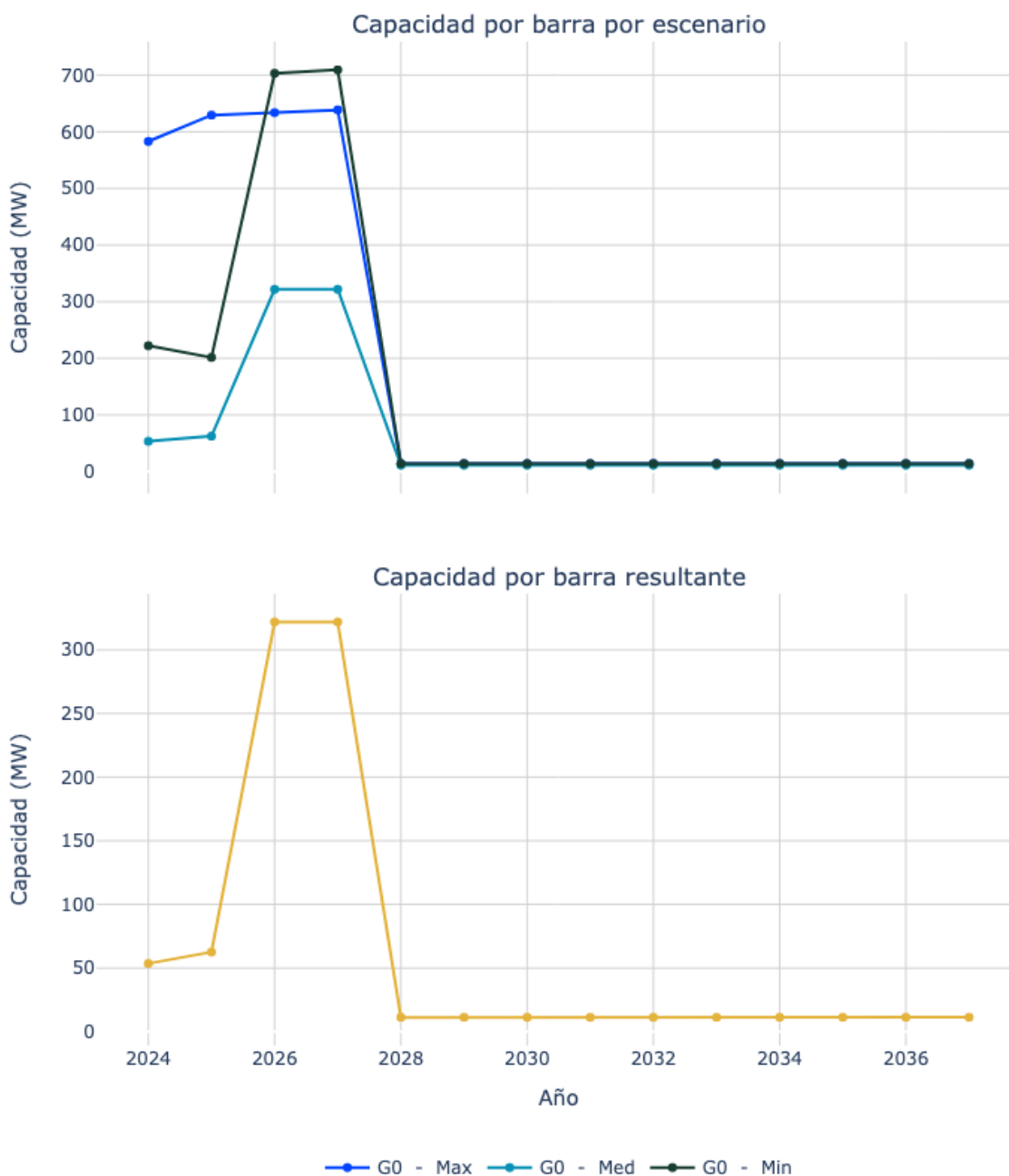
Figura 149. Capacidad de transporte de la subestación Valledupar34.5_B2.
