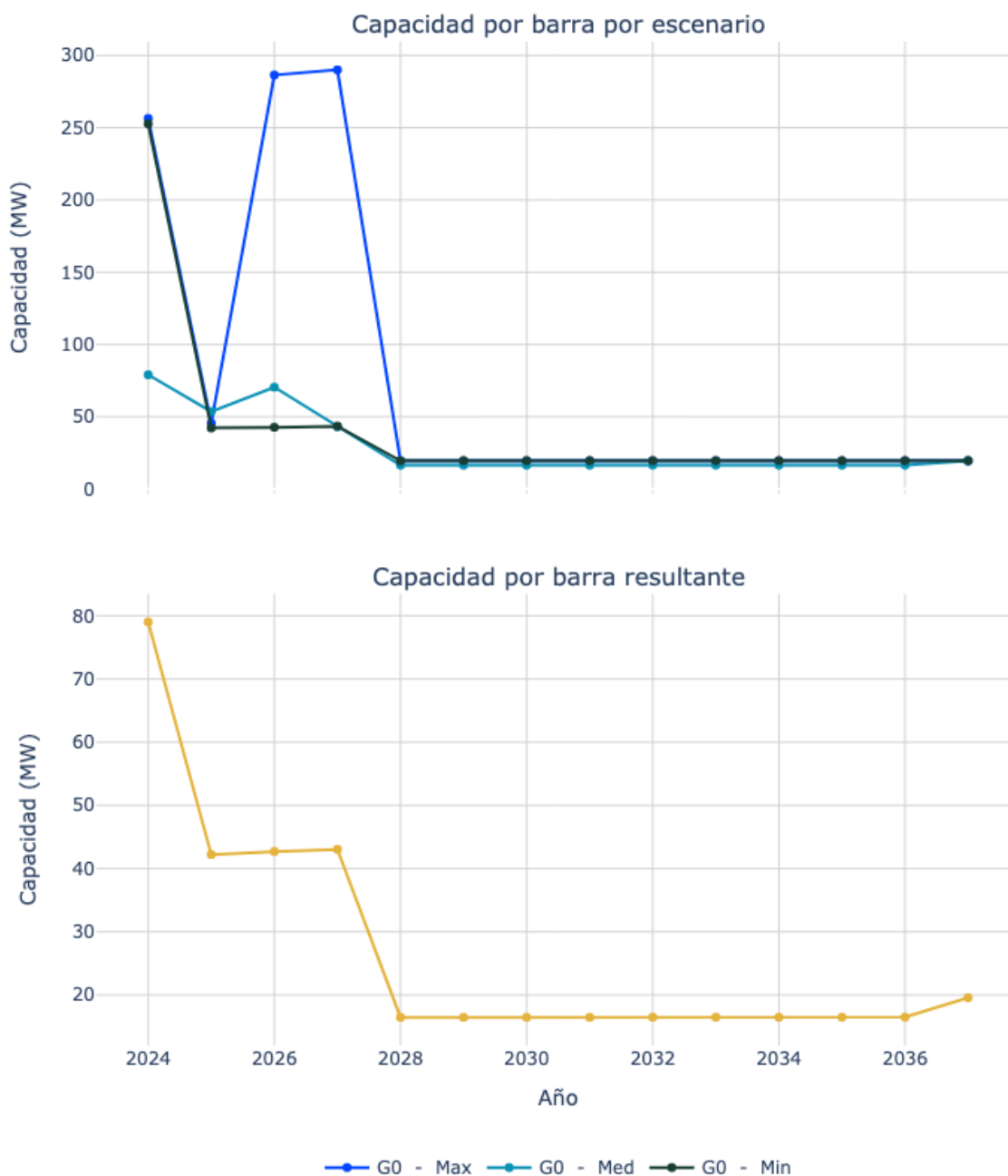
Figura 116. Capacidad de transporte de la subestación RIOHACHA 2 13.8 kV.
