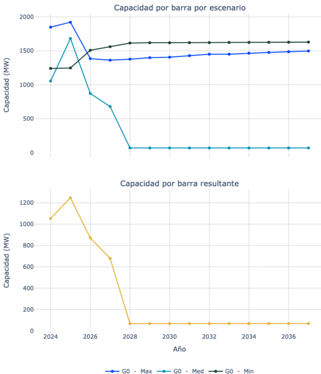
Figura 67. Capacidad de transporte de la subestación Fundacion 220.
