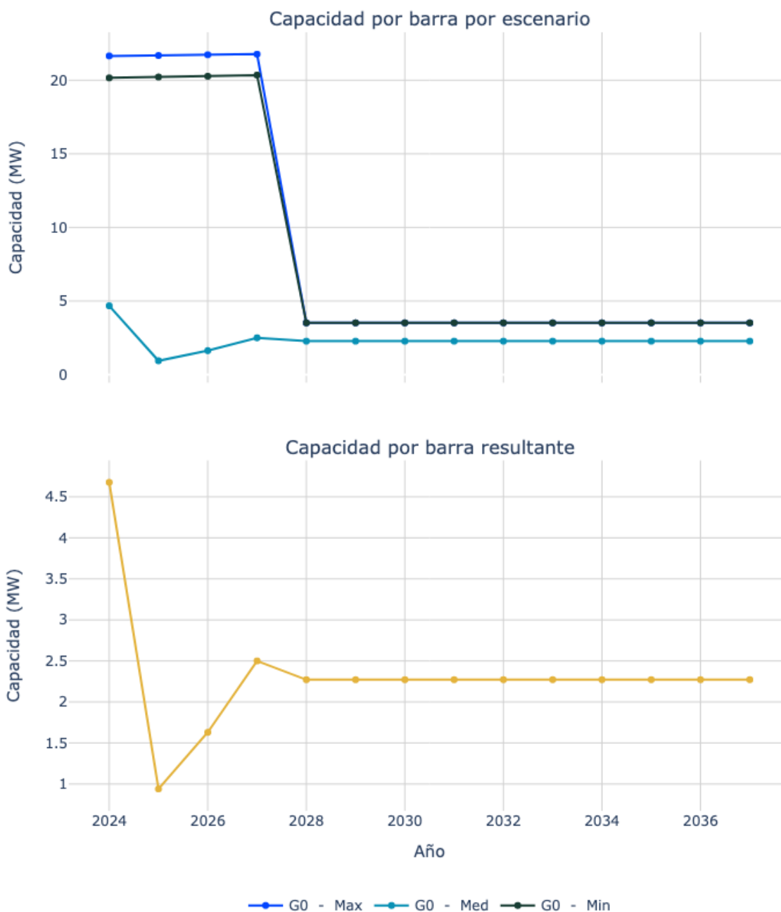
Figura 94. Capacidad de transporte de la subestación Loma del balsamo 34.5.
