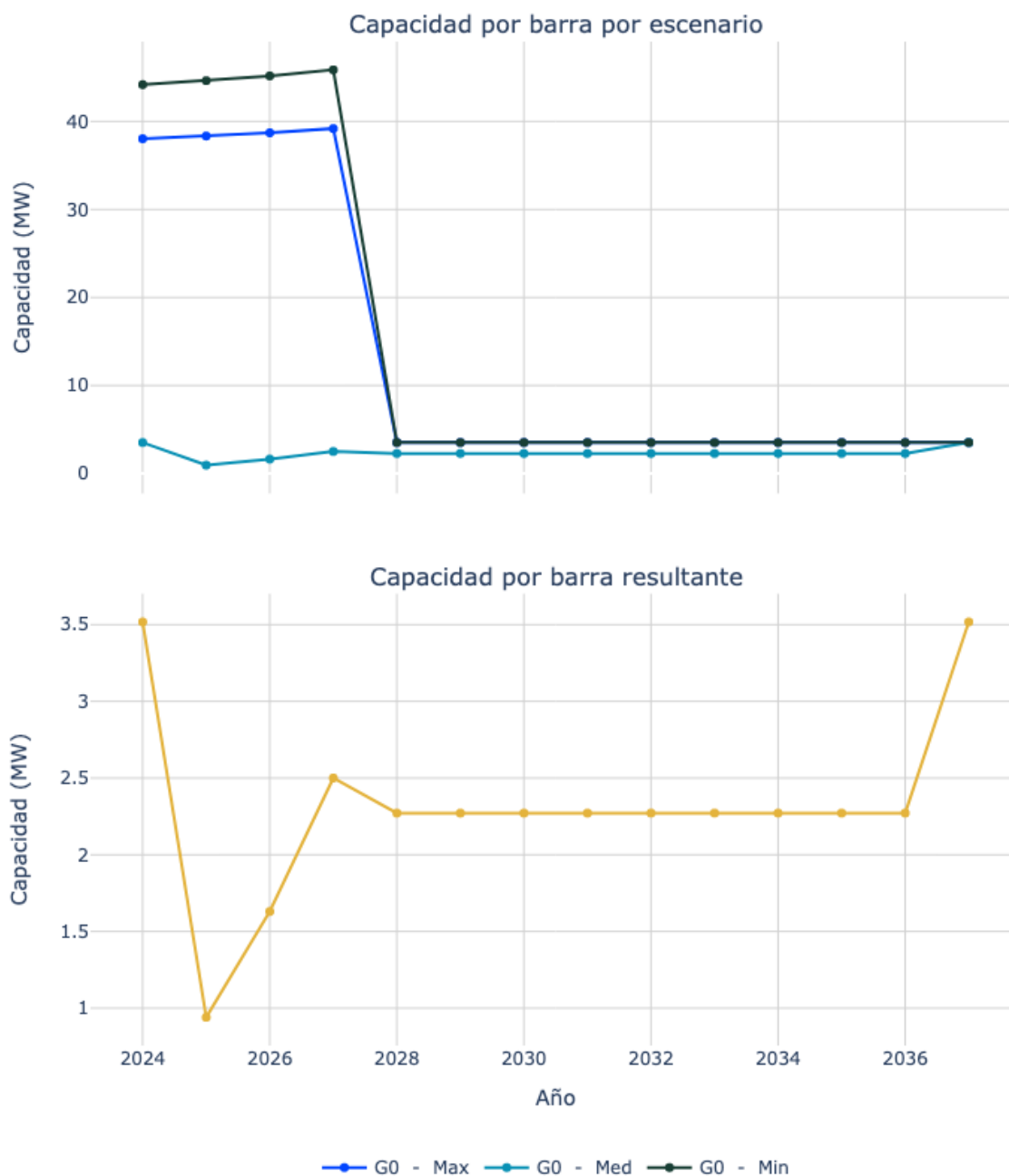
Figura 28. Capacidad de transporte de la subestación Bosconia 34.5.
