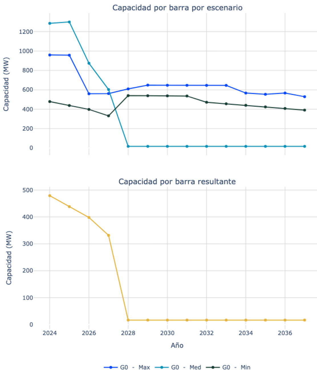
Figura 42. Capacidad de transporte de la subestación Copey 110.
