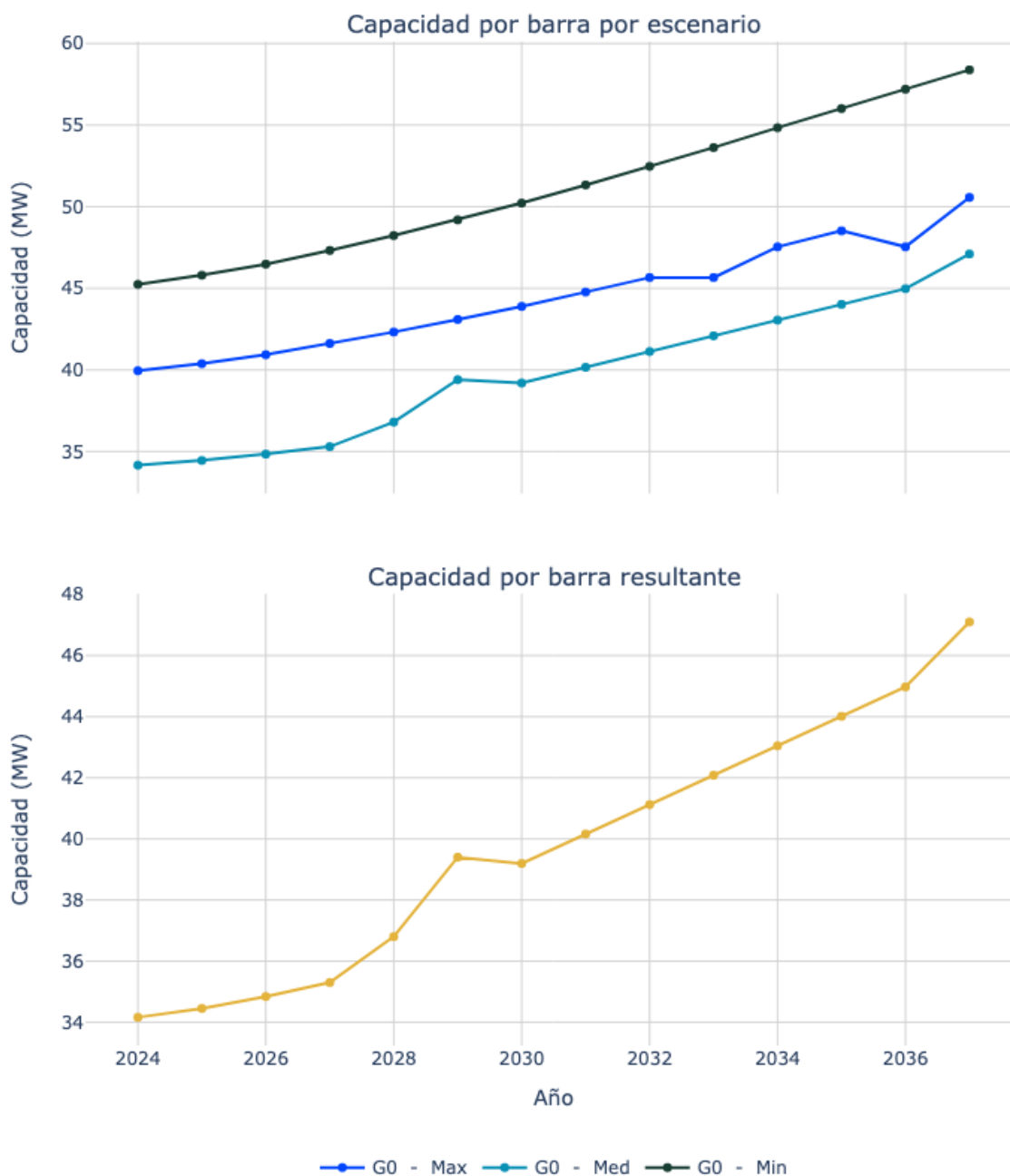
Figura 104. Capacidad de transporte de la subestación Mata de caña 34.5.
