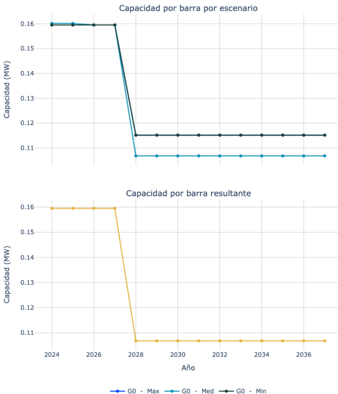
Figura 19. Capacidad de transporte de la subestación Astrea 34.5.
