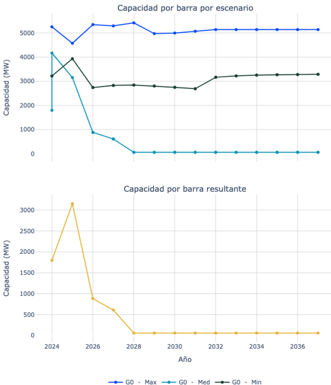
Figura 57. Capacidad de transporte de la subestación El Copey 500.
